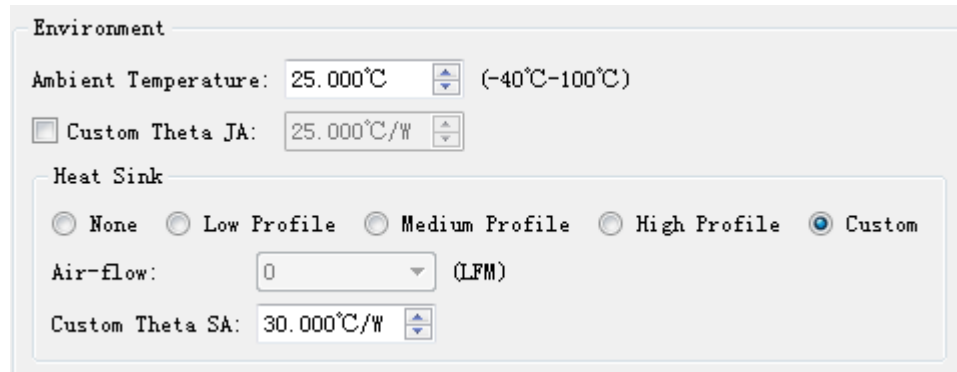
图 3-10 用户指定热阻抗 \theta_{SA}
