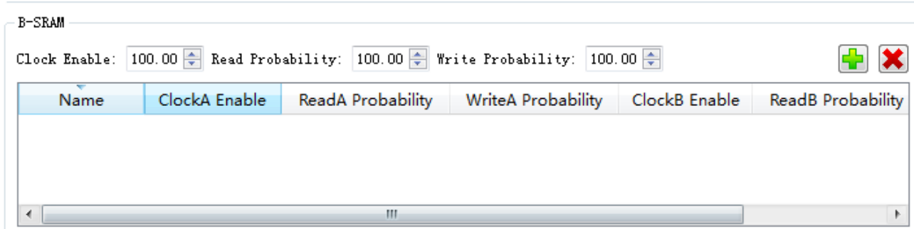
图 3-28 B-SRAM 配置区
