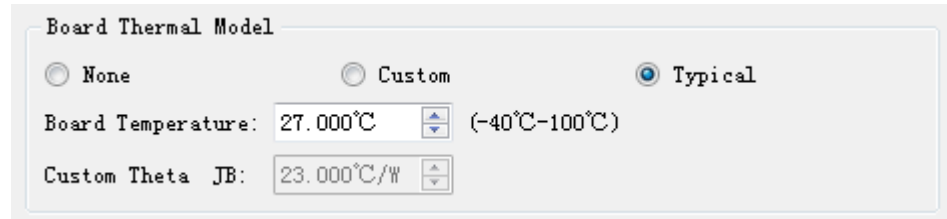
图 3-12 设置电路板散热模式决定热阻抗 \theta_{JB}
