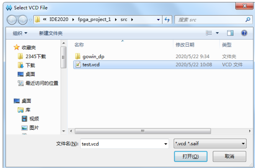
图 3-21 Select VCD File 对话框
