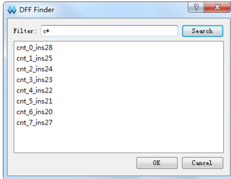
图 3-39 DFF Finder 对话框
