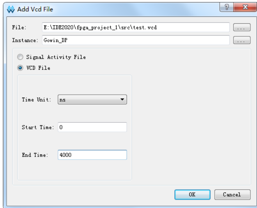
图 3-23 设置波形文件起止时间
