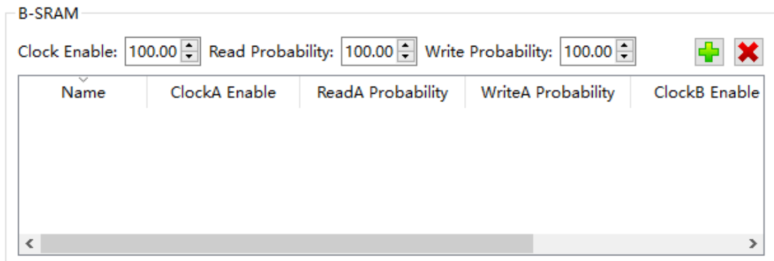
图 3-31 BSRAM 配置区
