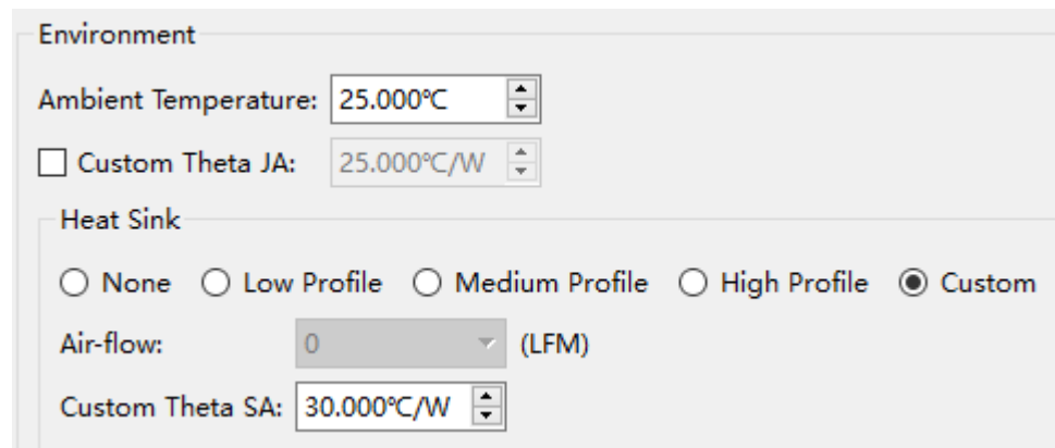
图 3-9 用户指定热阻抗 \theta_{SA}
