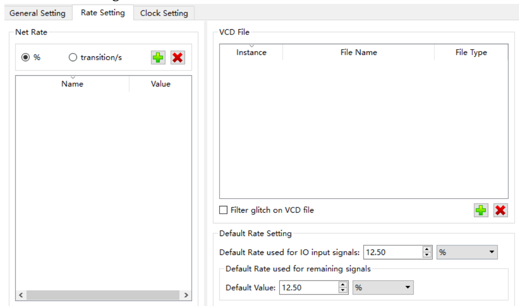
图 3-6 Rate Setting 窗口
