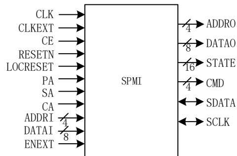
图 9-1SPMI 结构框图
