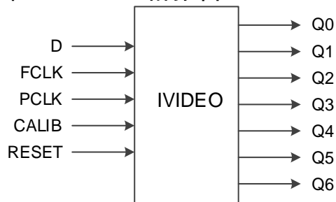
图 1-21 IVIDEO 结构框图
