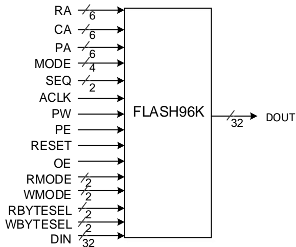
图 7-1 FLASH96K 结构框图
