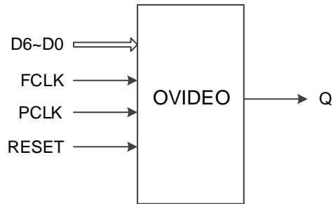
图 1-26 OVIDEO 结构框图
