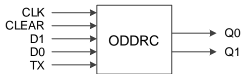
图 1-17 ODDRC 结构框图
