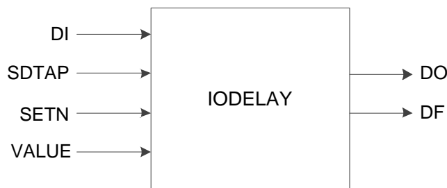
图 1-34 IODELAY 结构框图
