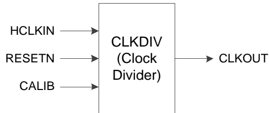
图 6-4 CLKDIV 结构框图
