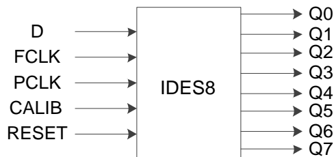
图 1-19 IDES8 结构框图
