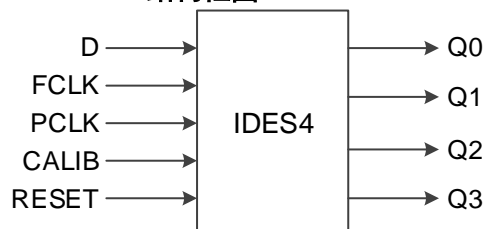
图 1-18 IDES4 结构框图
