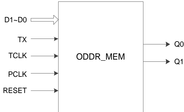
图 1-29 ODDR_MEM 结构框图
