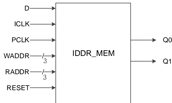
图 1-28 IDDR_MEM 结构框图
