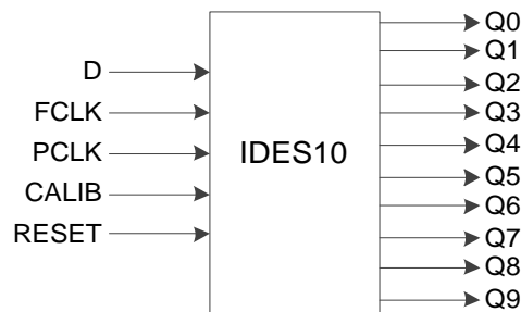
图 1-20 IDES10 结构框图
