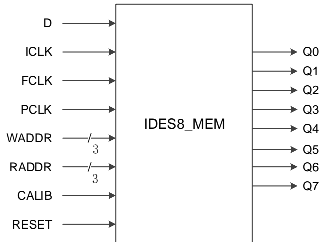
图 1-32 IDES8_MEM 结构框图
