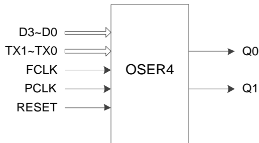
图 1-23 OSER4 结构框图
