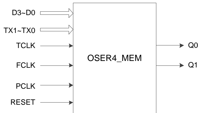
图 1-31 OSER4_MEM 结构框图
