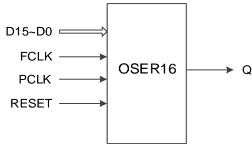
图 1-27 OSER16 结构框图
