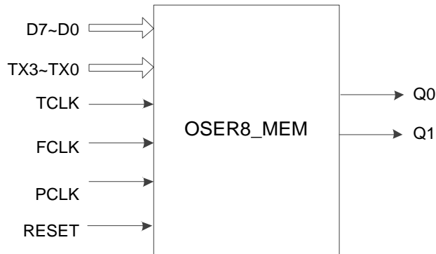
图 1-33 OSER8_MEM 结构框图
