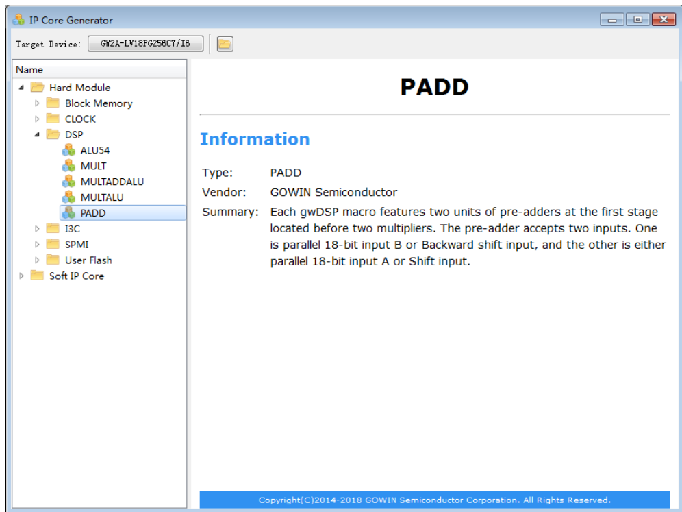
图 3-64 PADD 信息概要
