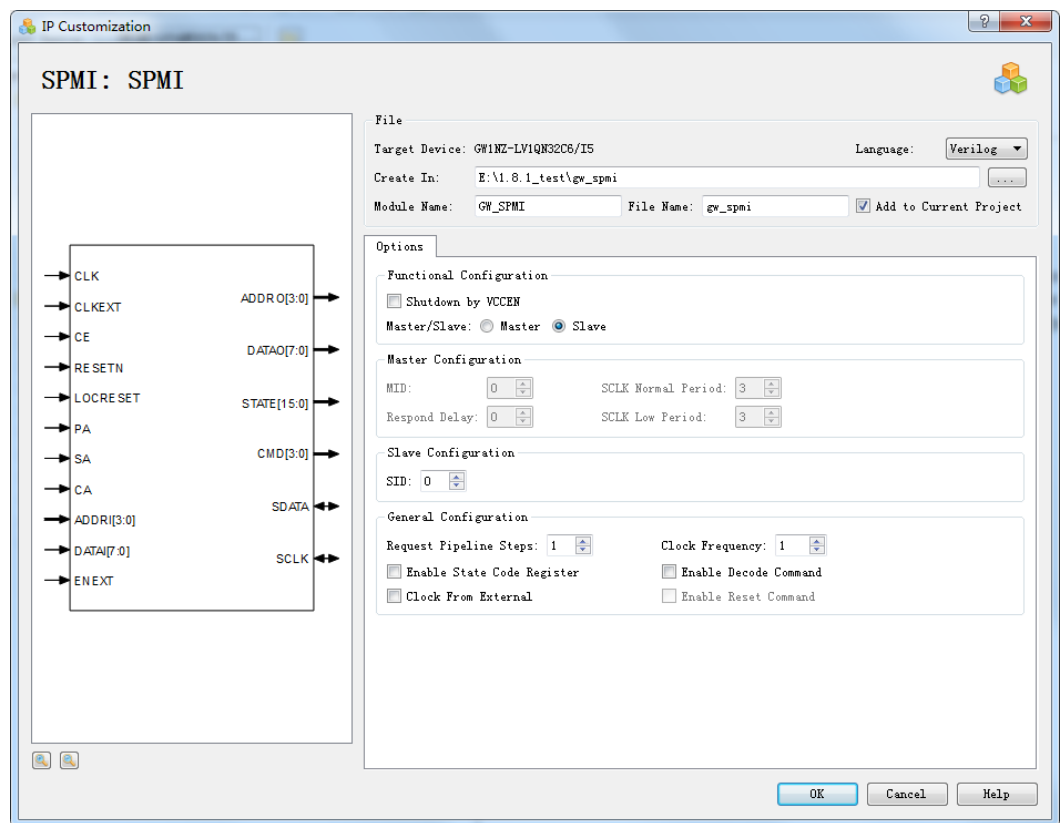
图 3-115 配置的 IP Customization
