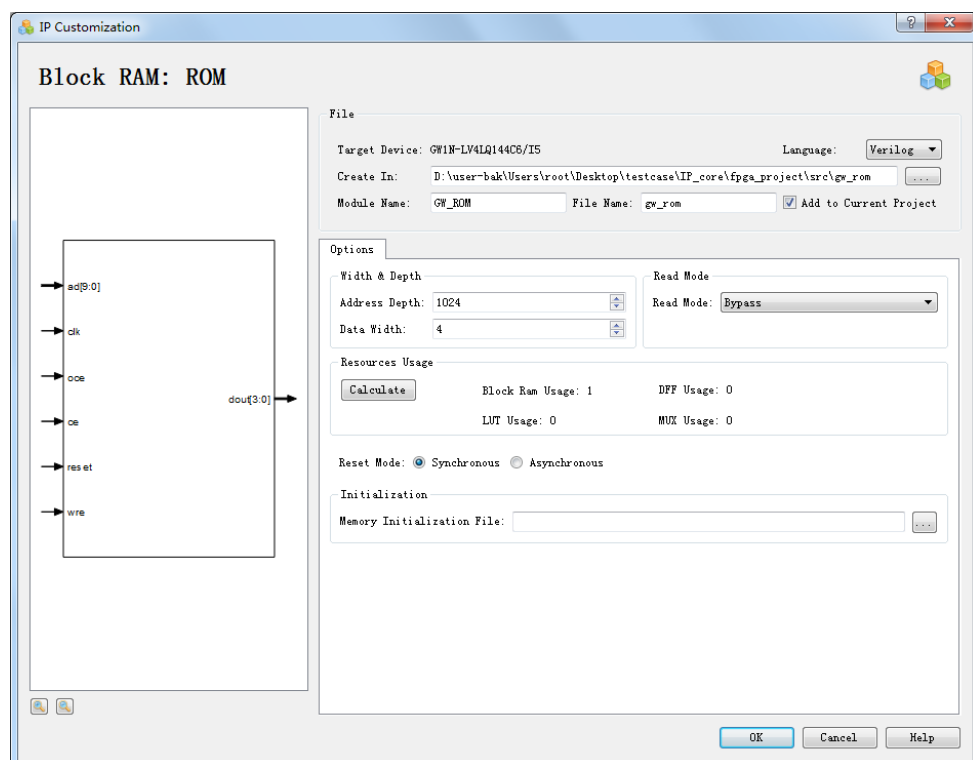
图 3-31 配置的 IP Customization
