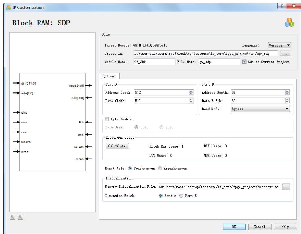
图 3-27 SDP 的 IP Customization 设置
