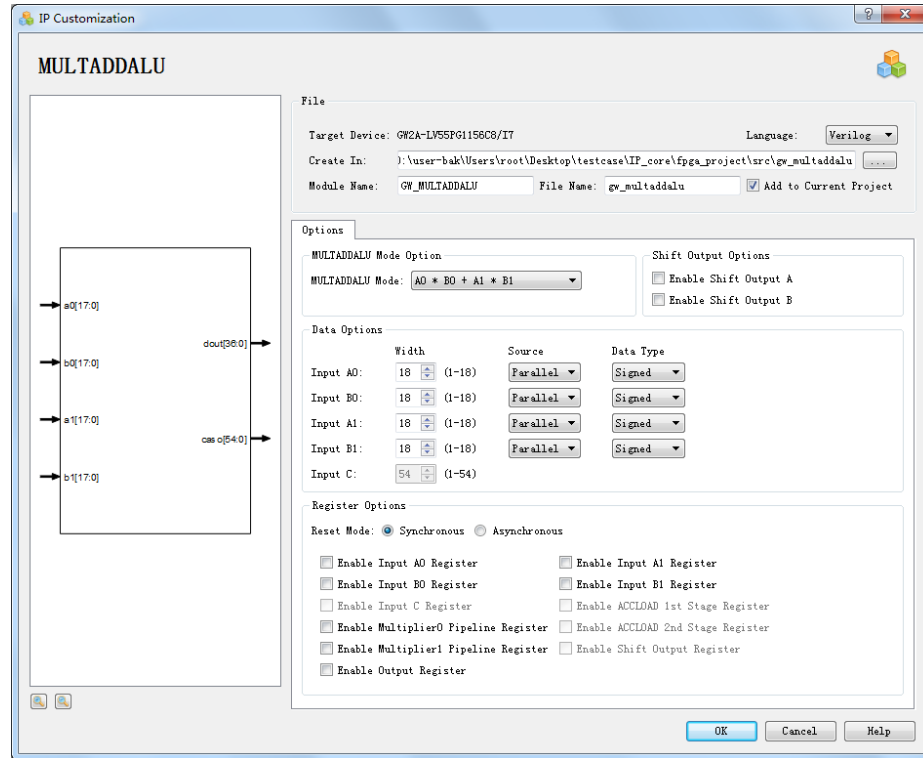
图 3-56 MULTADDALU IP Customization 设置
