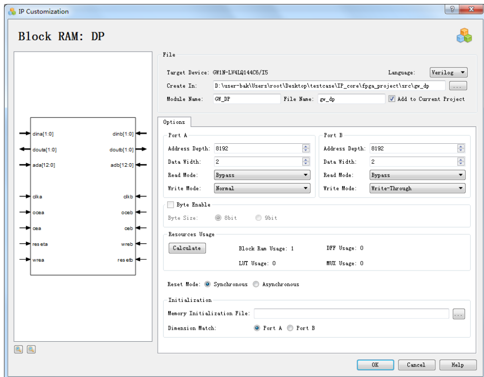
图 3-19 DP IP Customization 设置
