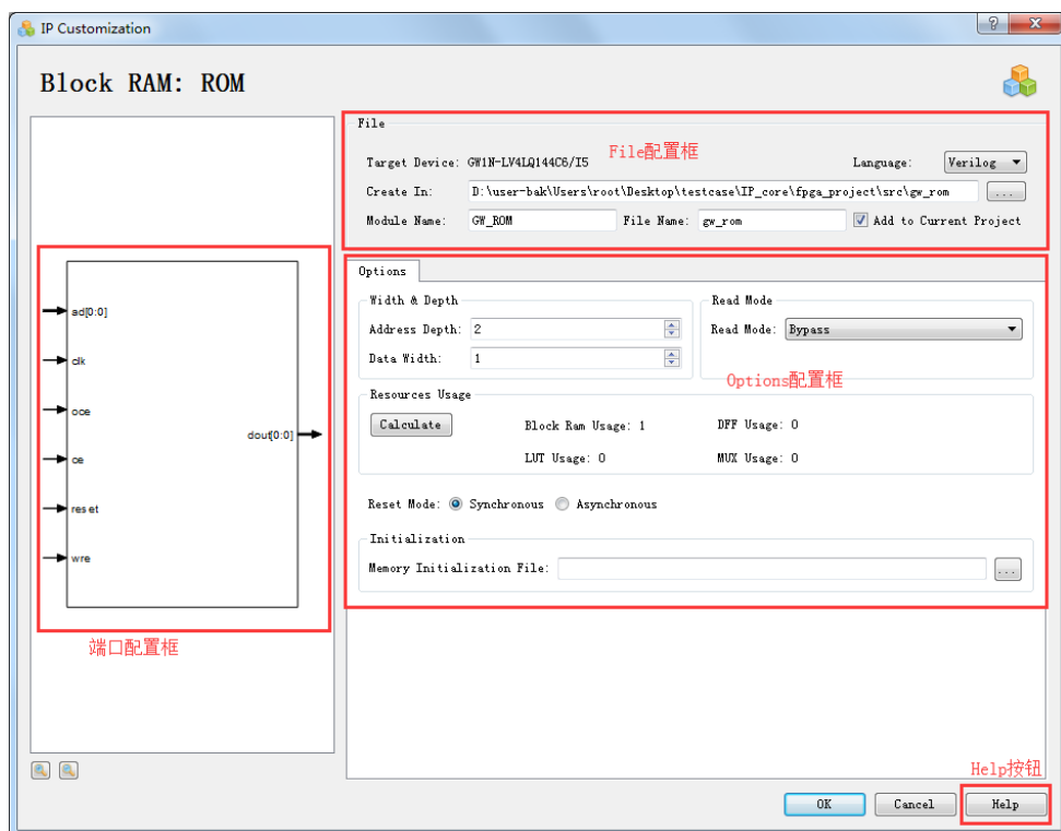
图 3-29 ROM 的 IP Customization 窗口结构
