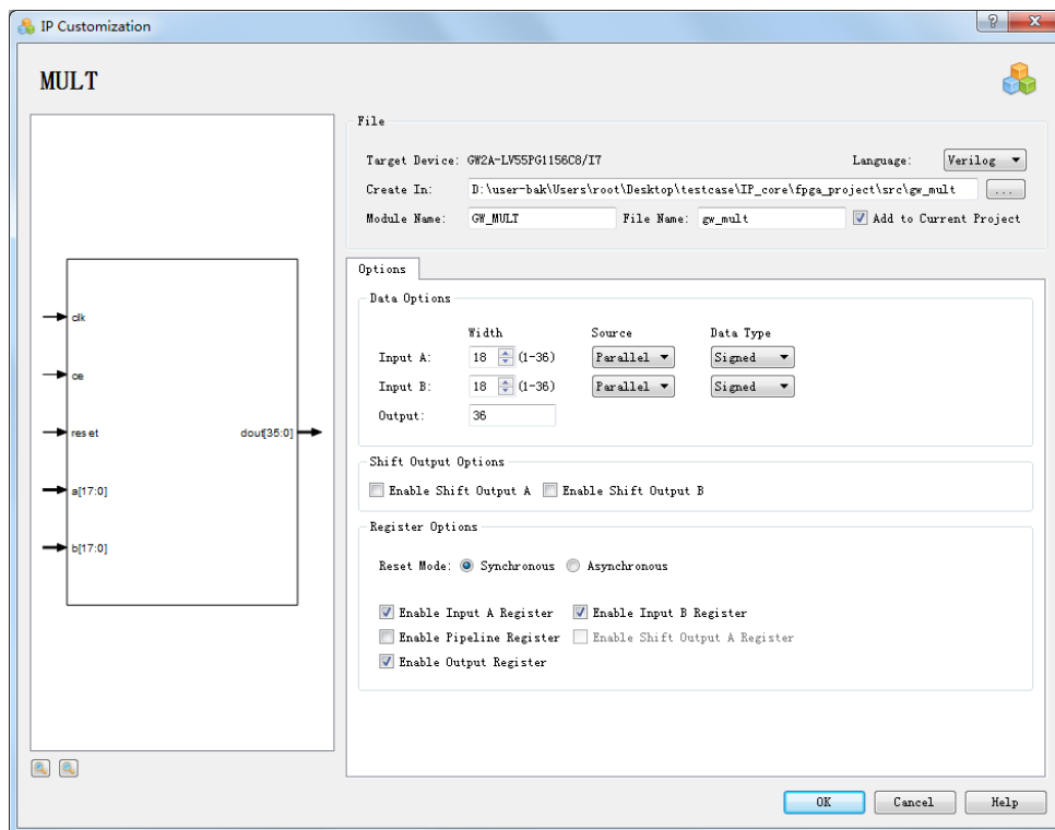
图 3-46 配置的 IP Customization
