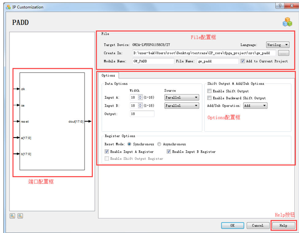
图 3-65 PADD 的 IP Customization 窗口结构
