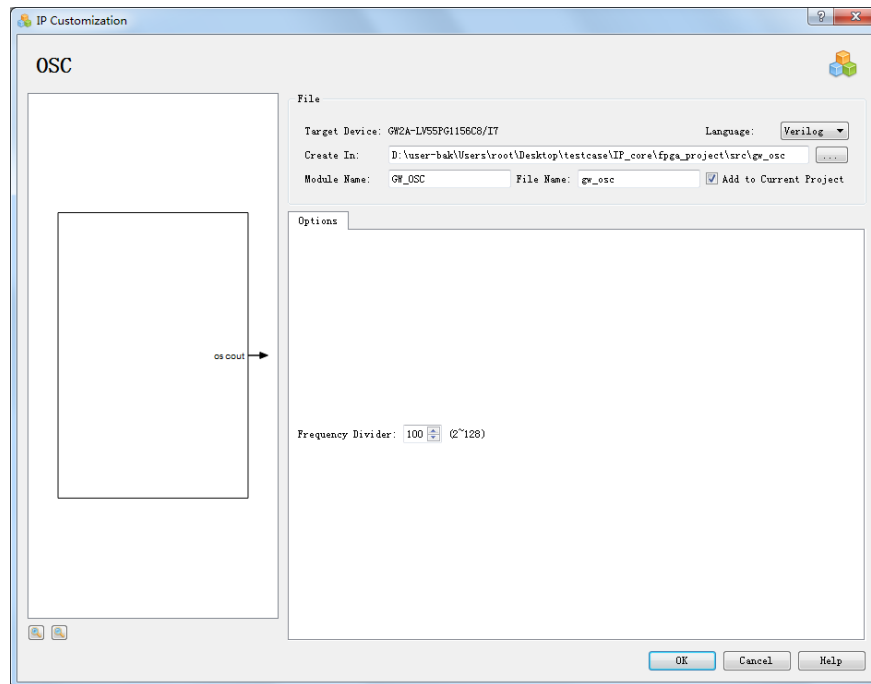
图 3-97 OSC IP Customization 设置
