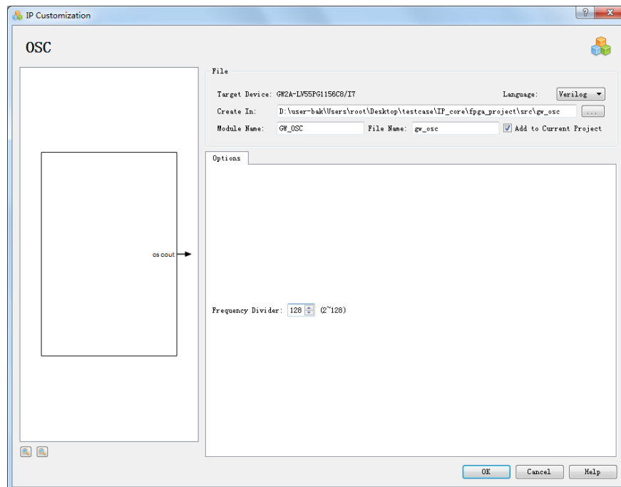
图 3-94 配置的 IP Customization
