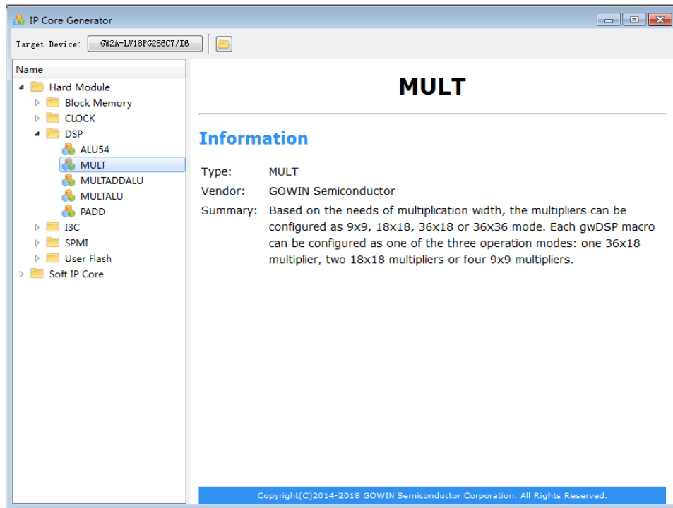
图 3-43 MULT 的信息概要
