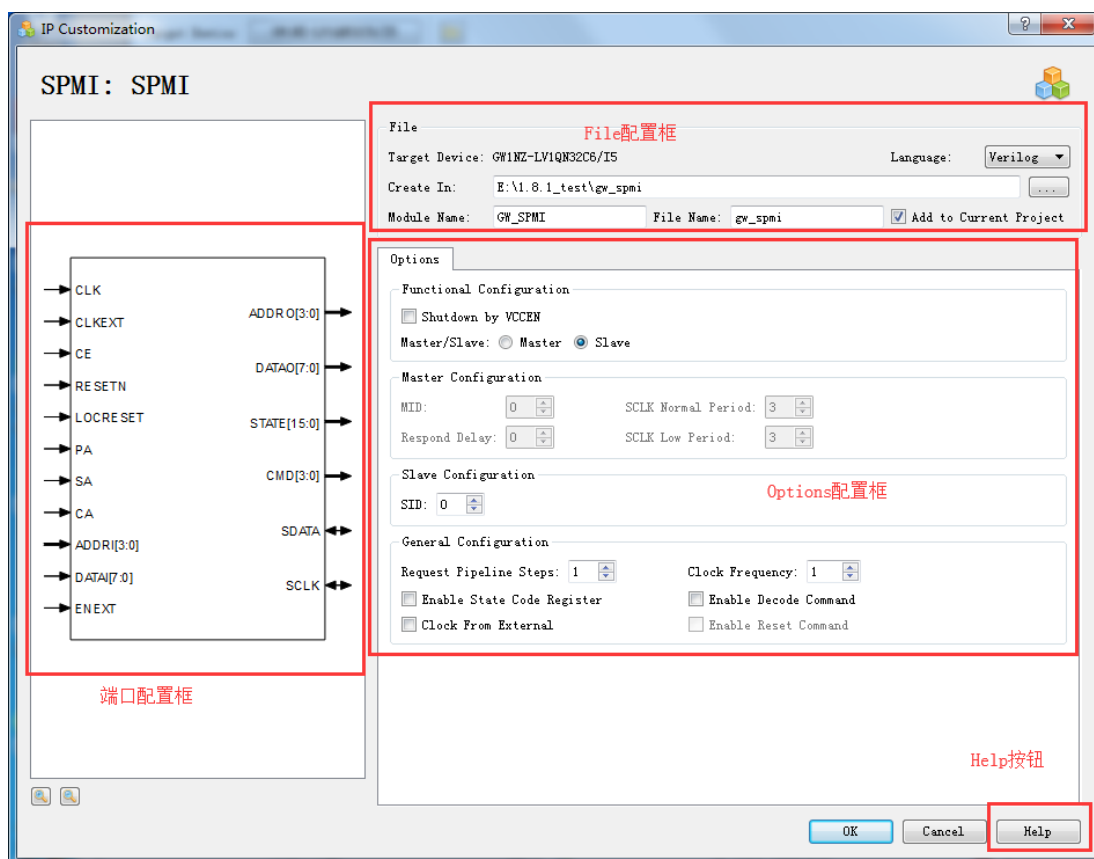
图 3-113 SPMI 的 IP Customization 窗口结构
