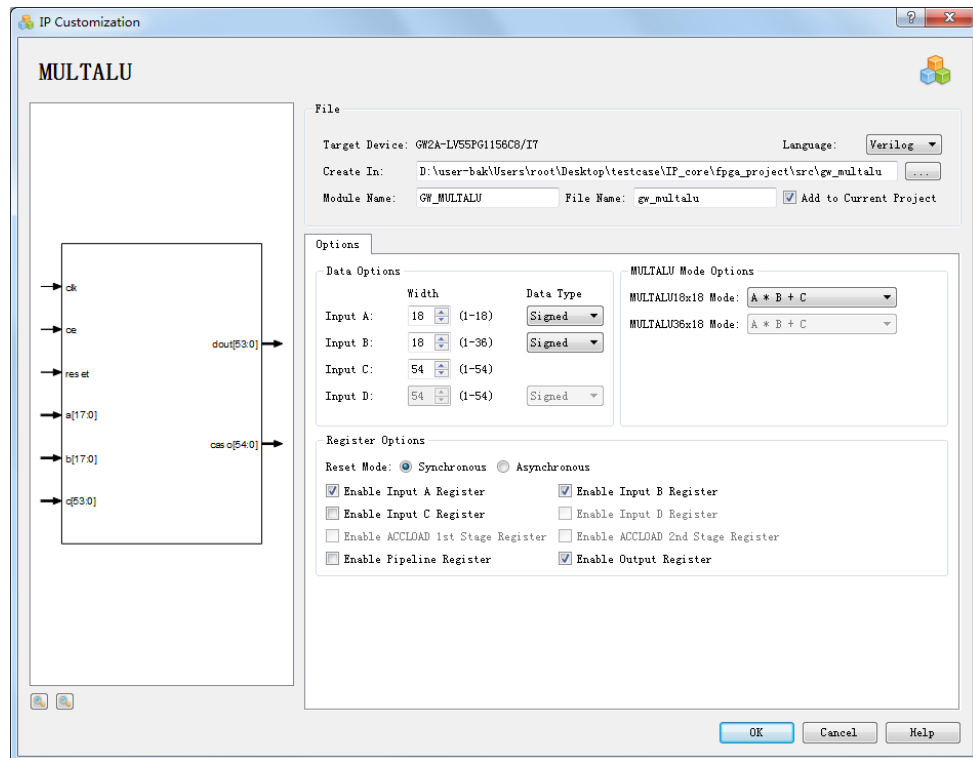
图 3-60 配置的 IP Customization
