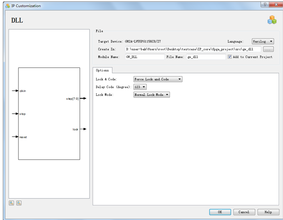
图 3-87 配置的 IP Customization
