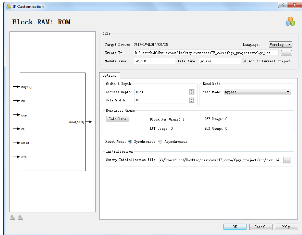
图 3-34 ROM 的 IP Customization 设置
