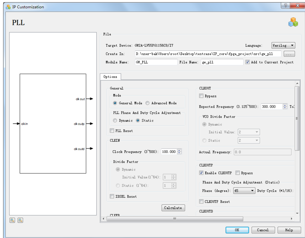
图 3-83 PLL IP Customization 设置
