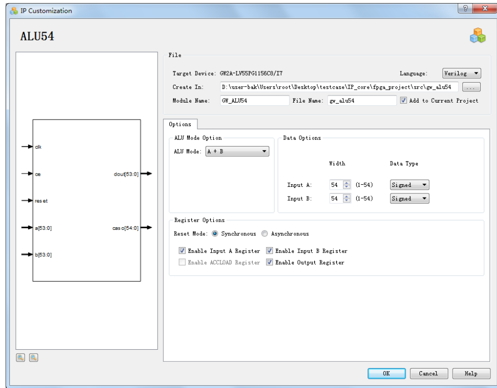
图 3-42 ALU54 IP Customization 设置
