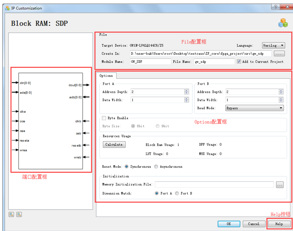
图 3-21 SDP 的 IP Customization 窗口结构
