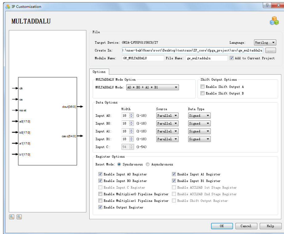
图 3-53 配置的 IP Customization
