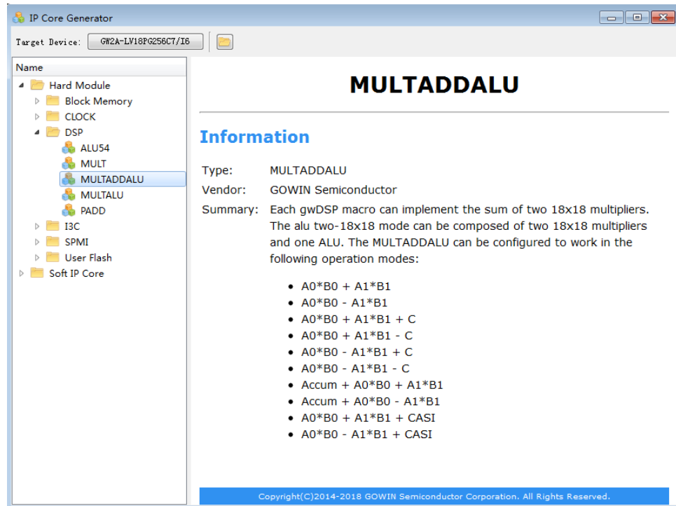
图 3-50 MULTADDALU 的信息概要
