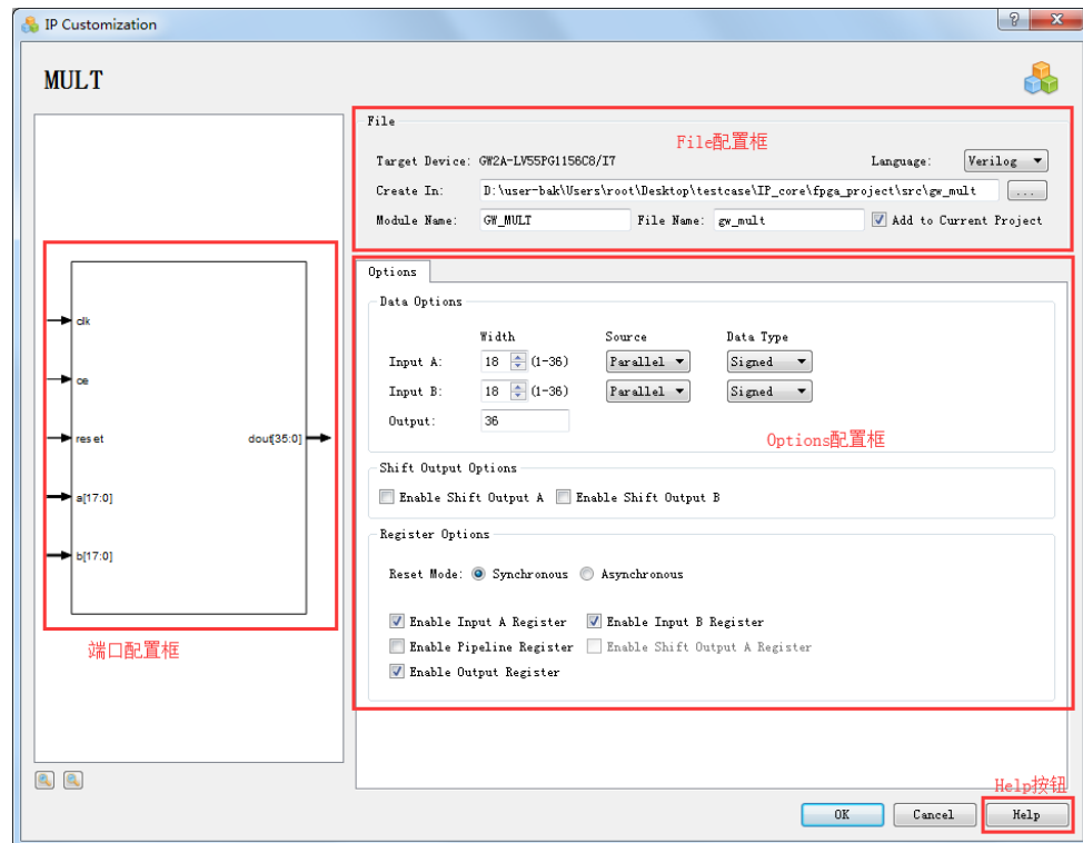
图 3-44 MULT 的 IP Customization 窗口结构
