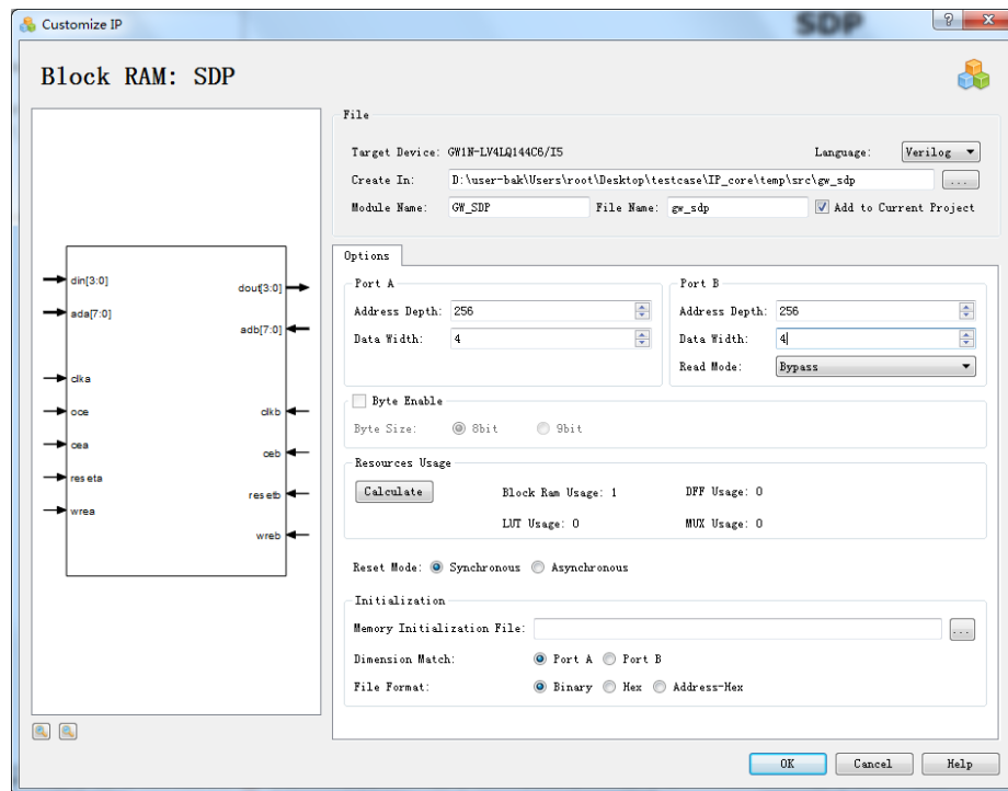
图 3-24 配置的 IP Customization
