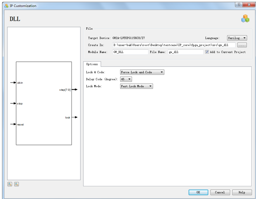
图 3-90 DLL IP Customization 设置
