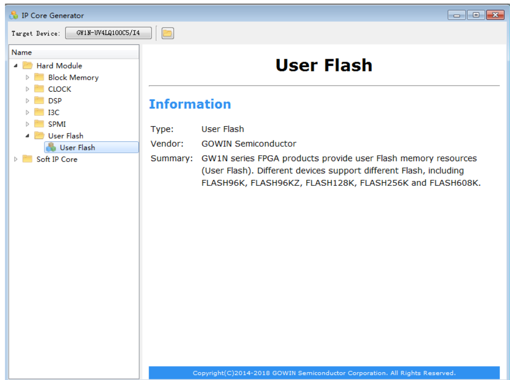
图 3-98 User Flash 的信息概要
