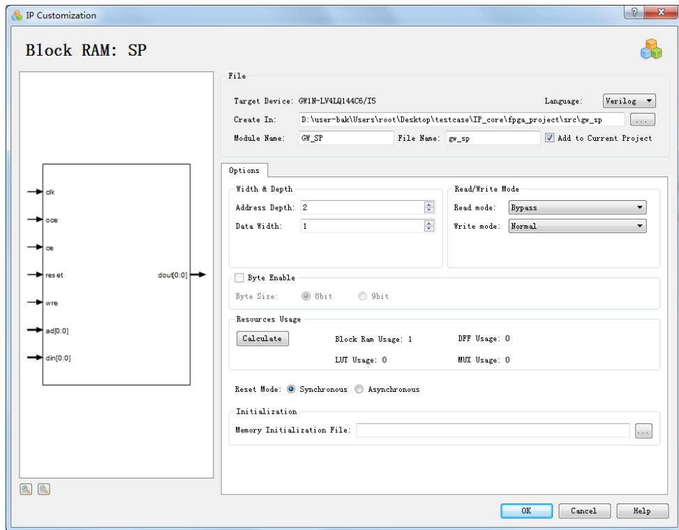
图 3-3 IP Customization 窗口
