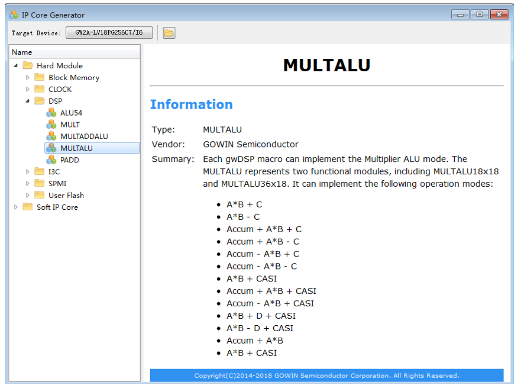
图 3-57 MULTALU 的信息概要
