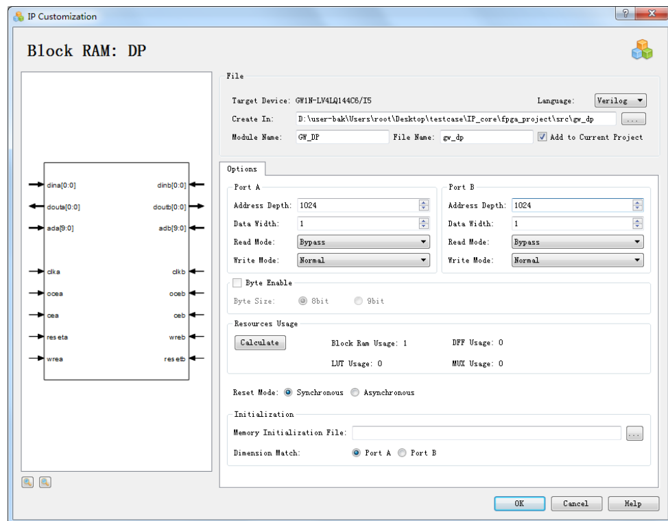
图 3-16 配置的 IP Customization
