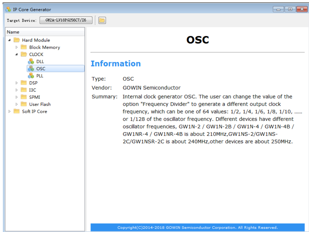
图 3-91 OSC 的信息概要
