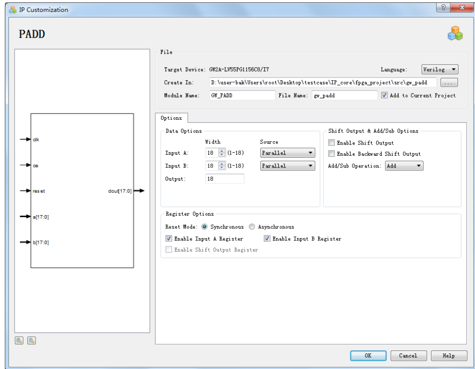
图 3-70 PADD IP Customization 设置
