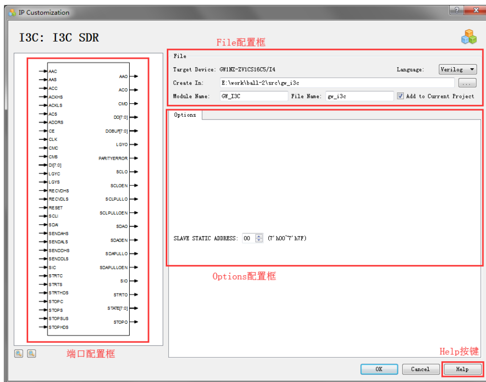
图 3-106 I3C 的 IP Customization 窗口结构
