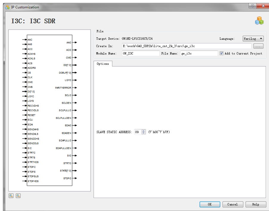
图 3-108 配置的 IP Customization
