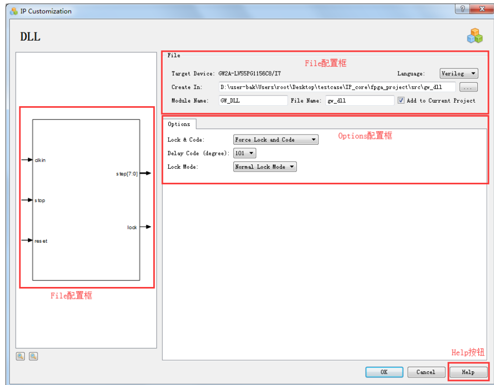
图 3-85 DLL 的 IP Customization 窗口结构
