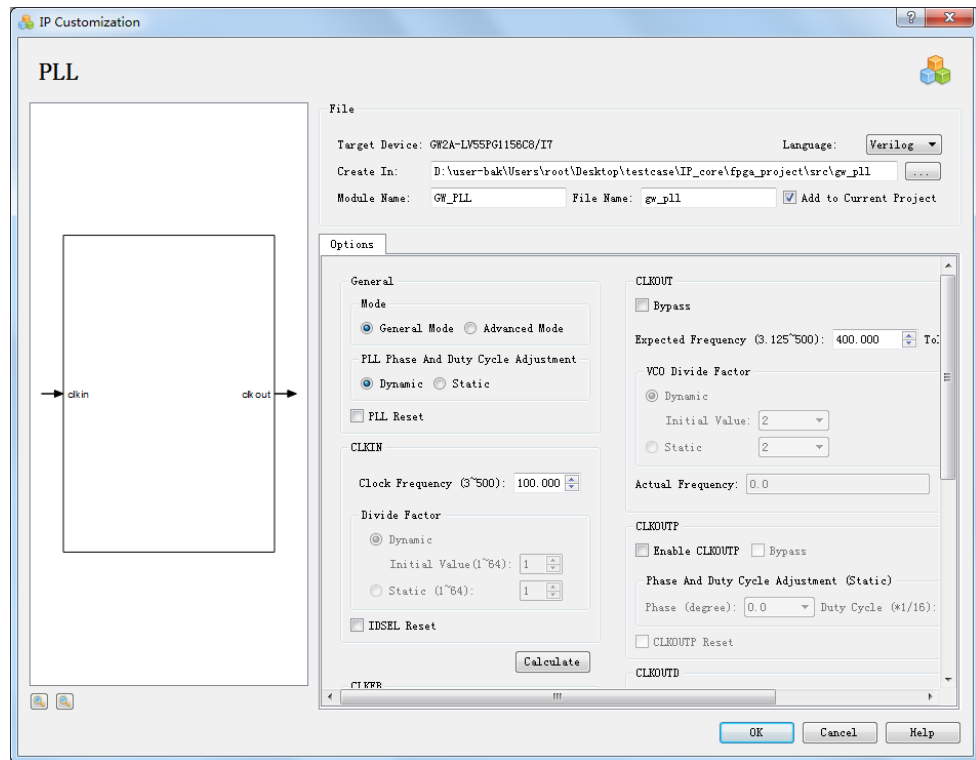
图 3-80 配置的 IP Customization
