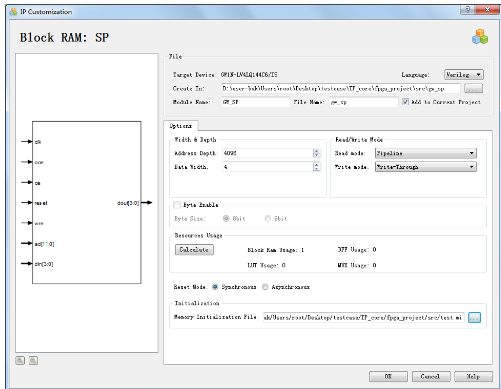
图 3-11 SP IP Customization 设置
