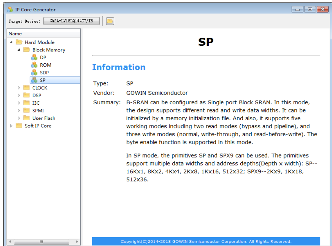
图 3-4 SP 的信息概要
