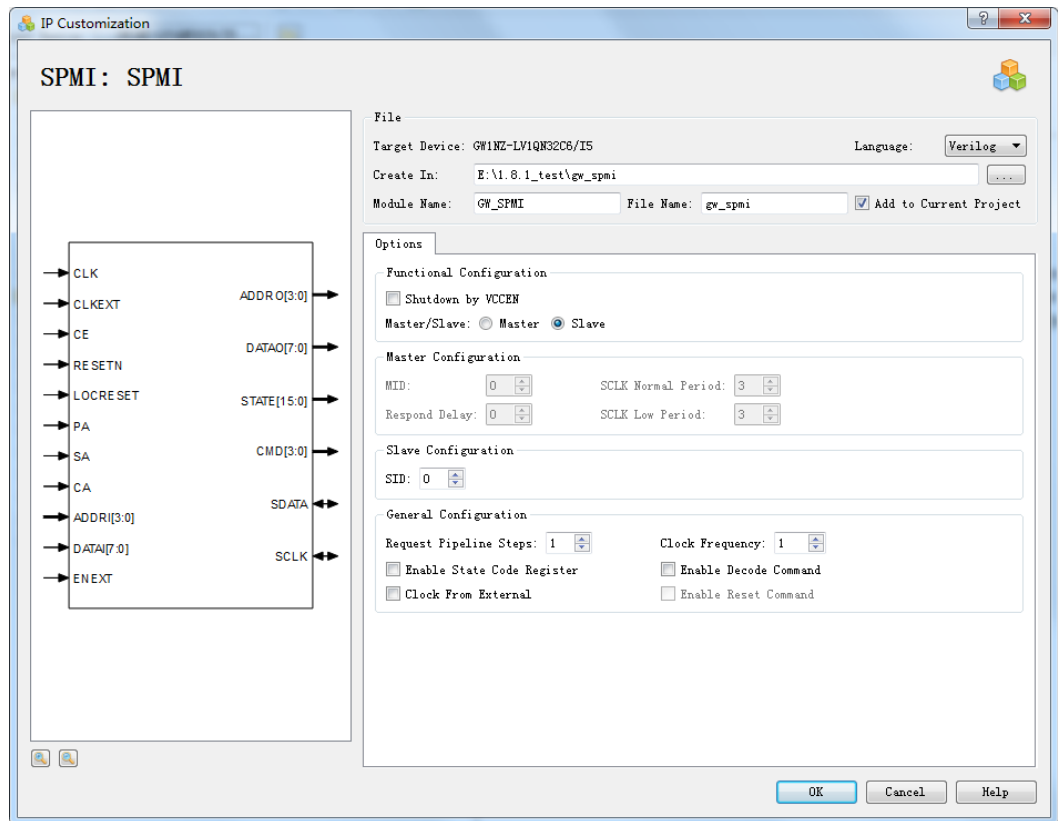
图 3-118 SPMI IP Customization 设置
