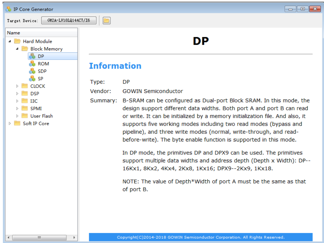
图 3-12 DP 的信息概要
