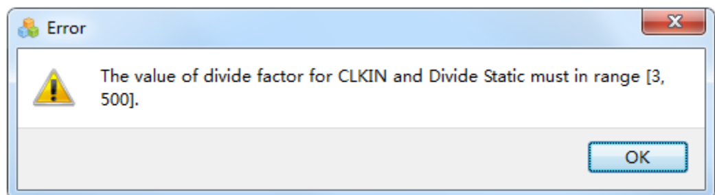
图 3-76 CLKIN Divide Factor 配置不合理的 error 窗口
