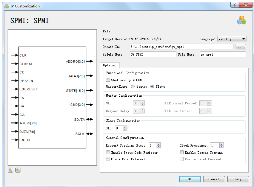
图 3-118 配置的 IP Customization
