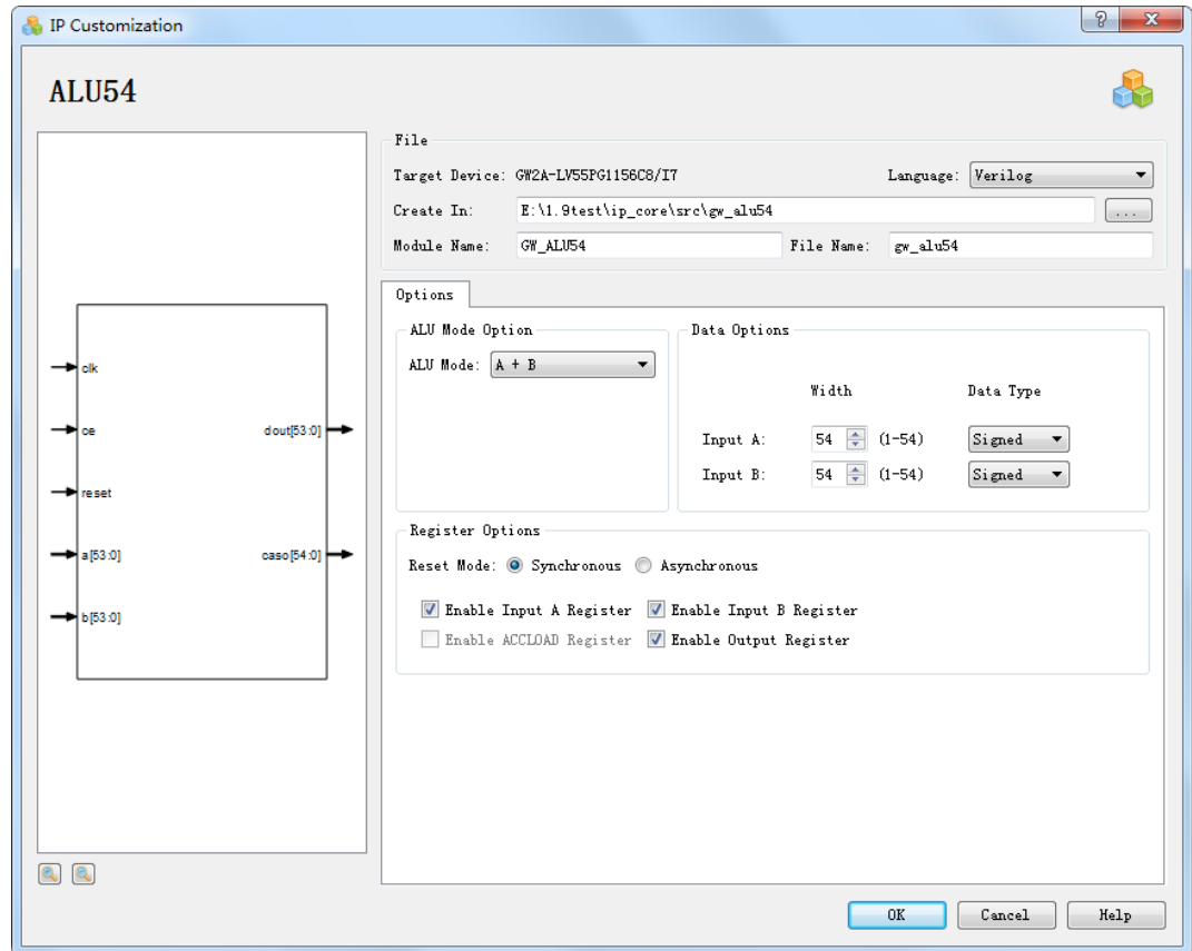
图 3-44 ALU54 IP Customization 设置
