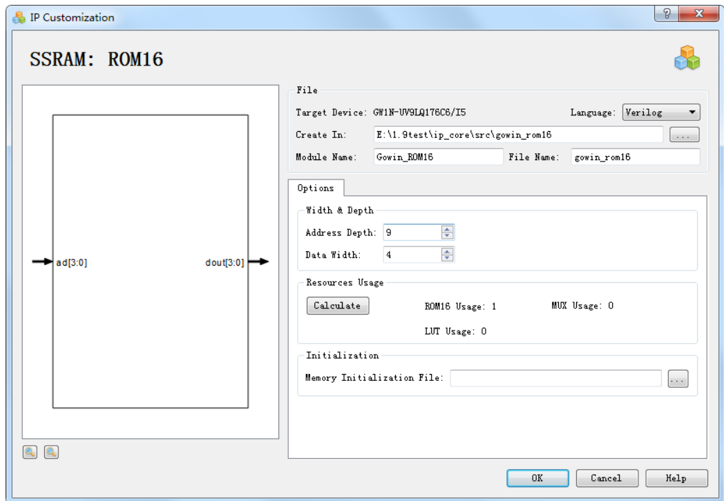
图 3-139 配置的 IP Customization
