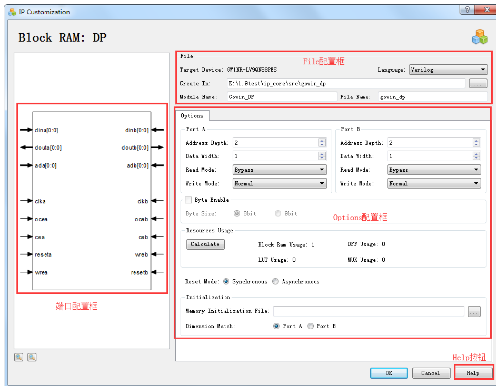
图 3-15 DP 的 IP Customization 窗口结构
