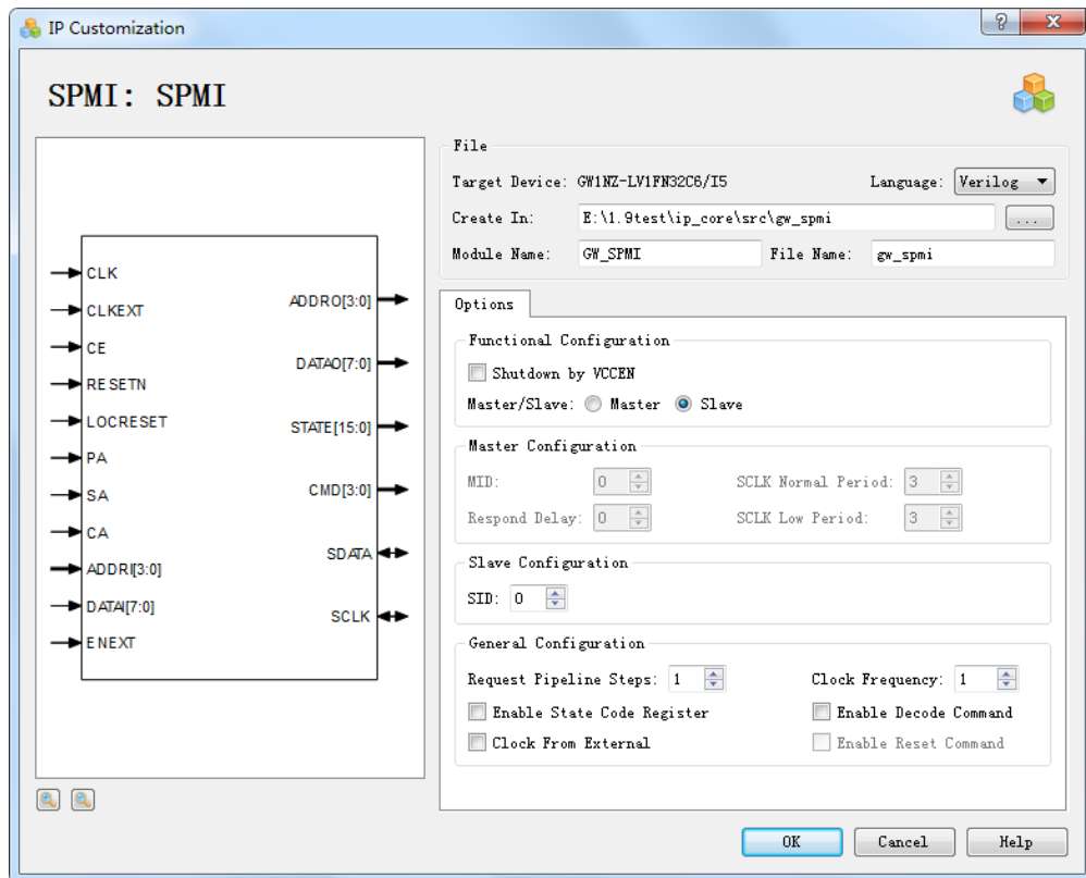
图 3-121 SPMI IP Customization 设置
