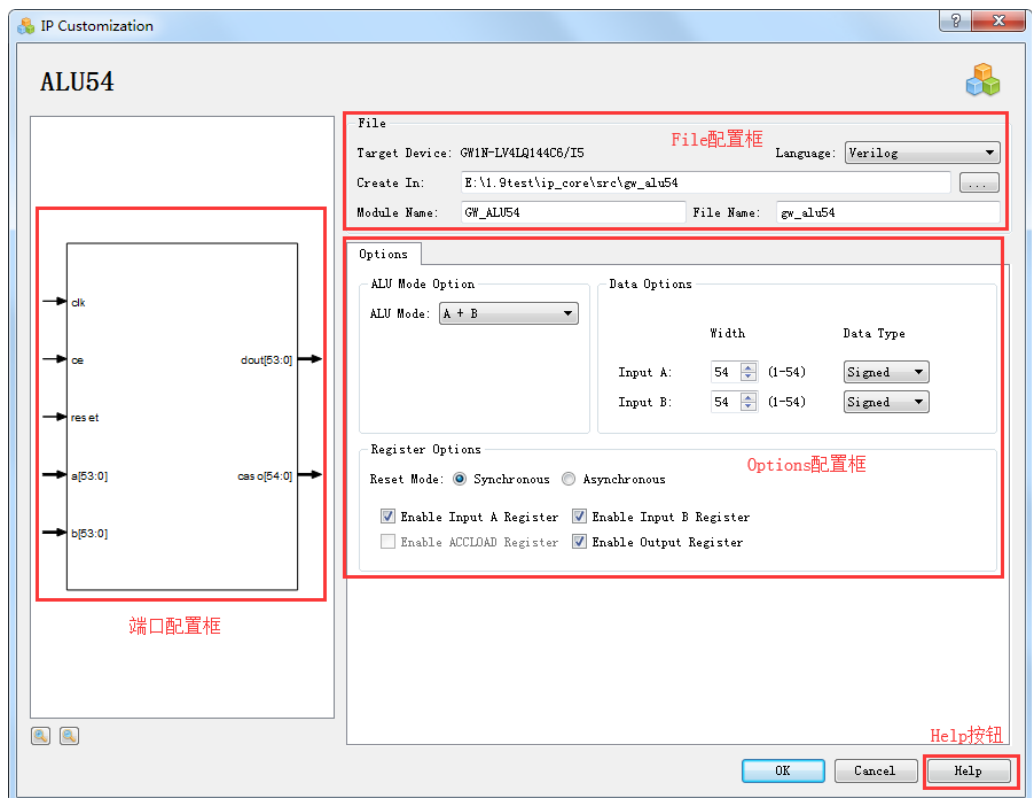
图 3-38 ALU54 的 IP Customization 窗口结构
