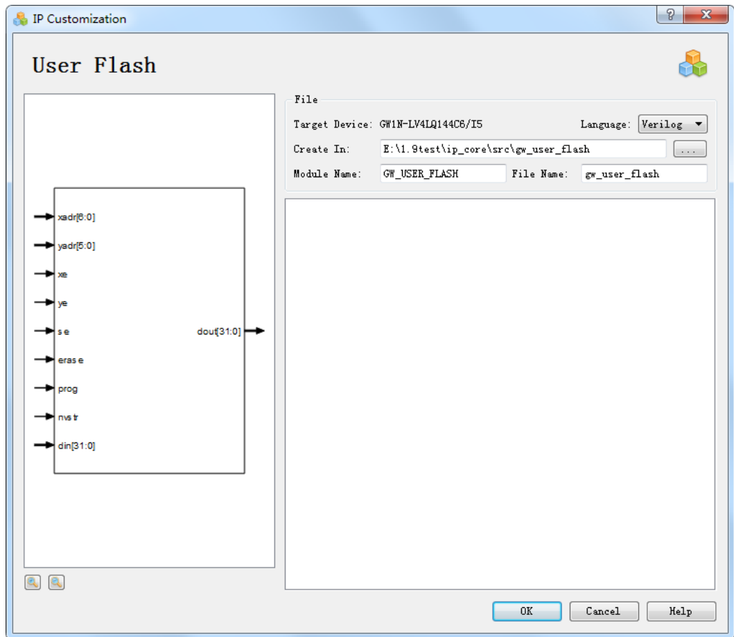
图 3-104 配置的 IP Customization
