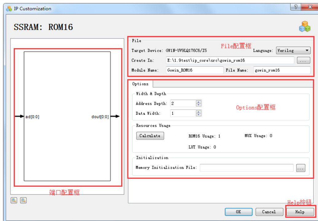
图 3-137 ROM16 的 IP Customization 窗口结构
