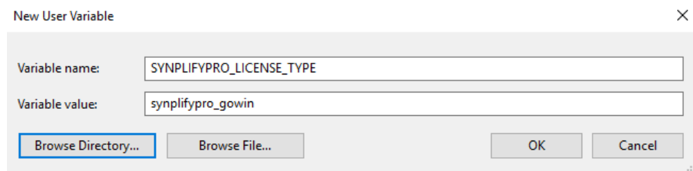
图 4-7 添加 SYNPLIFYPRO_LICENSE_TYPE
