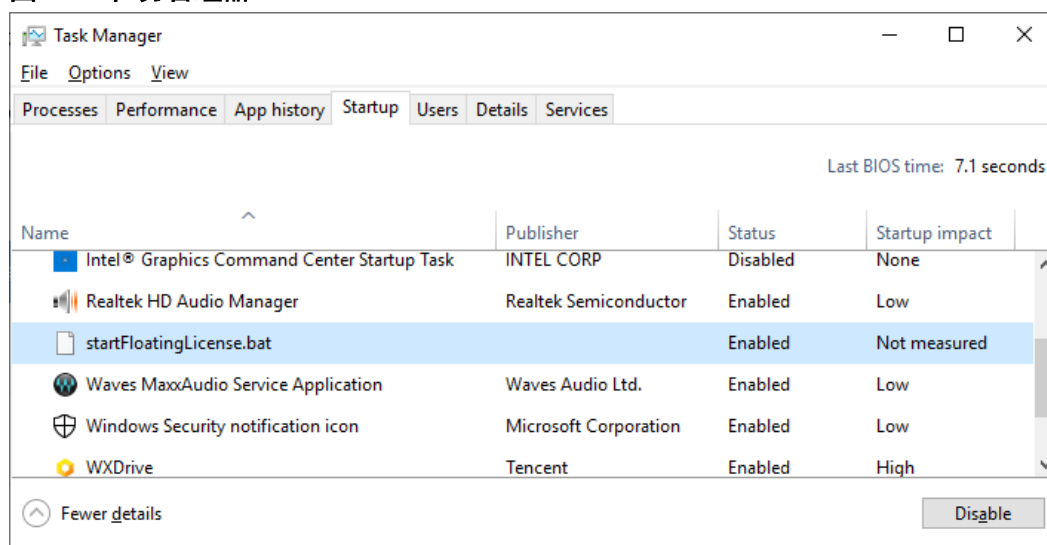
图 4-22 任务管理器
