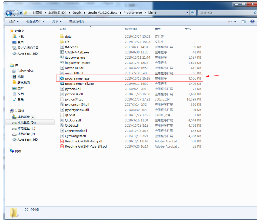
图 2-3 programmer.exe 启动
