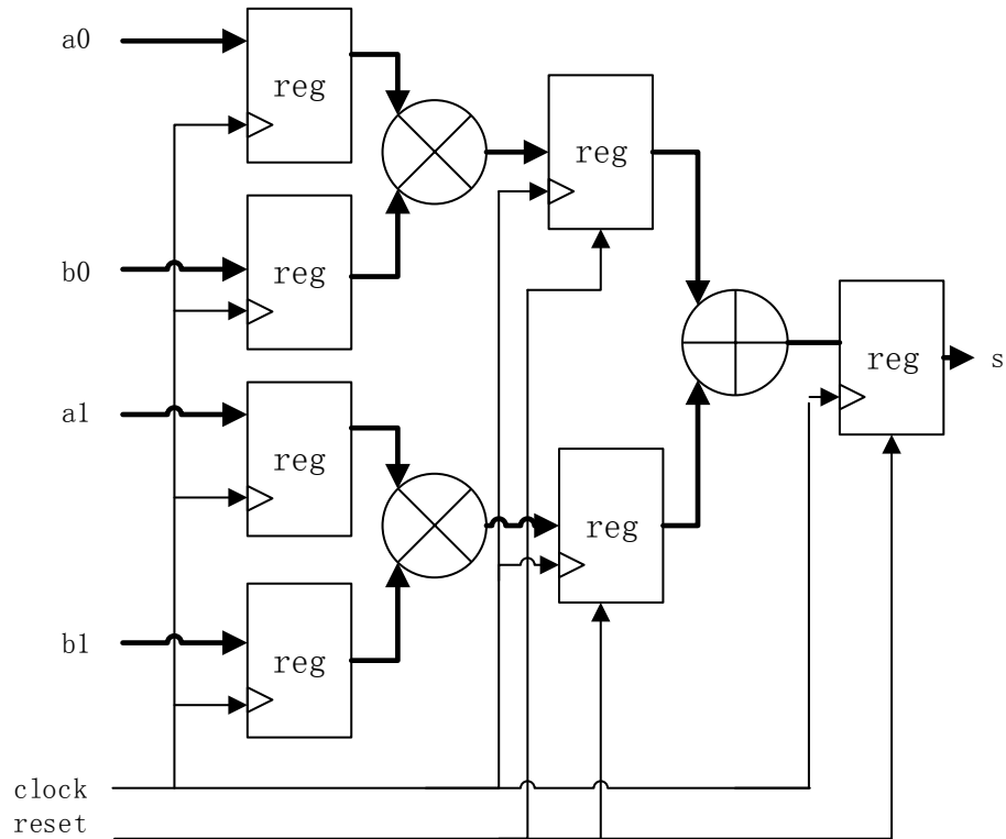
图 4-17 示例 2 DSP 电路图
