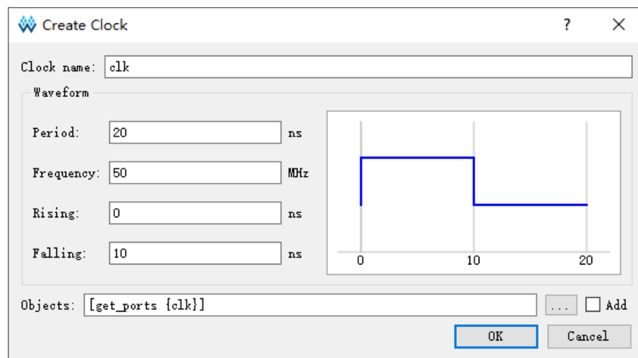
图 3-13 Clock 约束
