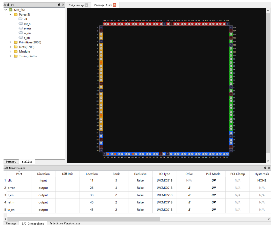
图 3-11 I/O 约束
