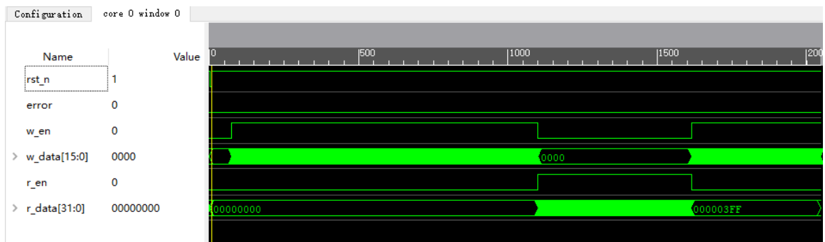
图 3-35 GAO 波形显示
