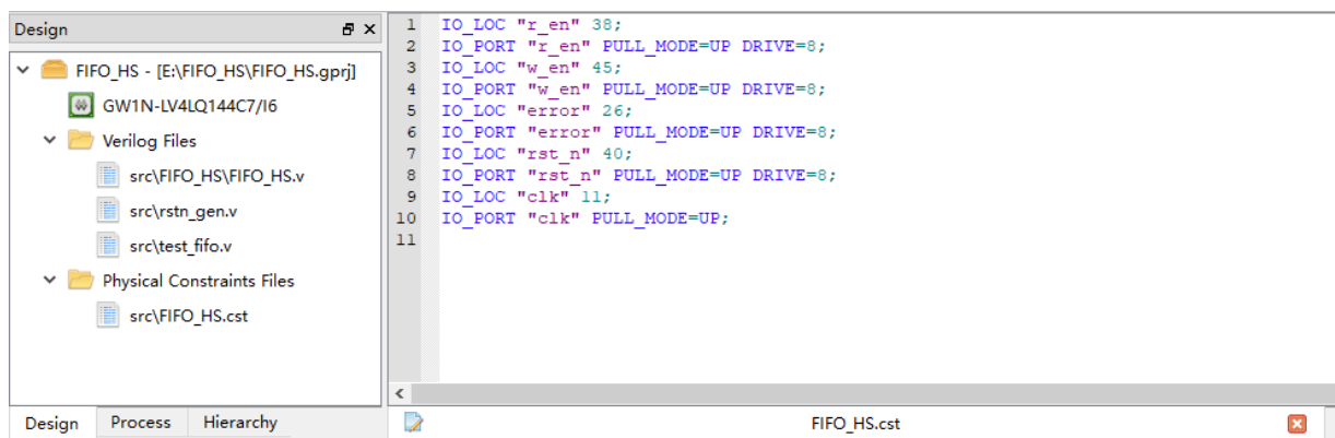
图 3-12 物理约束显示
