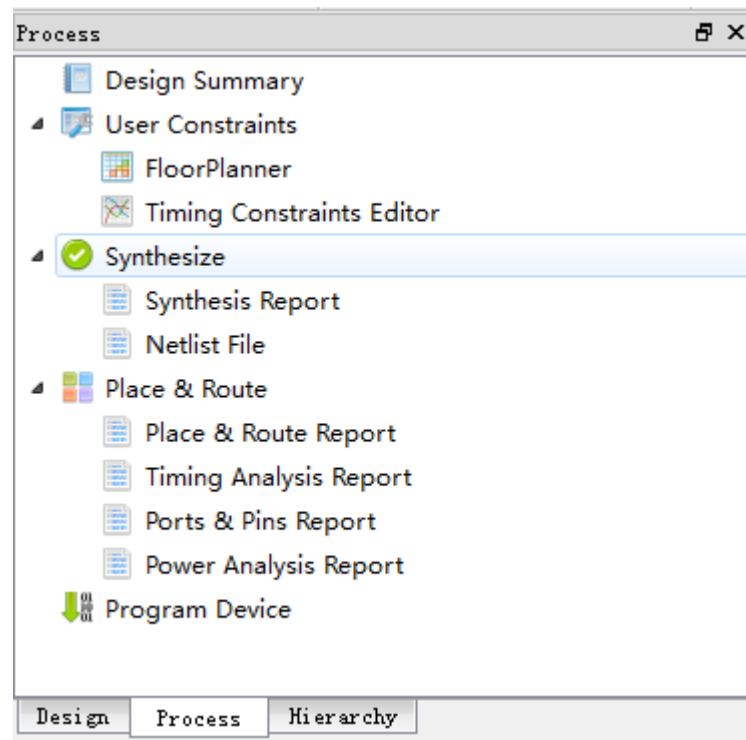
图 3-9 综合完成
