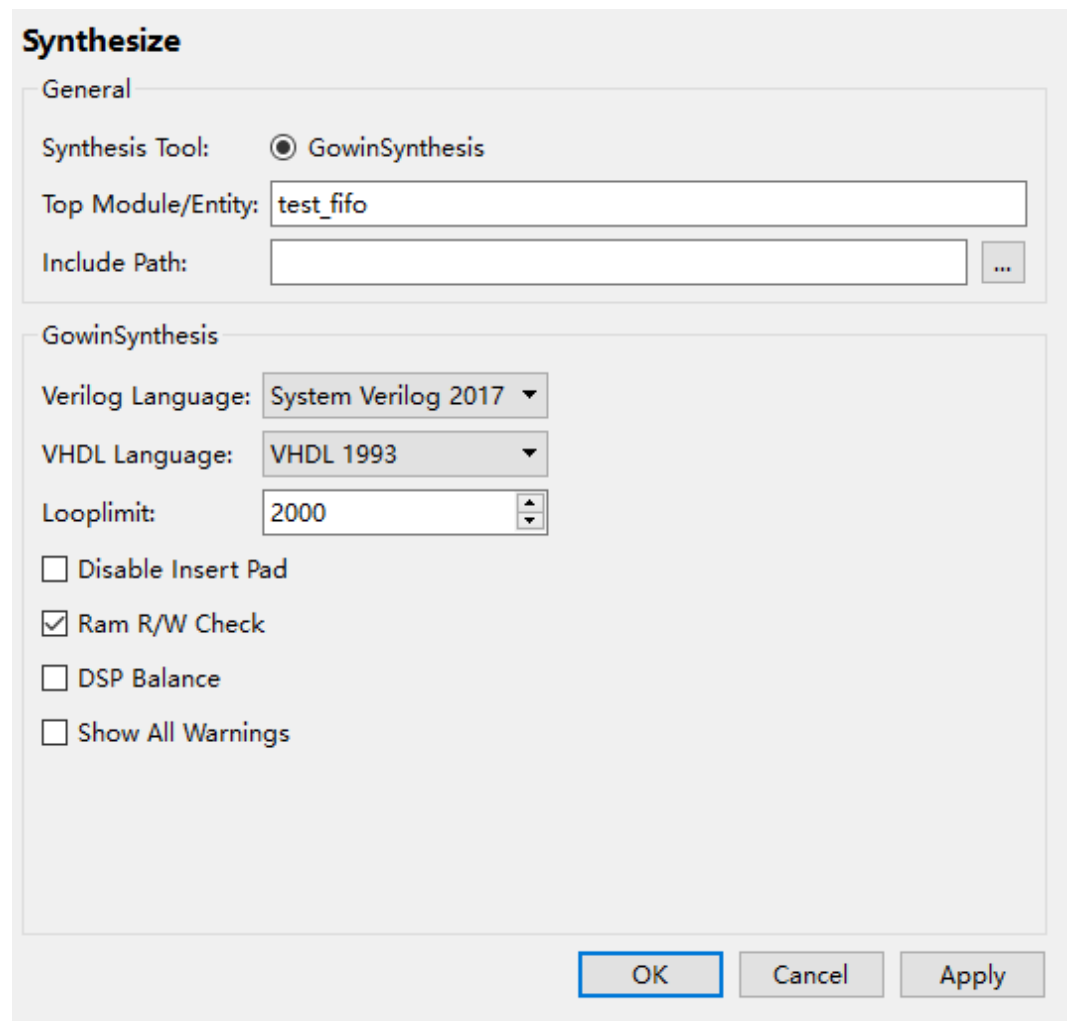
图 3-7 综合选项配置
