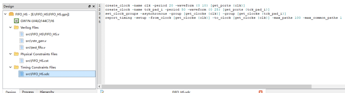
图 3-15 时序约束显示
