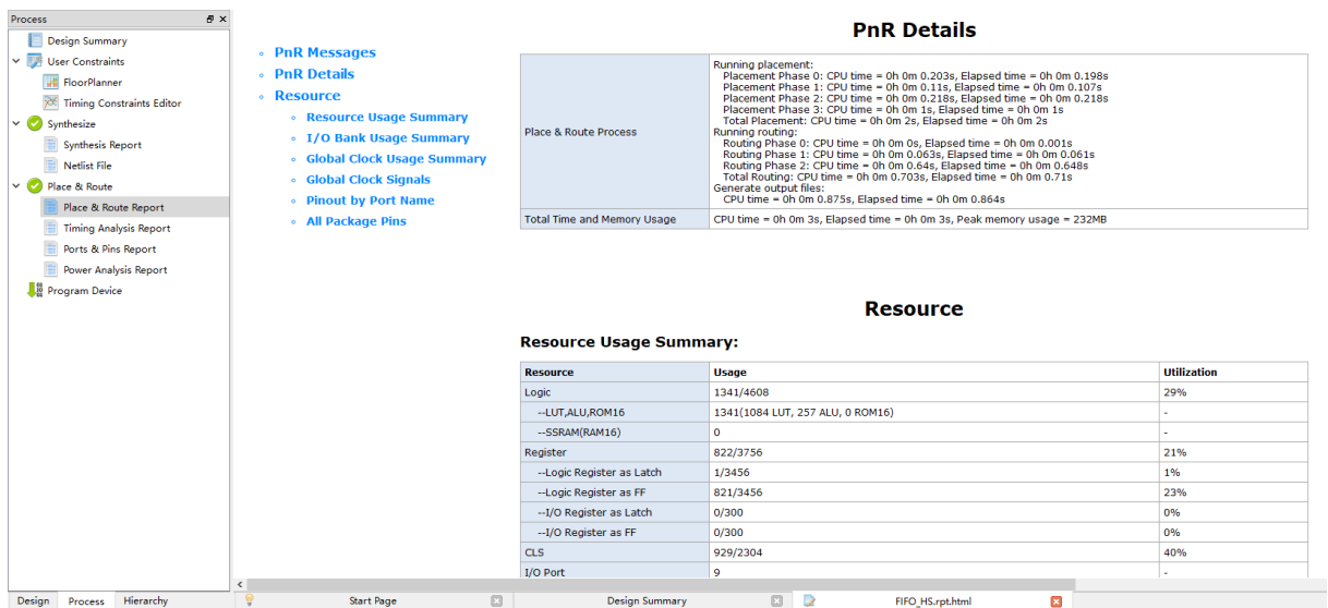
图 3-36 布局布线报告
