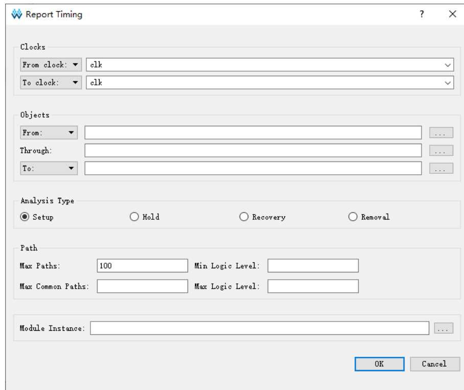
图 3-14 时序报告约束
