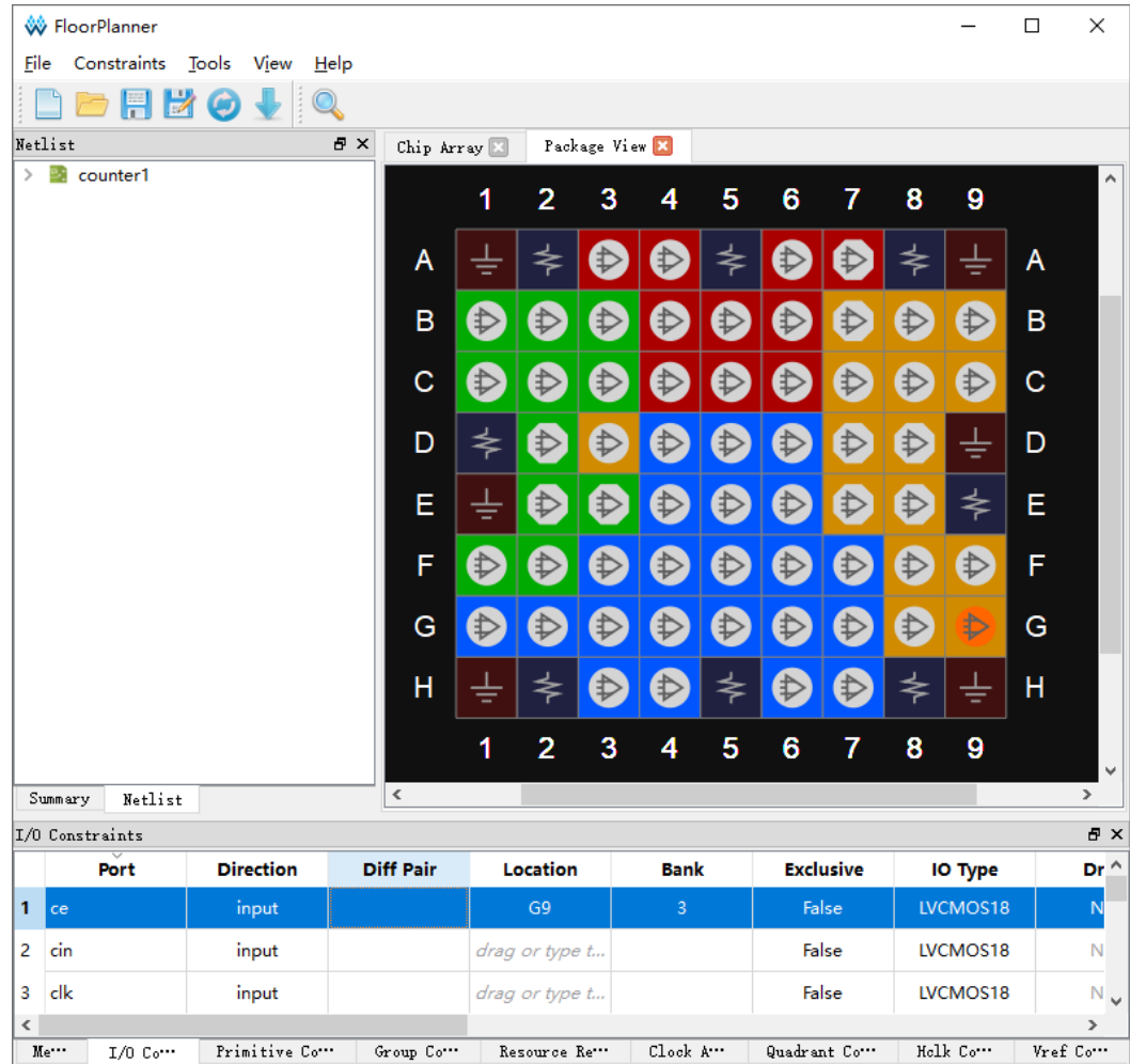
图 4-2 拖至 Package View 创建 I/O Constraints
