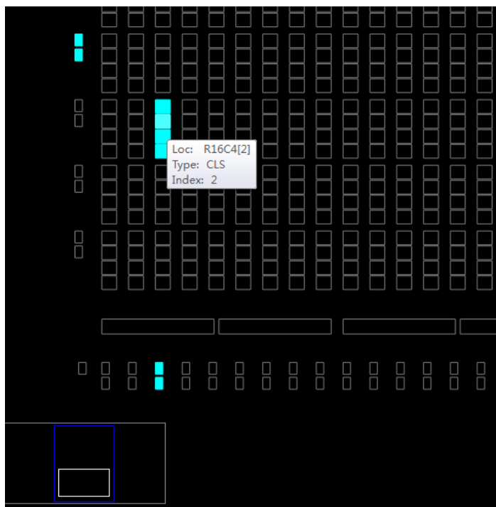
图 3-48 宏单元模式约束
