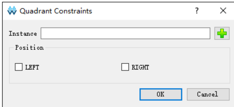
图 3-26 象限约束 (GW1N 系列)
