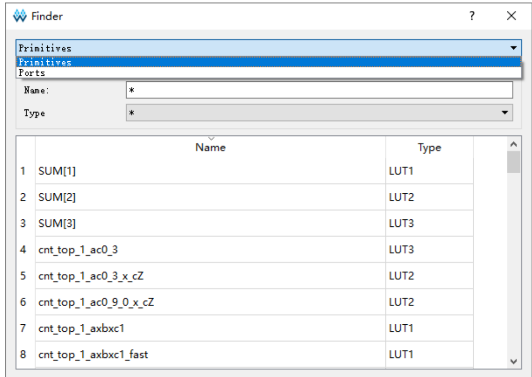
图 3-23 查找对话框
