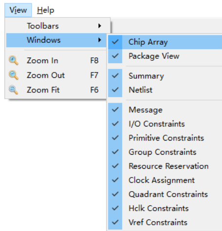
图 3-25 Windows 菜单
