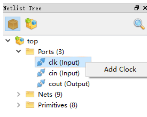
图 4-14 添加时钟
