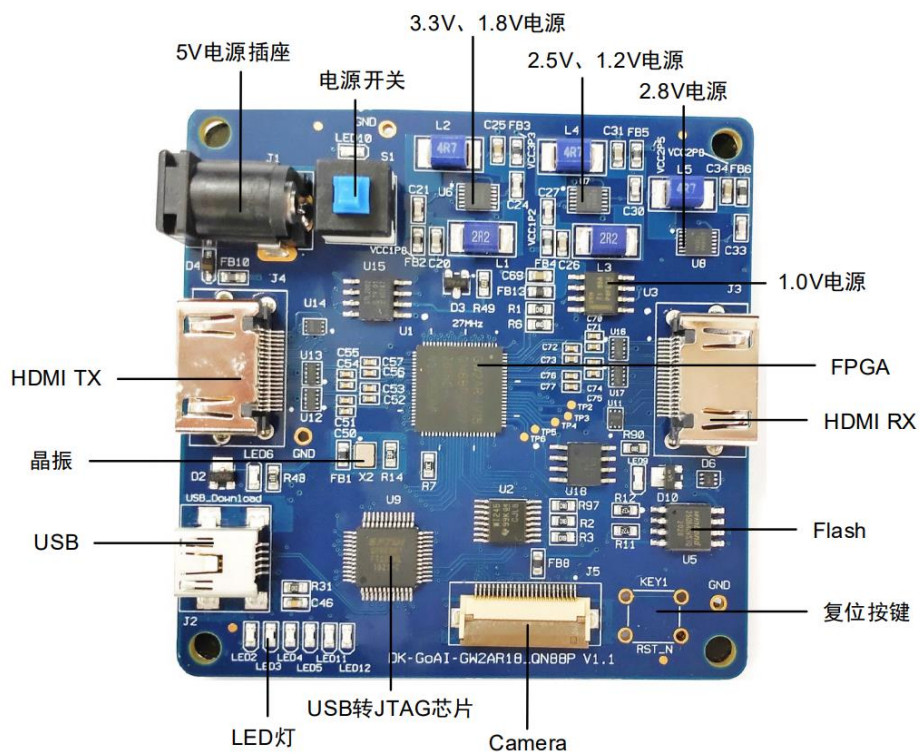
图 1 开发板 PCB 组件说明
