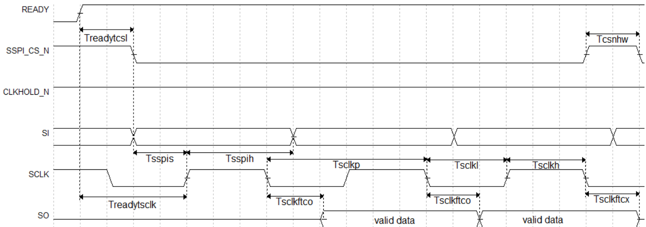
图 4-4 SSPI 配置模式时序图
