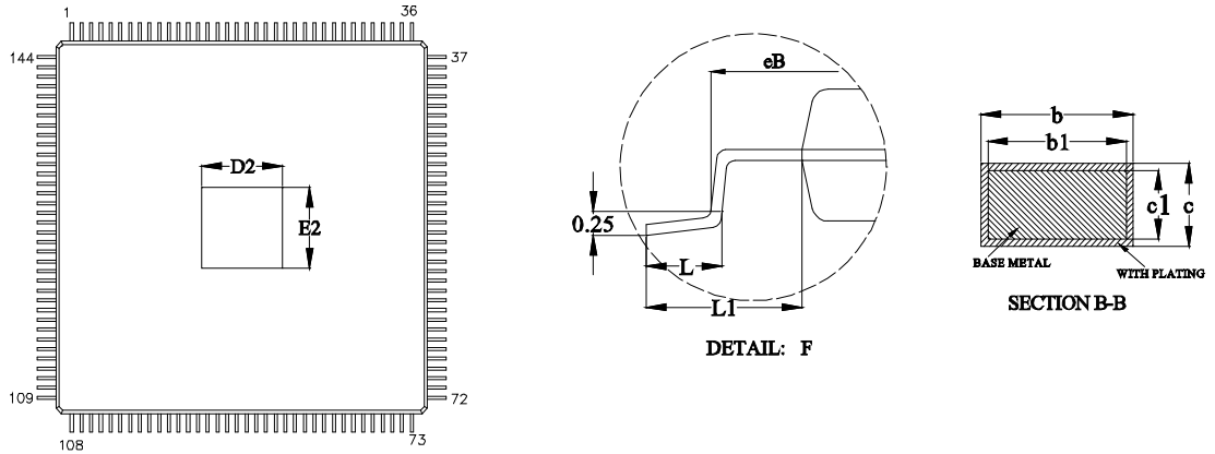
图 4-11 封装尺寸 EQ144
