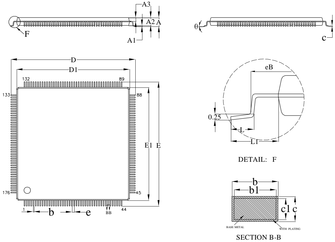
图 4-12 封装尺寸 LQ176
