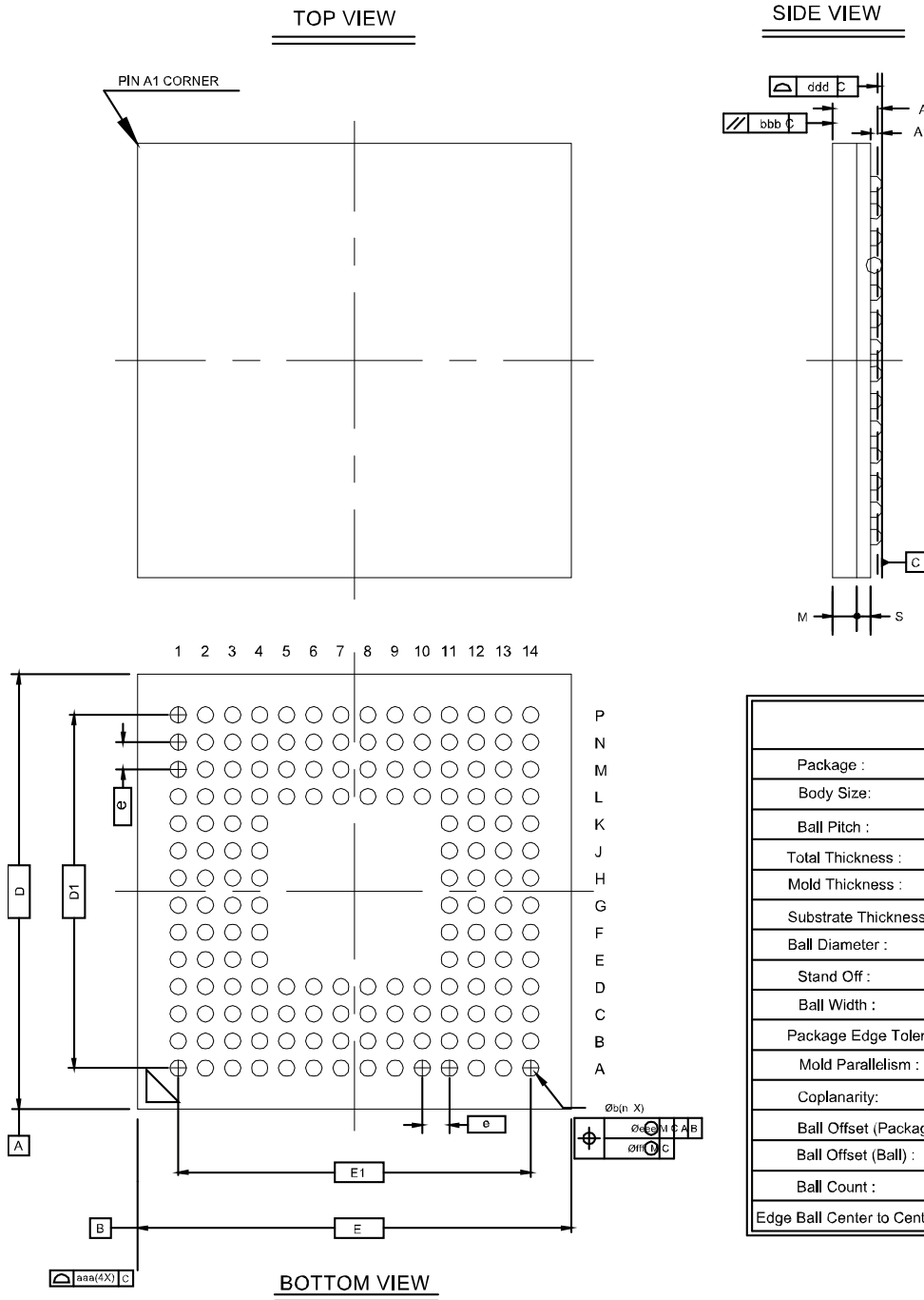
图 4-14 封装尺寸 MG160
