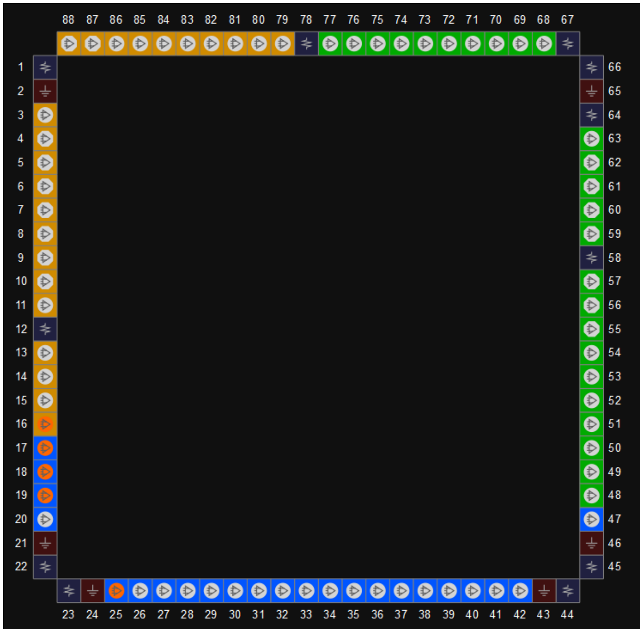
图 3-28 GW1N-6 器件 QN88 封装管脚分布示意图（顶视图）
