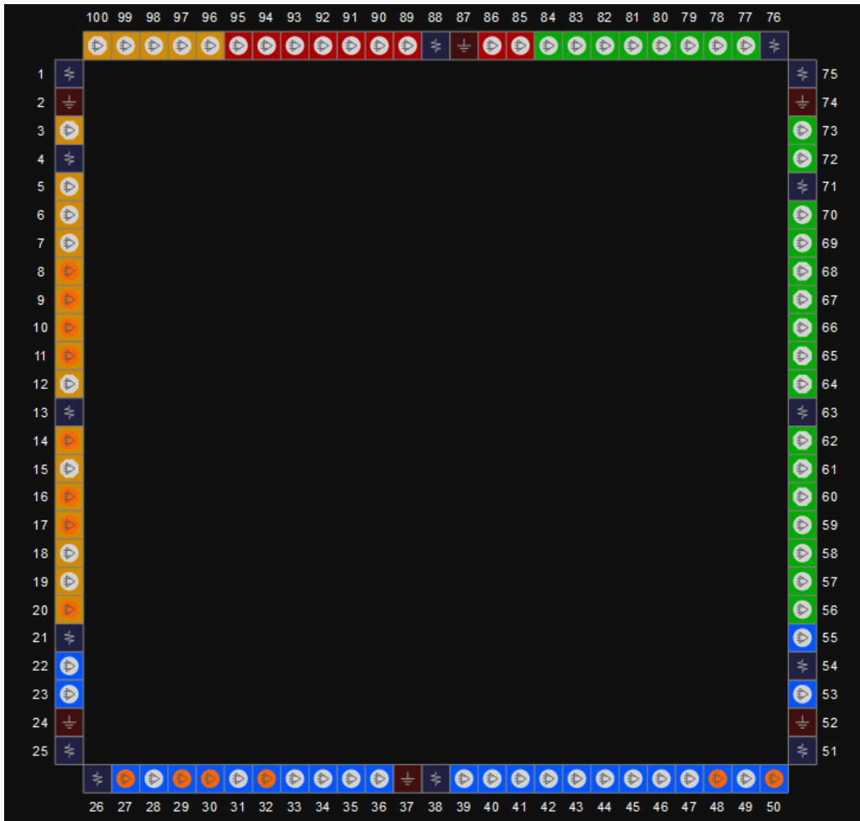
图 3-29 GW1N-6 器件 LQ100 封装管脚分布示意图（顶视图）
