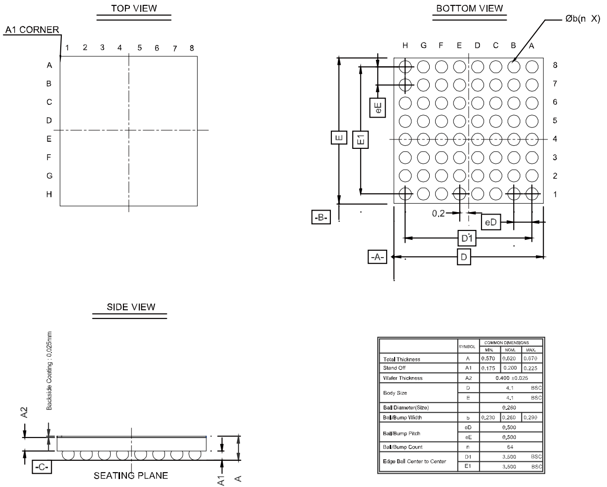
图 4-6 封装尺寸 CM64
