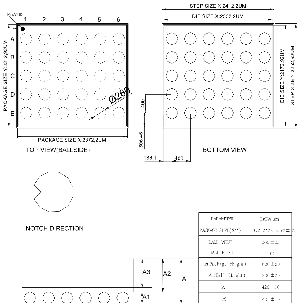
图 4-1 封装尺寸 CS30 (GW1N-1)
