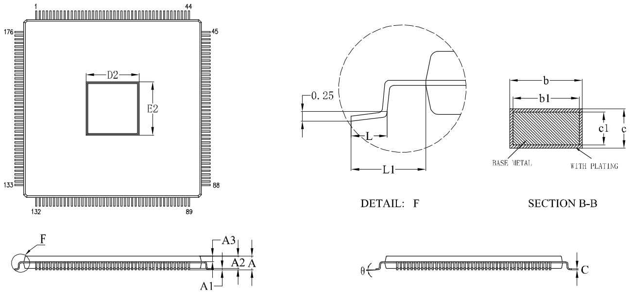
图 4-13 封装尺寸 EQ176
