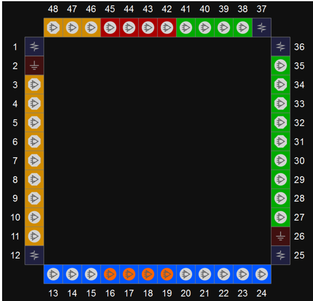
图 3-26 GW1N-6 器件 QN48 封装管脚分布示意图（顶视图）
