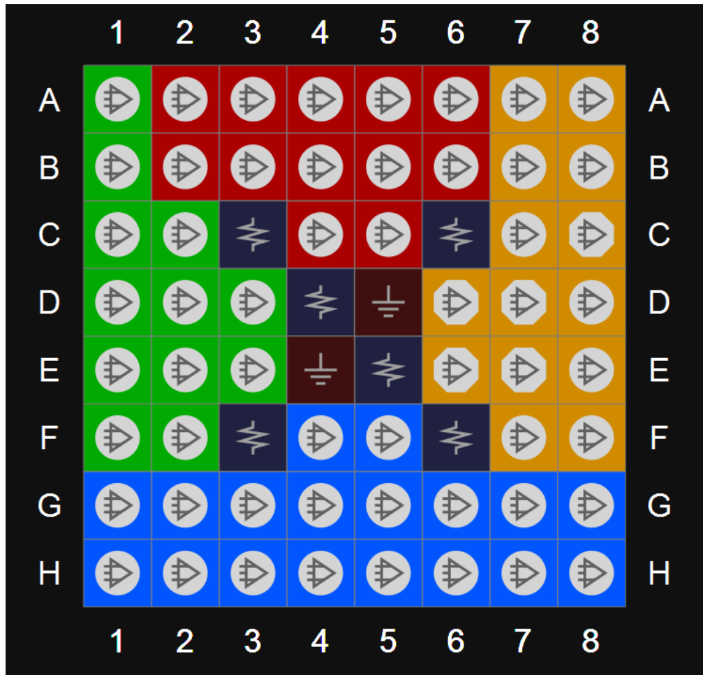
图 3-41 GW1N-9 器件 CM64 封装管脚分布示意图（顶视图）
