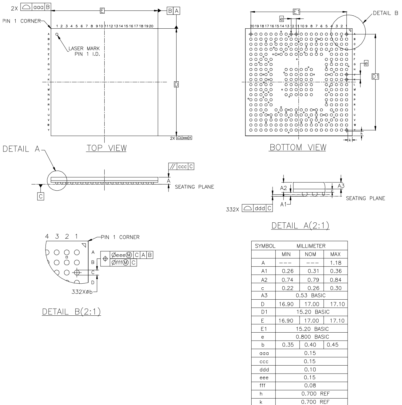
图 4-20 封装尺寸 UG332
