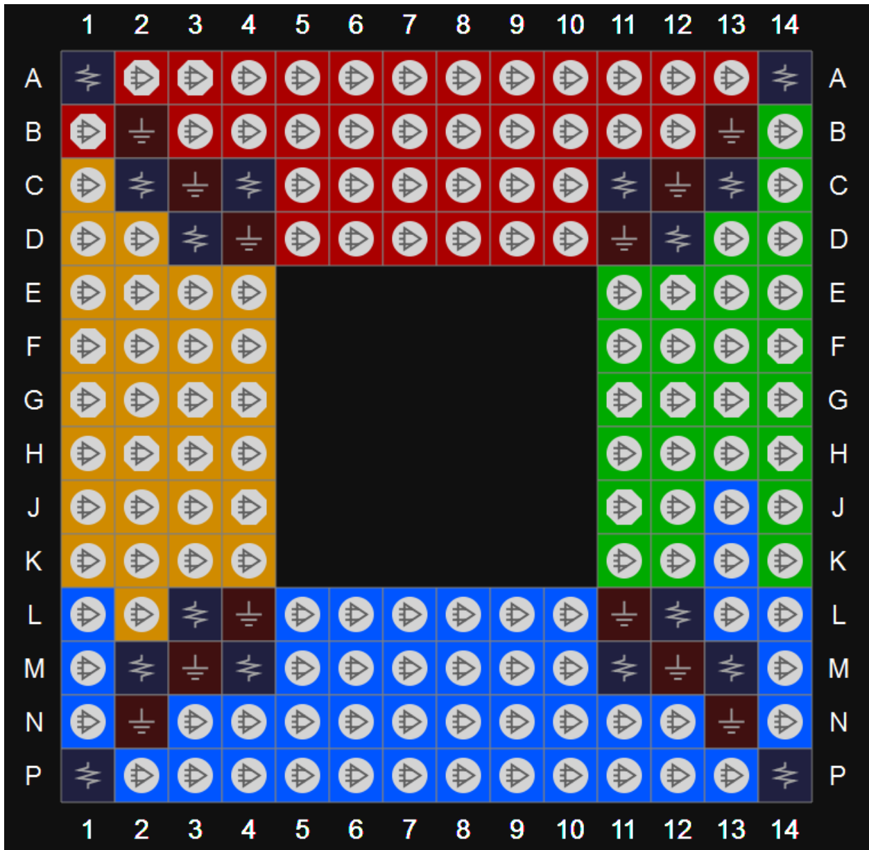
图 3-14 GW1N-2 器件 MG160 封装管脚分布示意图（顶视图）
