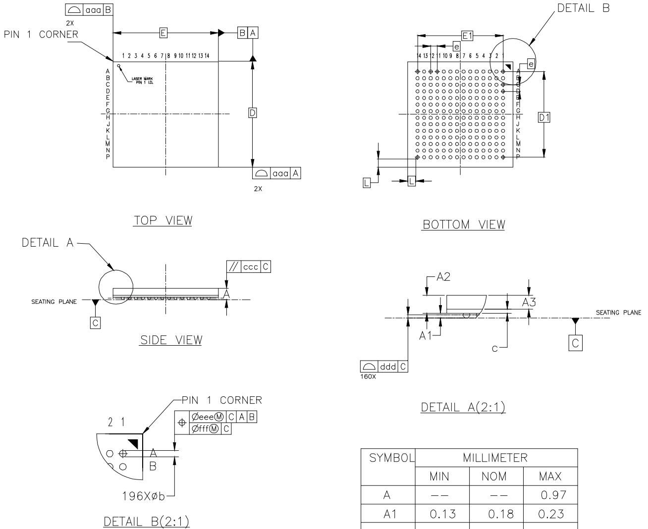
图 4-15 封装尺寸 MG196
