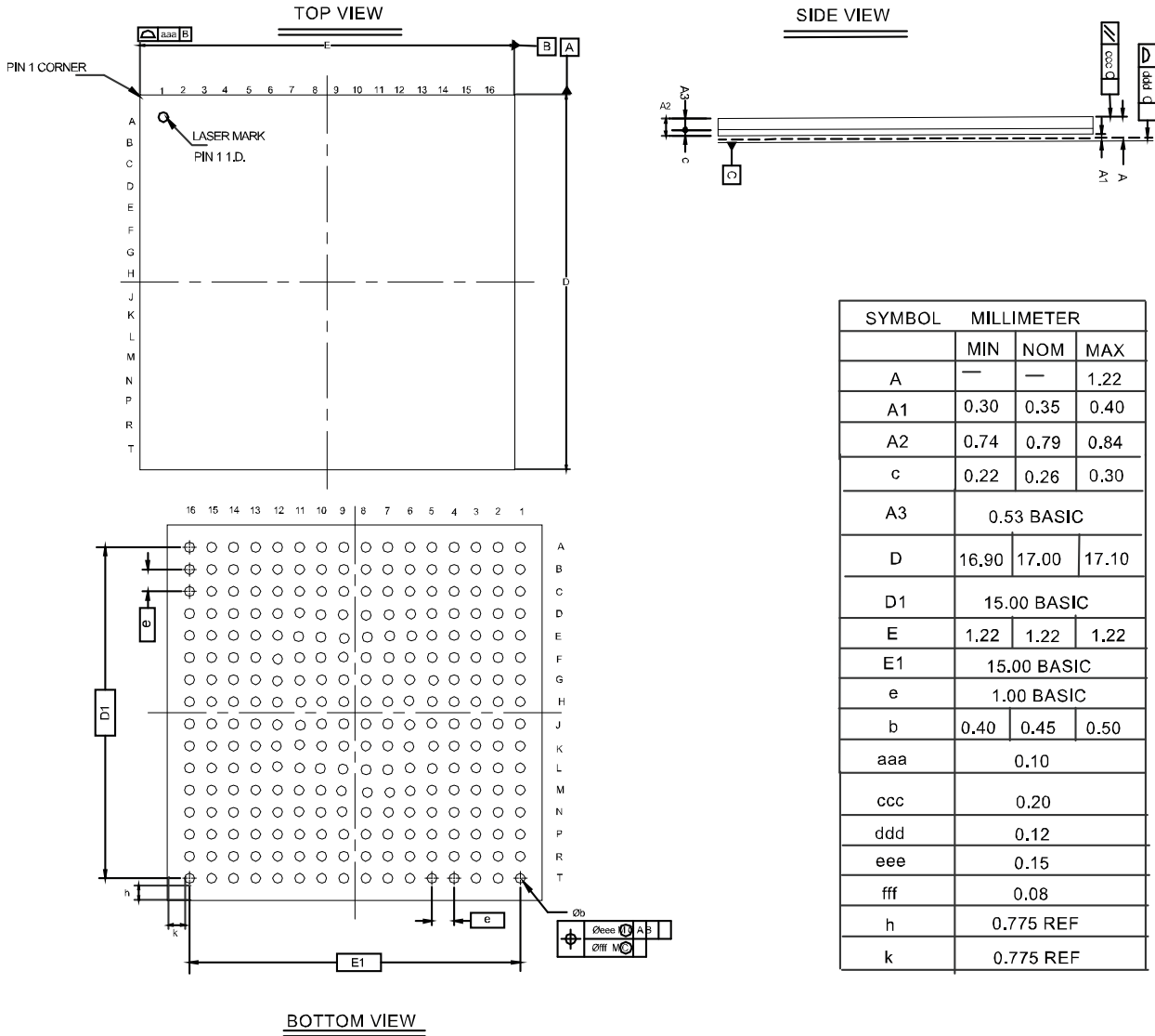
图 4-17 封装尺寸 PG256
