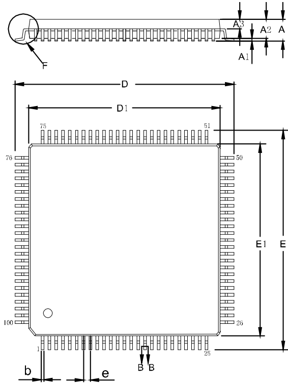
图 4-9 封装尺寸 LQ100
