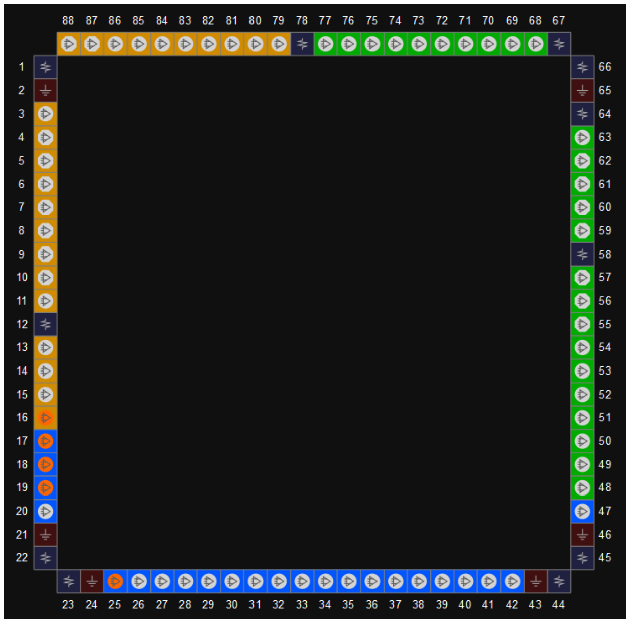
图 3-42 GW1N-9 器件 QN88 封装管脚分布示意图（顶视图）
