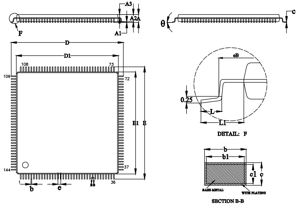
图 4-10 封装尺寸 LQ144
