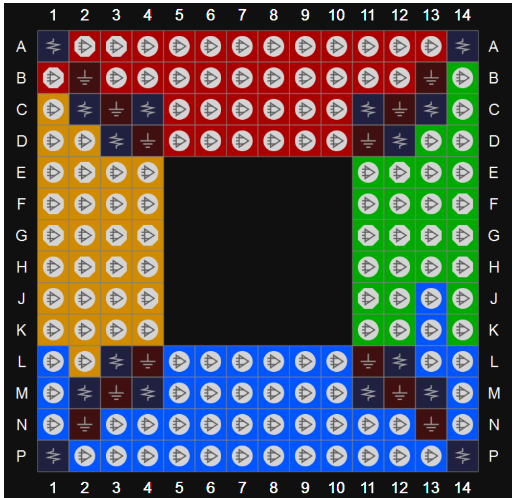
图 3-23 GW1N-4 器件 MG160 封装管脚分布示意图（顶视图）
