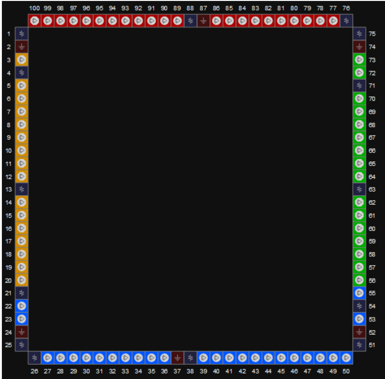
图 3-21 GW1N-4 器件 LQ100 封装管脚分布示意图（顶视图）
