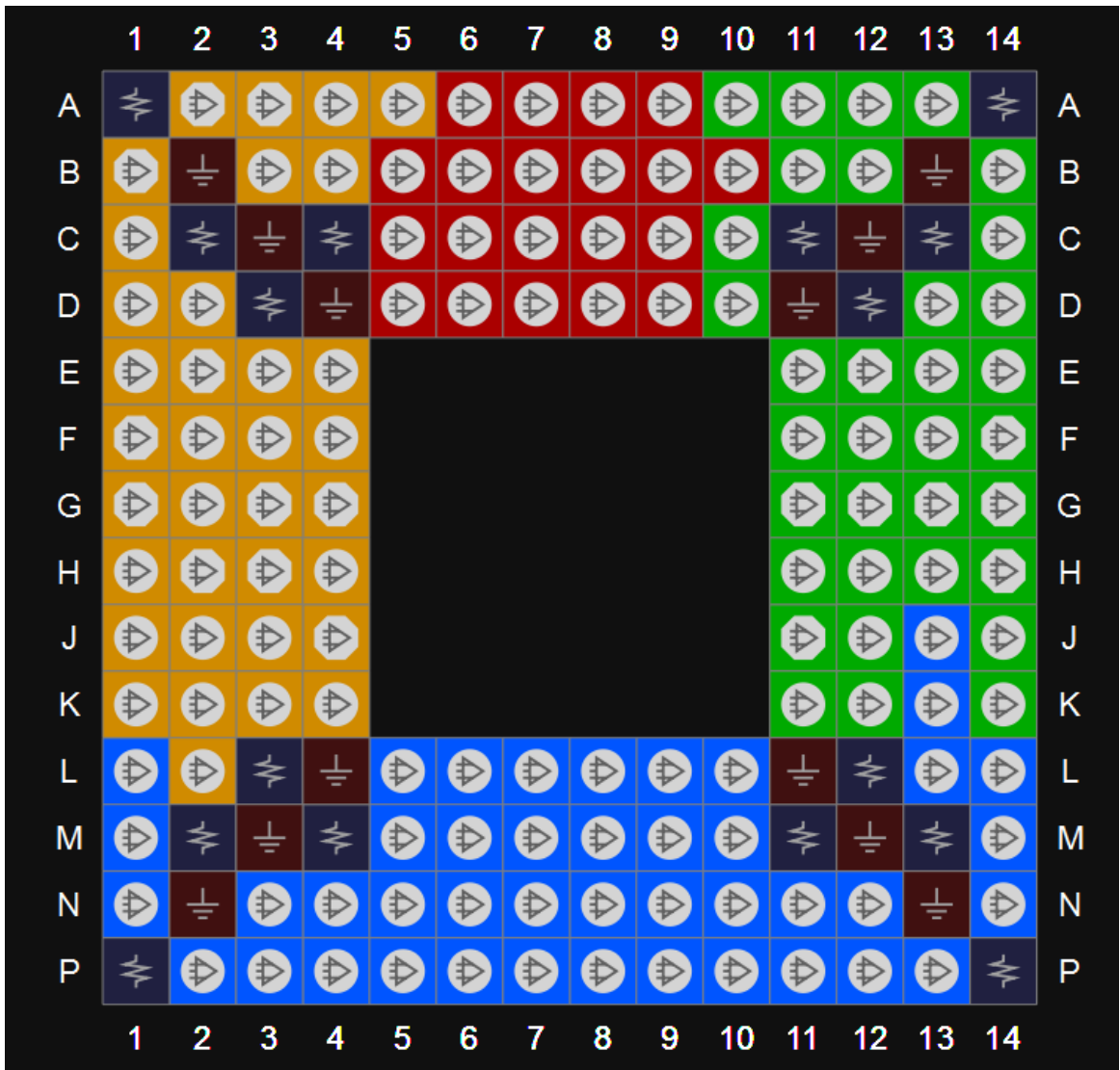
图 3-46 GW1N-9 器件 MG160 封装管脚分布示意图（顶视图）
