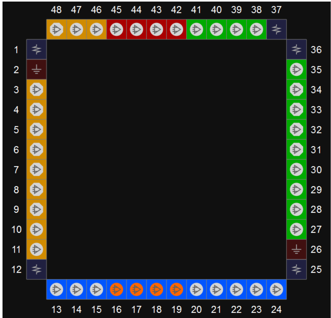
图 3-40 GW1N-9 器件 QN48 封装管脚分布示意图（顶视图）
