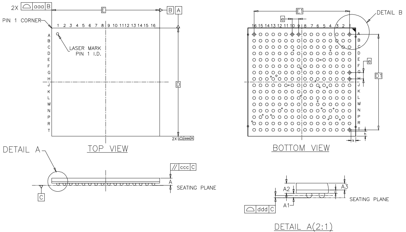
图 4-16 封装尺寸 PG256M
