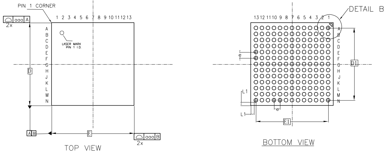
图 4-18 封装尺寸 UG169
