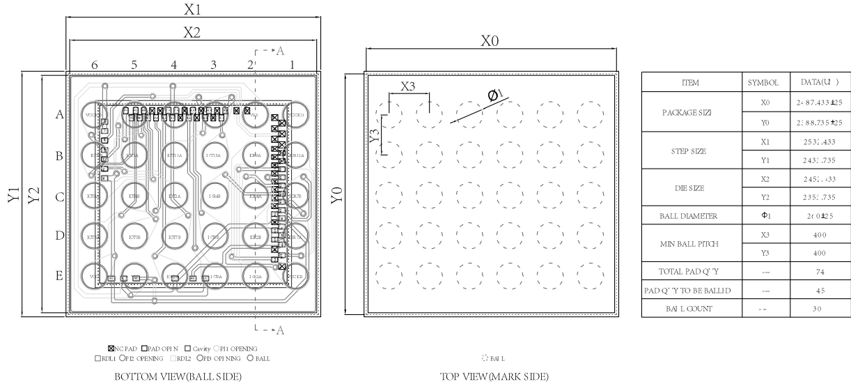
图 4-2 封装尺寸 CS30 (GW1N-1S)
