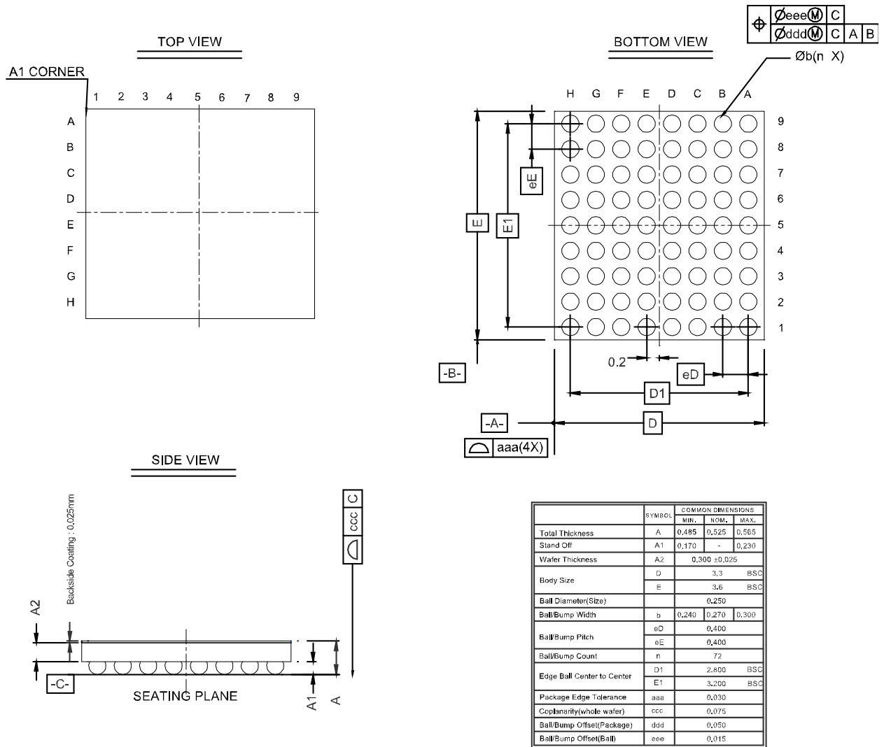
图 4-7 封装尺寸 CS72
