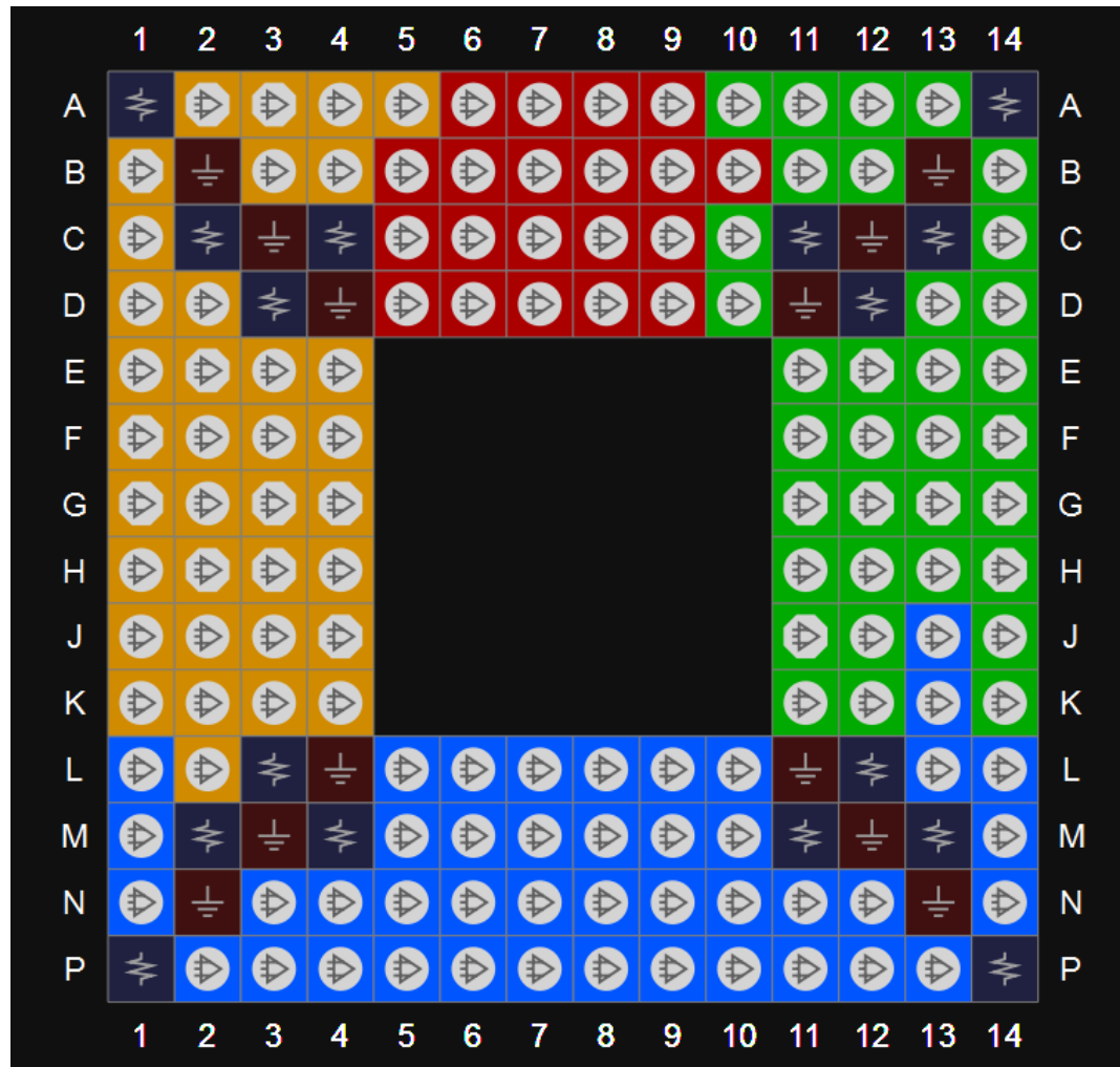
图 3-32 GW1N-6 器件 MG160 封装管脚分布示意图（顶视图）
