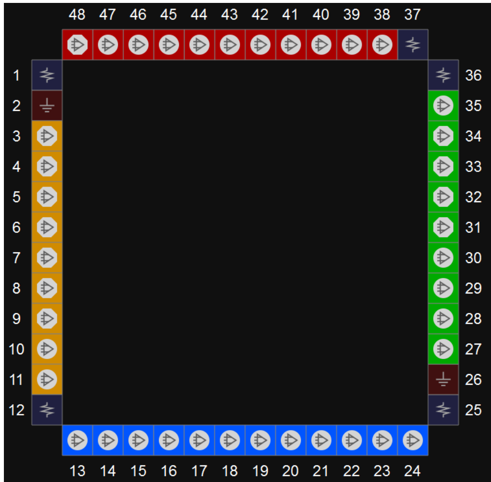
图 3-18 GW1N-4 器件 QN48 封装管脚分布示意图（顶视图）
