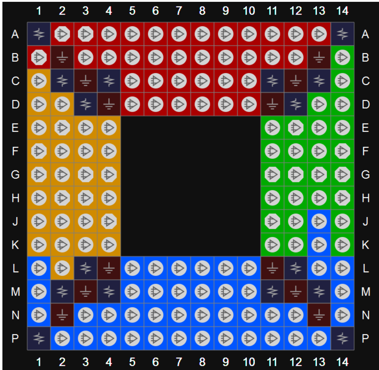
图 3-16 GW1N-2 器件 MG160 封装管脚分布示意图（顶视图）
