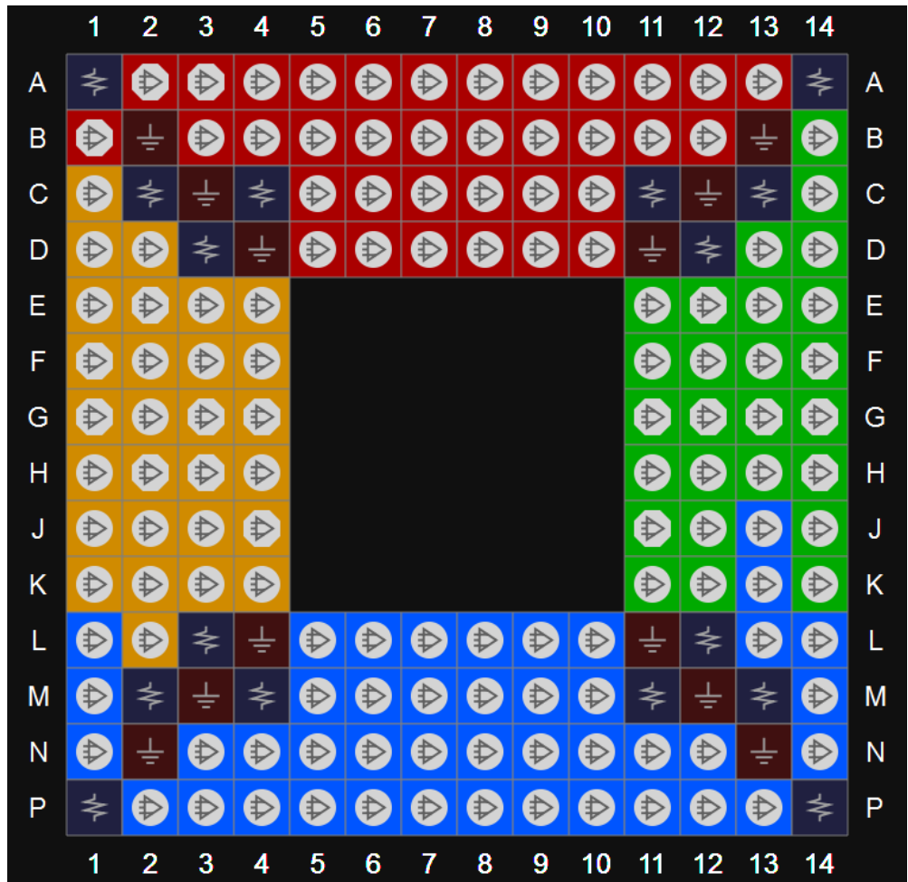
图 3-25 GW1N-4 器件 MG160 封装管脚分布示意图（顶视图）
