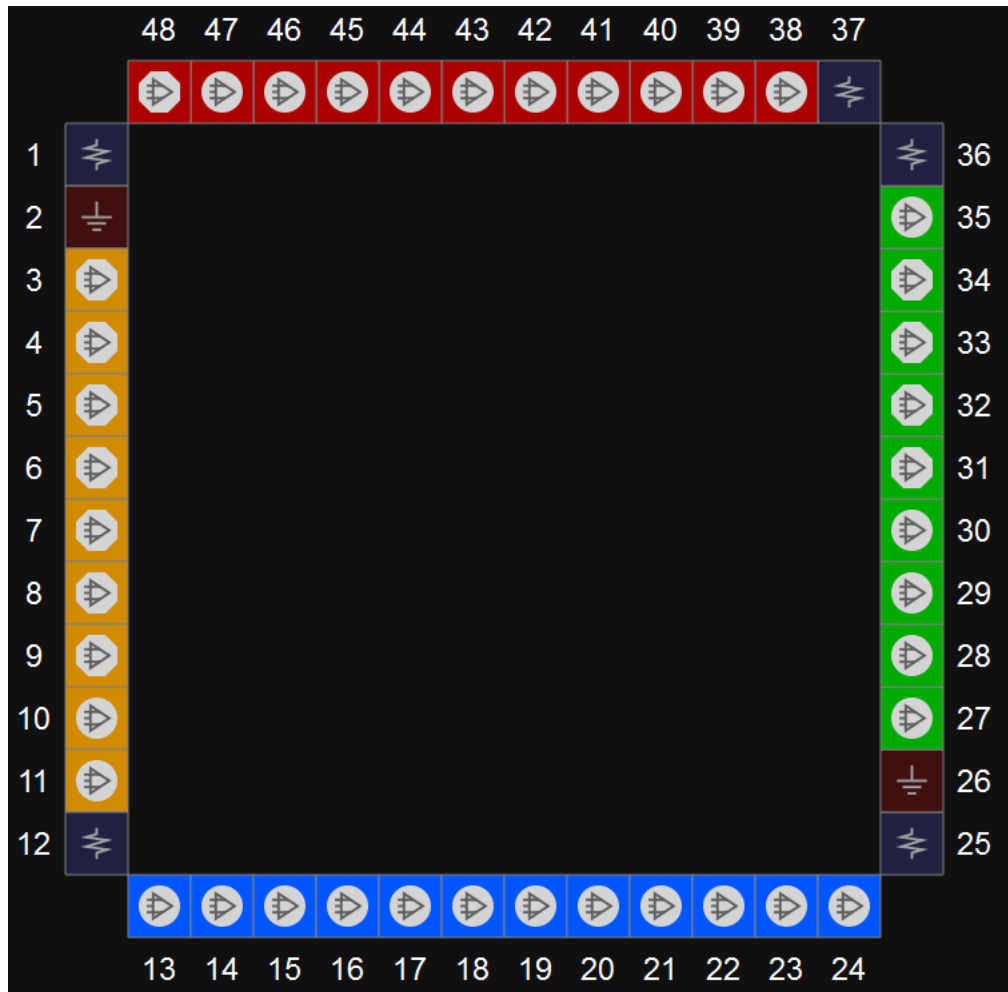
图 3-20 GW1N-4 器件 QN48 封装管脚分布示意图（顶视图）
