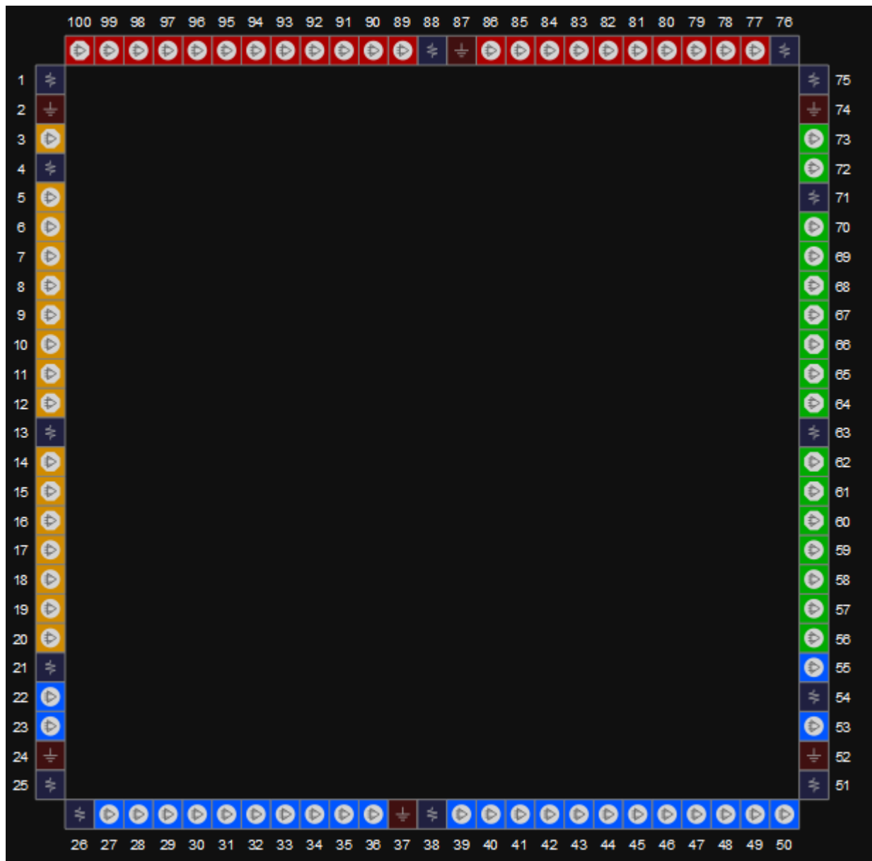
图 3-14 GW1N-2 器件 LQ100 封装管脚分布示意图（顶视图）
