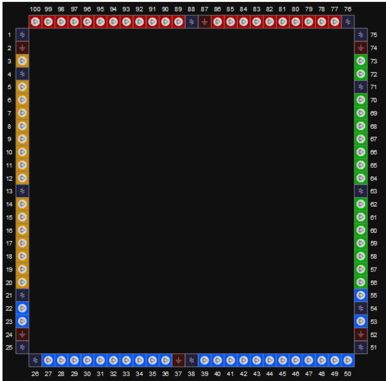
图 3-23 GW1N-4 器件 LQ100 封装管脚分布示意图（顶视图）
