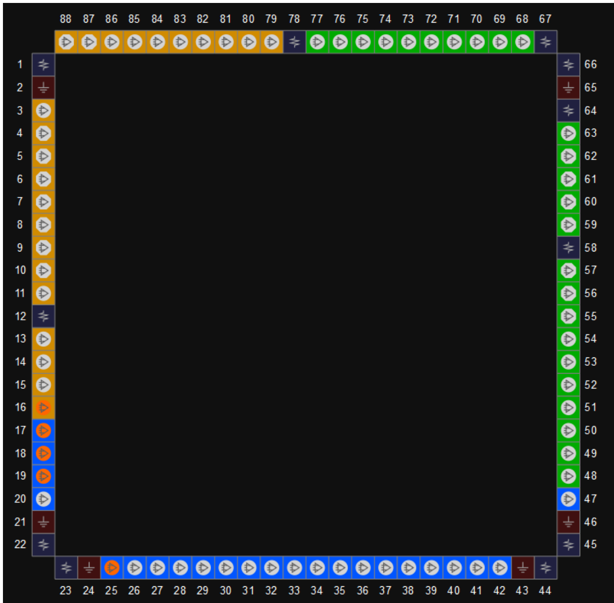
图 3-30 GW1N-6 器件 QN88 封装管脚分布示意图（顶视图）
