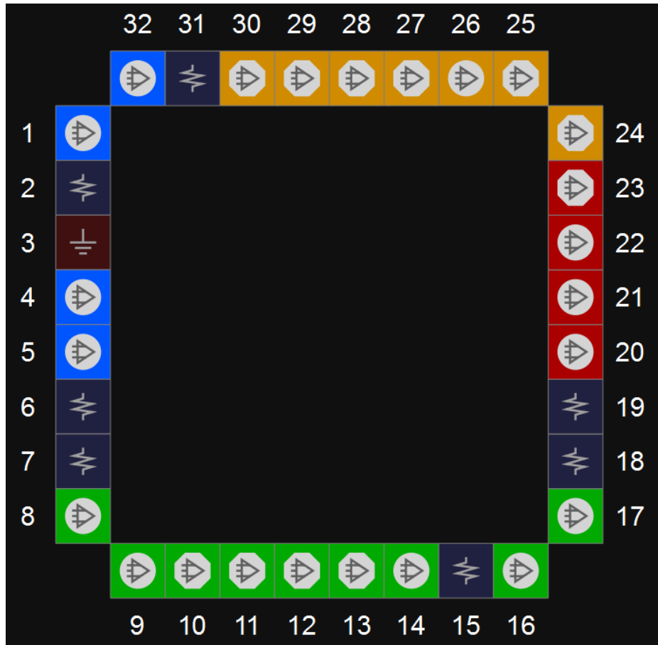
图 3-19 GW1N-4 器件 QN32 封装管脚分布示意图（顶视图）
