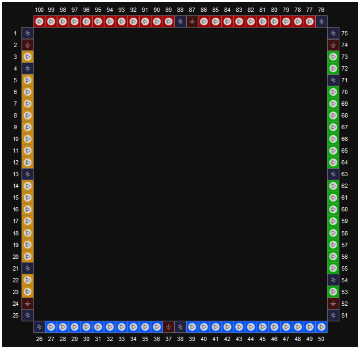
图 3-8 GW1N-1 器件 LQ100X-UV 封装管脚分布示意图（顶视图）
