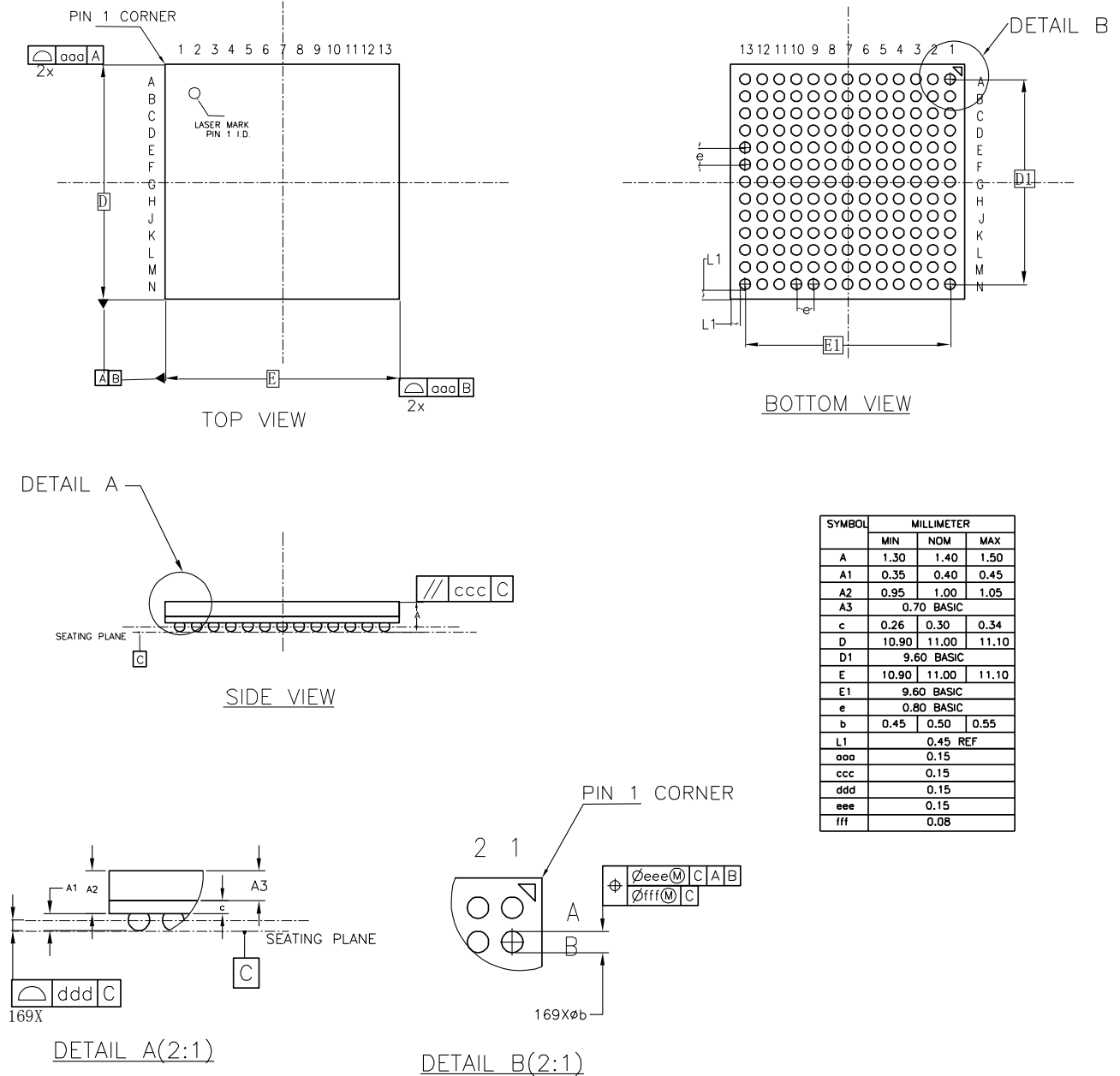
图 4-18 封装尺寸 UG169
