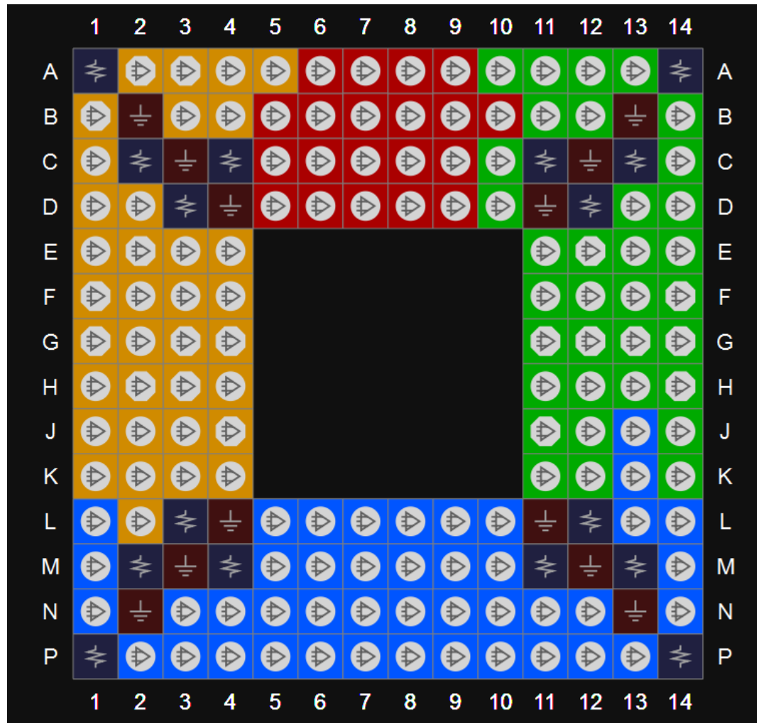
图 3-34 GW1N-6 器件 MG160 封装管脚分布示意图（顶视图）
