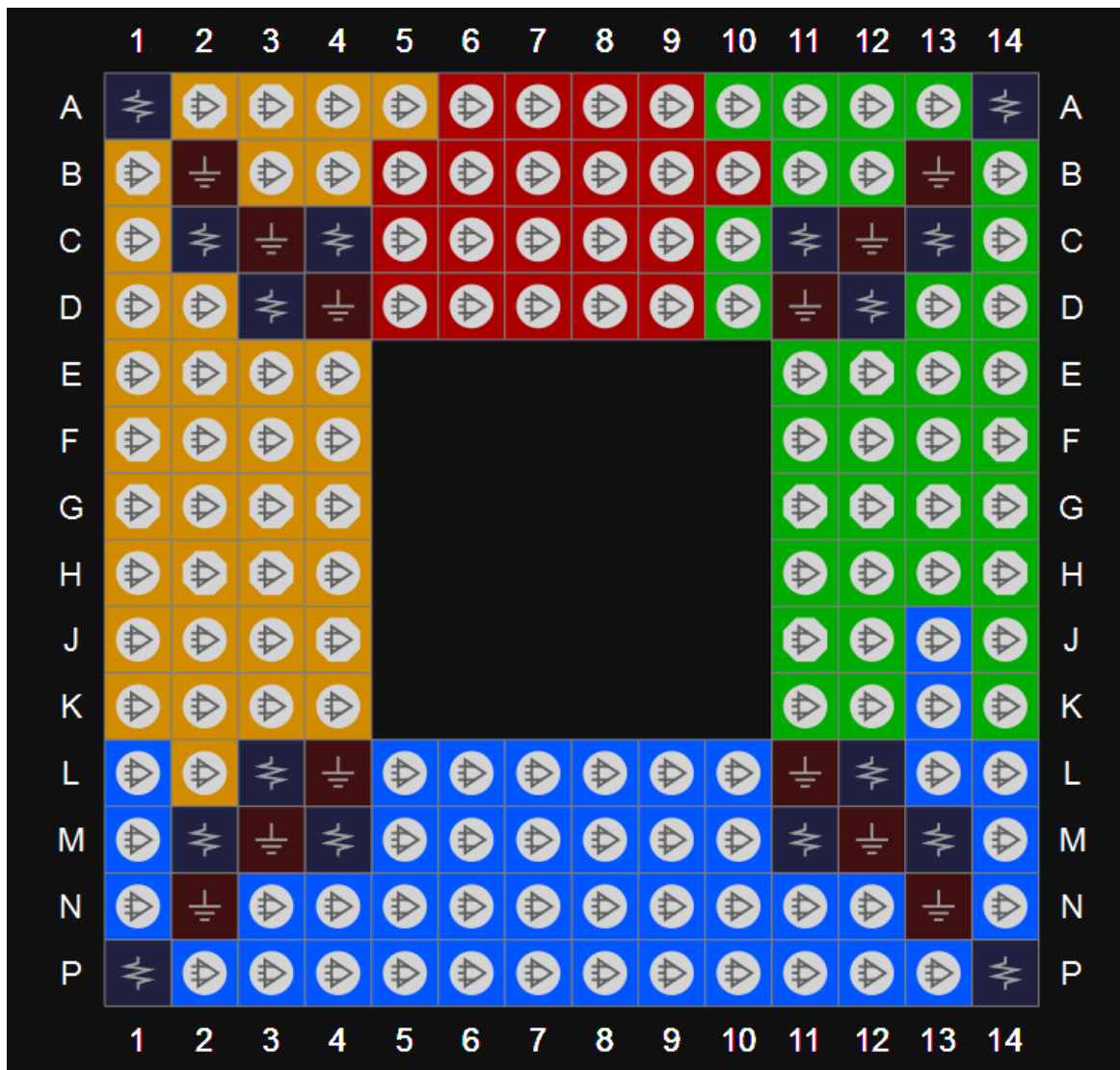
图 3-48 GW1N-9 器件 MG160 封装管脚分布示意图（顶视图）
