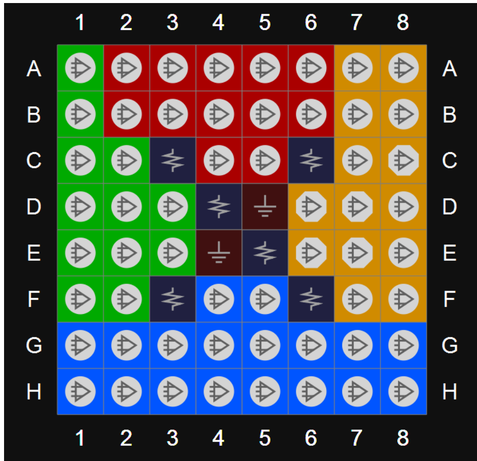
图 3-29 GW1N-6 器件 CM64 封装管脚分布示意图（顶视图）
