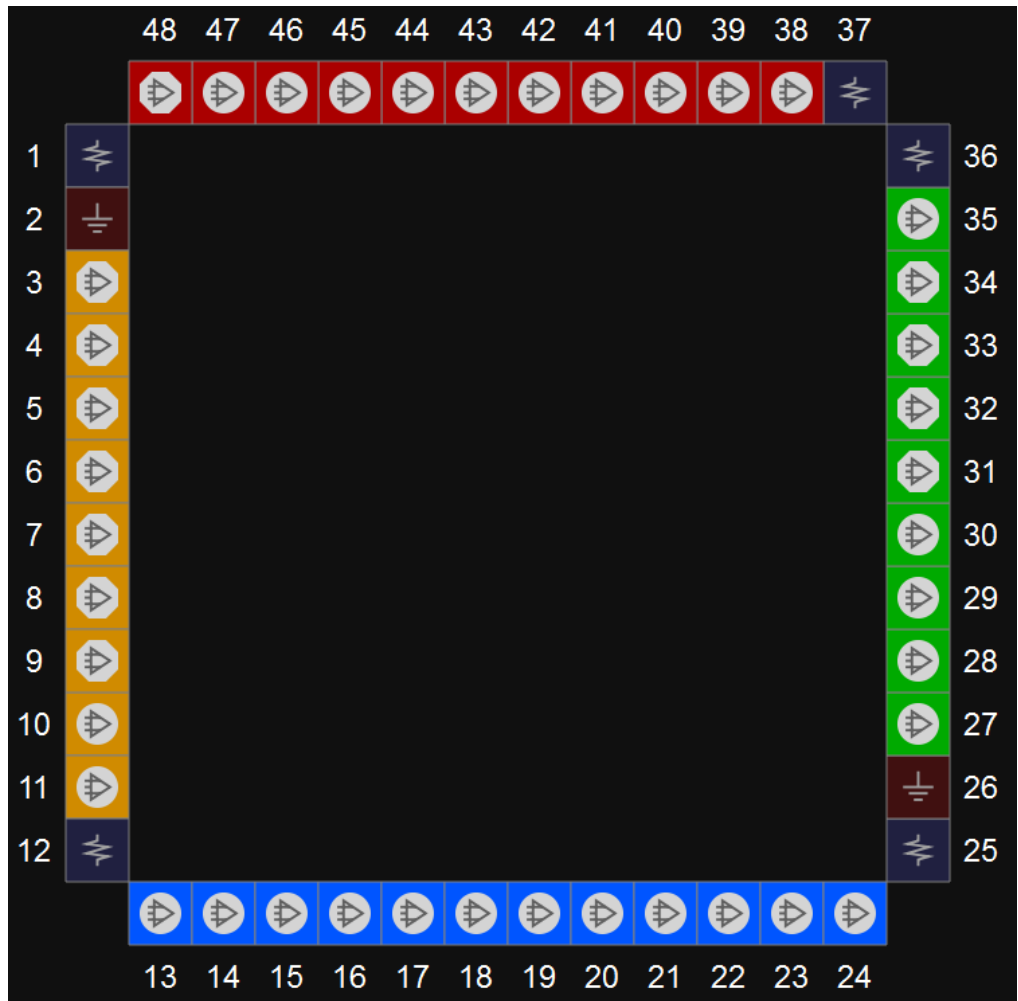
图 3-11 GW1N-2 器件 QN48 封装管脚分布示意图（顶视图）
