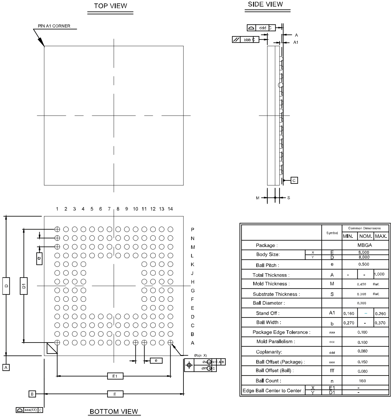
图 4-14 封装尺寸 MG160
