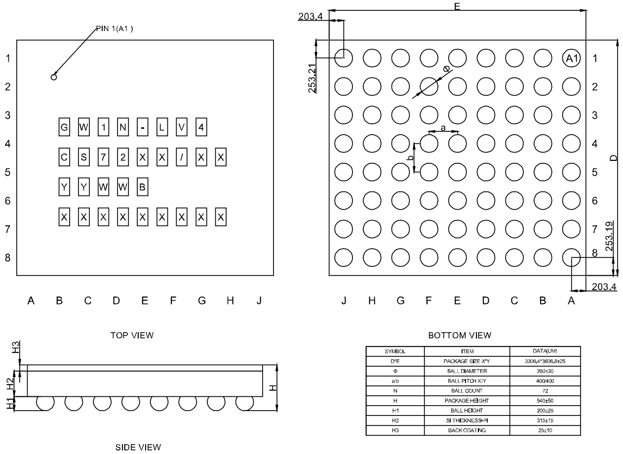
图 4-7 封装尺寸 CS72
