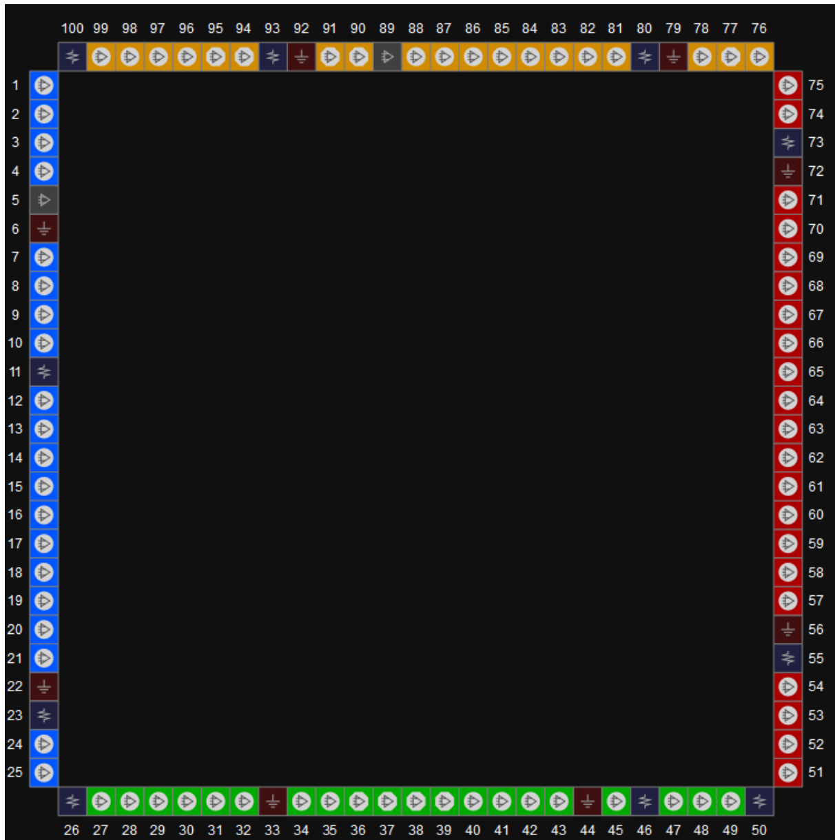
图 3-7 GW1N-1 器件 LQ100X-LV 封装管脚分布示意图（顶视图）
