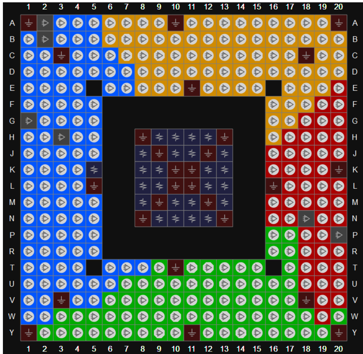
图 3-55 GW1N-9 器件 UG332 管脚分布示意图（顶视图）
