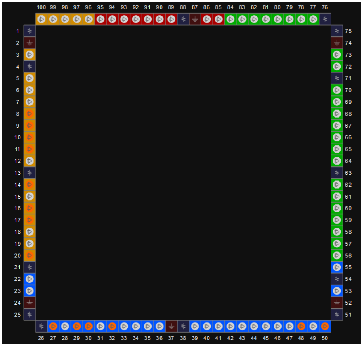
图 3-45 GW1N-9 器件 LQ100 封装管脚分布示意图（顶视图）
