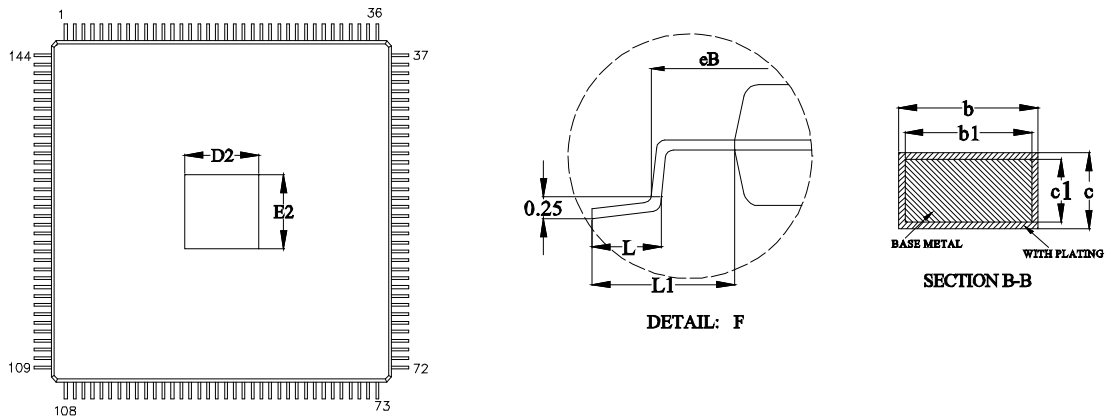
图 4-11 封装尺寸 EQ144
