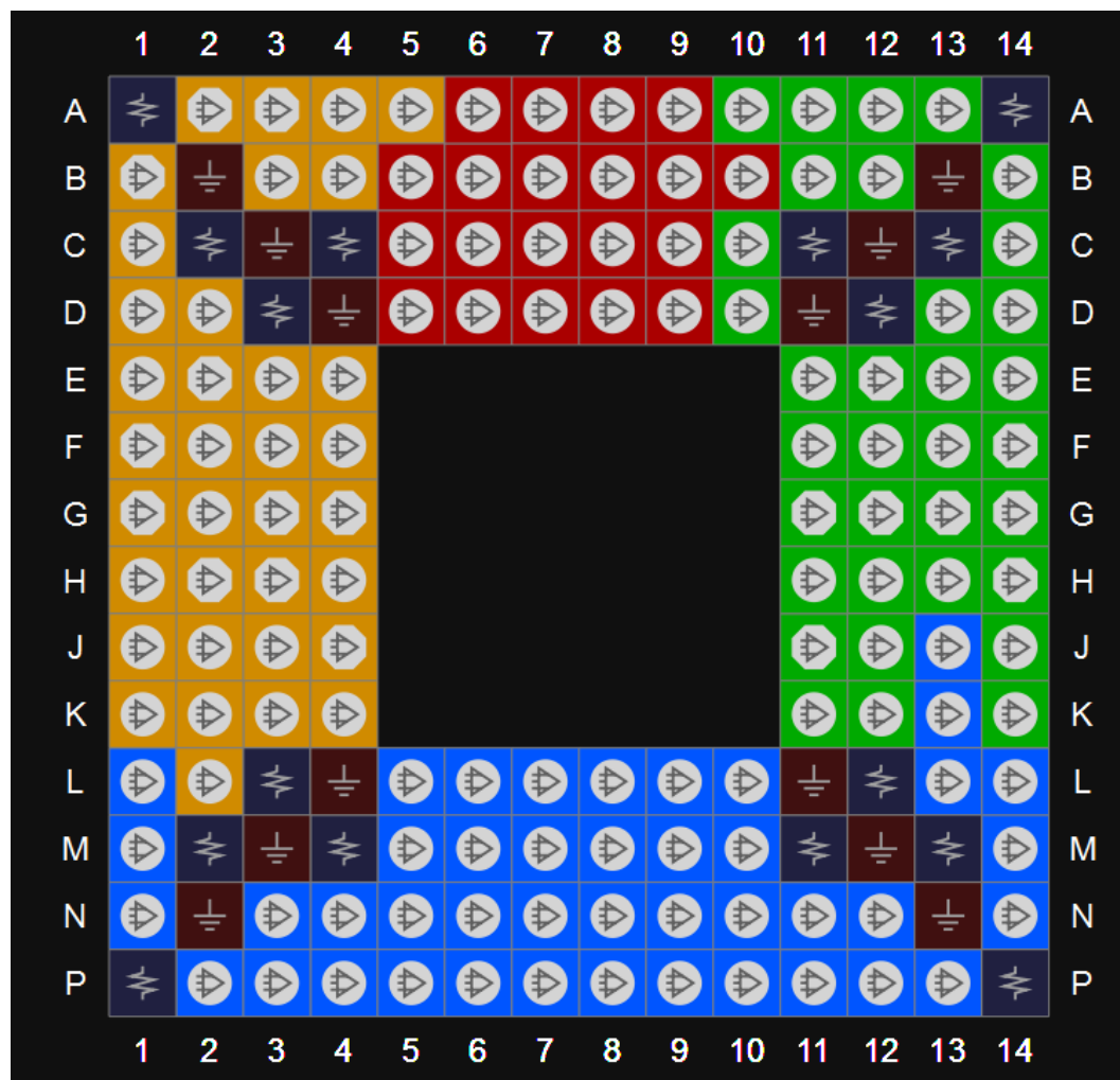
图 3-35 GW1N-6 器件 MG160 封装管脚分布示意图（顶视图）
