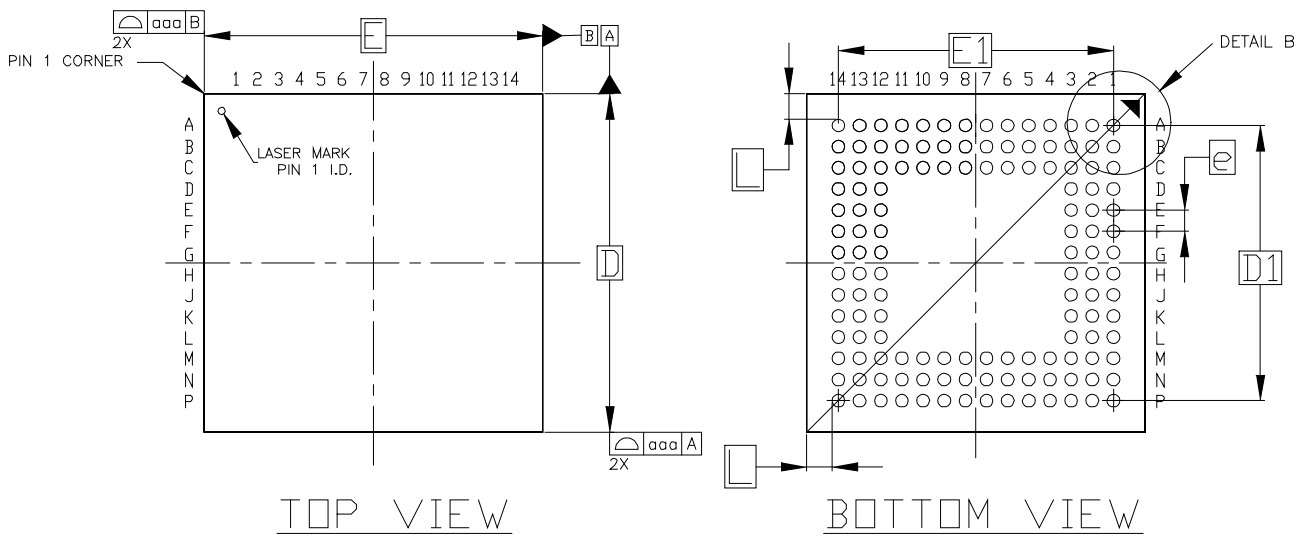
图 4-14 封装尺寸 MG132X
