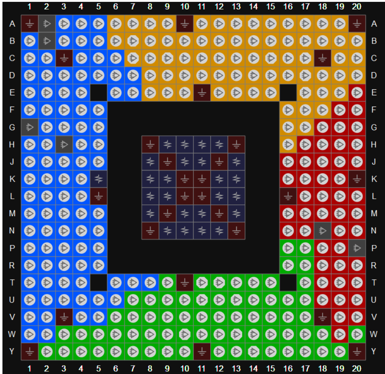
图 3-56 GW1N-9 器件 UG332 管脚分布示意图（顶视图）
