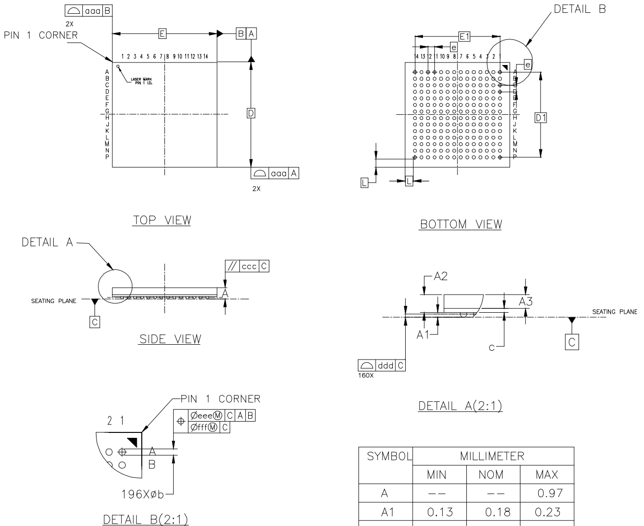
图 4-16 封装尺寸 MG196
