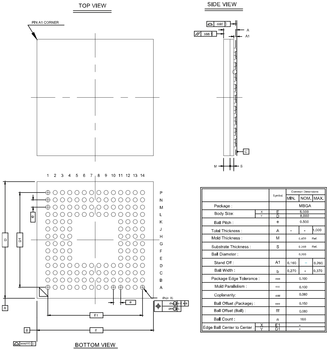
图 4-15 封装尺寸 MG160
