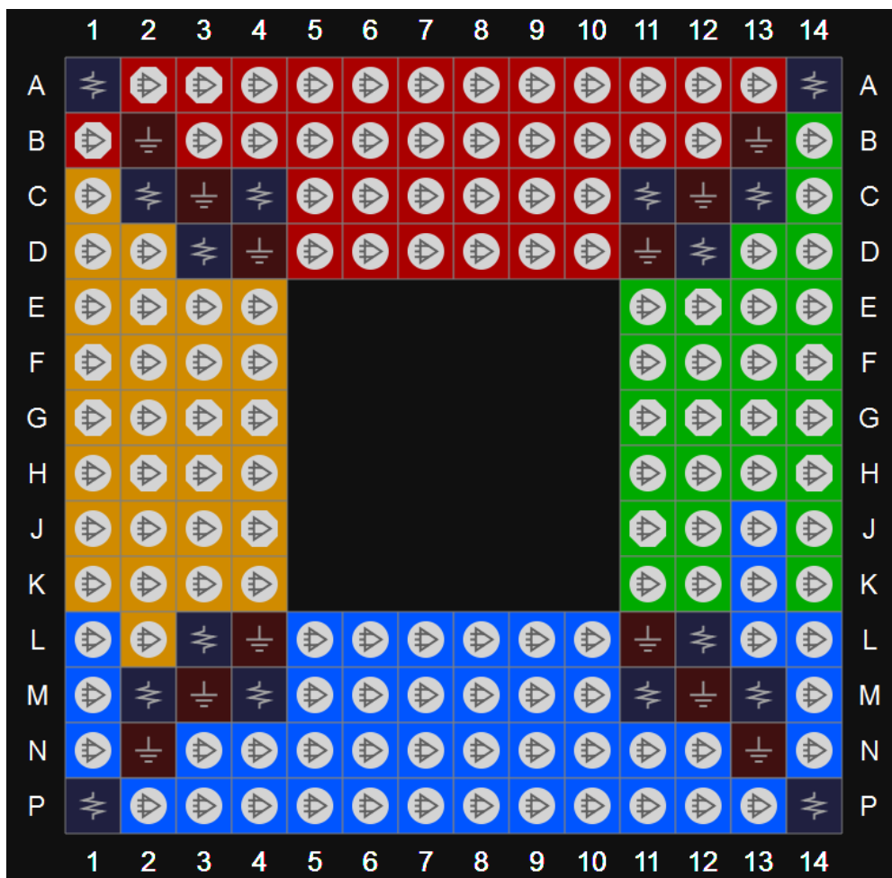
图 3-26 GW1N-4/GW1N-4B 器件 MG160 封装管脚分布示意图（顶视图）
