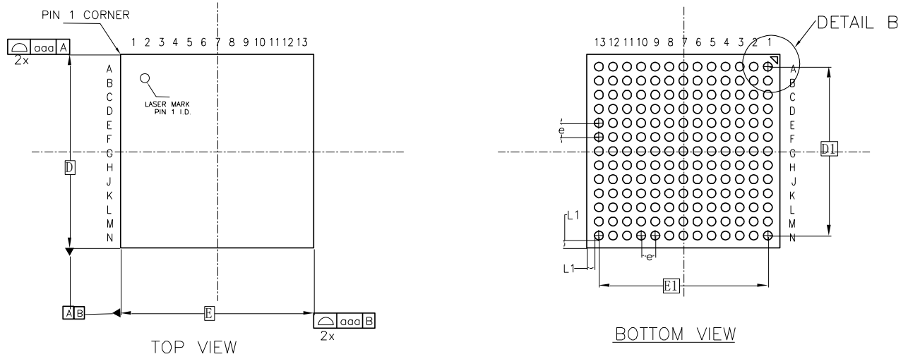
图 4-19 封装尺寸 UG169
