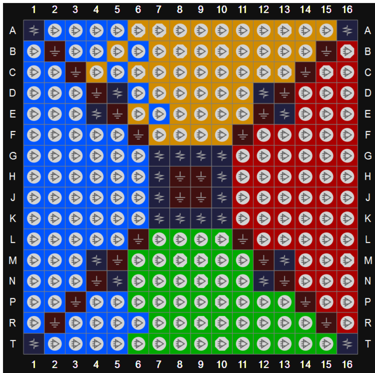
图 3-27 GW1N-4/GW1N-4B 器件 PG256 封装管脚分布示意图（顶视图）
