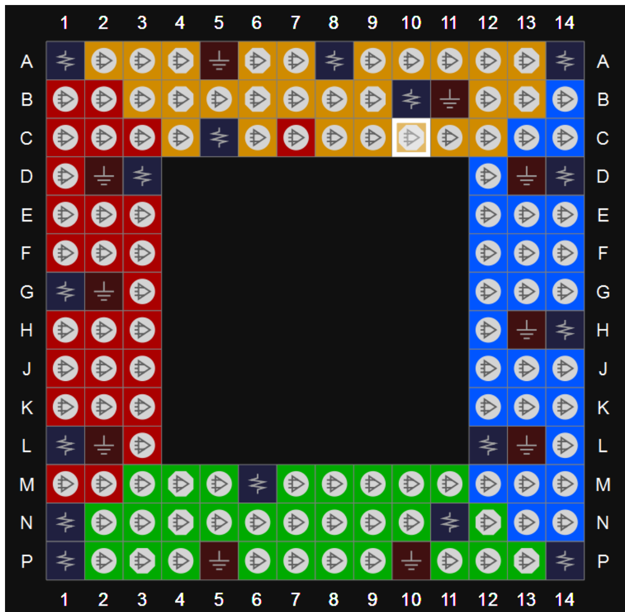
图 3-24 GW1N-4/GW1N-4B 器件 MG132X 封装管脚分布示意图（顶视图）
