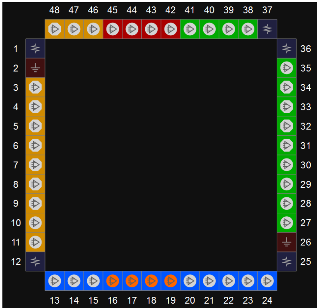
图 3-43 GW1N-9 器件 QN48 封装管脚分布示意图（顶视图）
