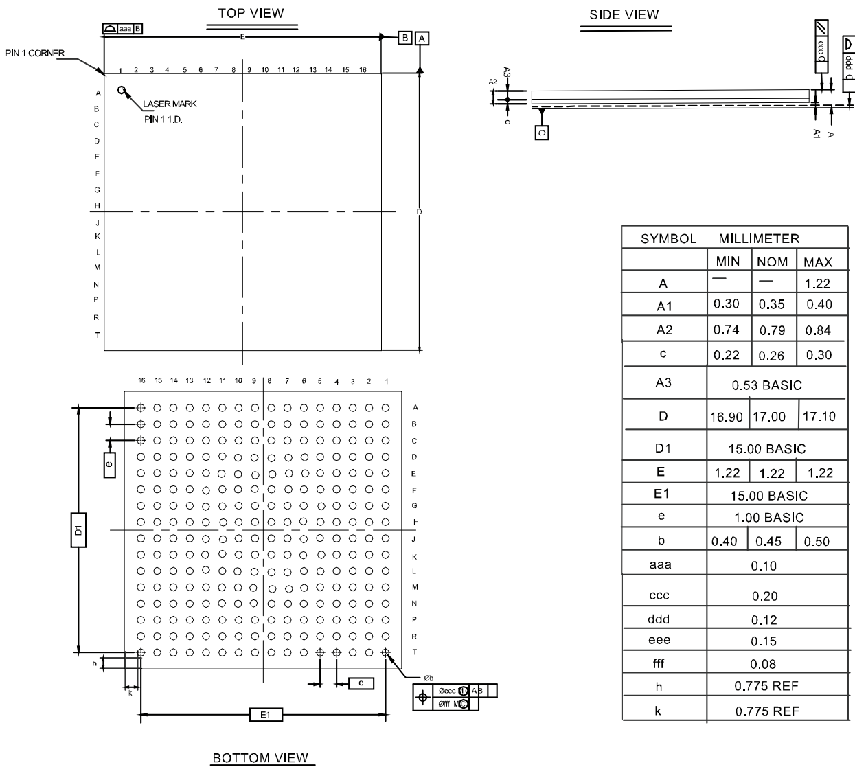
图 4-18 封装尺寸 PG256
