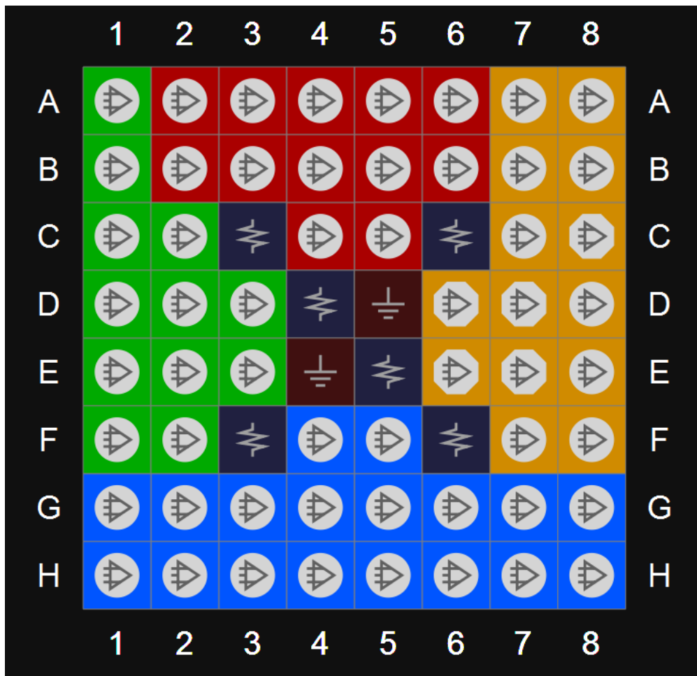
图 3-44 GW1N-9 器件 CM64 封装管脚分布示意图（顶视图）
