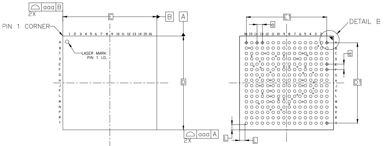
图 4-20 封装尺寸 UG256
