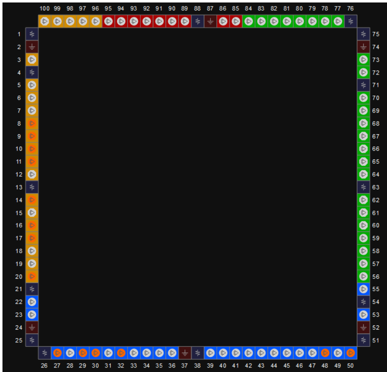
图 3-46 GW1N-9 器件 LQ100 封装管脚分布示意图（顶视图）
