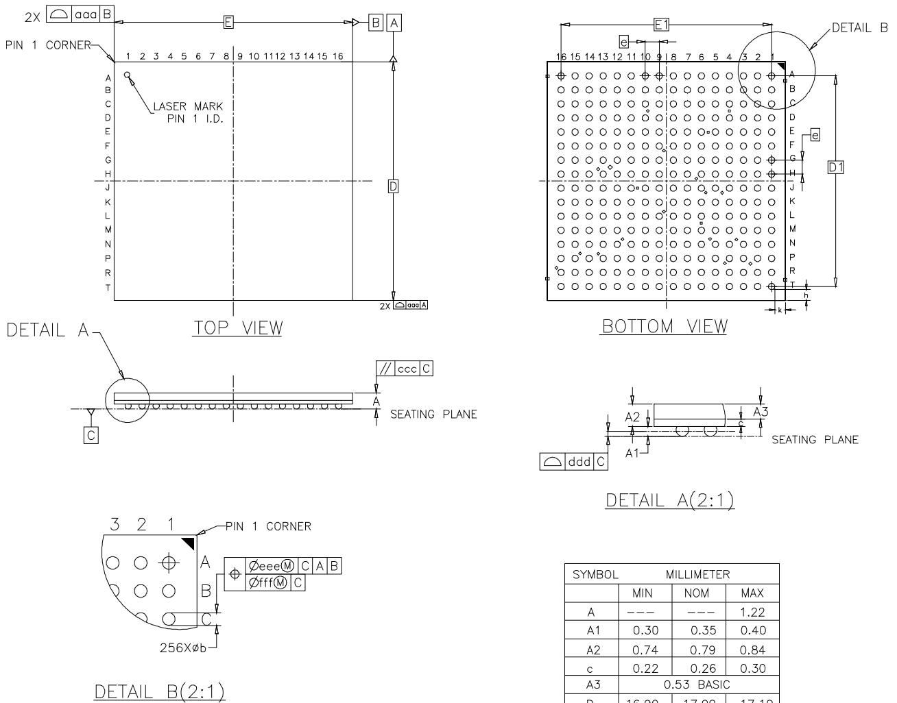
图 4-17 封装尺寸 PG256M
