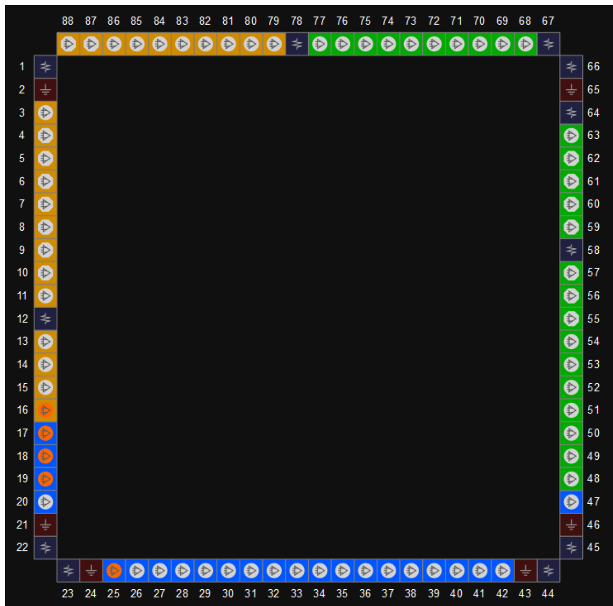
图 3-31 GW1N-6 器件 QN88 封装管脚分布示意图（顶视图）
