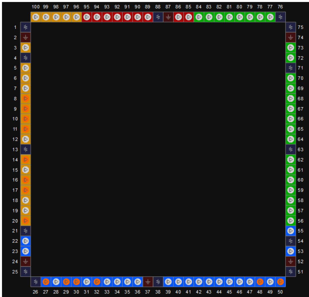
图 3-32 GW1N-6 器件 LQ100 封装管脚分布示意图（顶视图）
