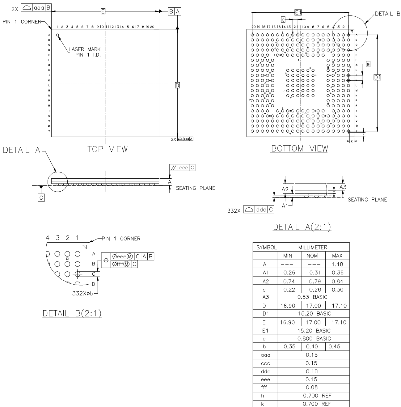
图 4-21 封装尺寸 UG332
