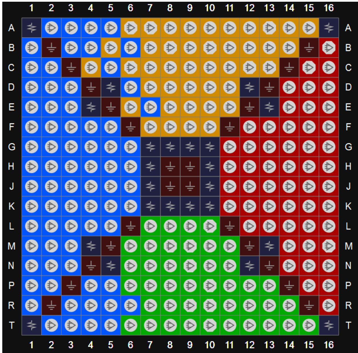
图 3-40 GW1N-4 器件 PG256 封装管脚分布示意图（顶视图）
