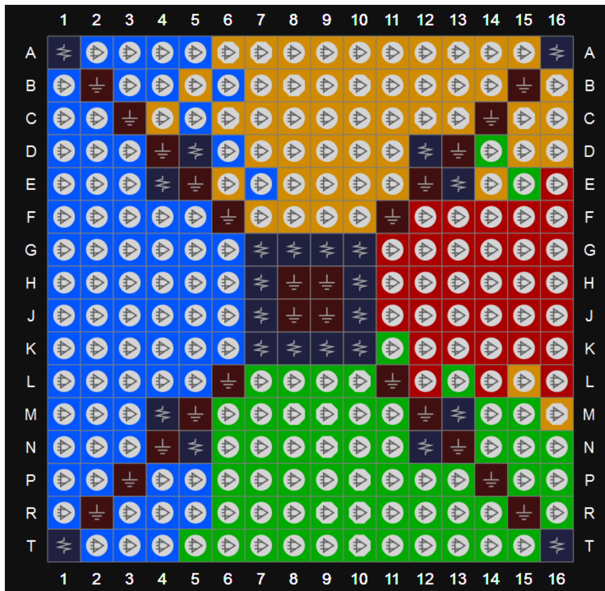
图 3-55 GW1N-9 器件 PG256 封装管脚分布示意图（顶视图）
