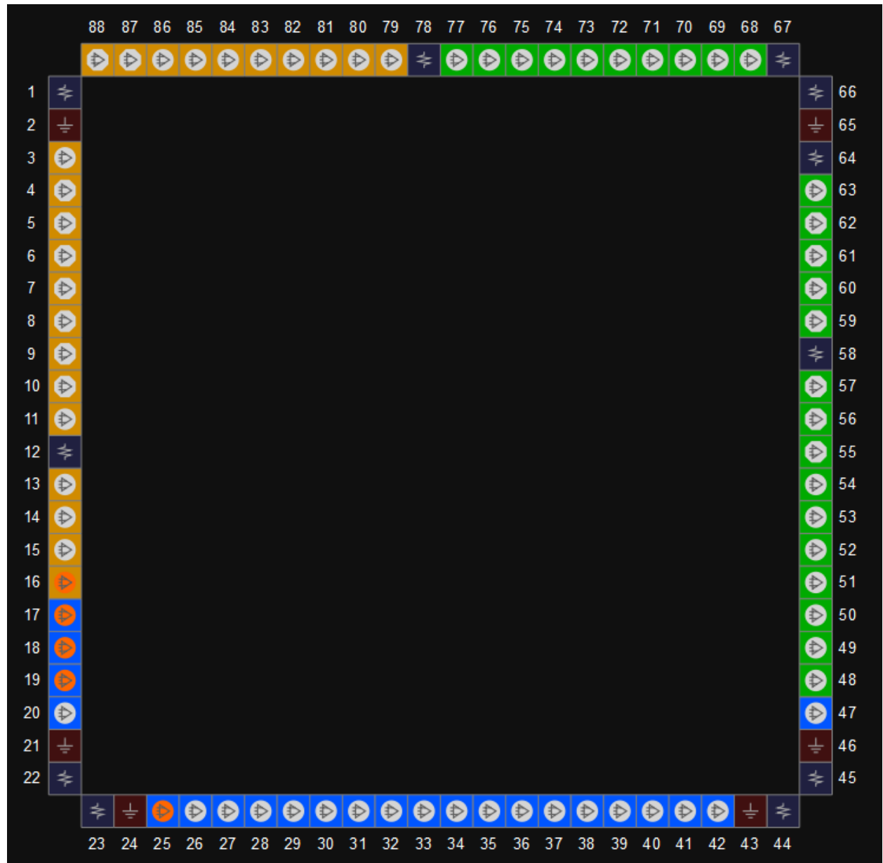
图 3-45 GW1N-9 器件 QN88 封装管脚分布示意图（顶视图）
