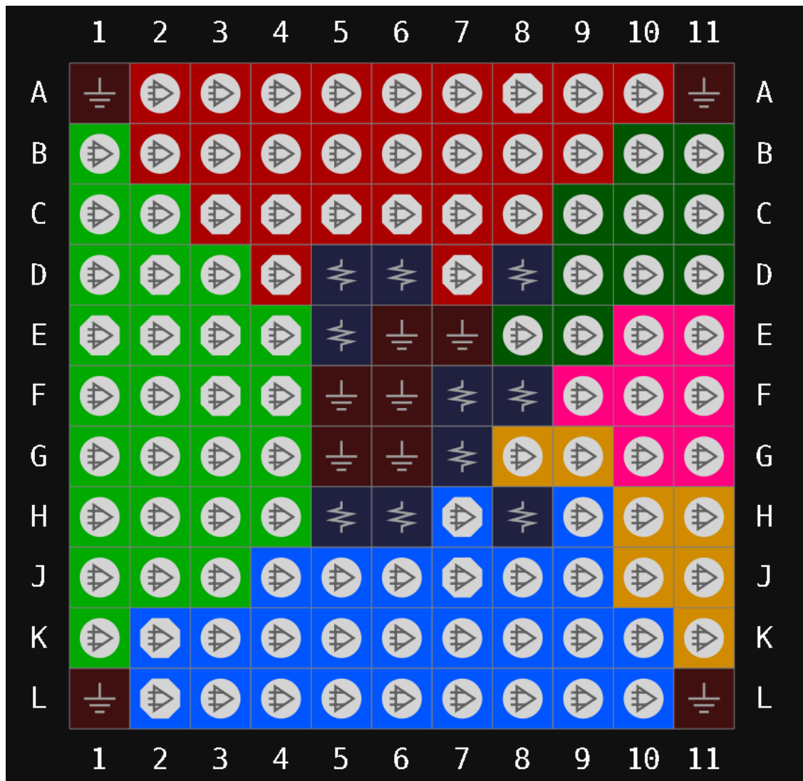
图 3-25 GW1N-2 器件 MG121 封装管脚分布示意图 (UV 版本 顶视图)
