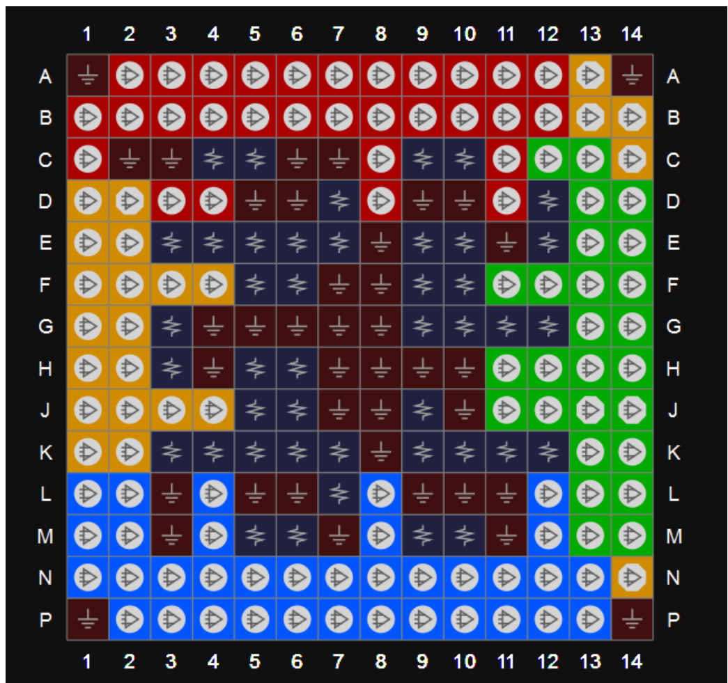
图 3-54 GW1N-9 器件 MG196 封装管脚分布示意图（顶视图）
