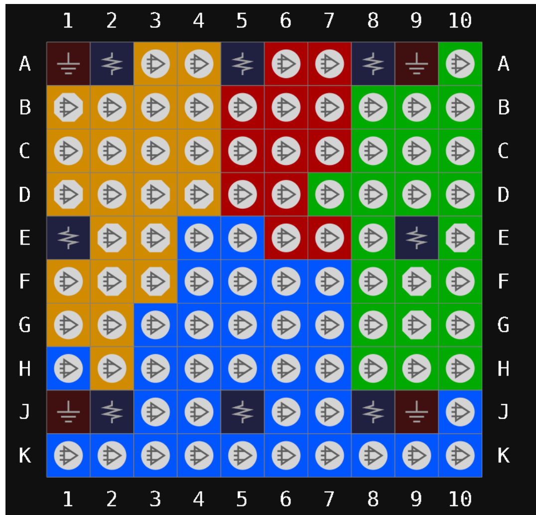
图 3-59 GW1N-9 器件 MG100T 管脚分布示意图（顶视图）
