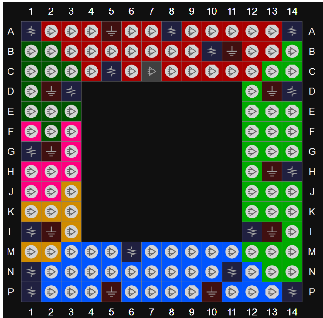
图 3-22 GW1N-2 器件 MG132 封装管脚分布示意图 (UV 版本 顶视图)
