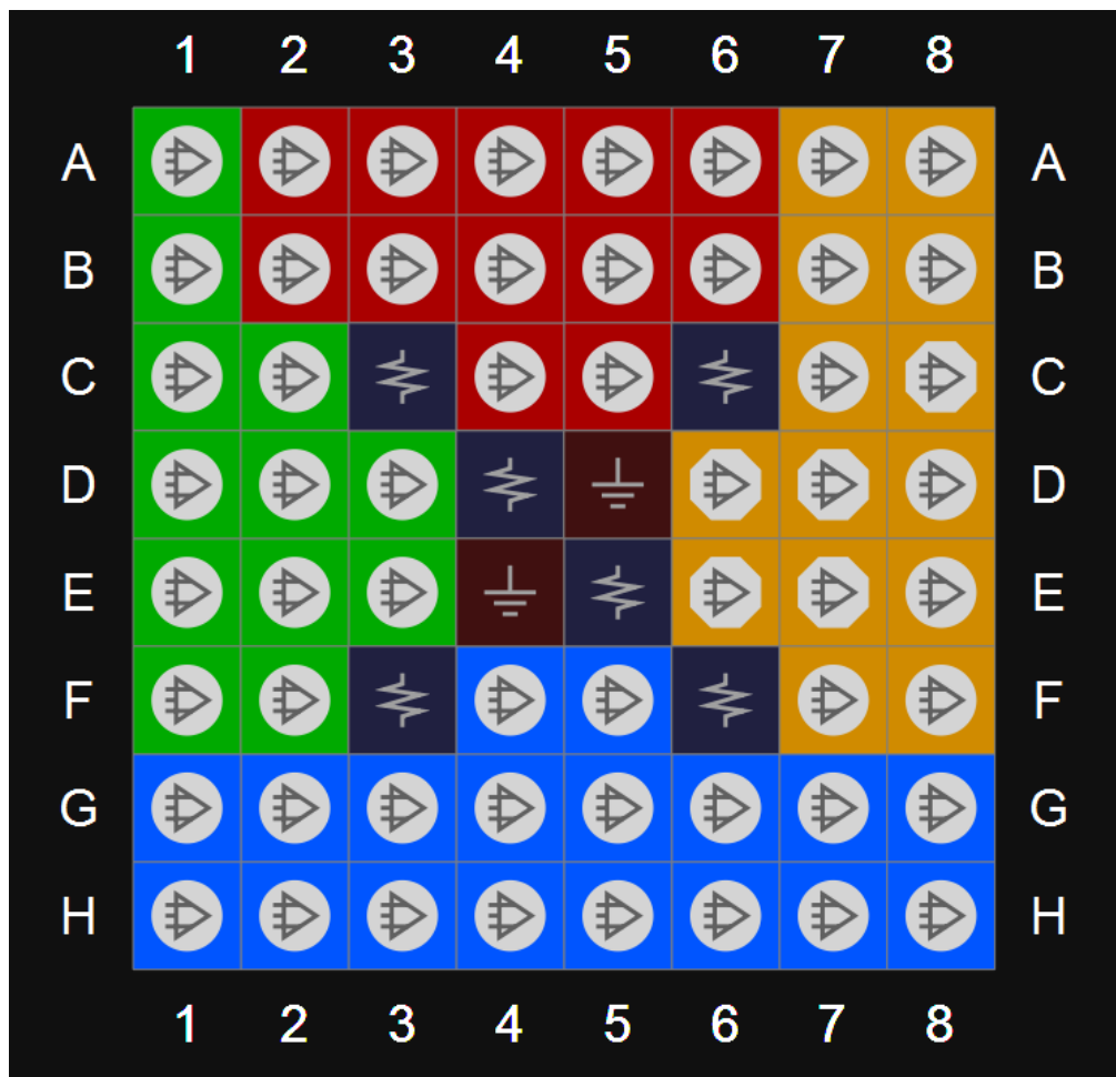
图 3-43 GW1N-9 器件 CM64 封装管脚分布示意图（顶视图）
