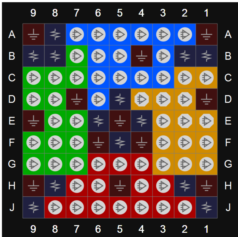
图 3-44 GW1N-9 器件 CS81M 封装管脚分布示意图（顶视图）
