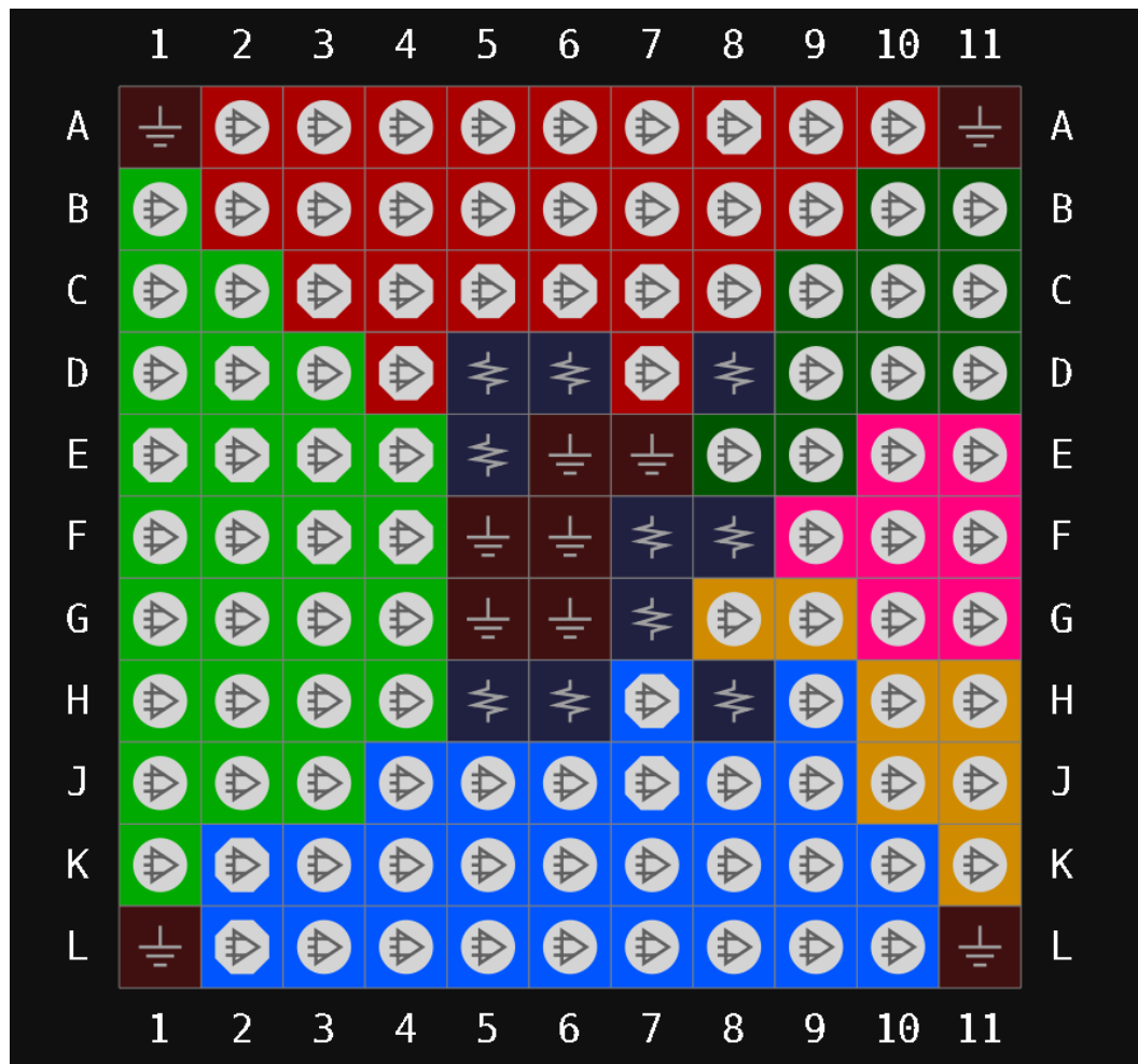
图 3-24 GW1N-2 器件 MG121 封装管脚分布示意图 (LV 版本 顶视图)
