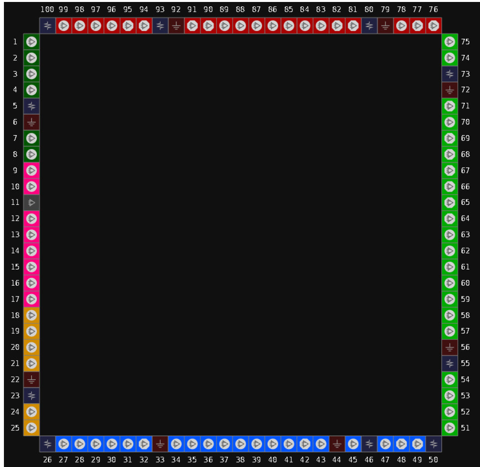
图 3-28 GW1N-1P5 器件 LQ100X 封装管脚分布示意图 (LV 版本顶视图)
