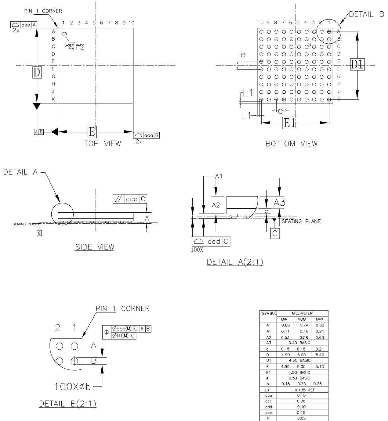
图 4-16 封装尺寸 MG100/ MG100T
