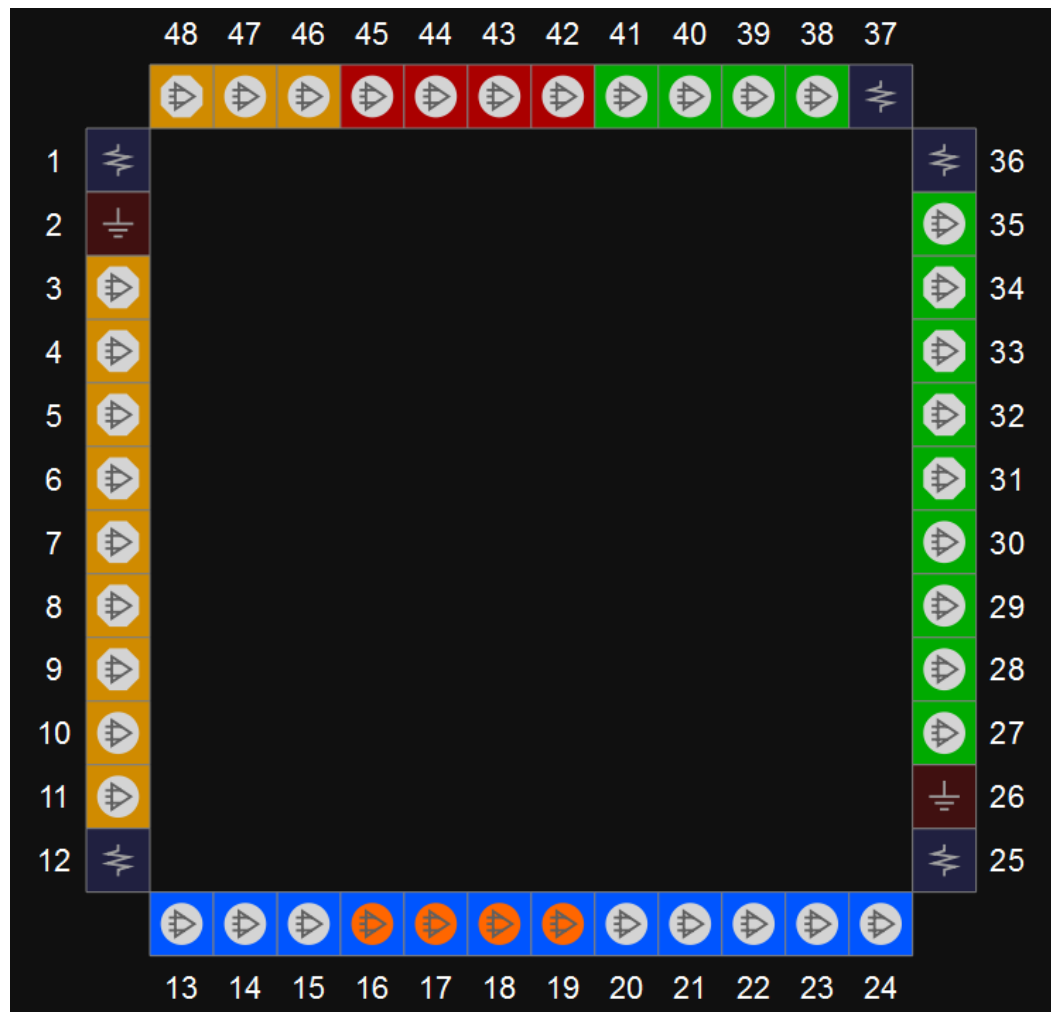
图 3-42 GW1N-9 器件 QN48 封装管脚分布示意图（顶视图）
