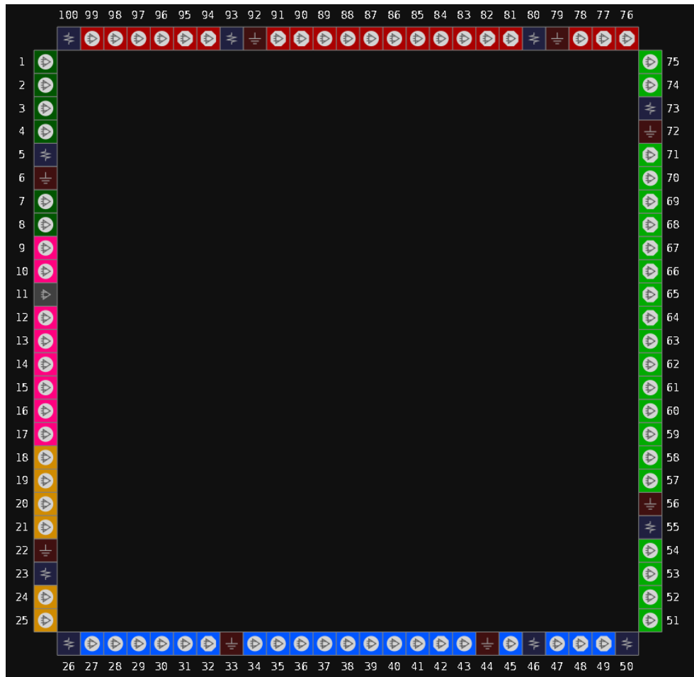
图 3-30 GW1N-1P5 器件 LQ100 封装管脚分布示意图 (LV 版本顶视图)
