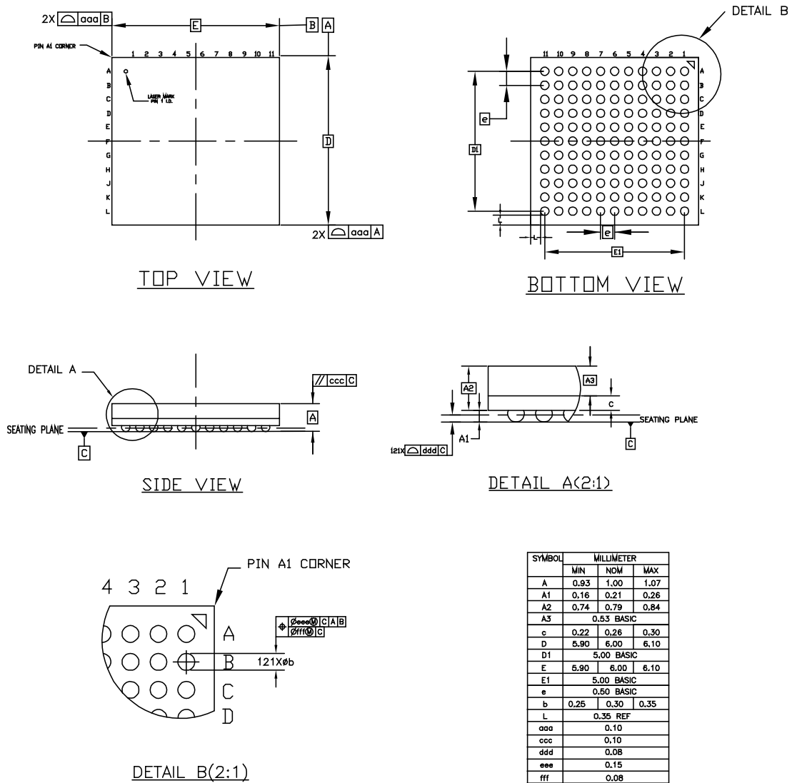
图 4-17 封装尺寸 MG121/ MG121X
