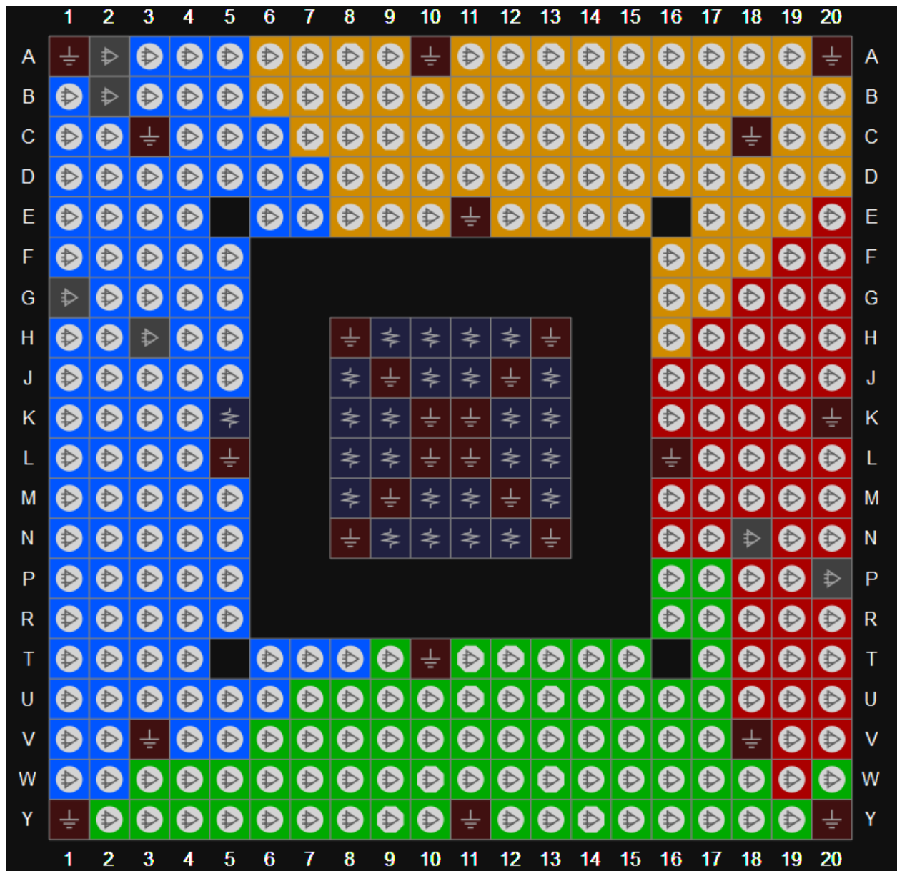
图 3-57 GW1N-9 器件 UG332 管脚分布示意图（顶视图）
