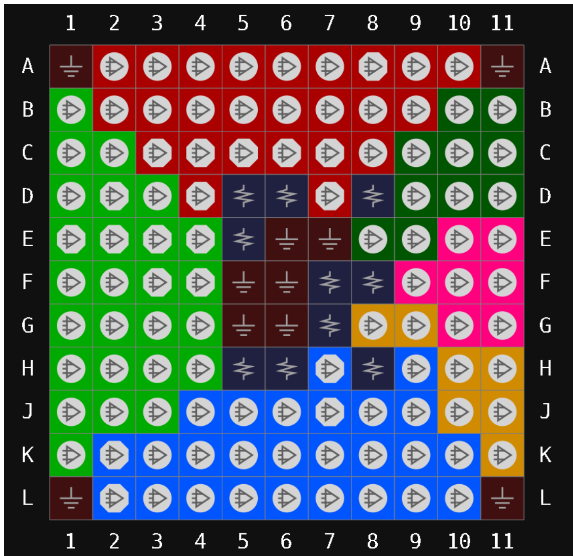
图 3-27 GW1N-2 器件 MG121X 封装管脚分布示意图（UV 版本 顶视图）
