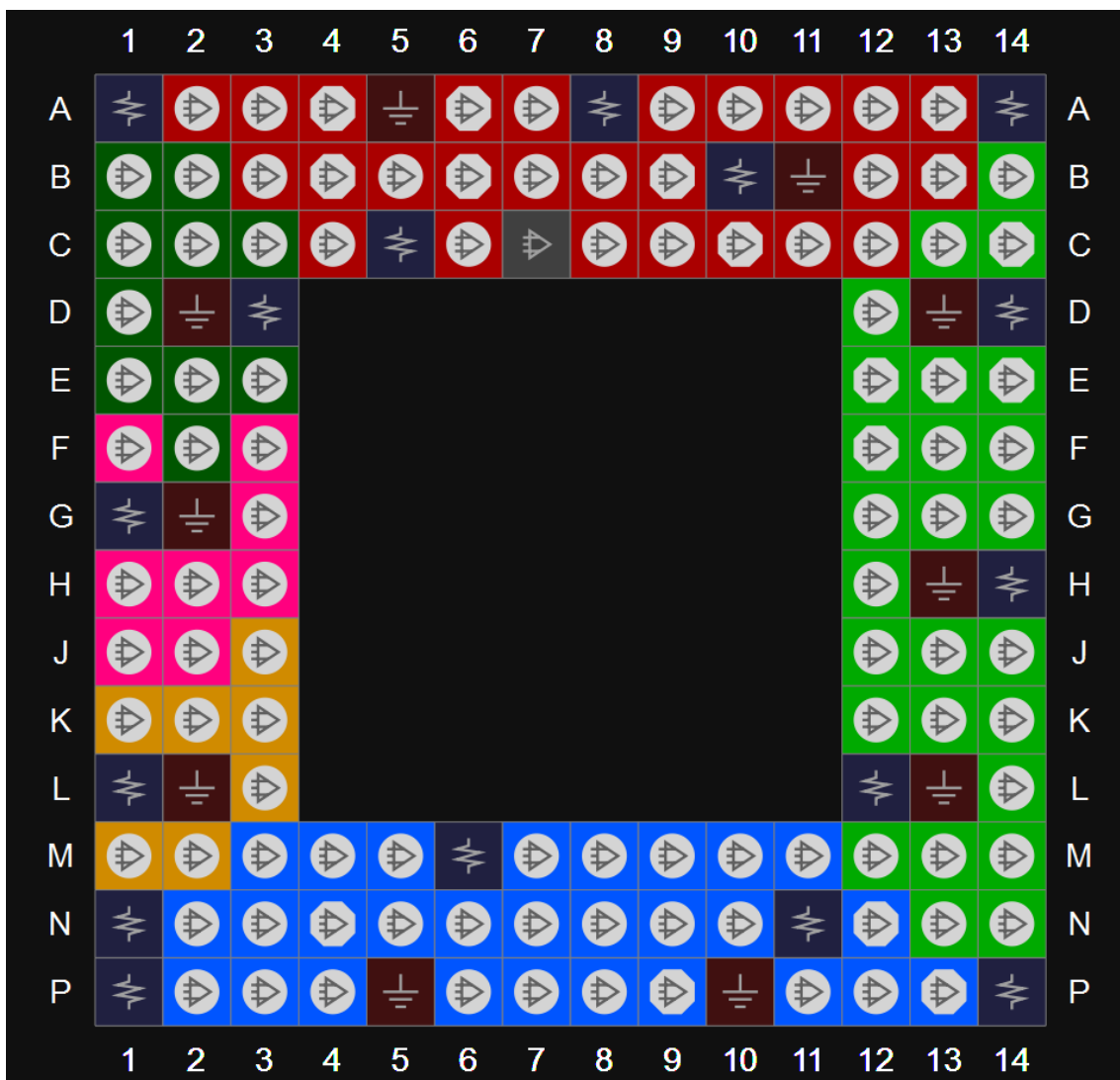
图 3-23 GW1N-2 器件 MG132 封装管脚分布示意图 (LV 版本 顶视图)
