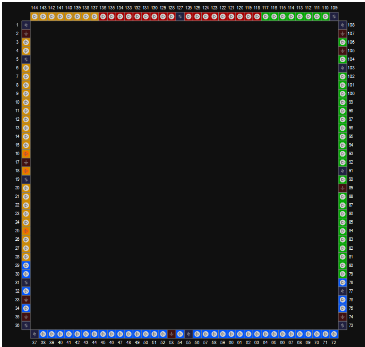
图 3-48 GW1N-9 器件 LQ144 封装管脚分布示意图（顶视图）
