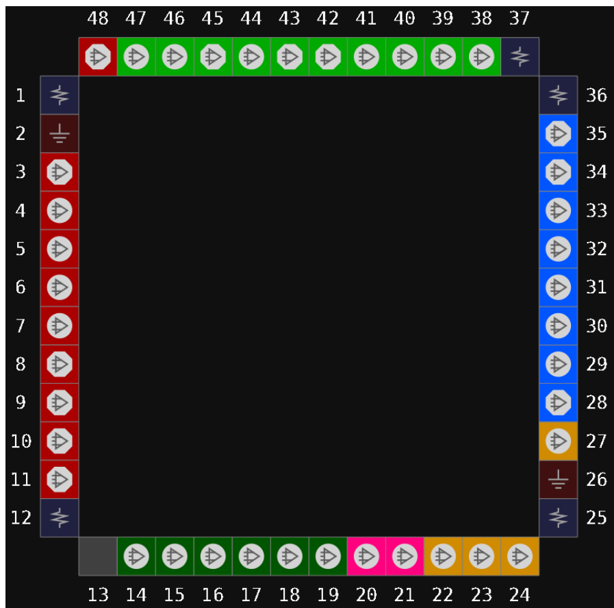
图 3-19 GW1N-2 器件 QN48 封装管脚分布示意图（顶视图）
