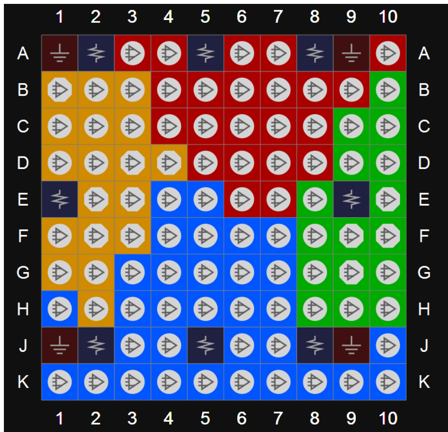
图 3-47 GW1N-9 器件 MG100 封装管脚分布示意图（顶视图）
