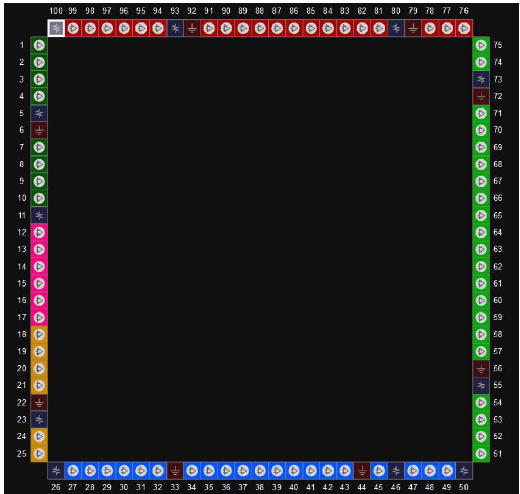
图 3-11 GW1N-2 器件 LQ100X 封装管脚分布示意图（UV 版本,顶视图）
