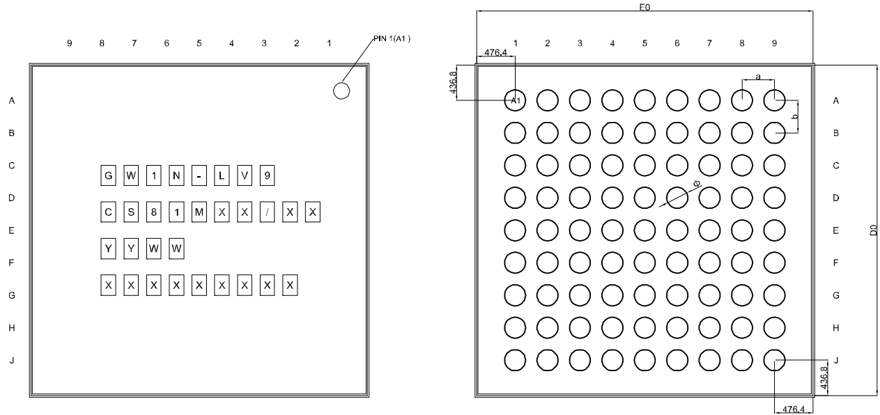
图 4-9 封装尺寸 CS81M
