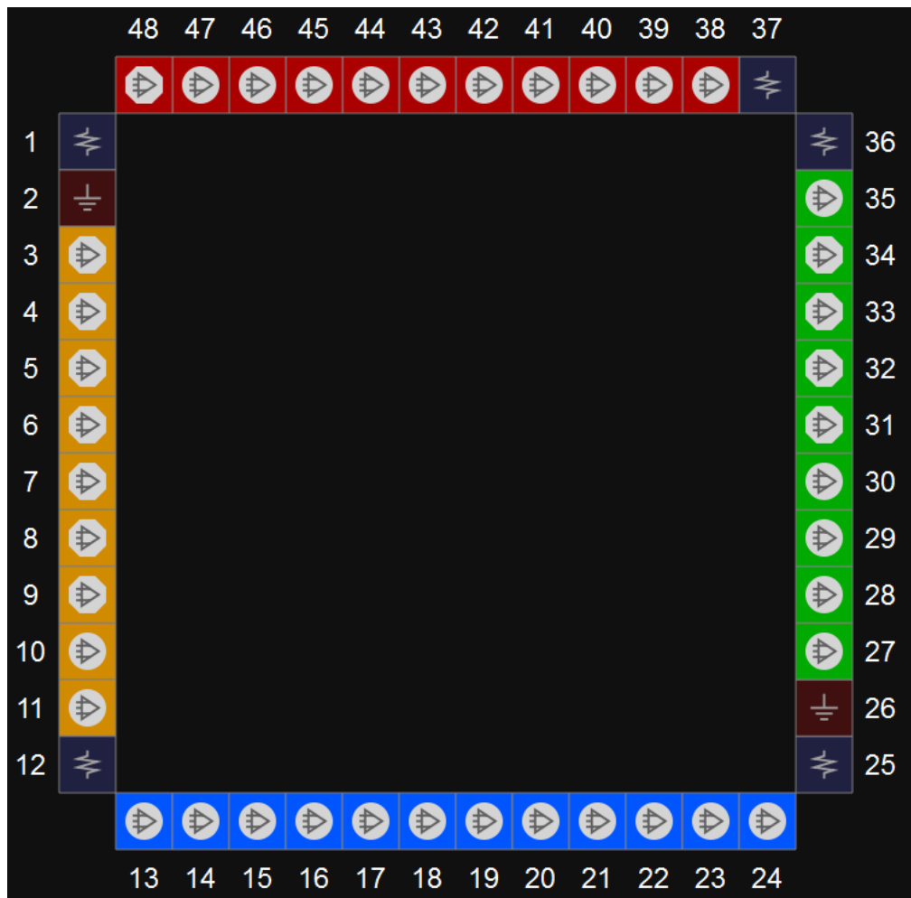
图 3-33 GW1N-4 器件 QN48 封装管脚分布示意图（顶视图）
