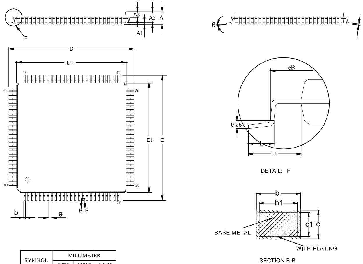
图 4-11 封装尺寸 LQ100/LQ100X
