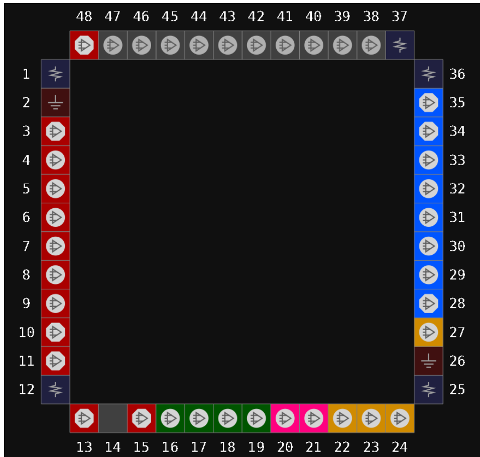
图 3-20 GW1N-2 器件 QN48H 封装管脚分布示意图（顶视图）
