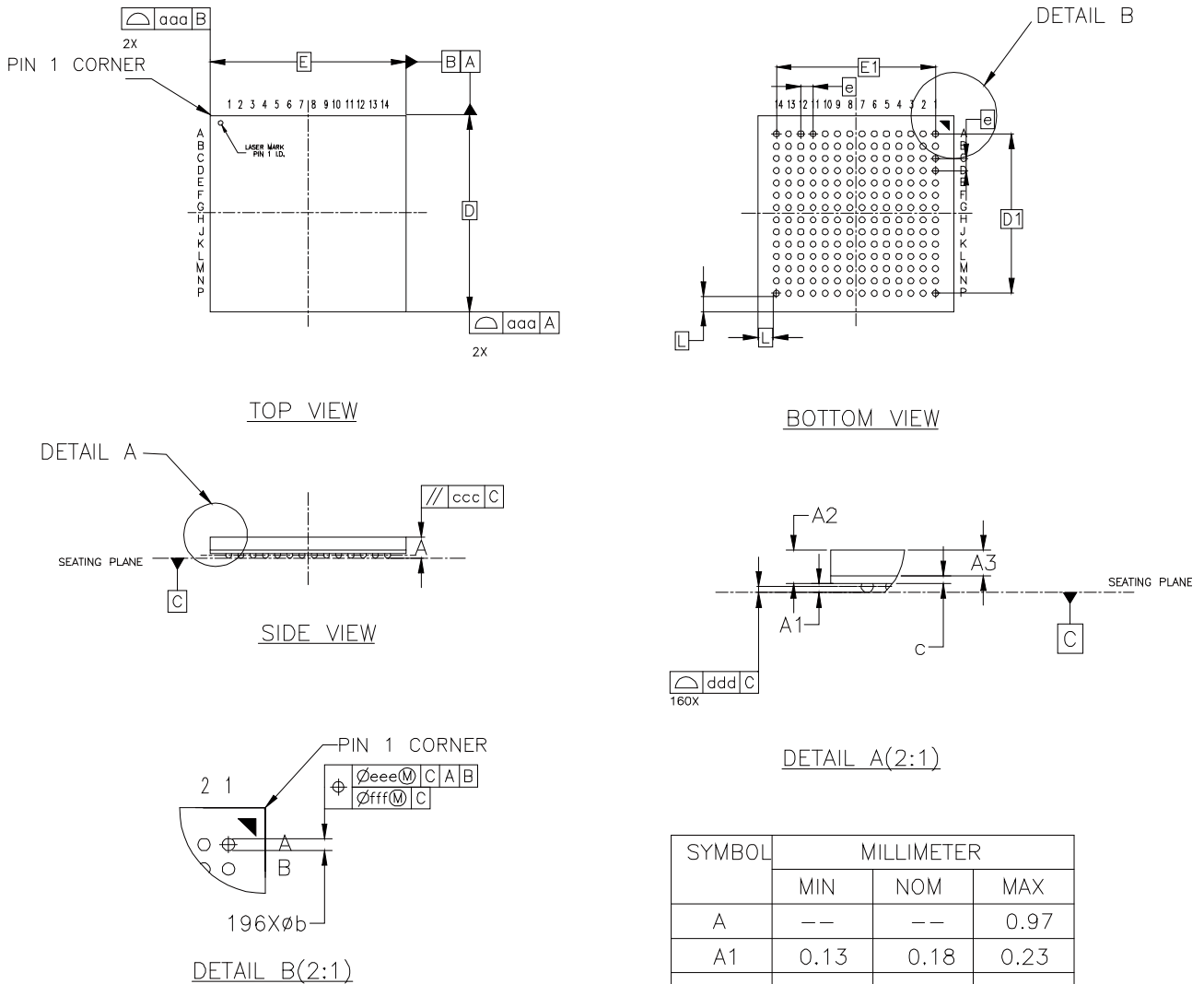
图 4-20 封装尺寸 MG196
