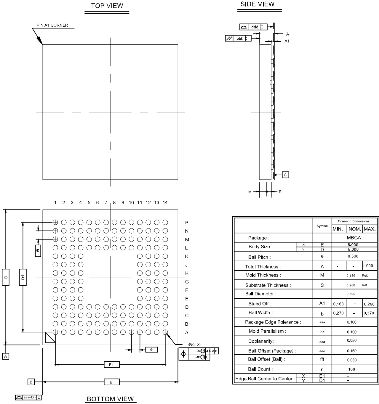
图 4-19 封装尺寸 MG160
