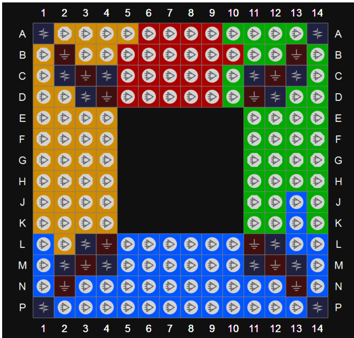
图 3-50 GW1N-9 器件 MG160 封装管脚分布示意图（顶视图）
