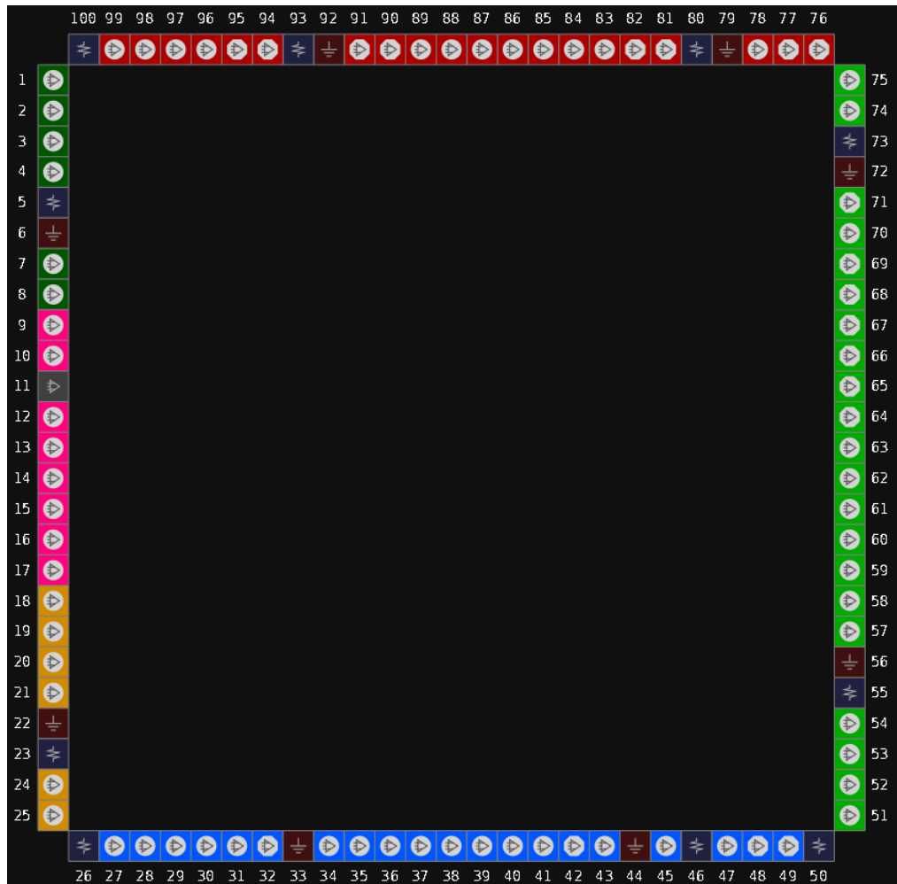
图 3-29 GW1N-1P5 器件 LQ100X 封装管脚分布示意图 (UV 版本顶视图)
