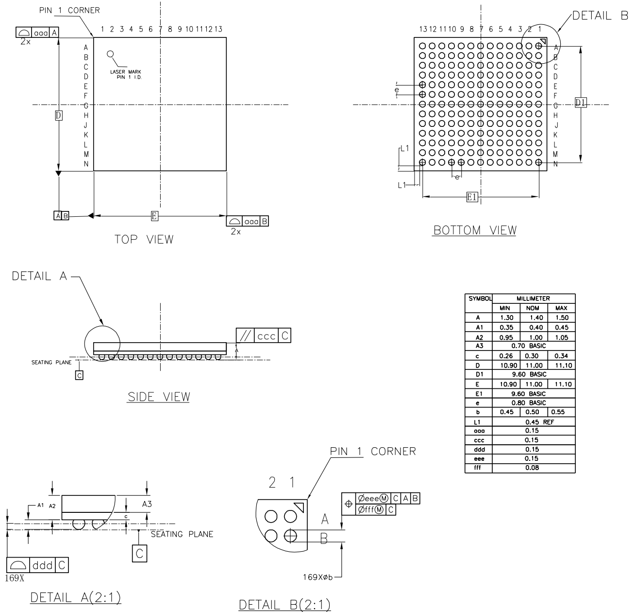
图 4-23 封装尺寸 UG169
