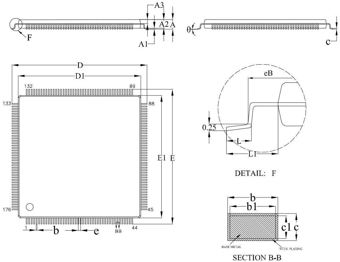
图 4-14 封装尺寸 LQ176
