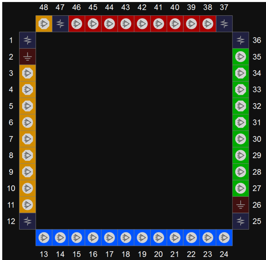
图 3-58 GW1N-9 器件 QN48F 管脚分布示意图（顶视图）
