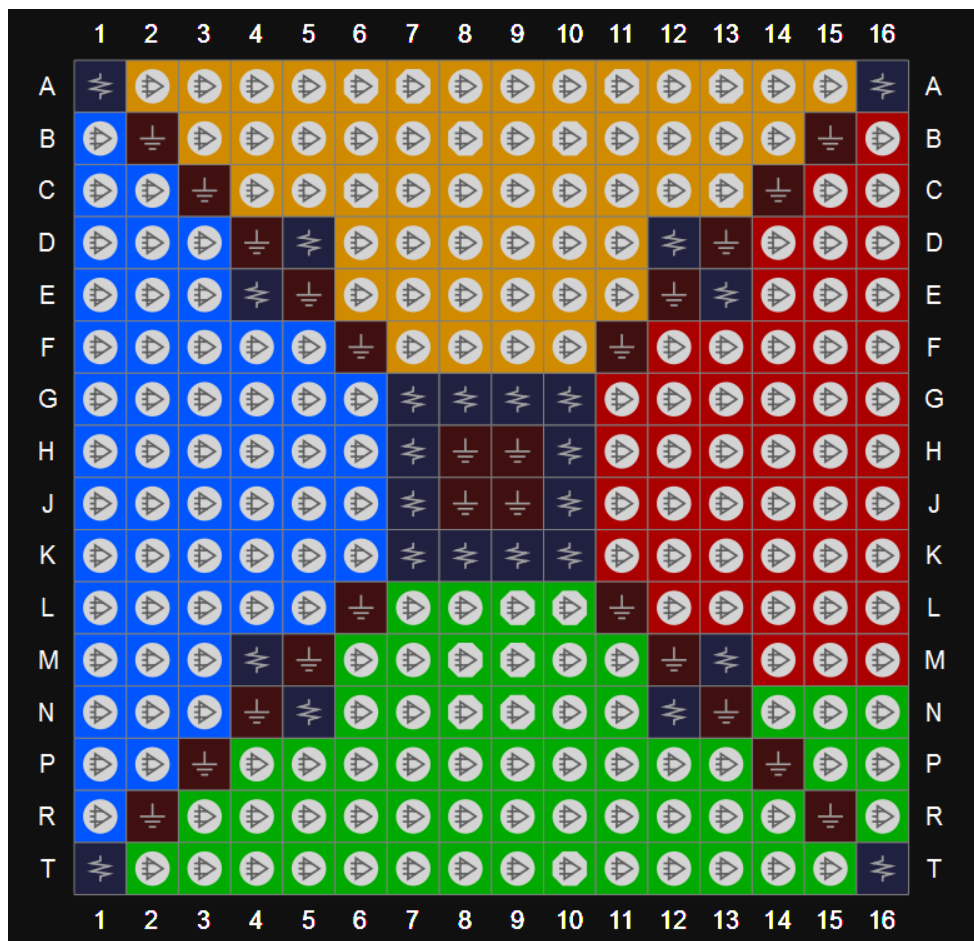
图 3-56 GW1N-9 器件 UG256 封装管脚分布示意图（顶视图）
