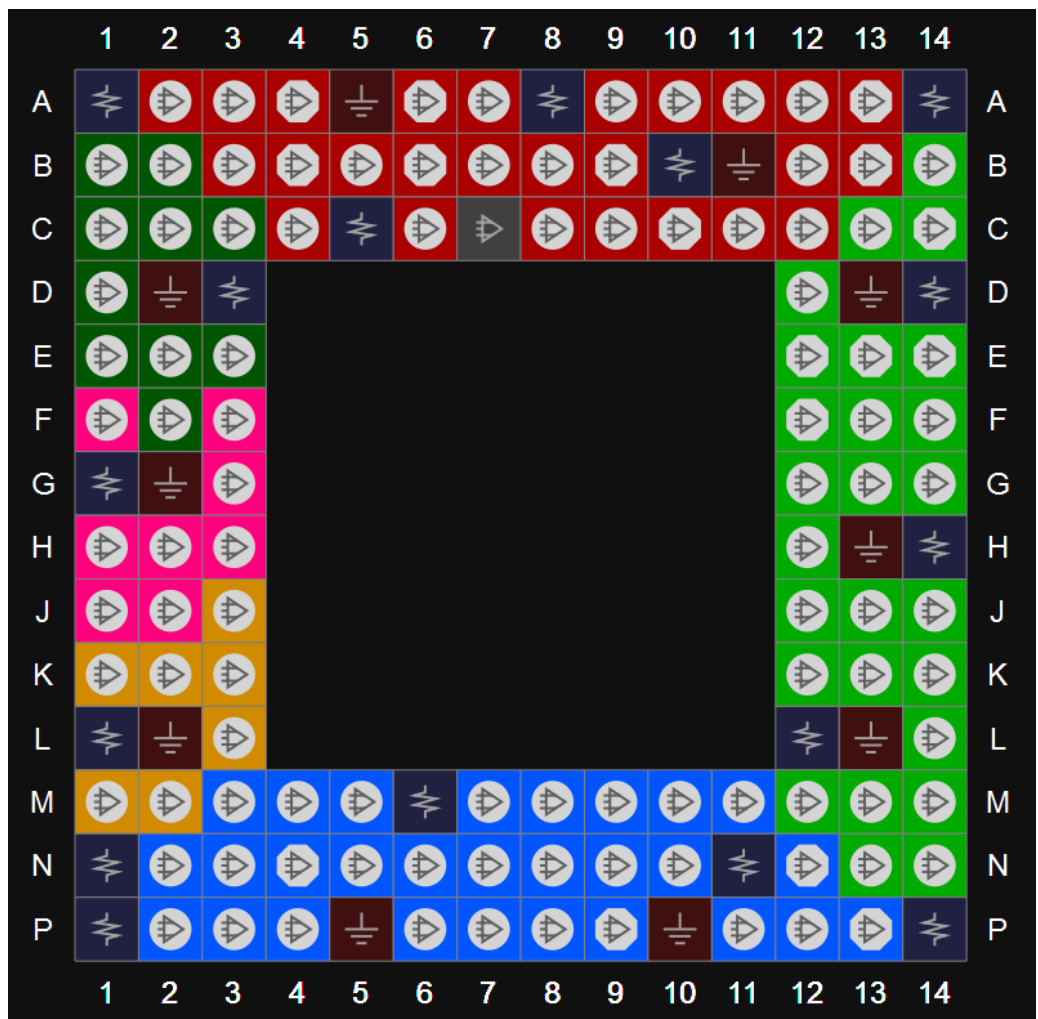
图 3-9 GW1N-2 器件 MG132X 封装管脚分布示意图（UV 版本,顶视图）
