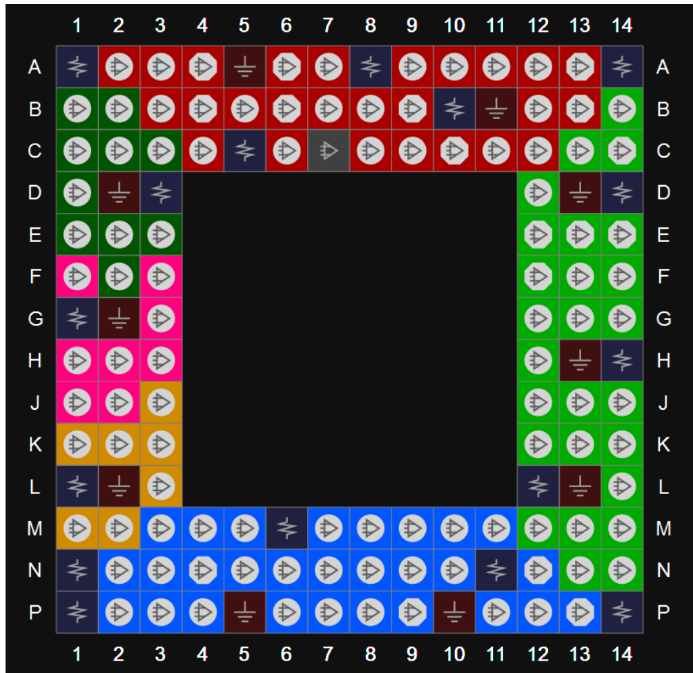
图 3-10 GW1N-2 器件 MG132X 封装管脚分布示意图（LV 版本,顶视图）
