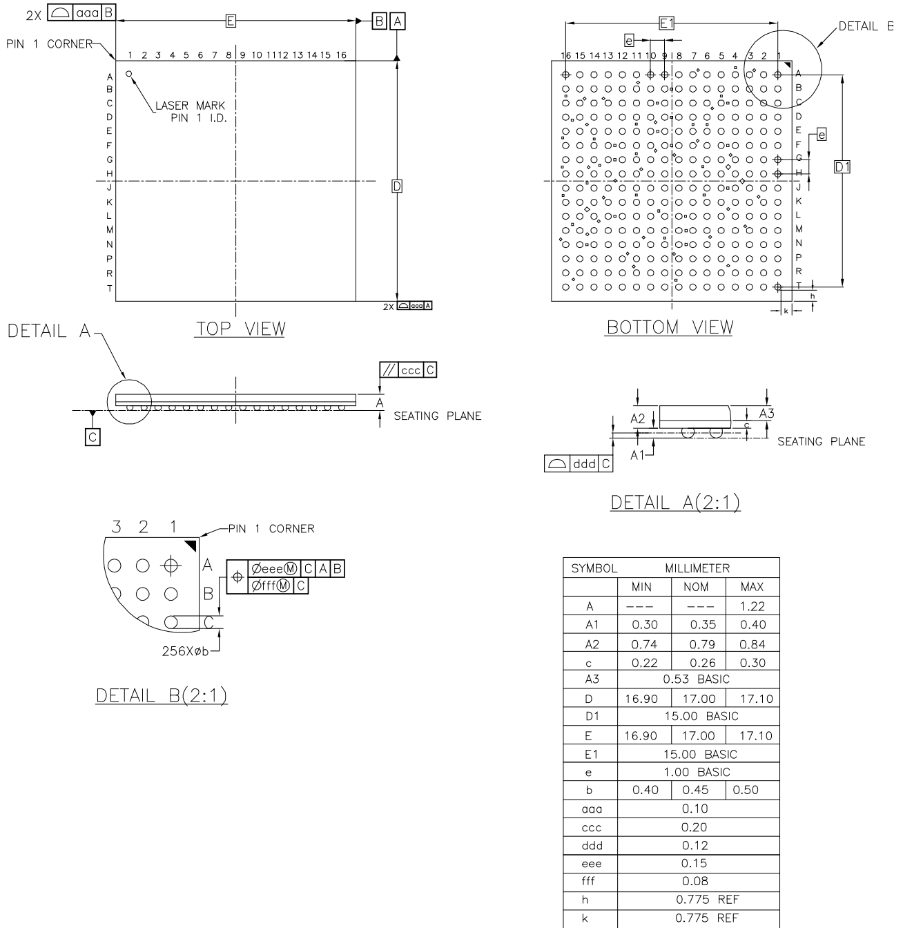
图 4-21 封装尺寸 PG256
