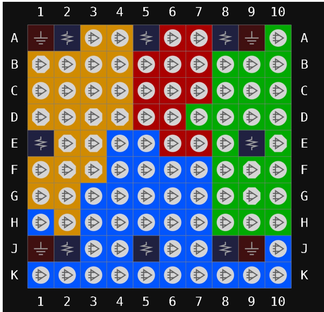
图 3-55 GW1N-9 器件 MG100T 管脚分布示意图（顶视图）
