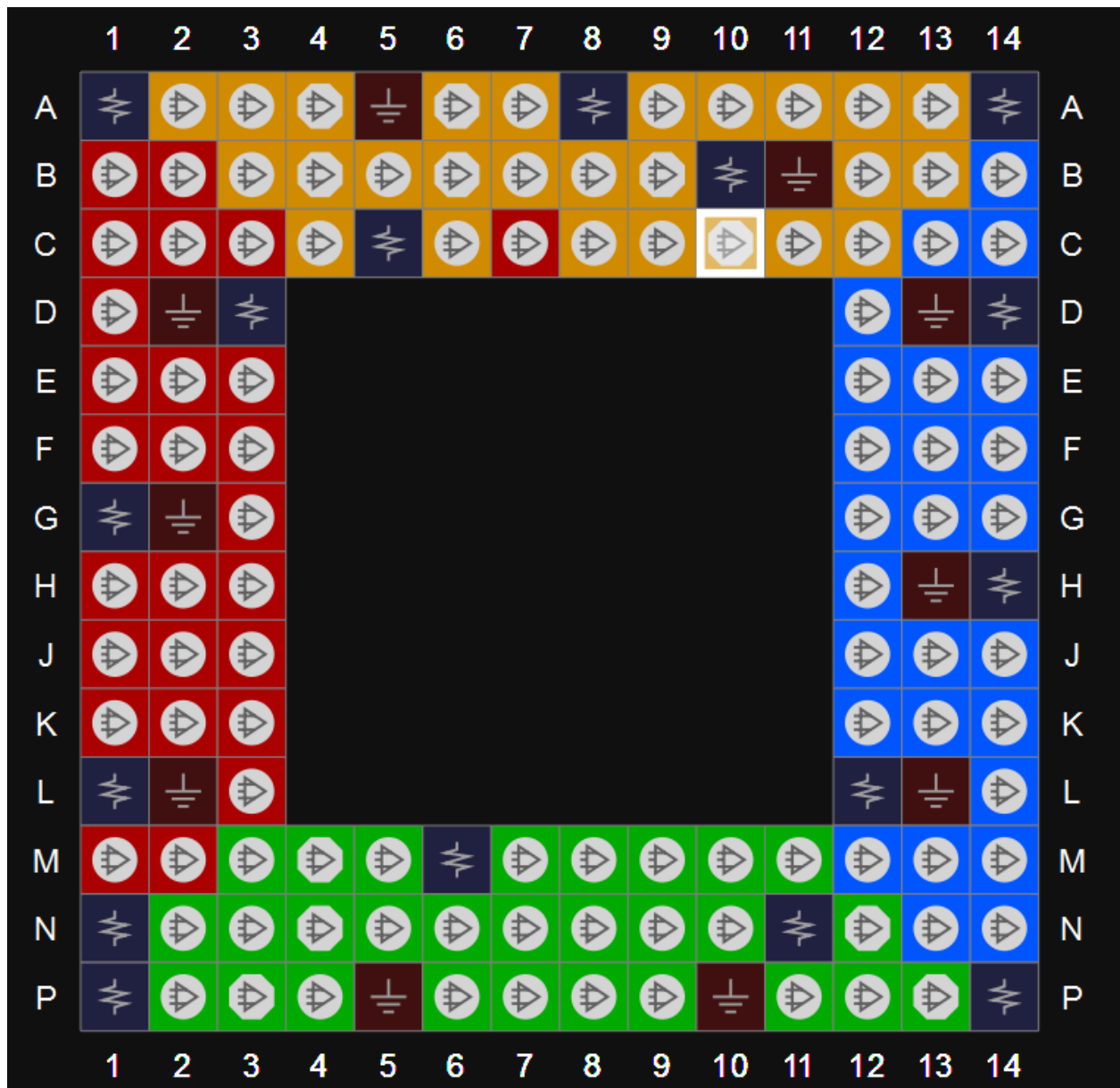
图 3-33 GW1N-4 器件 MG132X 封装管脚分布示意图（顶视图）
