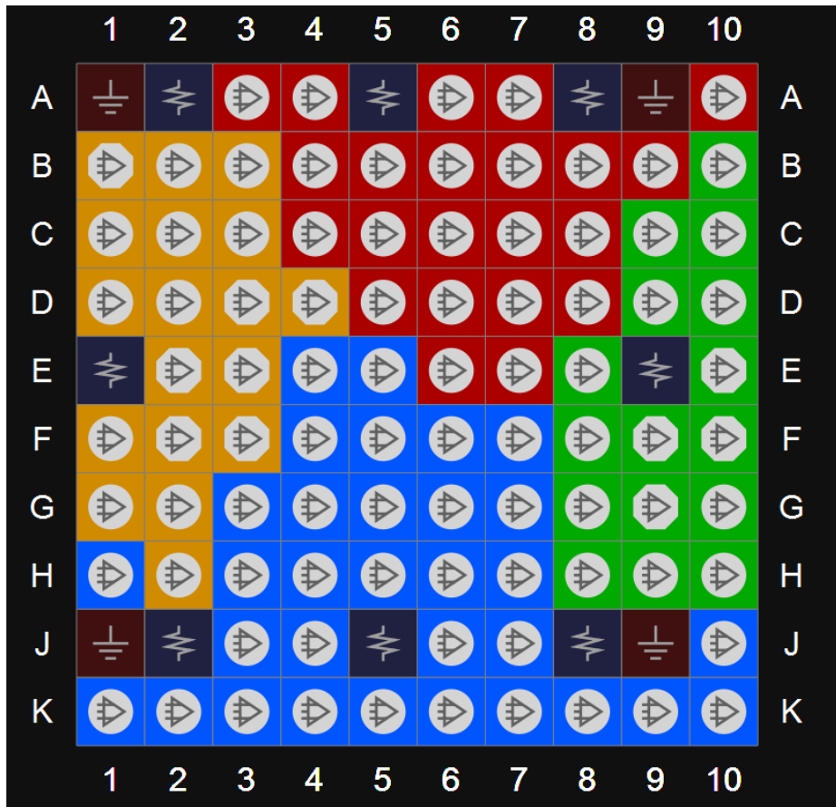
图 3-43 GW1N-9 器件 MG100 封装管脚分布示意图（顶视图）
