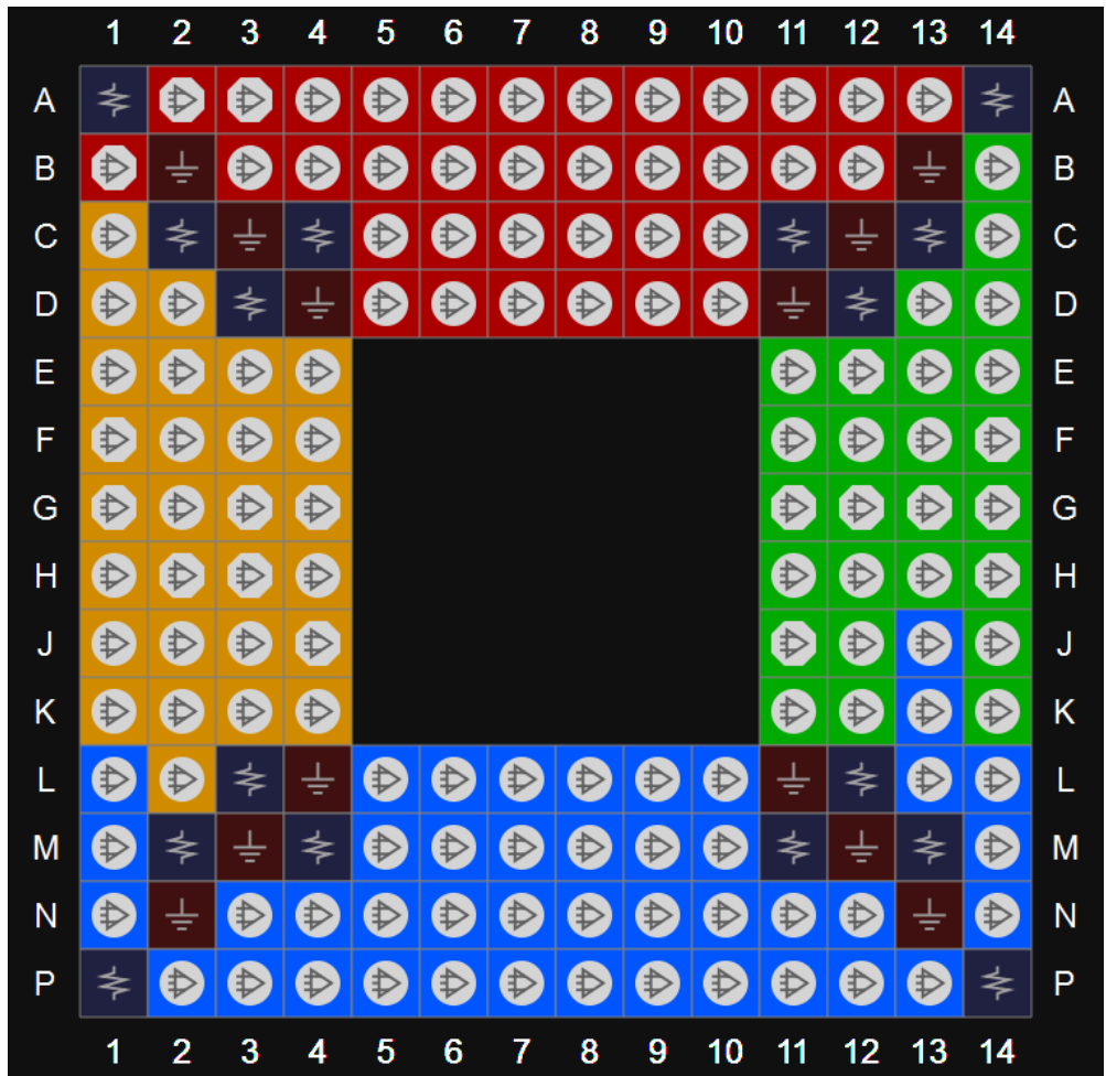
图 3-35 GW1N-4 器件 MG160 封装管脚分布示意图（顶视图）
