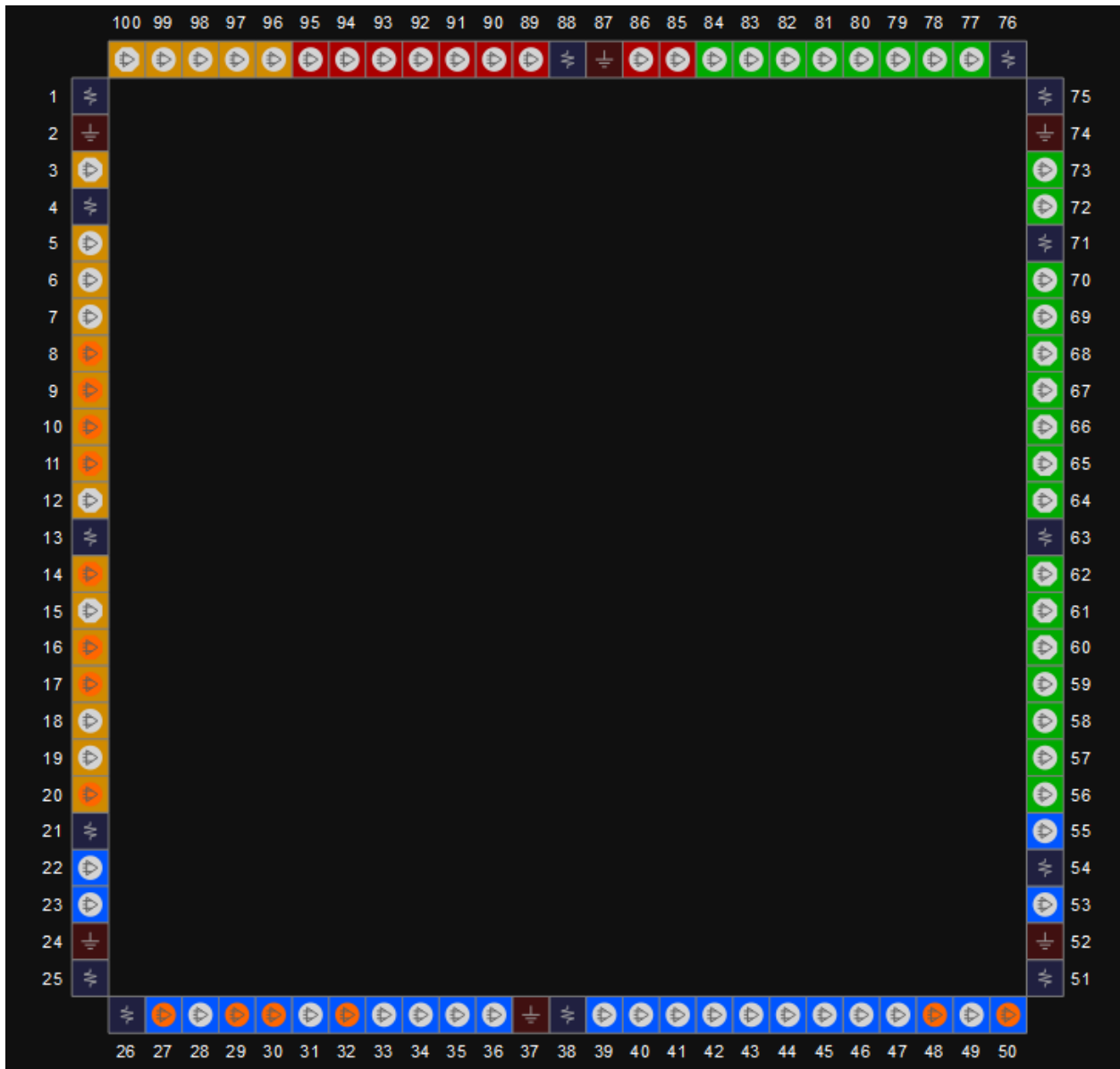
图 3-42 GW1N-9 器件 LQ100 封装管脚分布示意图（顶视图）
