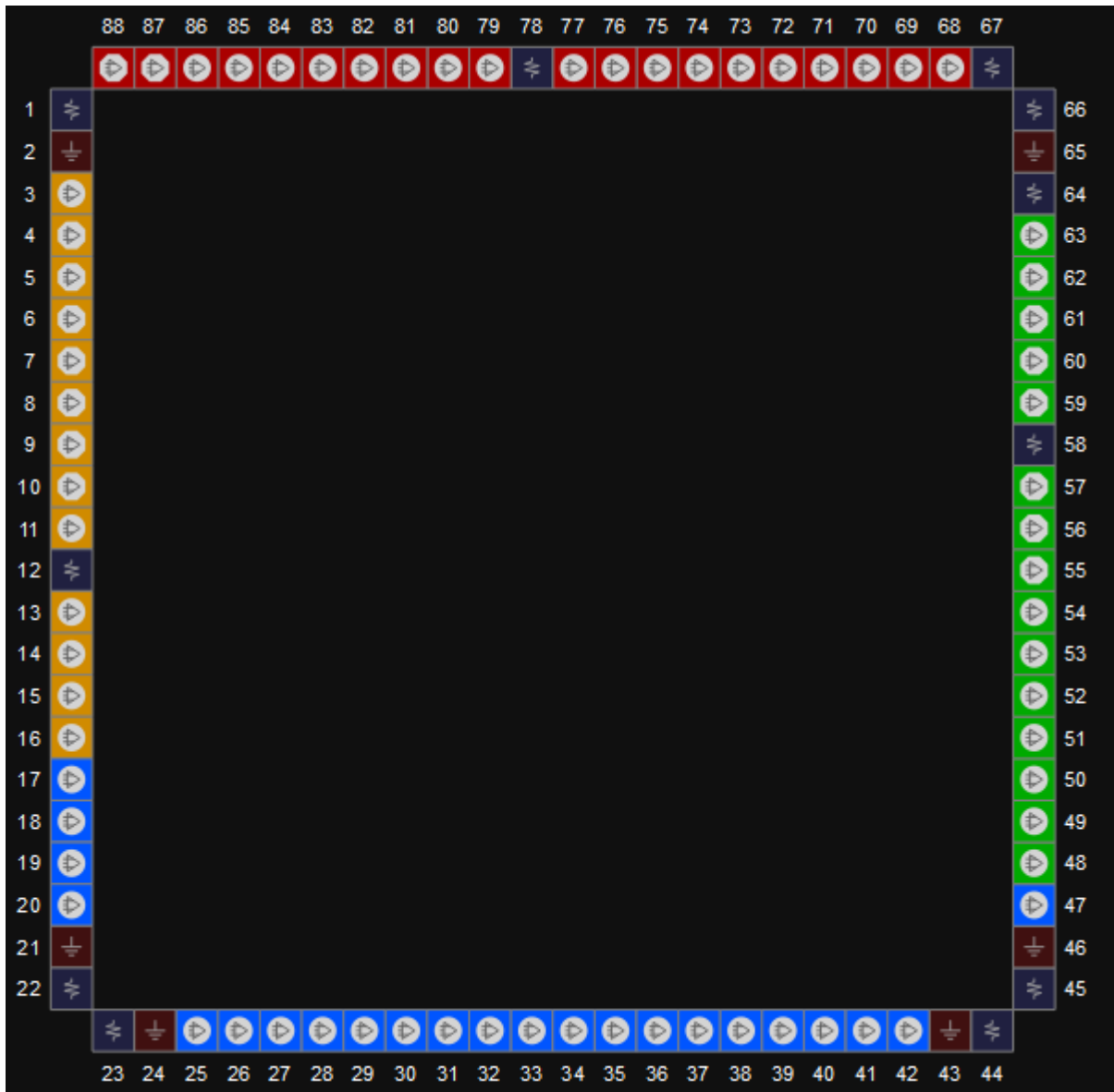
图 3-31 GW1N-4 器件 QN88 封装管脚分布示意图（顶视图）
