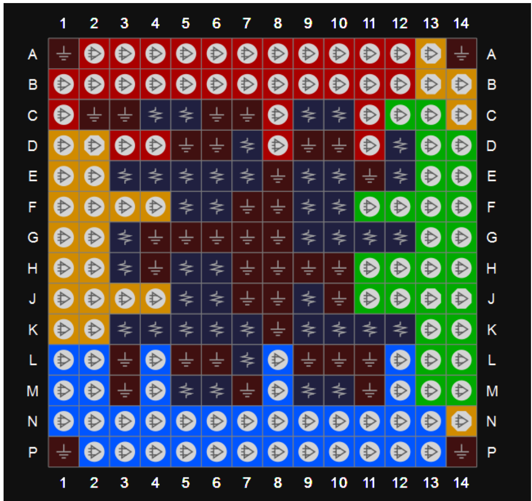
图 3-50 GW1N-9 器件 MG196 封装管脚分布示意图（顶视图）
