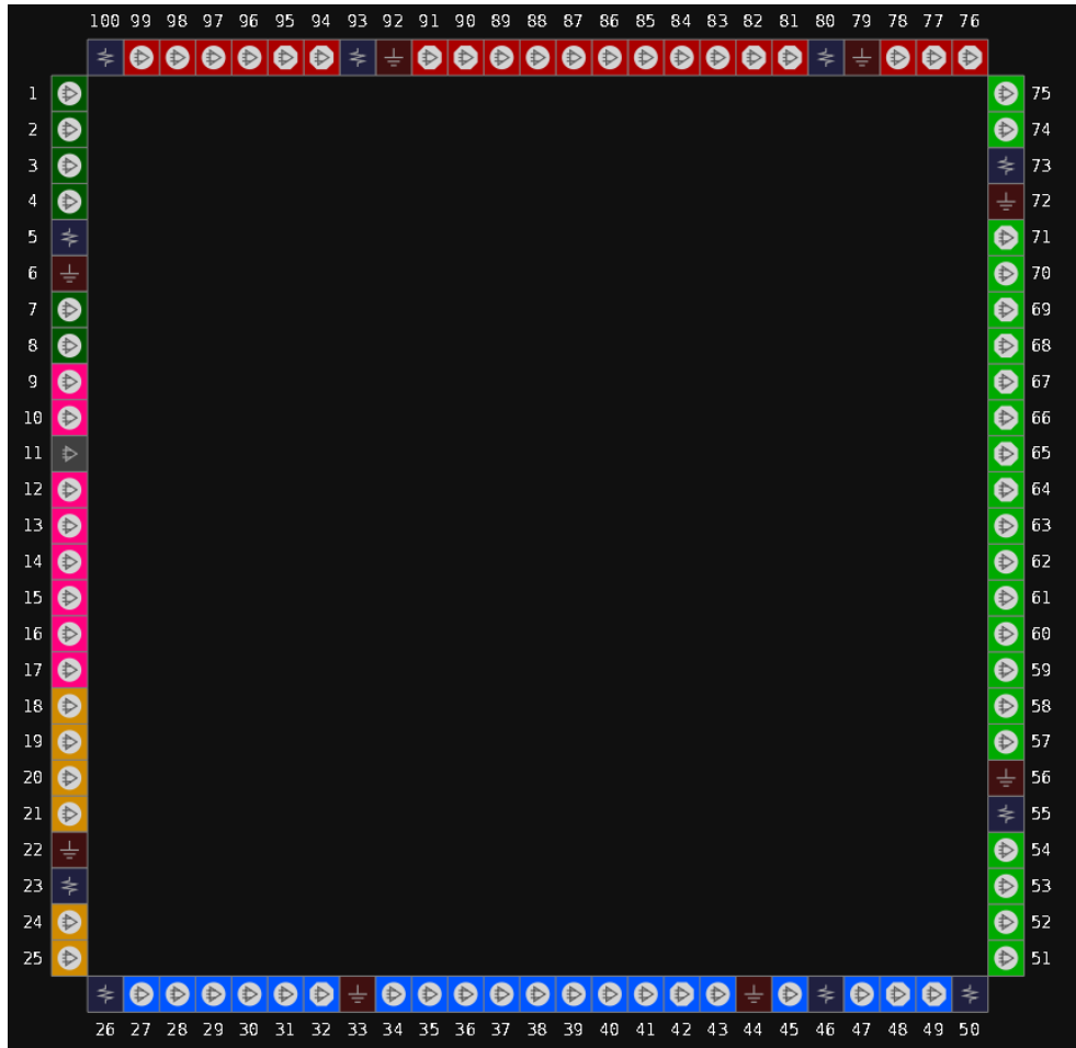
图 3-26 GW1N-1P5 器件 LQ100 封装 LV 版本管脚分布示意图（顶视图）
