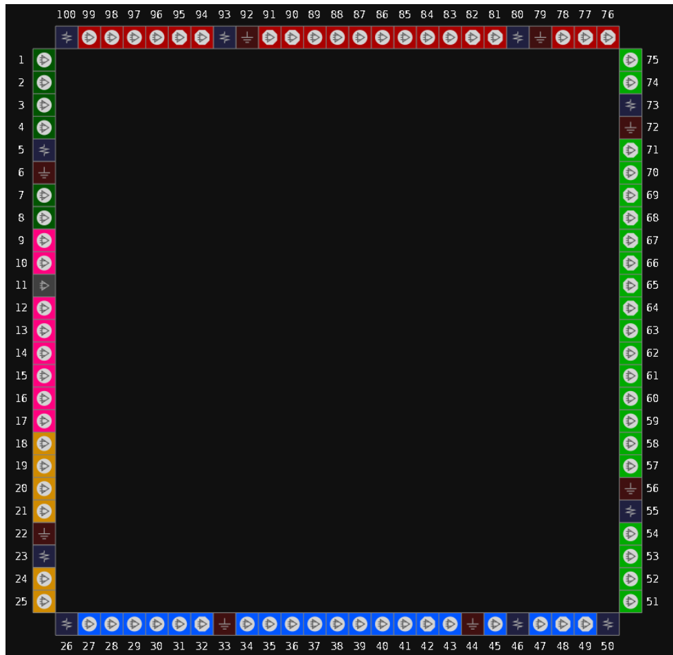
图 3-24 GW1N-1P5 器件 LQ100X 封装 LV 版本管脚分布示意图（顶视图）
