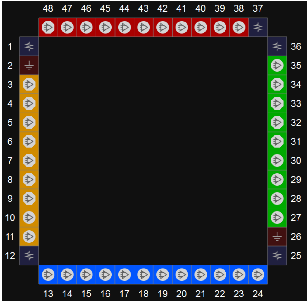
图 3-29 GW1N-4 器件 QN48 封装管脚分布示意图（顶视图）
