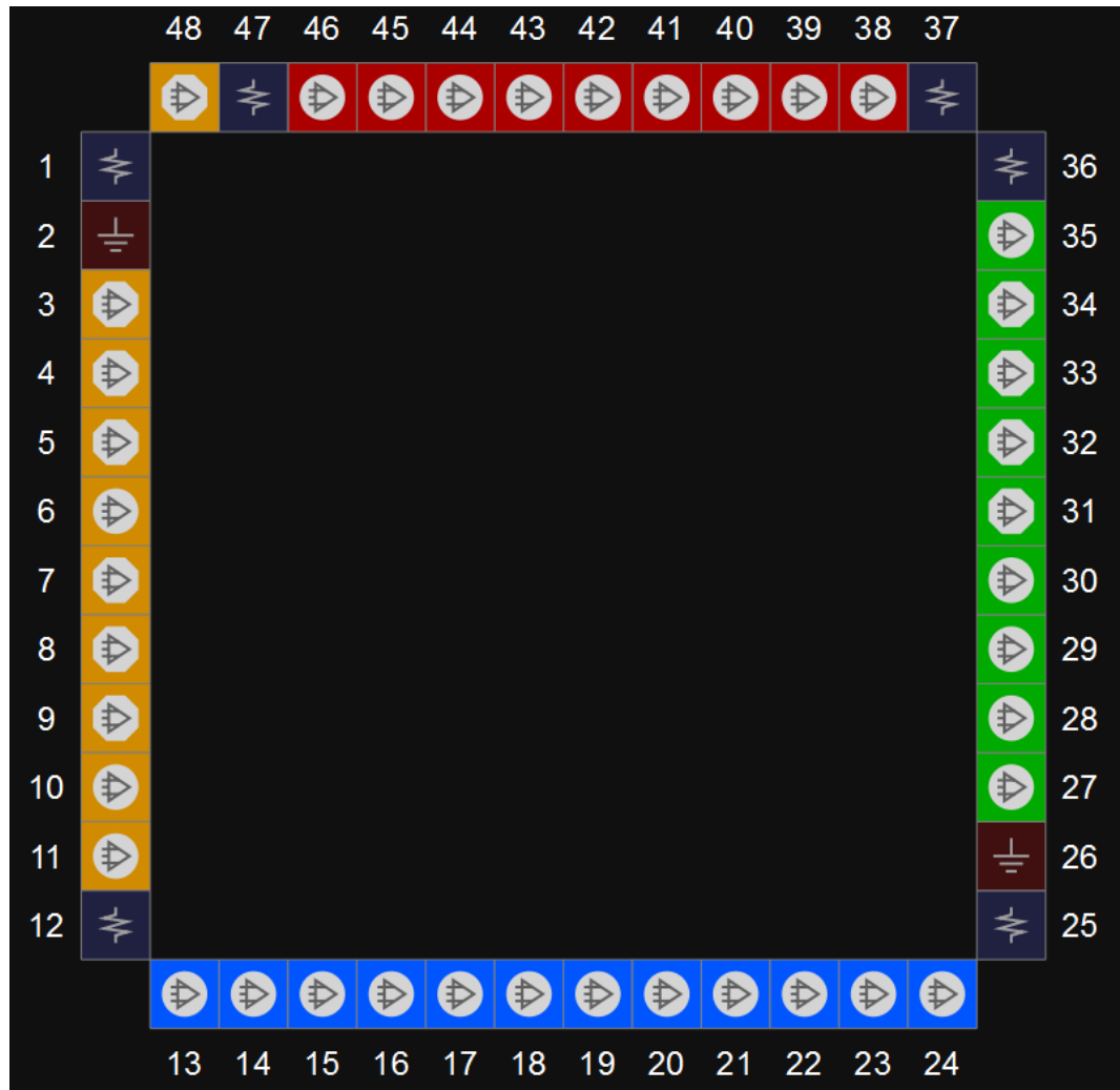
图 3-54 GW1N-9 器件 QN48F 管脚分布示意图（顶视图）
