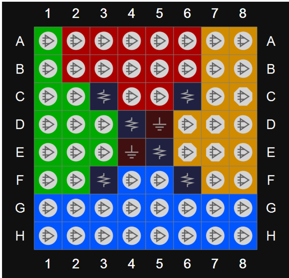
图 3-39 GW1N-9 器件 CM64 封装管脚分布示意图（顶视图）
