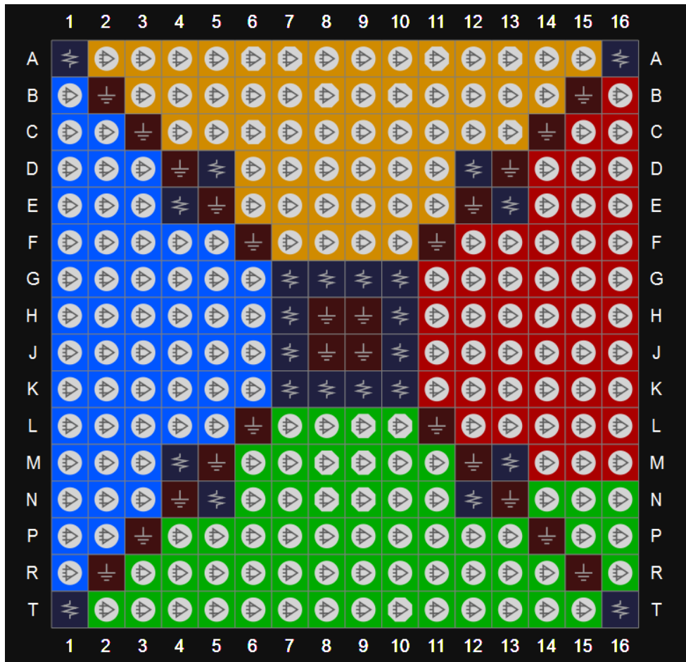
图 3-52 GW1N-9 器件 UG256 封装管脚分布示意图（顶视图）
