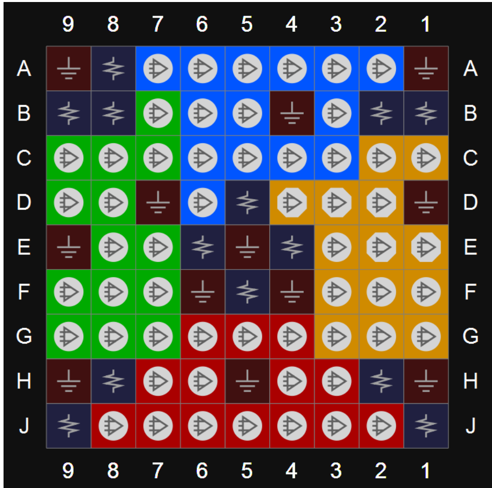
图 3-40 GW1N-9 器件 CS81M 封装管脚分布示意图（顶视图）
