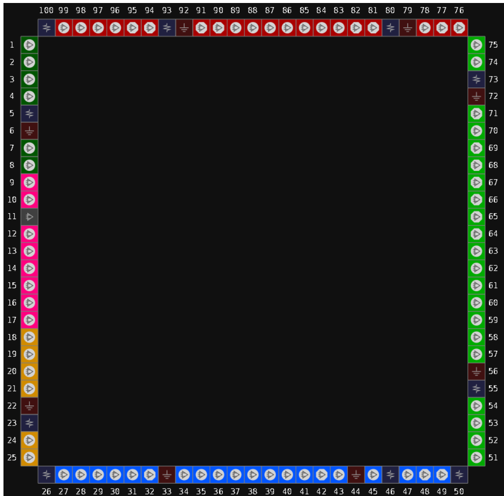
图 3-27 GW1N-1P5 器件 LQ100 封装 UV 版本管脚分布示意图（顶视图）
