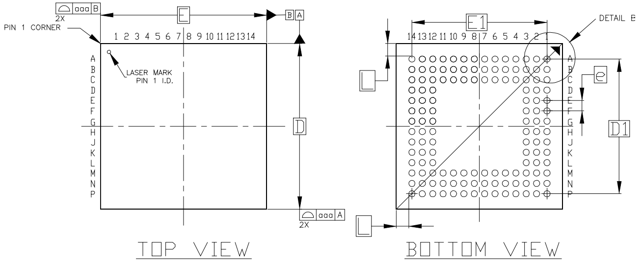
图 4-17 封装尺寸 MG132/MG132X / MG132H
