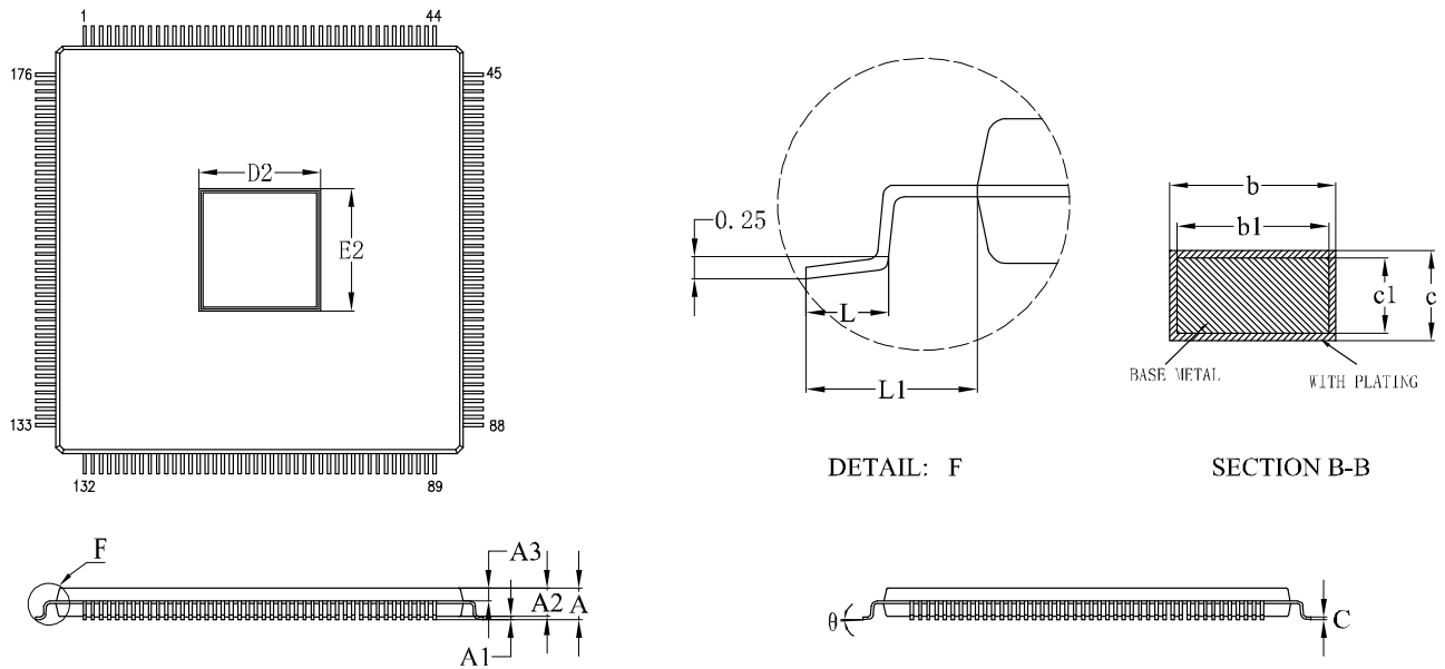
图 4-15 封装尺寸 EQ176
