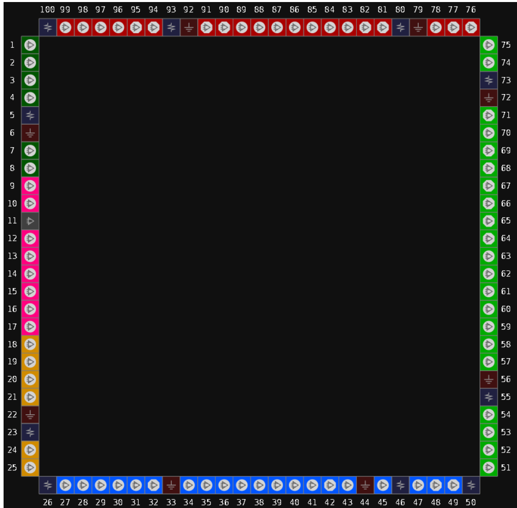
图 3-25 GW1N-1P5 器件 LQ100X 封装 UV 版本管脚分布示意图（顶视图）
