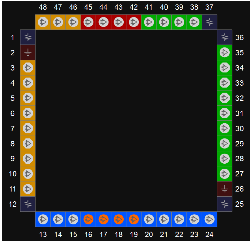
图 3-38 GW1N-9 器件 QN48 封装管脚分布示意图（顶视图）
