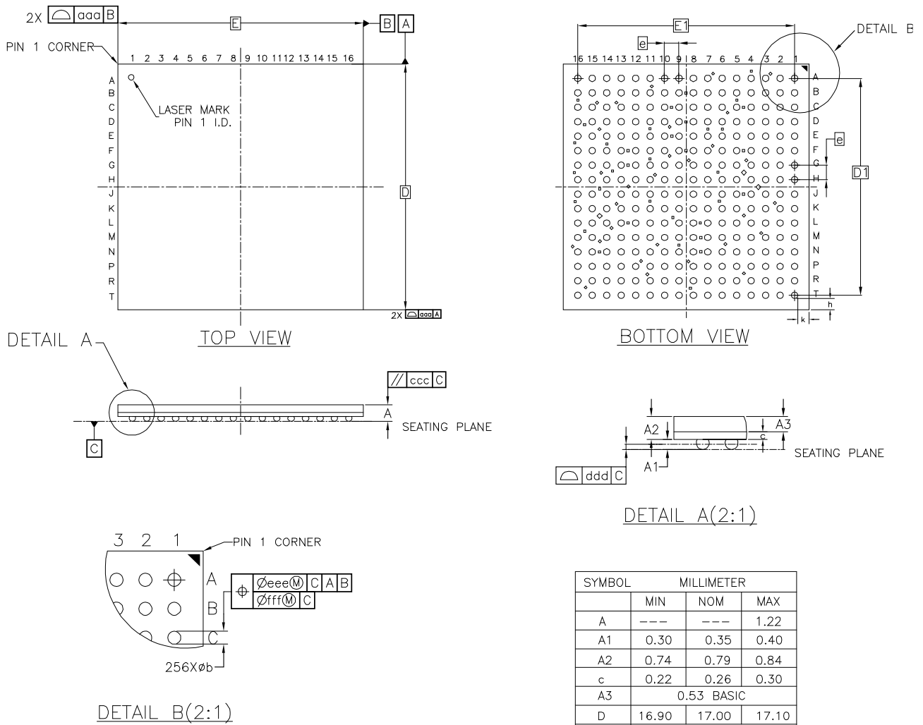
图 4-26 封装尺寸 PG256
