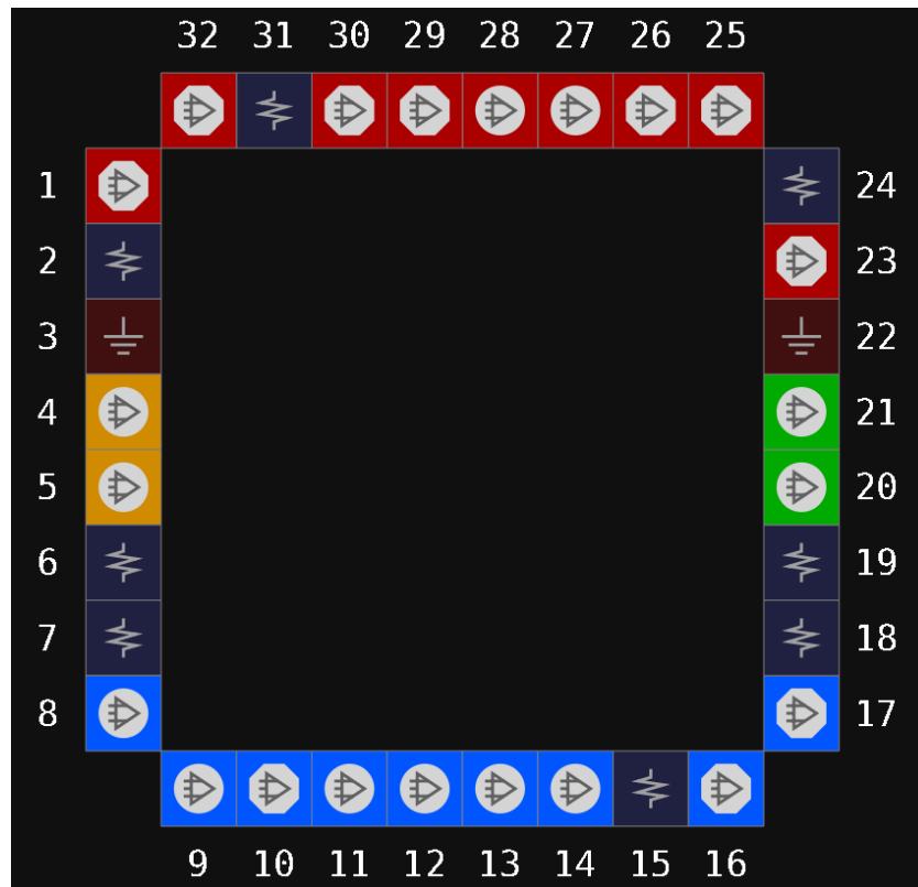
图 3-31 GW1N-2 器件 QN32X UV 版本封装管脚分布示意图（顶视图）
