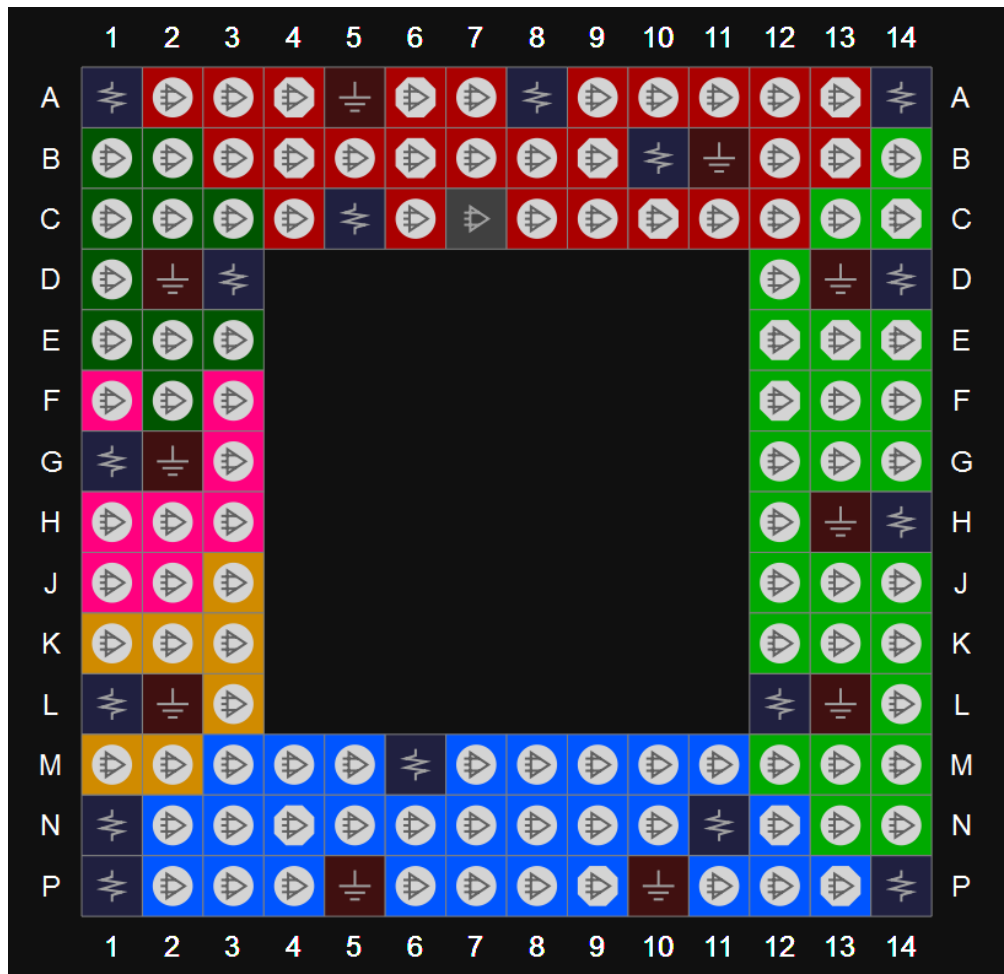
图 3-11 GW1N-2 器件 MG132X 封装管脚分布示意图 (LV 版本,顶视图)
