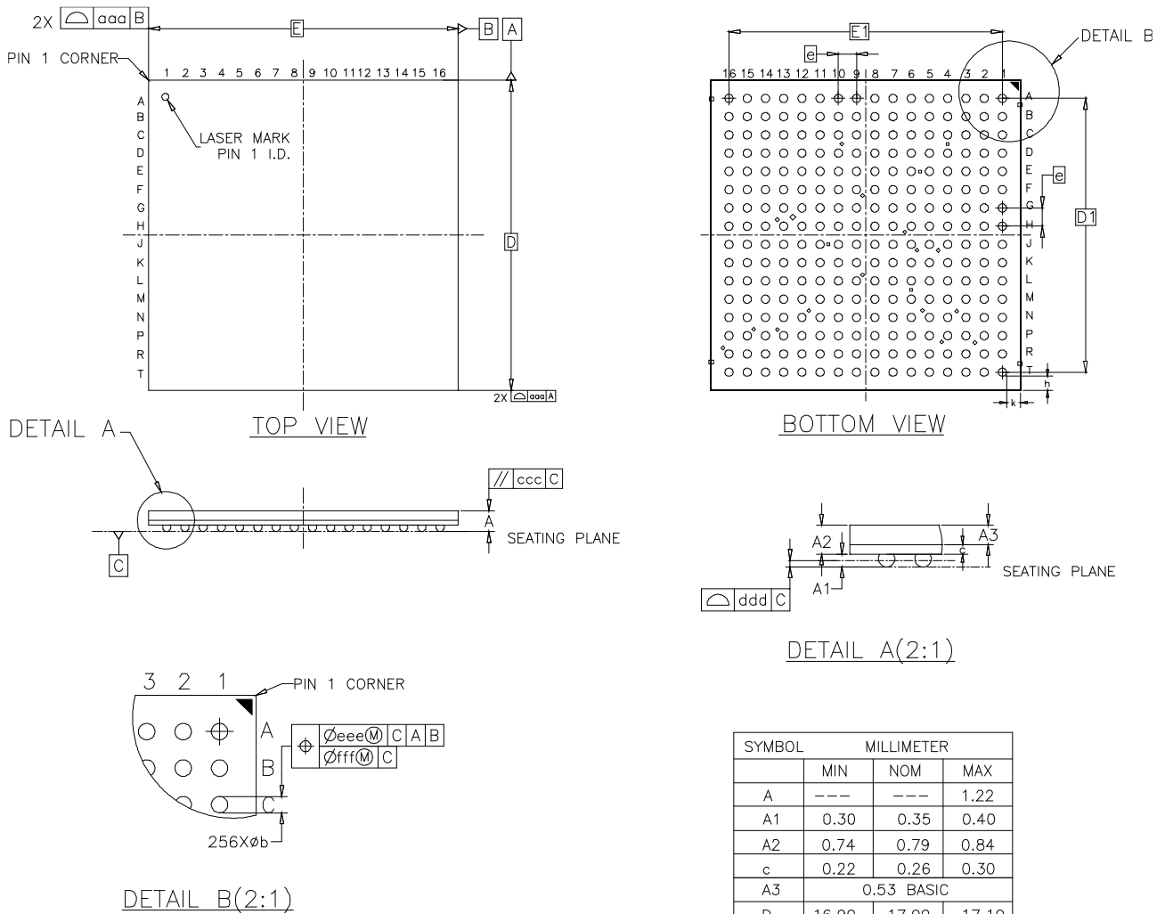
图 4-25 封装尺寸 PG256M
