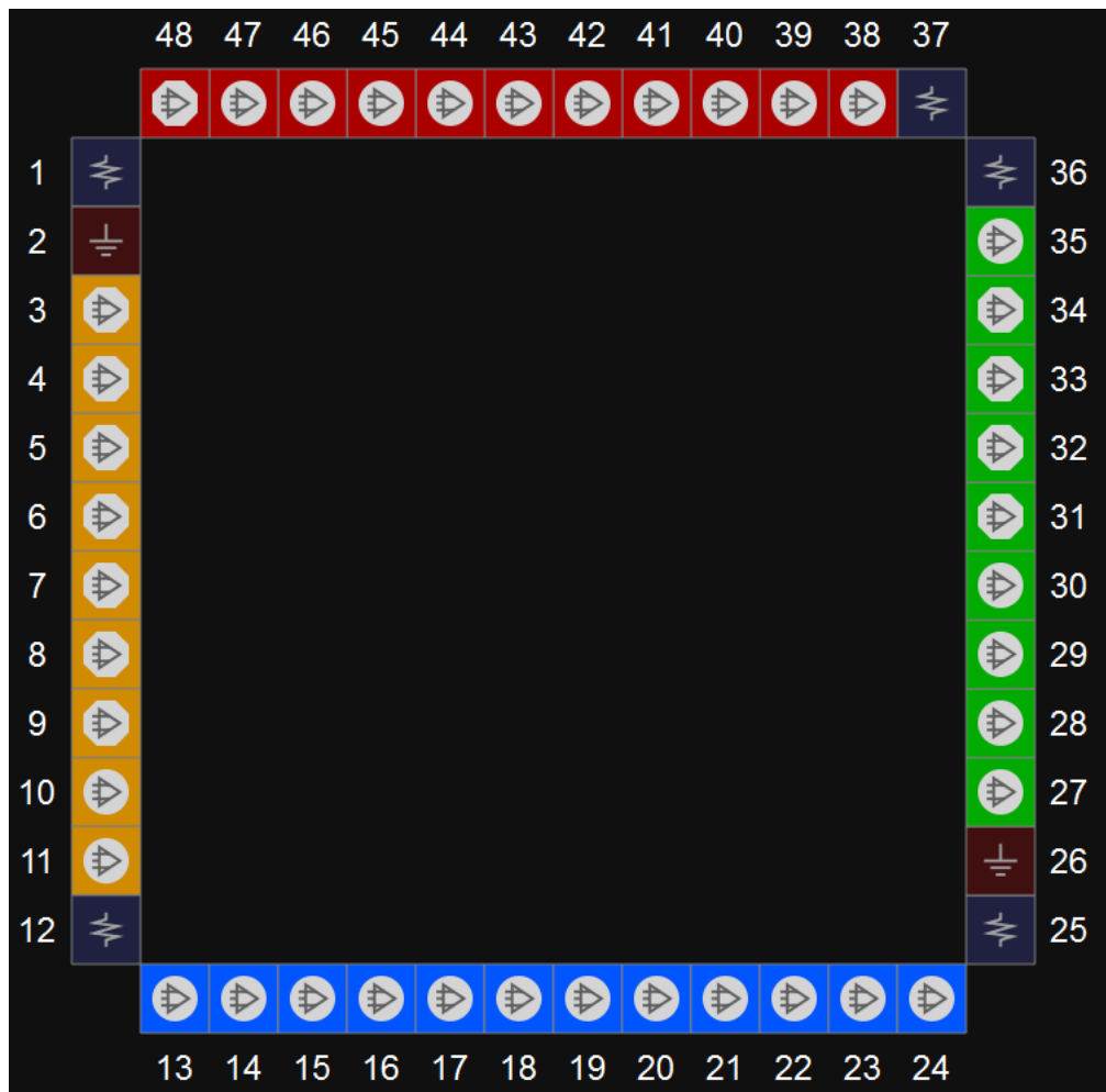
图 3-40 GW1N-4 器件 QN48 封装管脚分布示意图（顶视图）
