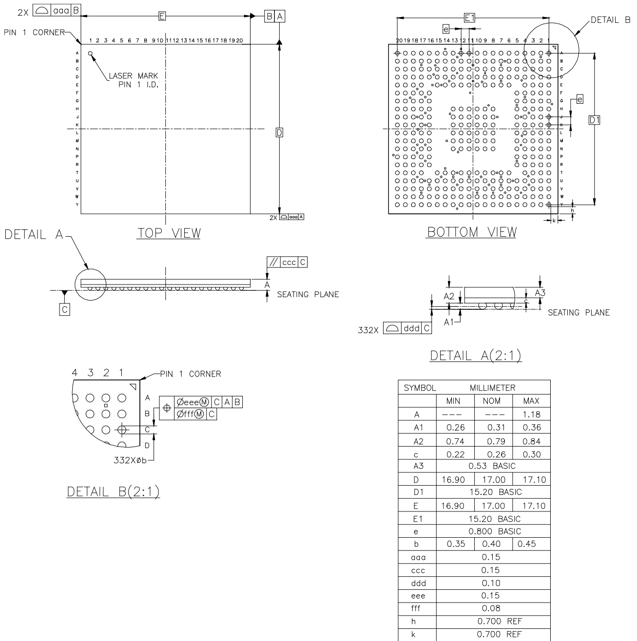
图 4-29 封装尺寸 UG332
