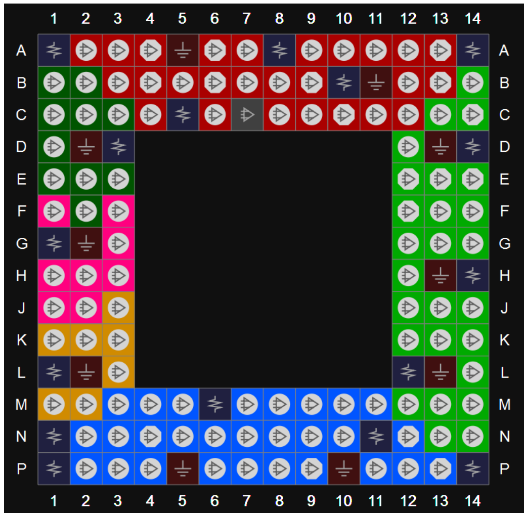
图 3-10 GW1N-2 器件 MG132X 封装管脚分布示意图 (UV 版本,顶视图)
