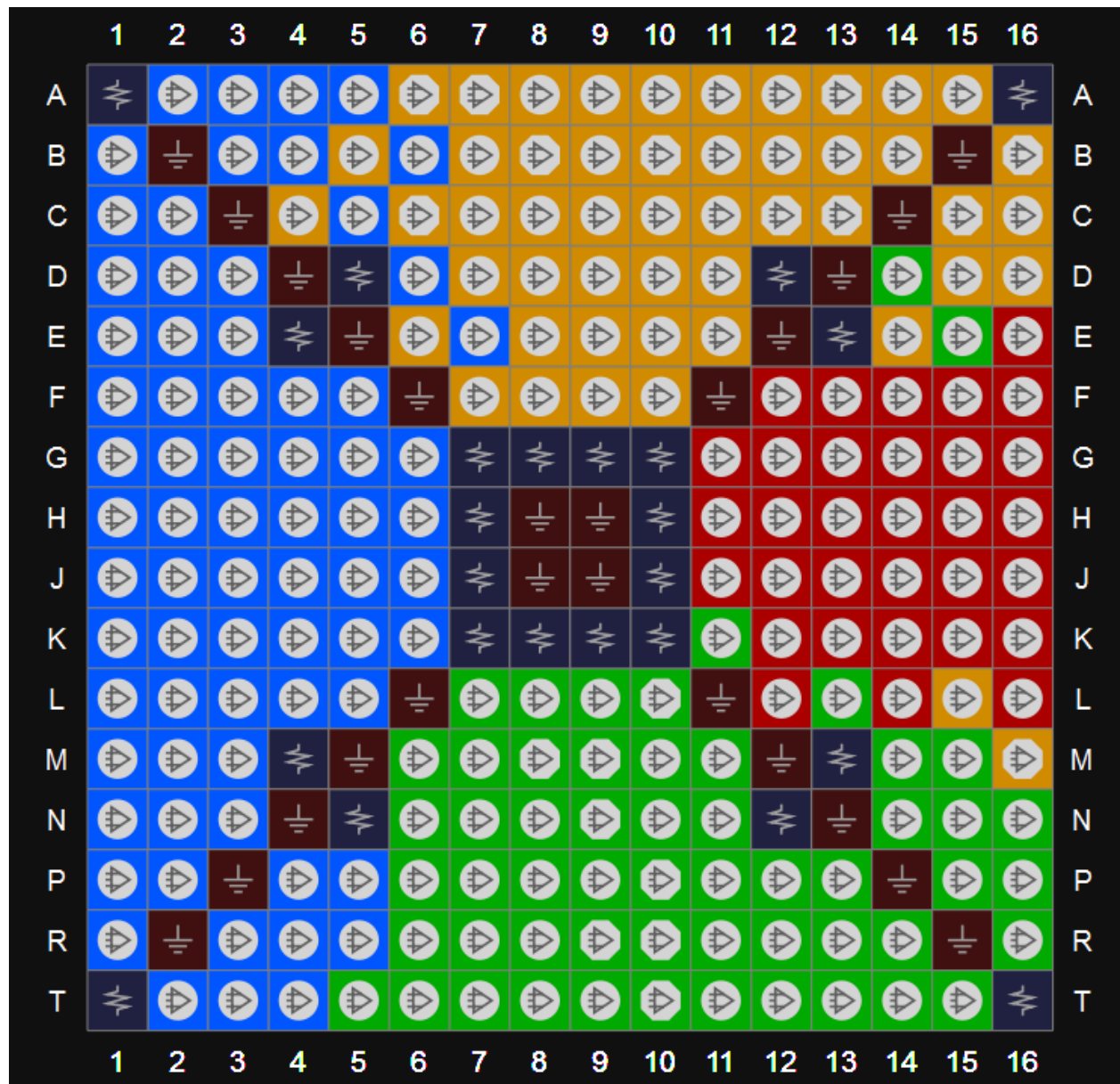
图 3-63 GW1N-9 器件 PG256 封装管脚分布示意图（顶视图）
