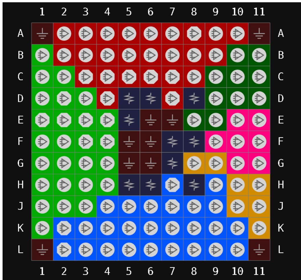
图 3-25 GW1N-2 器件 MG121 封装管脚分布示意图 (LV 版本 顶视图)
