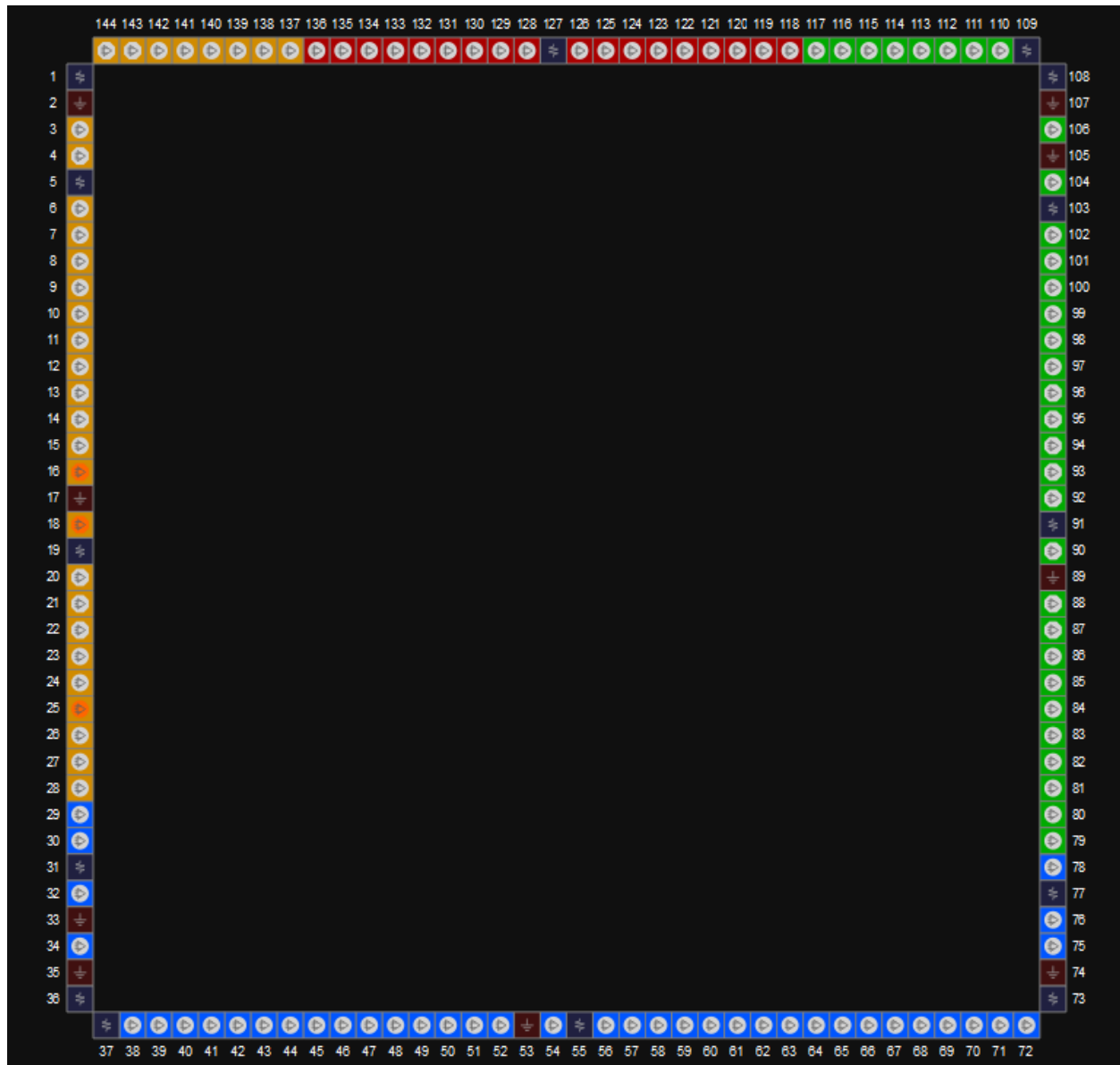
图 3-56 GW1N-9 器件 LQ144 封装管脚分布示意图（顶视图）
