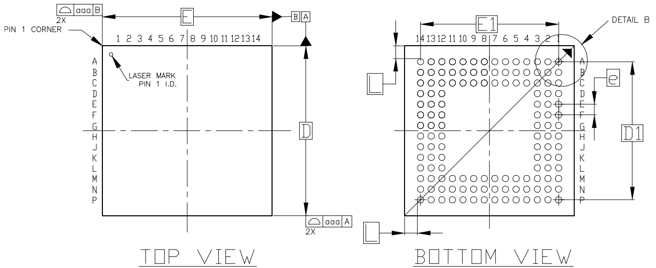
图 4-22 封装尺寸 MG132/MG132X / MG132H
