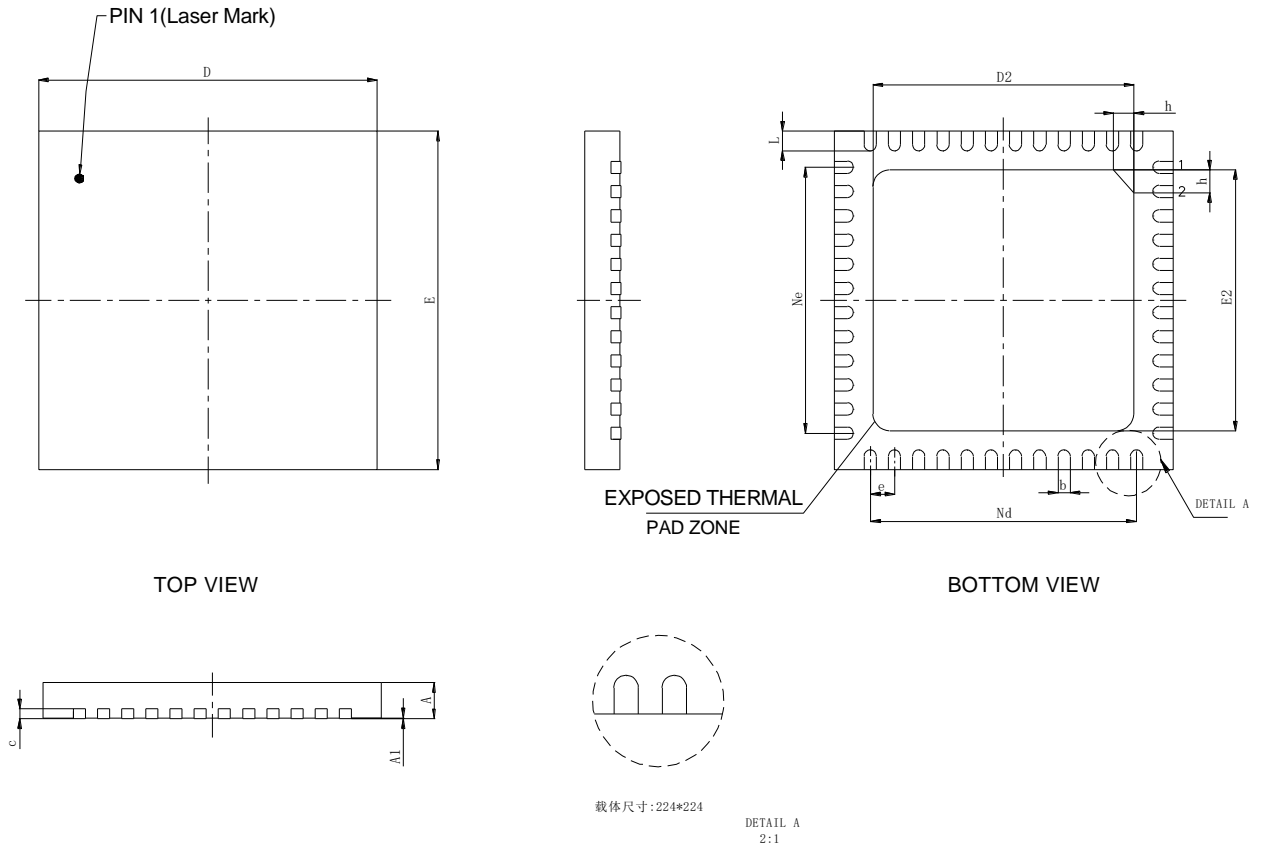
图 4-10 封装尺寸 QN48X
