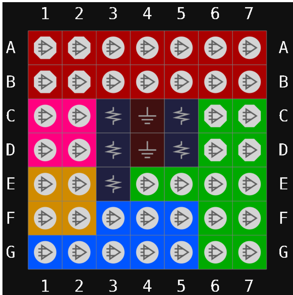
图 3-29 GW1N-2 器件 MG49 封装管脚分布示意图（顶视图）
