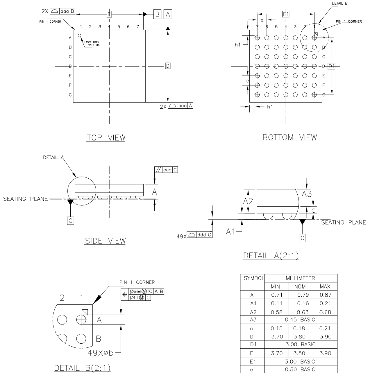
图 4-19 封装尺寸 MG49
