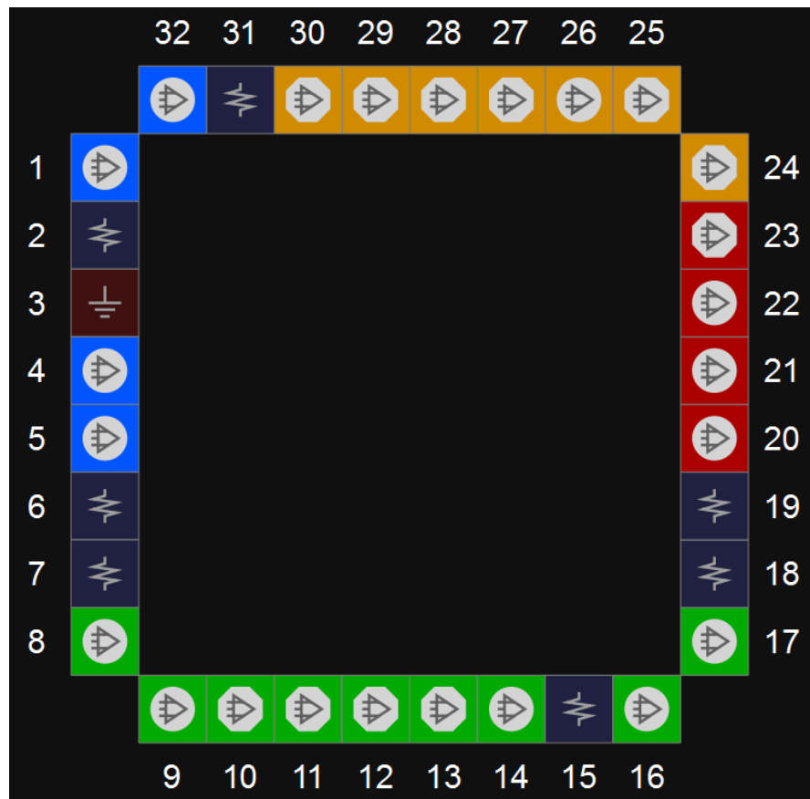
图 3-39 GW1N-4 器件 QN32 封装管脚分布示意图（顶视图）
