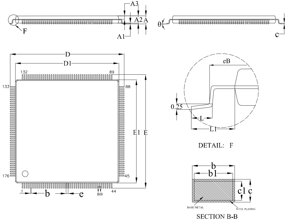
图 4-17 封装尺寸 LQ176
