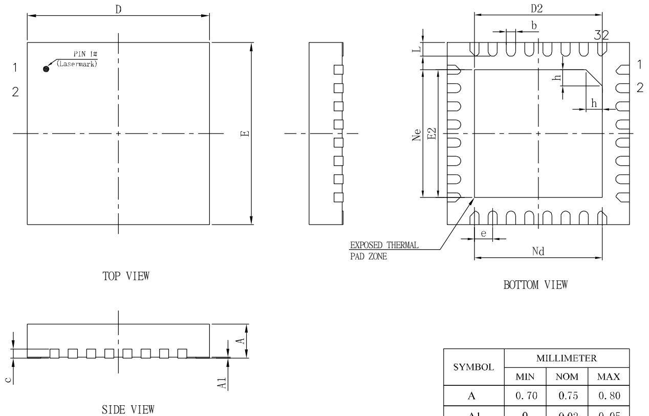
图 4-6 封装尺寸 FN32(GW1N-1S)
