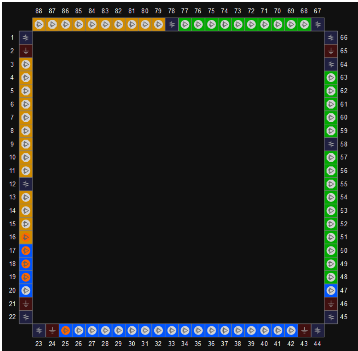
图 3-53 GW1N-9 器件 QN88 封装管脚分布示意图（顶视图）
