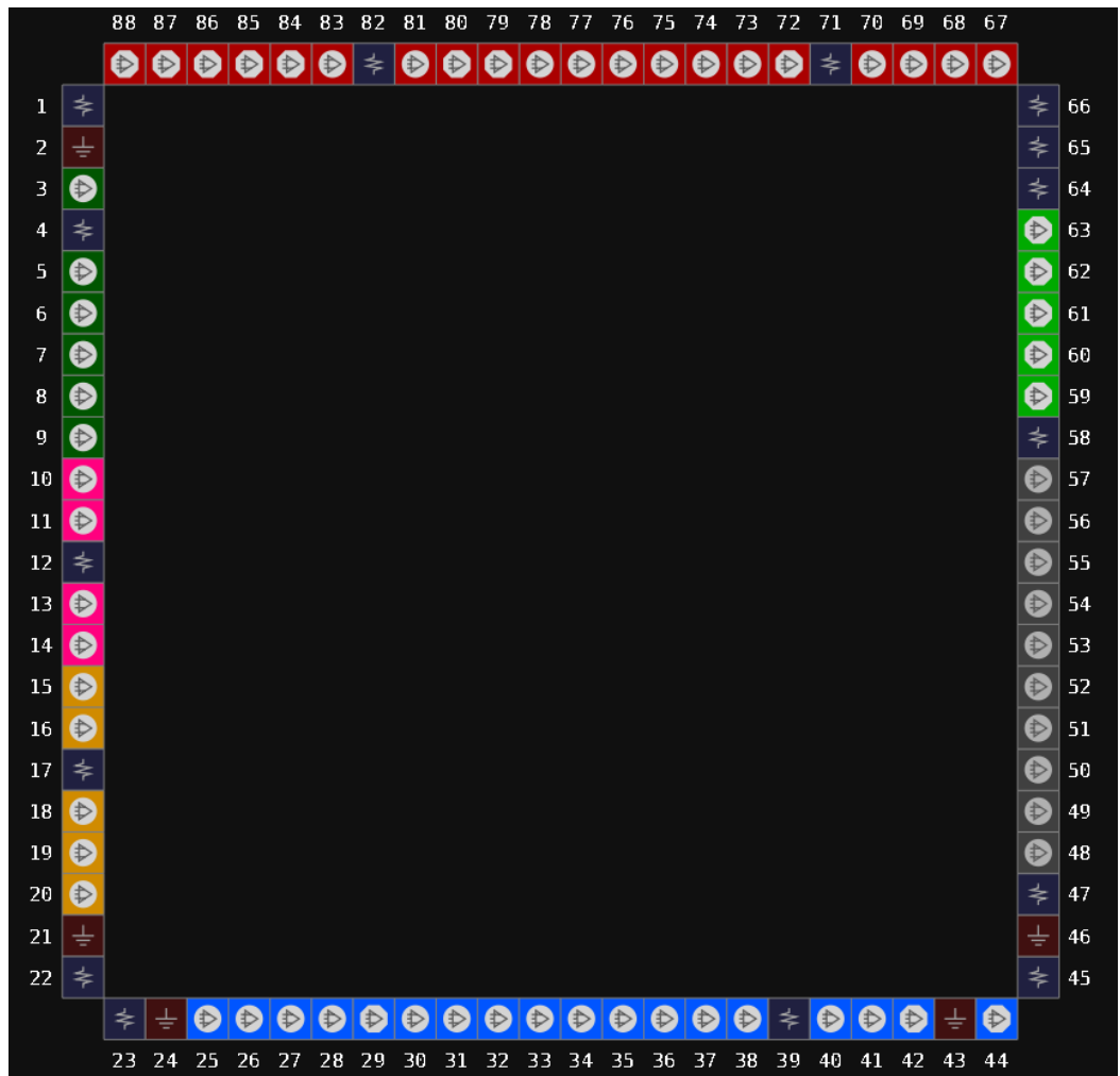
图 3-32 GW1N-2 器件 QN88 封装管脚分布示意图（顶视图）
