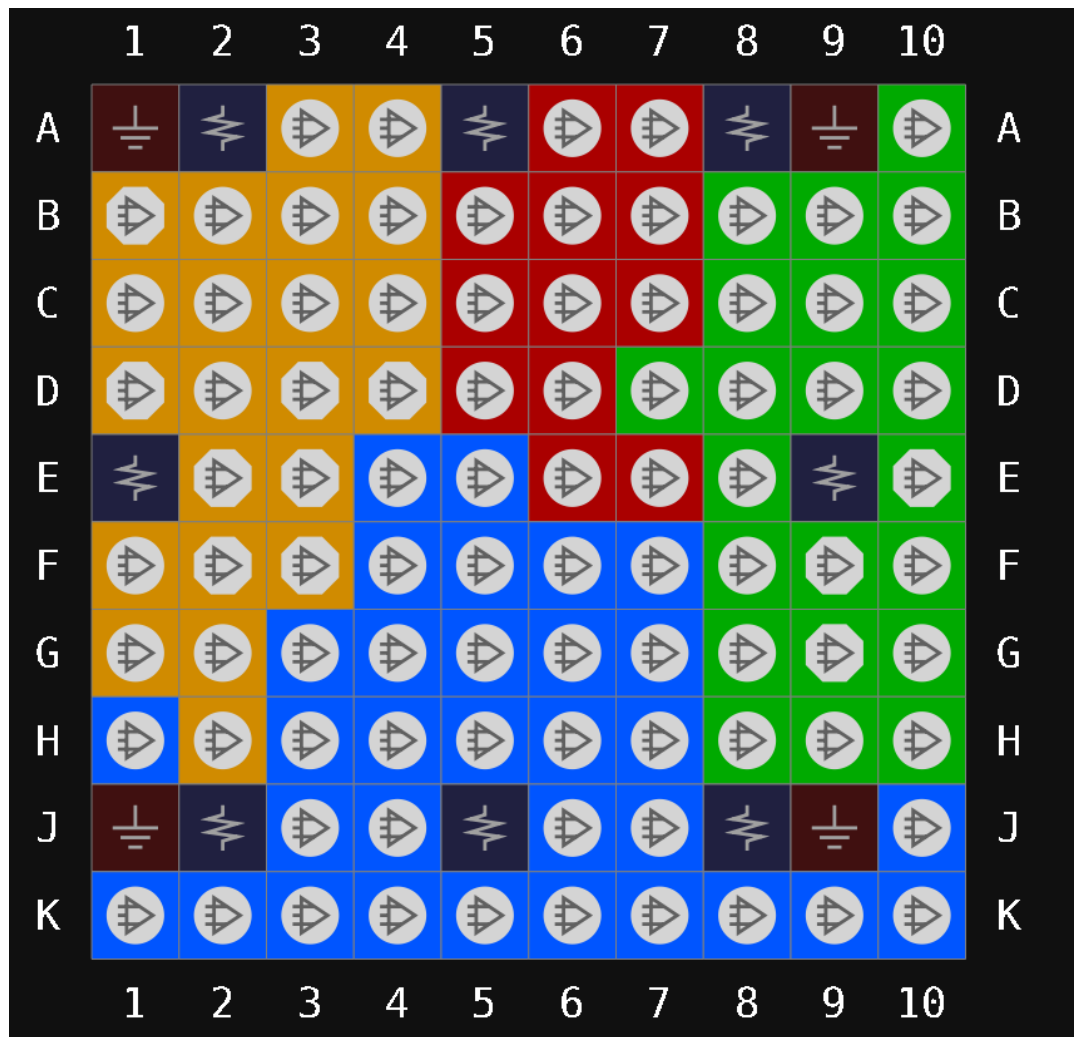
图 3-67 GW1N-9 器件 MG100T 管脚分布示意图（顶视图）
