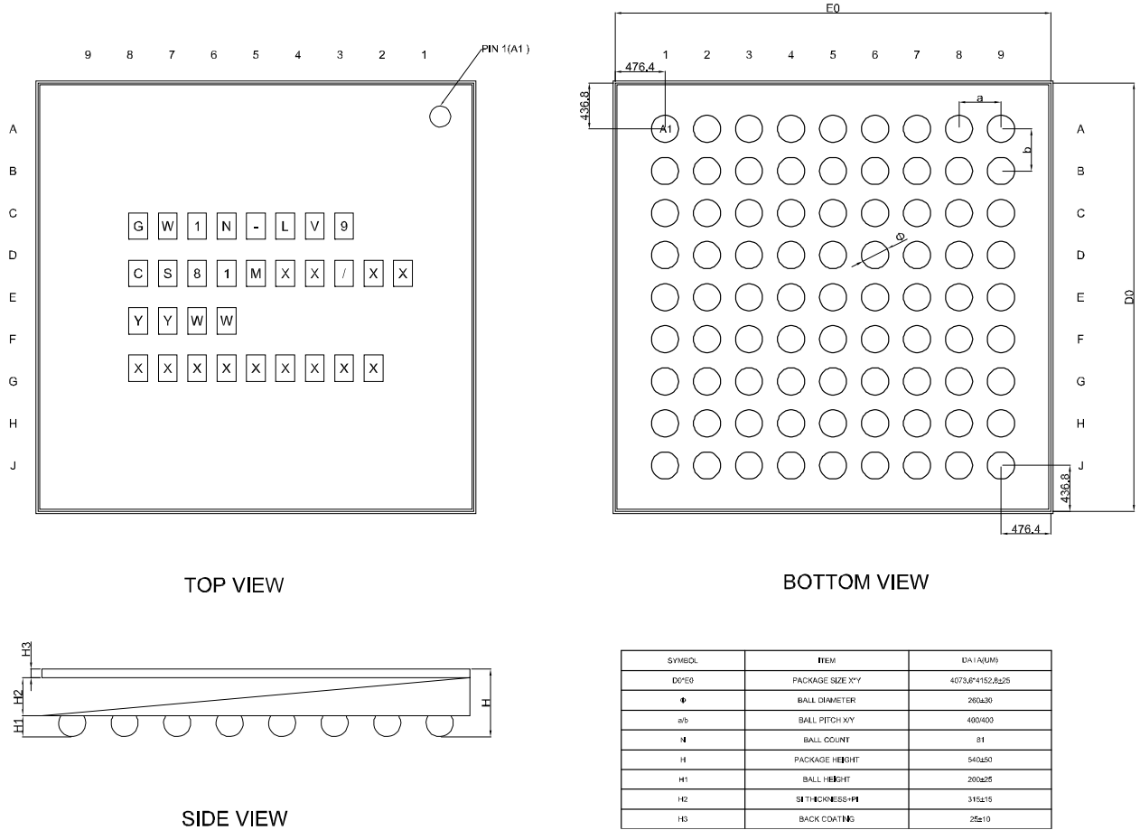
图 4-12 封装尺寸 CS81M
