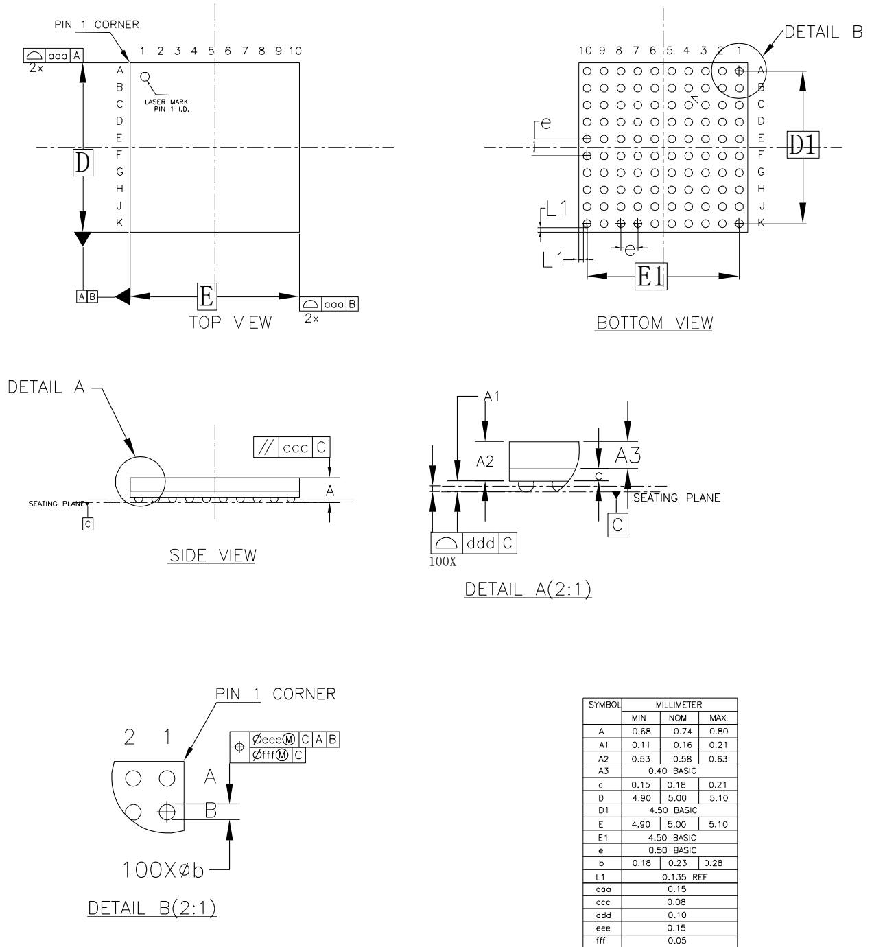
图 4-20 封装尺寸 MG100/ MG100T
