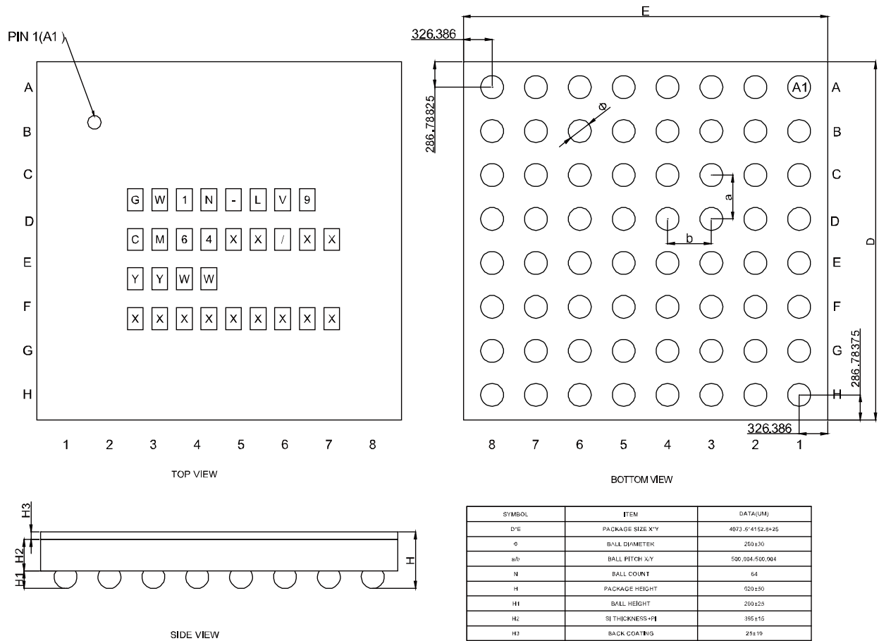
图 4-11 封装尺寸 CM64
