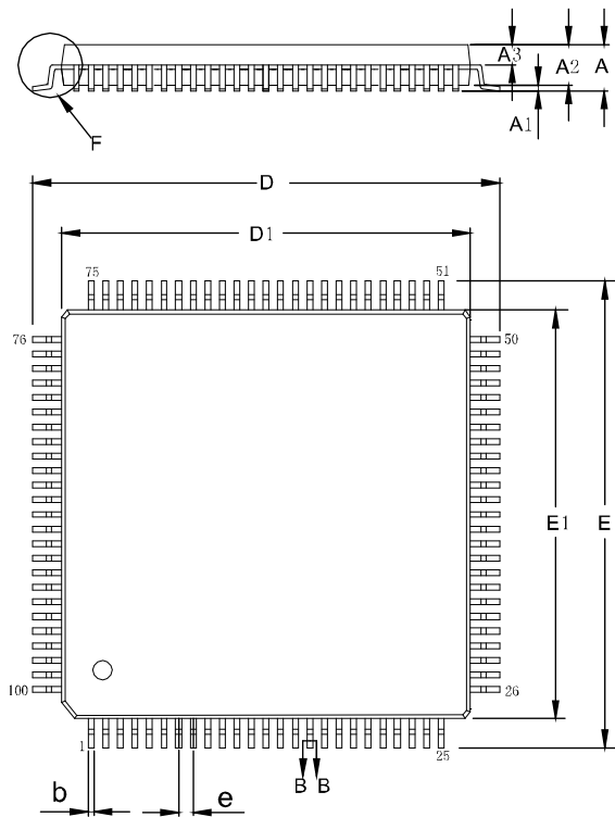
图 4-14 封装尺寸 LQ100/LQ100X
