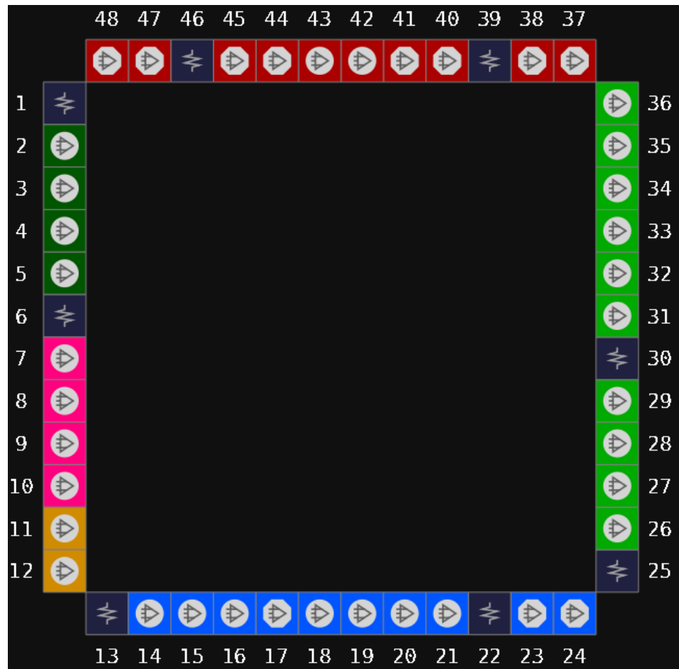
图 3-38 GW1N-1P5 器件 QN48X 封装管脚分布示意图 (UV 版本, 顶视图)
