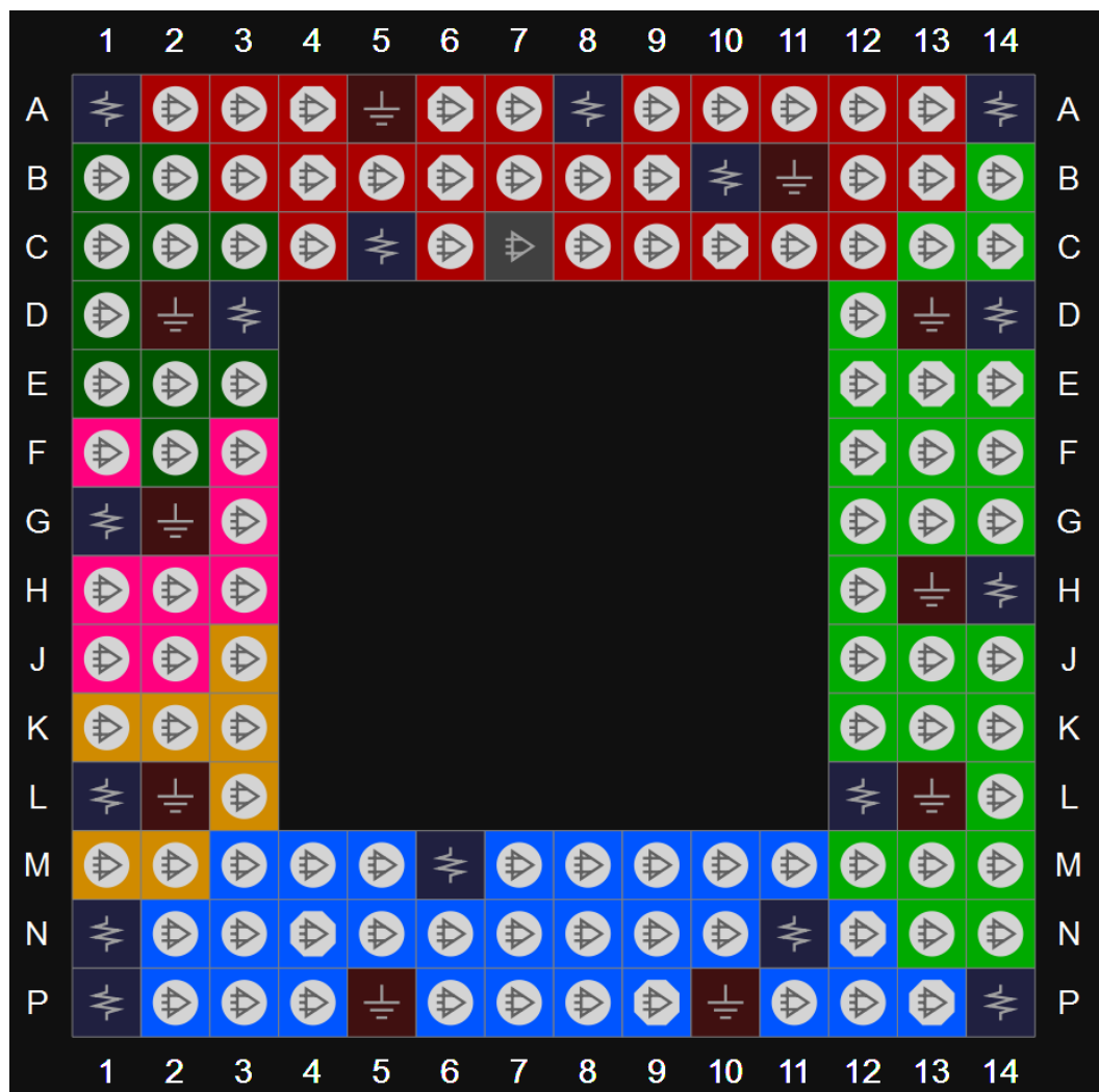
图 3-23 GW1N-2 器件 MG132 封装管脚分布示意图 (UV 版本 顶视图)
