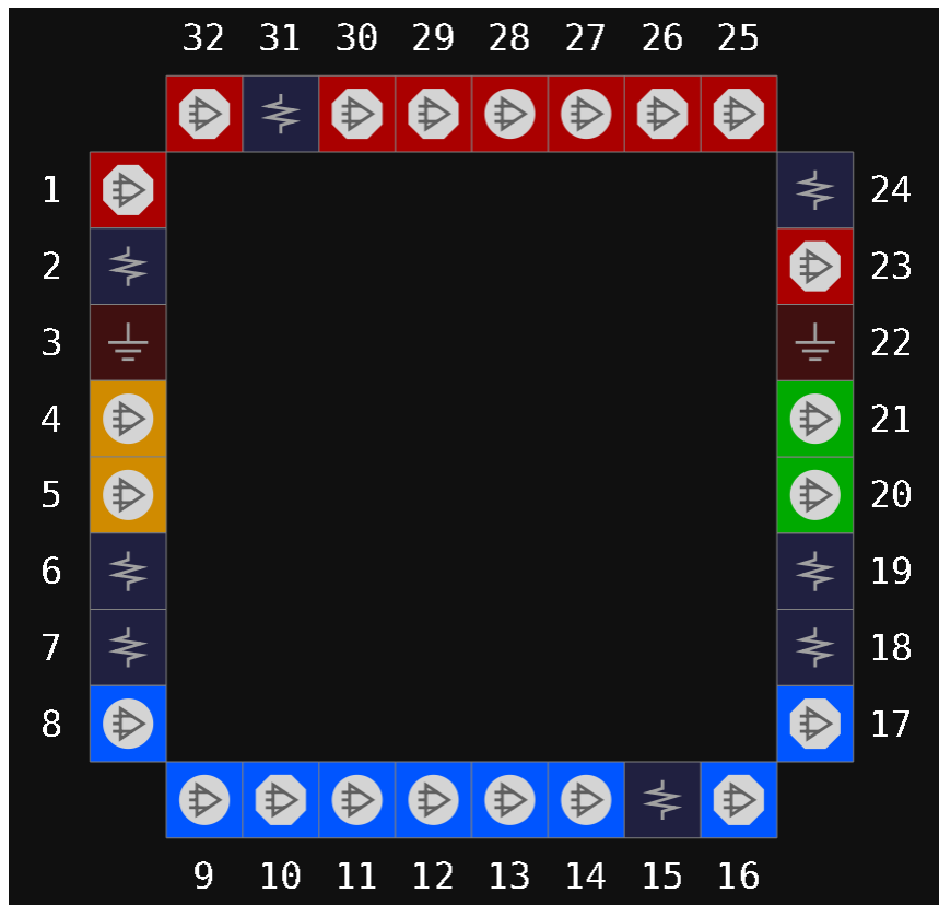
图 3-30 GW1N-2 器件 QN32X LV 版本封装管脚分布示意图（顶视图）
