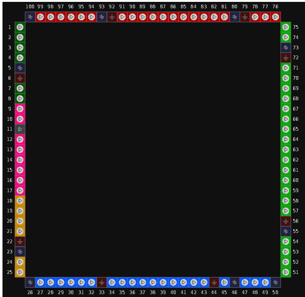
图 3-33 GW1N-1P5 器件 LQ100X 封装管脚分布示意图 (LV 版本, 顶视图)
