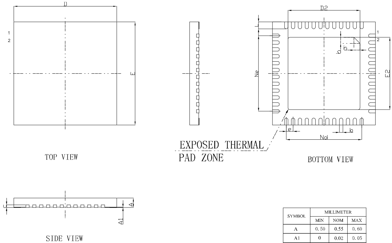
图 4-9 封装尺寸 QN48/QN48F/QN48H
