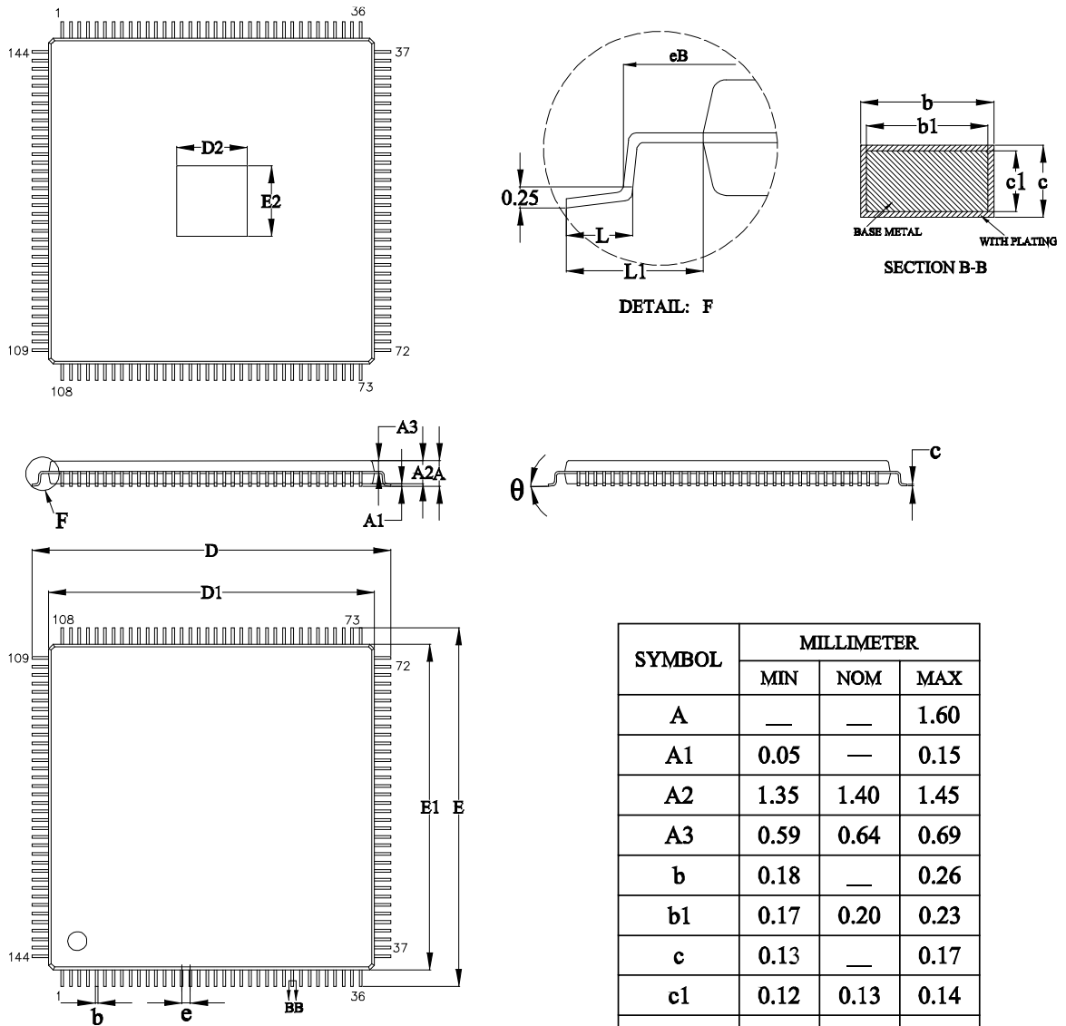
图 4-16 封装尺寸 EQ144
