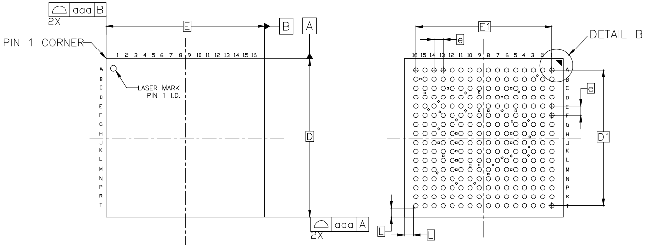
图 4-28 封装尺寸 UG256
