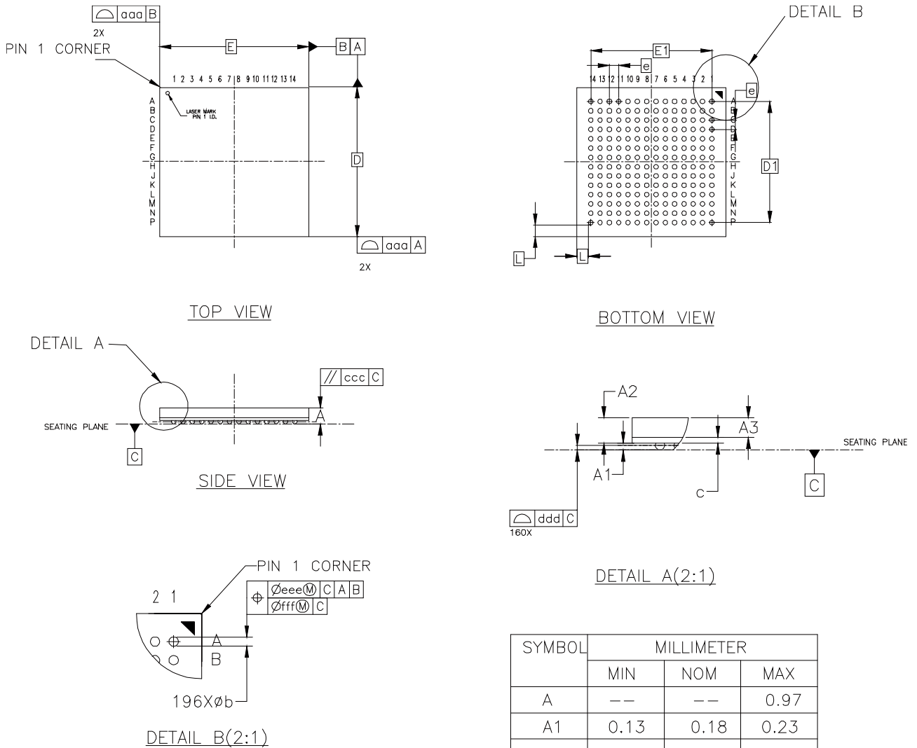
图 4-24 封装尺寸 MG196
