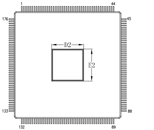
图 4-18 封装尺寸 EQ176
