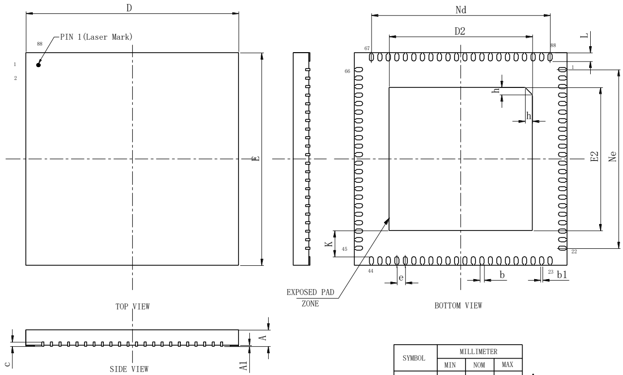
图 4-13 封装尺寸 QN88
