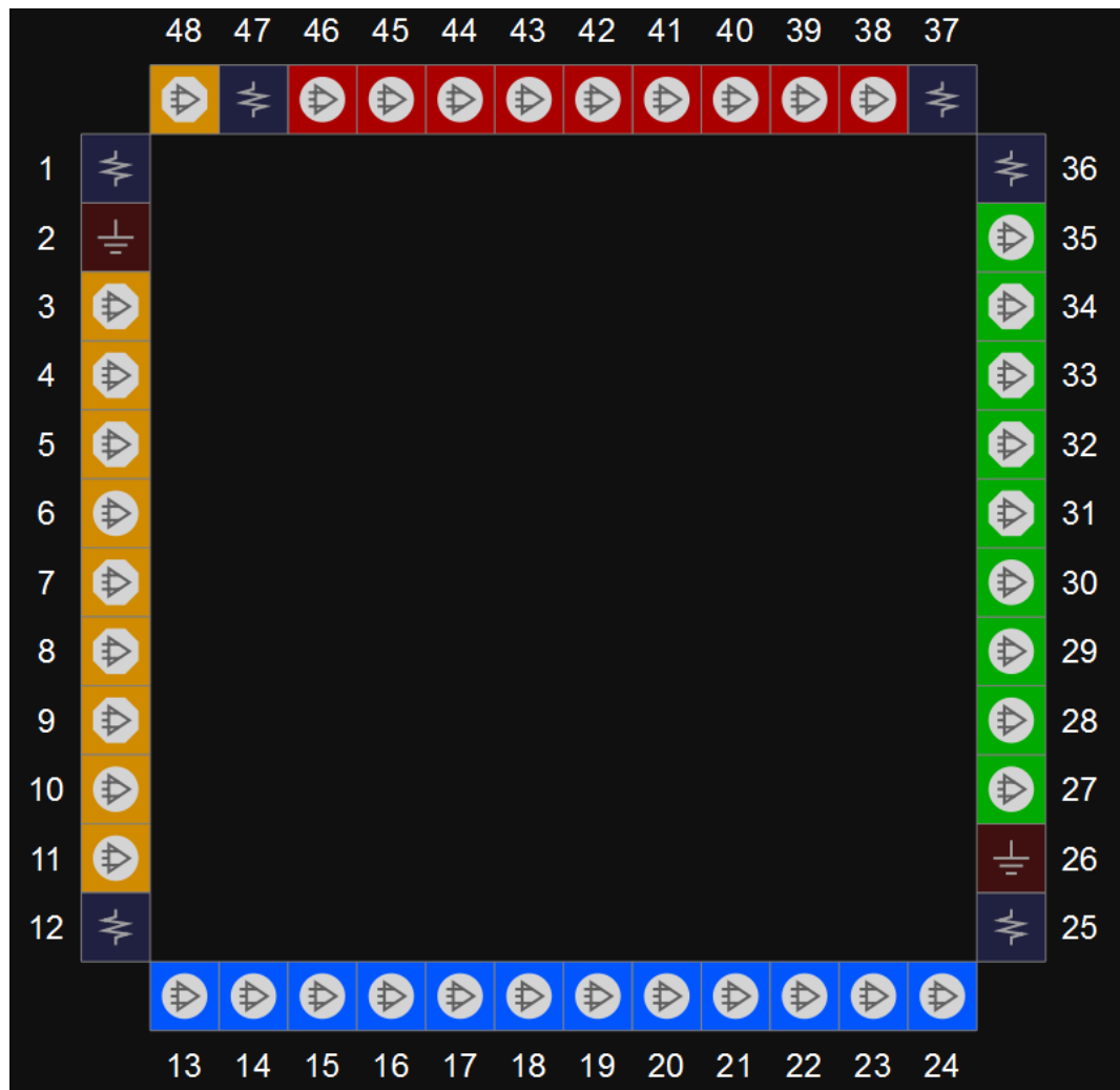
图 3-66 GW1N-9 器件 QN48F 管脚分布示意图（顶视图）
