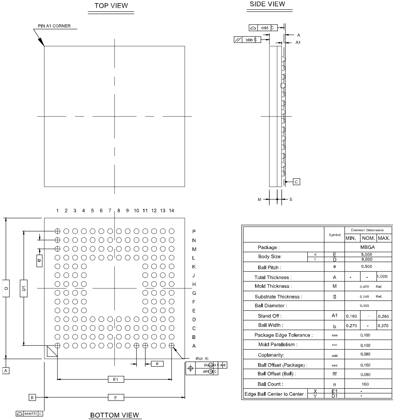
图 4-23 封装尺寸 MG160
