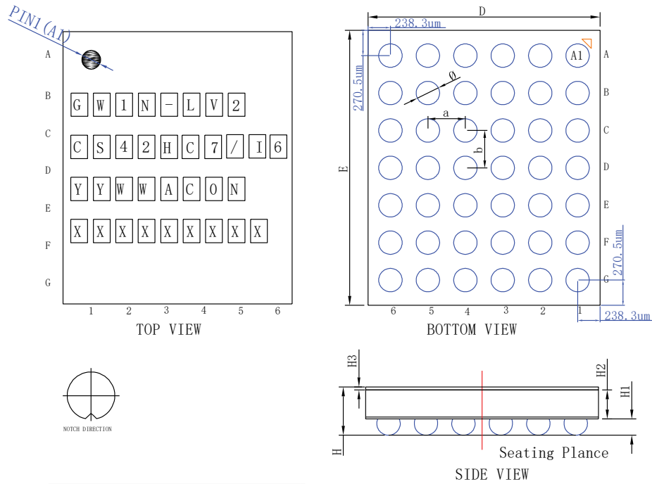
图 4-4 封装尺寸 CS42H
