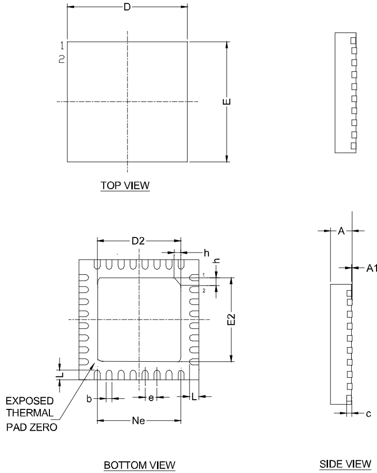
图 4-7 封装尺寸 QN32(GW1N-1/4)
