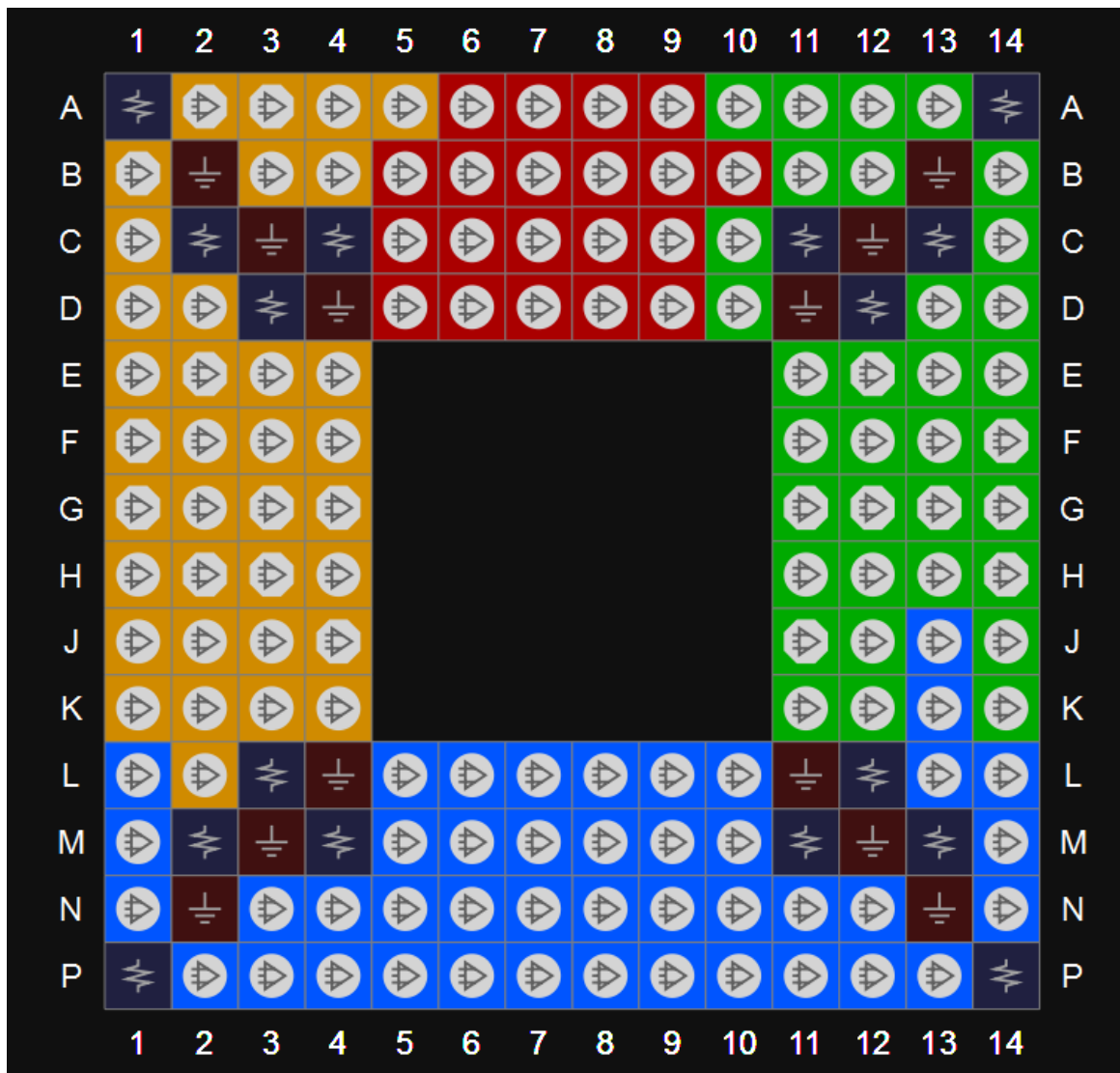
图 3-58 GW1N-9 器件 MG160 封装管脚分布示意图（顶视图）
