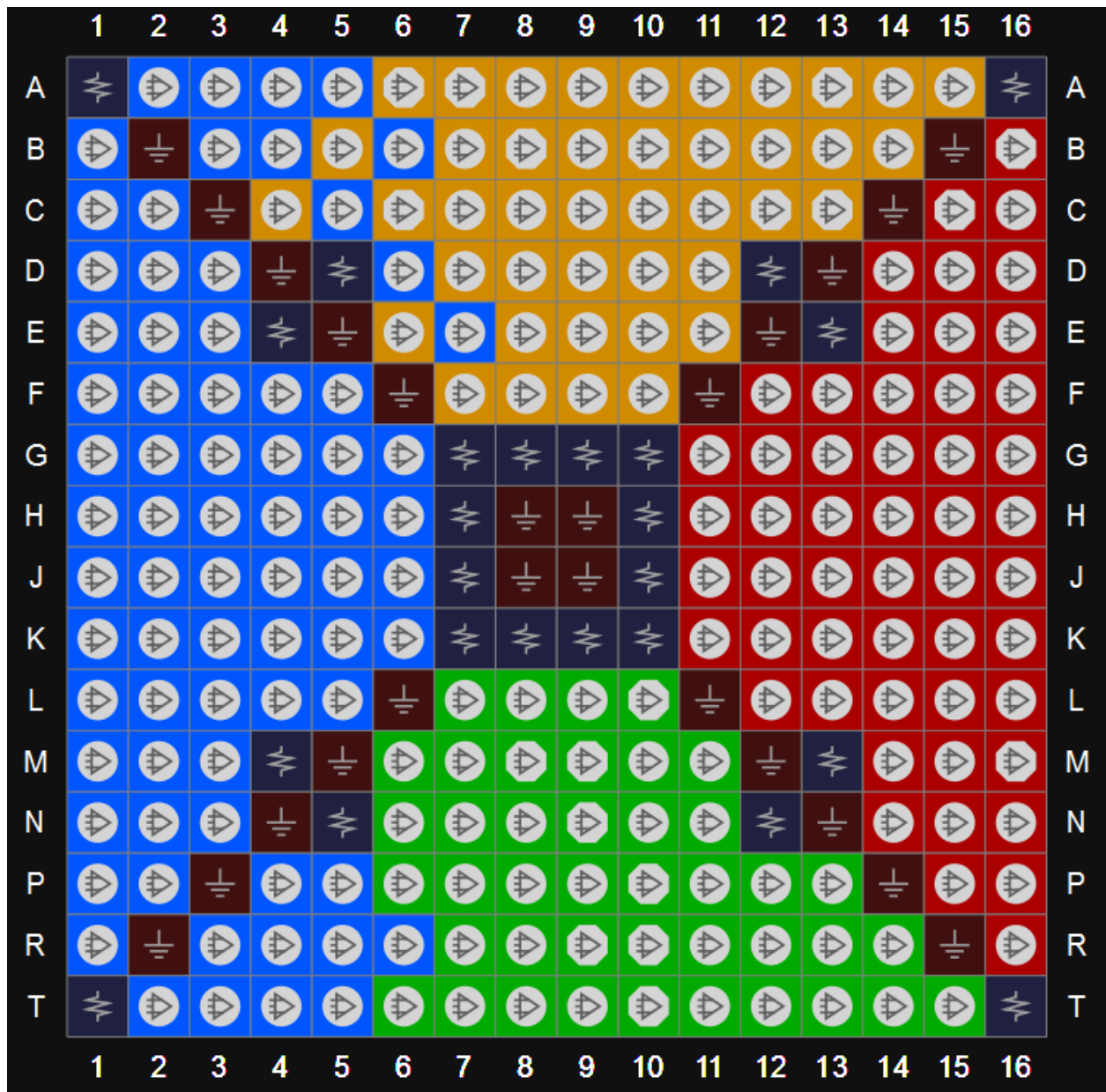
图 3-48 GW1N-4 器件 PG256 封装管脚分布示意图（顶视图）
