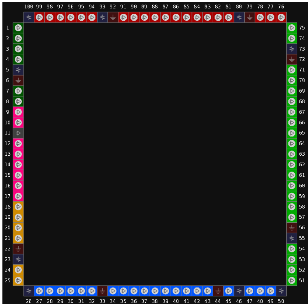
图 3-36 GW1N-1P5 器件 LQ100 封装管脚分布示意图 (UV 版本, 顶视图)
