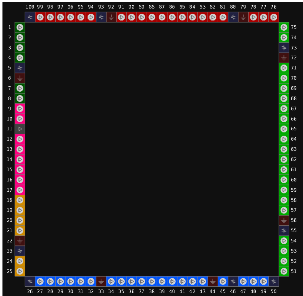
图 3-35 GW1N-1P5 器件 LQ100 封装管脚分布示意图 (LV 版本, 顶视图)
