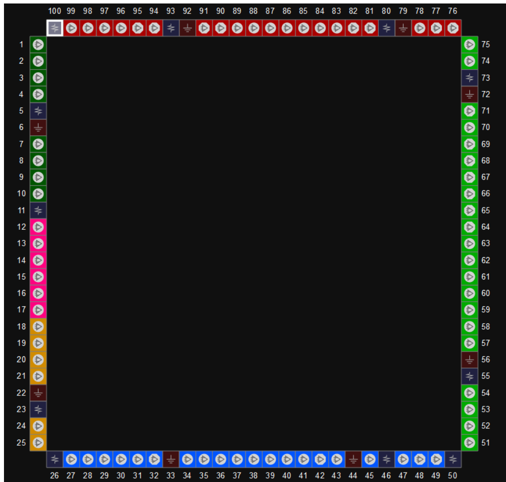
图 3-14 GW1N-2 器件 LQ100 封装管脚分布示意图 (UV 版本,顶视图)
