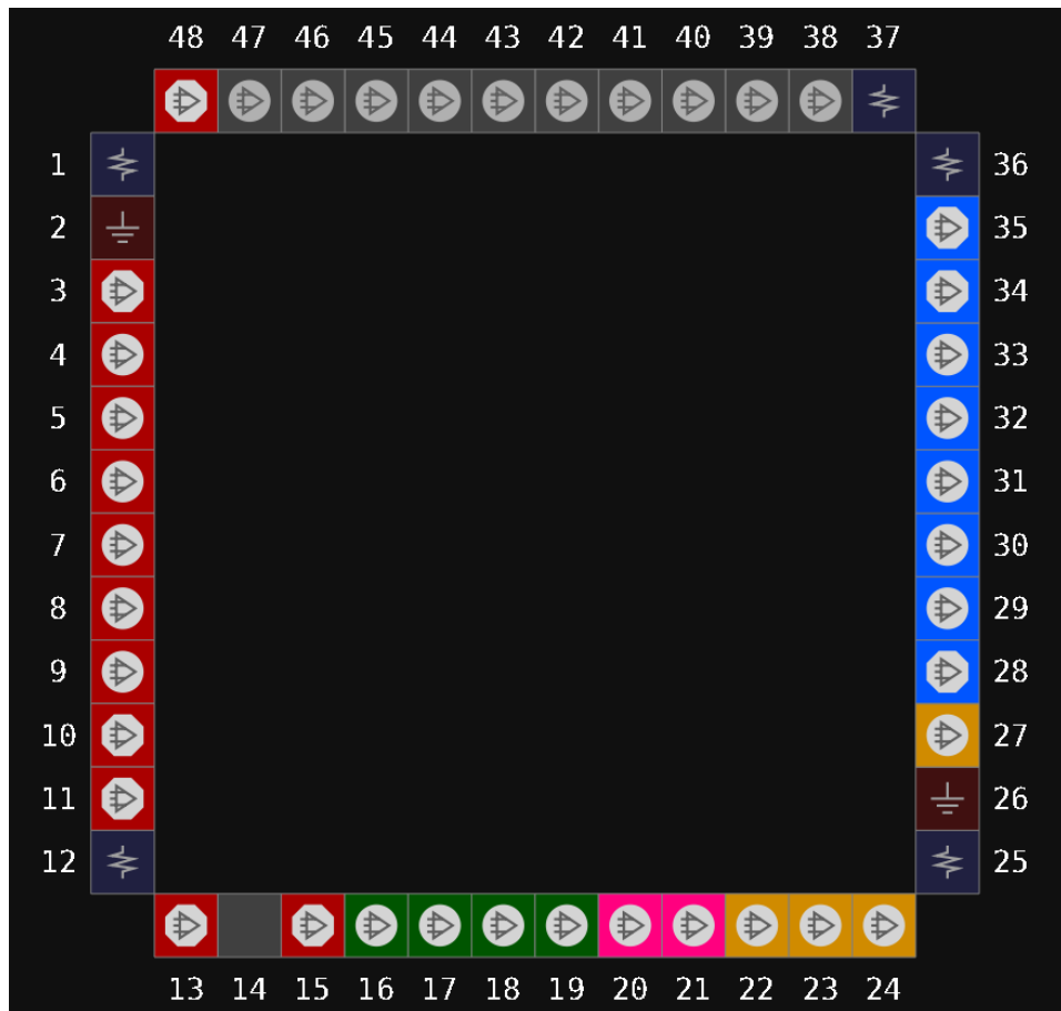
图 3-21 GW1N-2 器件 QN48H 封装管脚分布示意图（顶视图）
