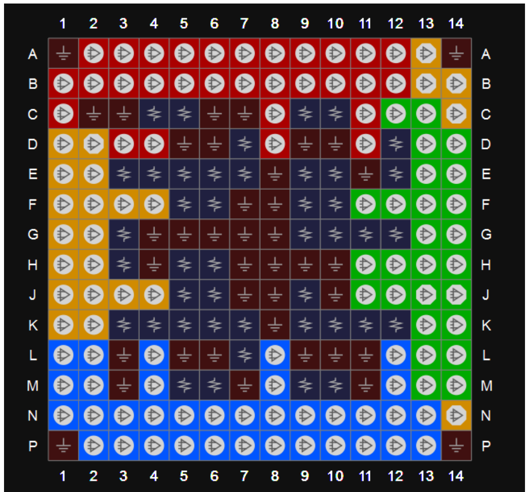
图 3-62 GW1N-9 器件 MG196 封装管脚分布示意图（顶视图）
