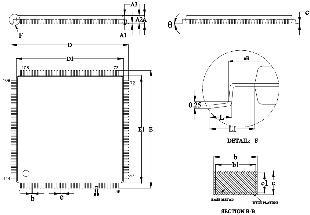
图 4-15 封装尺寸 LQ144 / LQ144X
