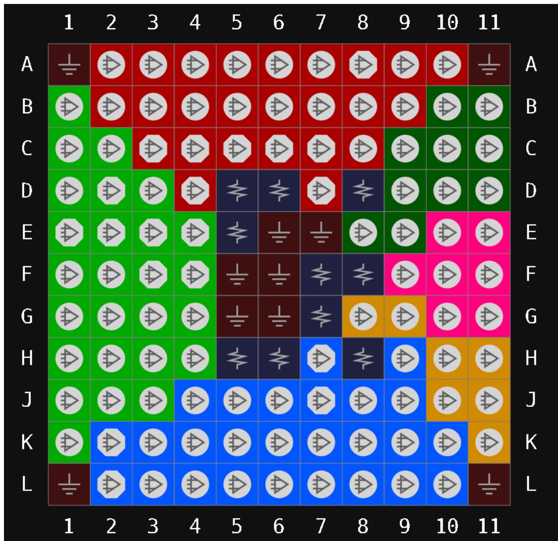
图 3-26 GW1N-2 器件 MG121 封装管脚分布示意图 (UV 版本 顶视图)
