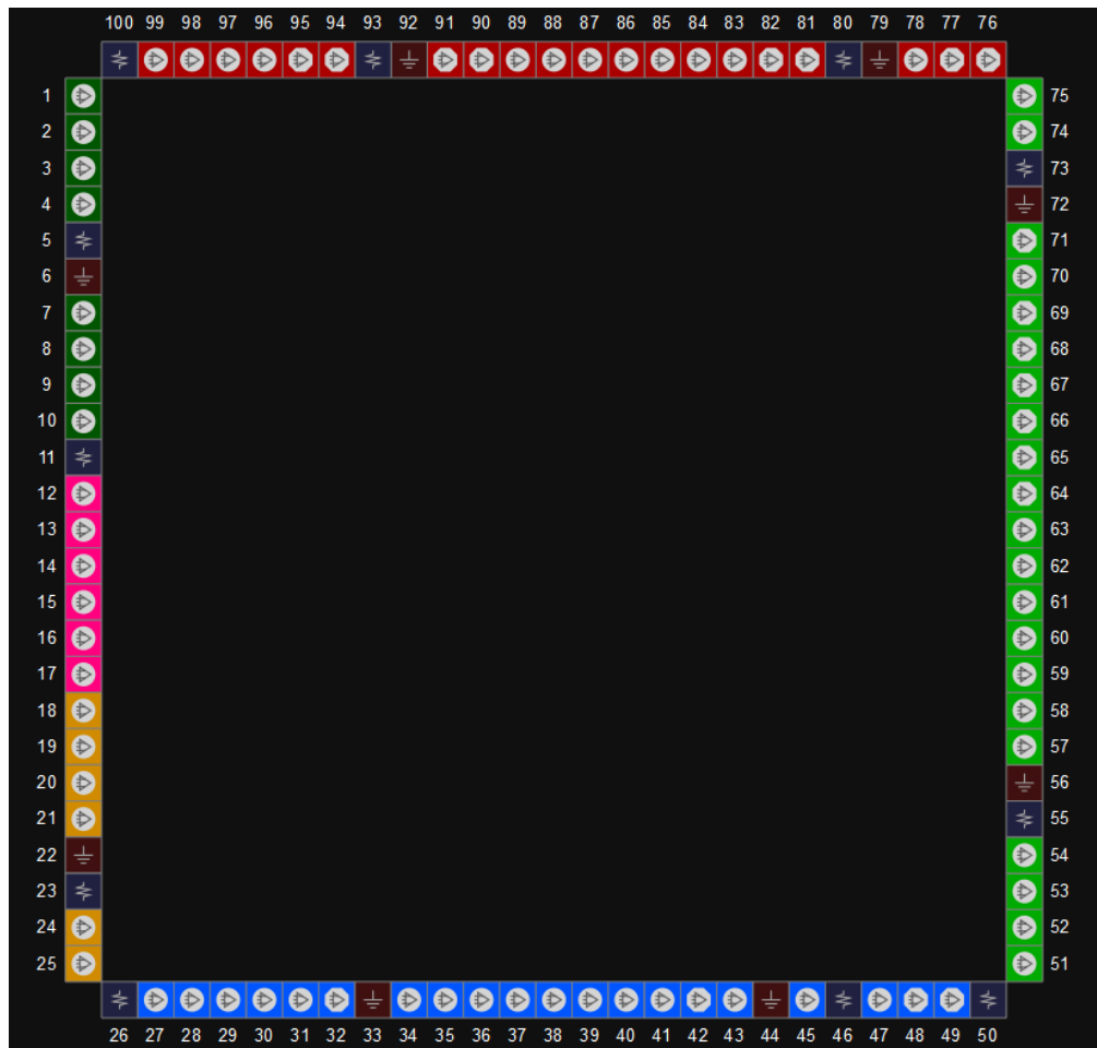
图 3-15 GW1N-2 器件 LQ100 封装管脚分布示意图 (LV 版本,顶视图)
