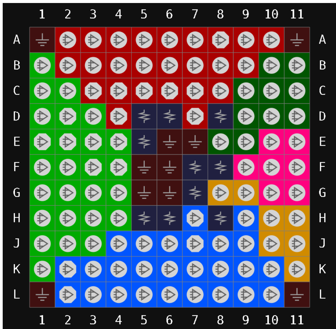
图 3-28 GW1N-2 器件 MG121X 封装管脚分布示意图 (UV 版本 顶视图)
