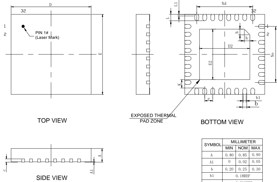
图 4-8 封装尺寸 QN32X
