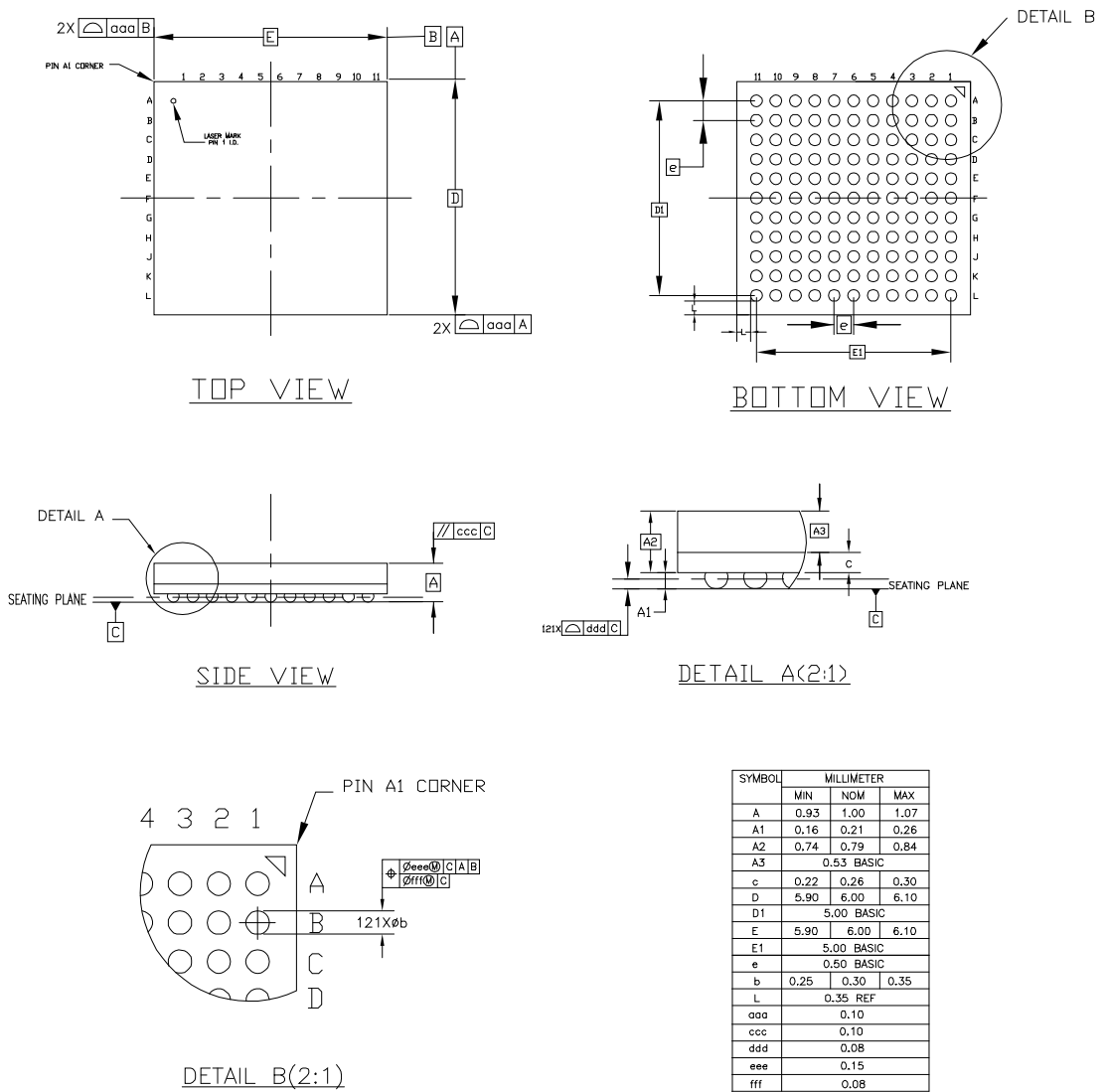
图 4-21 封装尺寸 MG121/ MG121X
