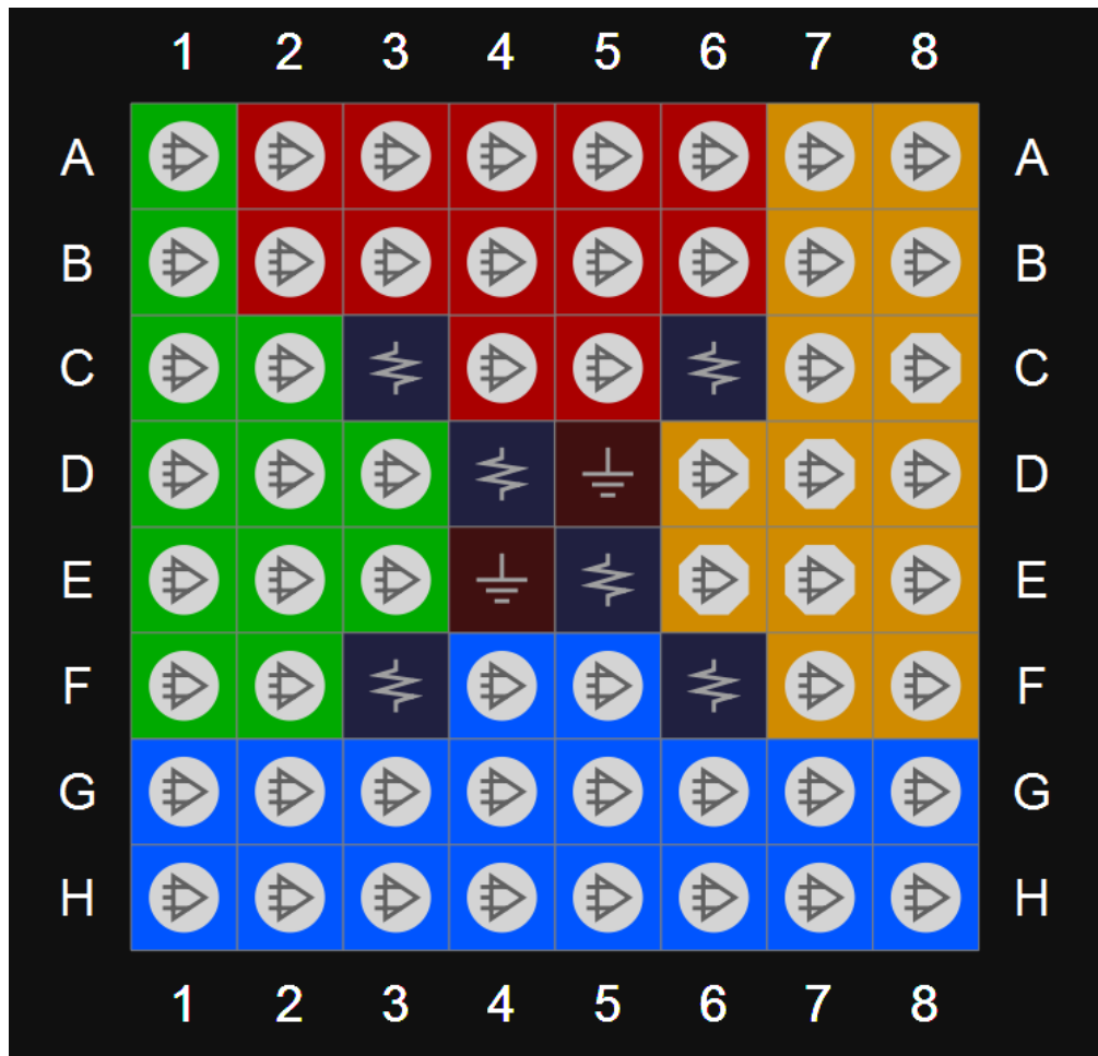
图 3-57 GW1N-9 器件 CM64 封装管脚分布示意图（顶视图）
