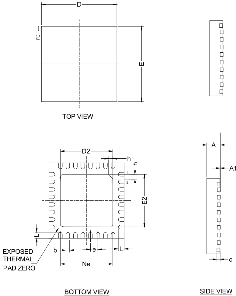
图 4-8 封装尺寸 QN32(GW1N-1/4)
