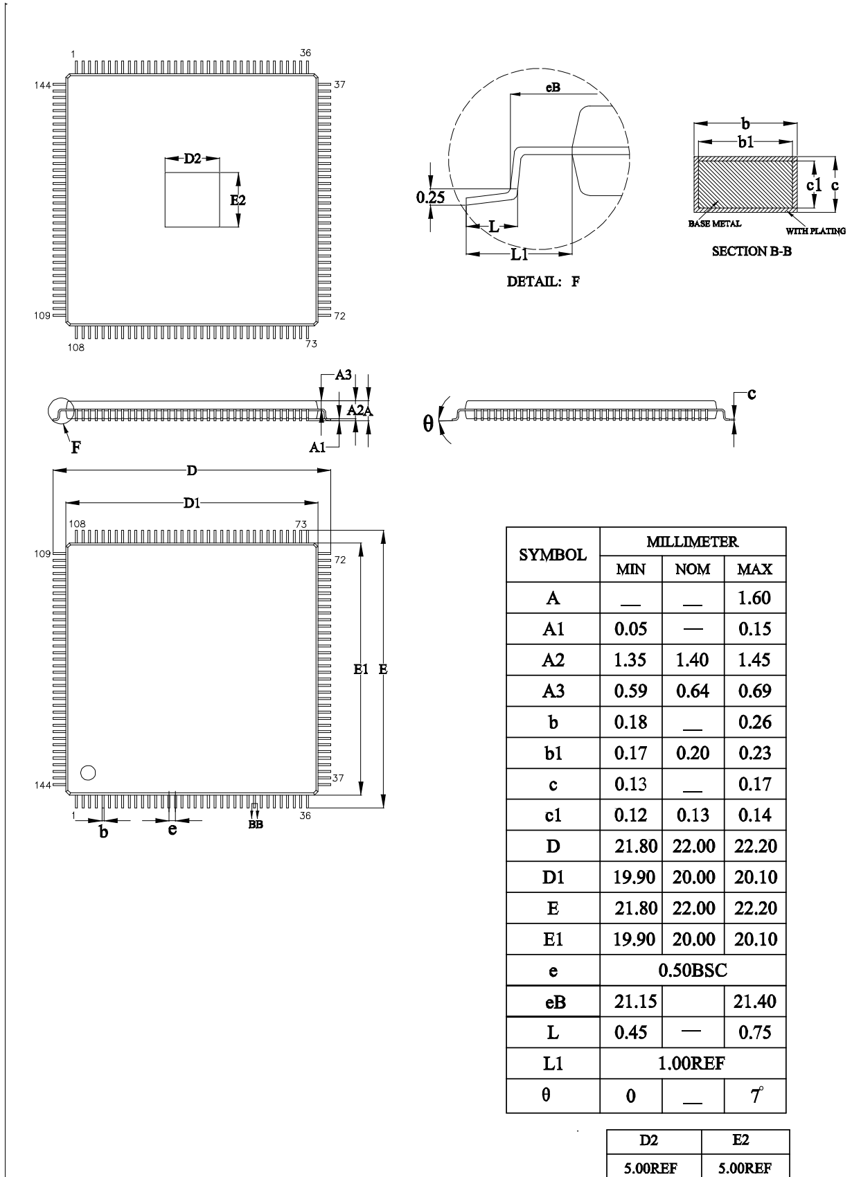
图 4-19 封装尺寸 EQ144
