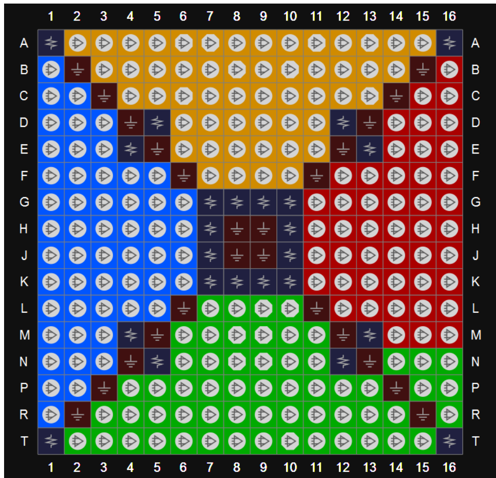
图 3-70 GW1N-9 器件 UG256 封装管脚分布示意图（顶视图）
