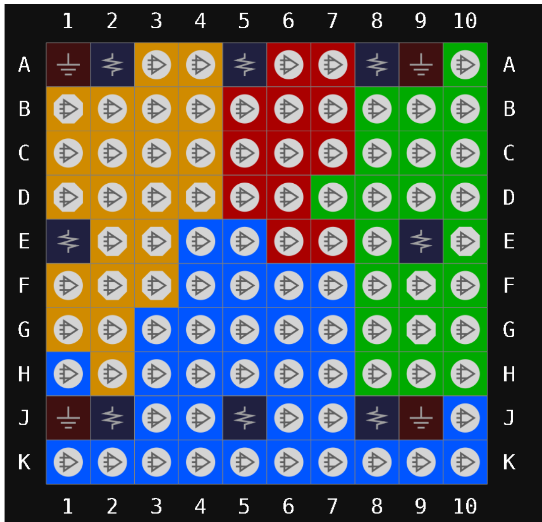
图 3-73 GW1N-9 器件 MG100T 管脚分布示意图（顶视图）
