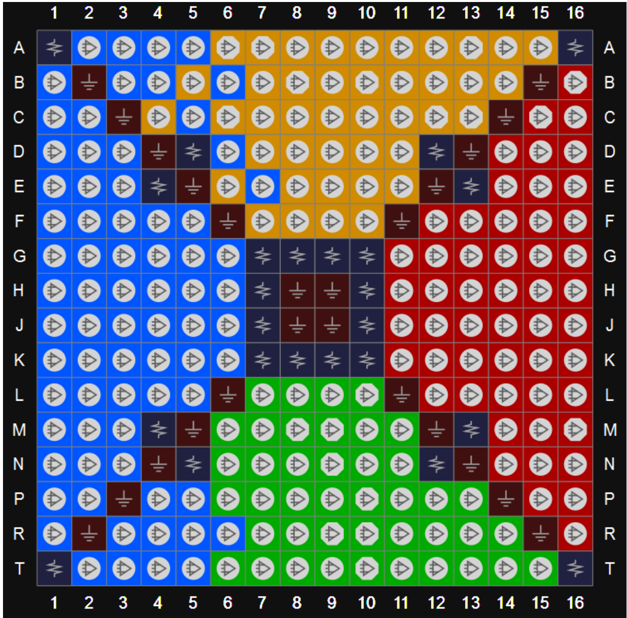
图 3-54 GW1N-4 器件 PG256 封装管脚分布示意图（顶视图）
