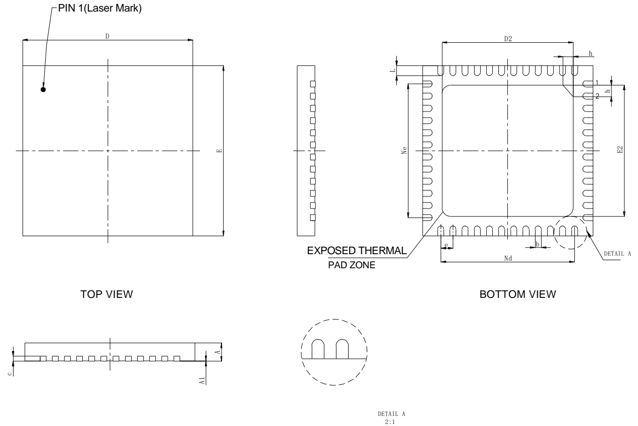
图 4-13 封装尺寸 QN48X
