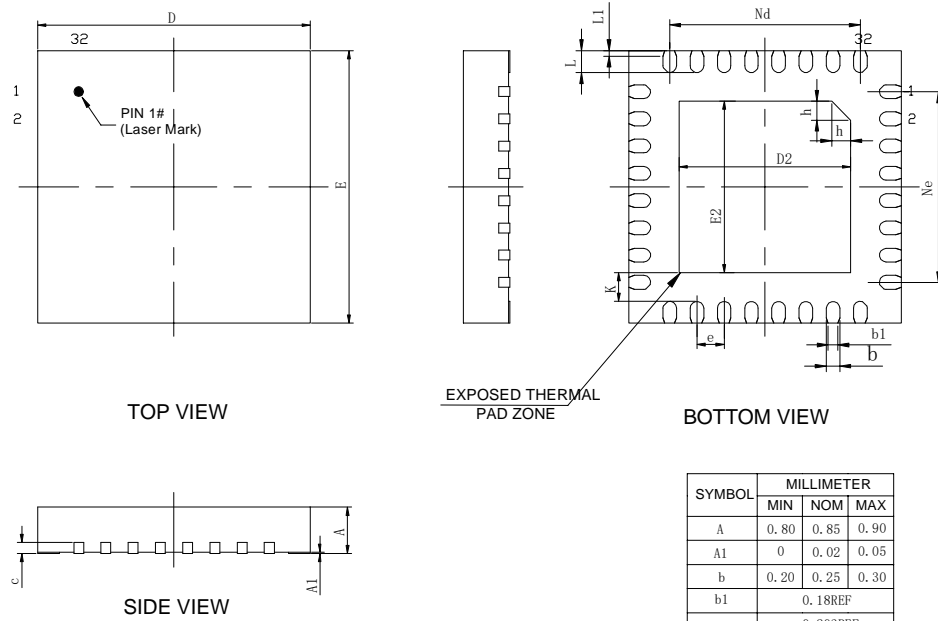
图 4-9 封装尺寸 QN32 (GW1N-2)
