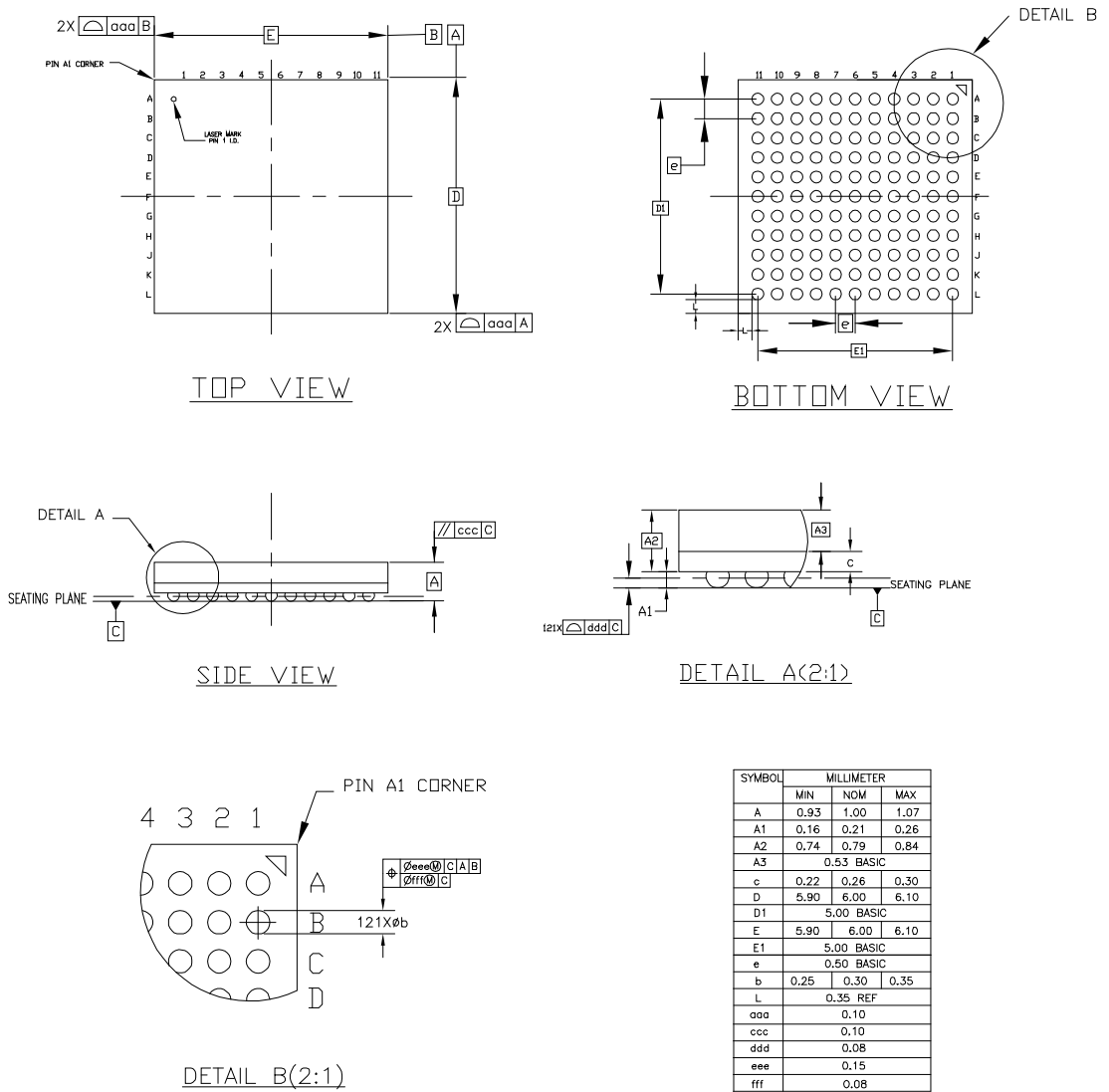
图 4-24 封装尺寸 MG121/ MG121X
