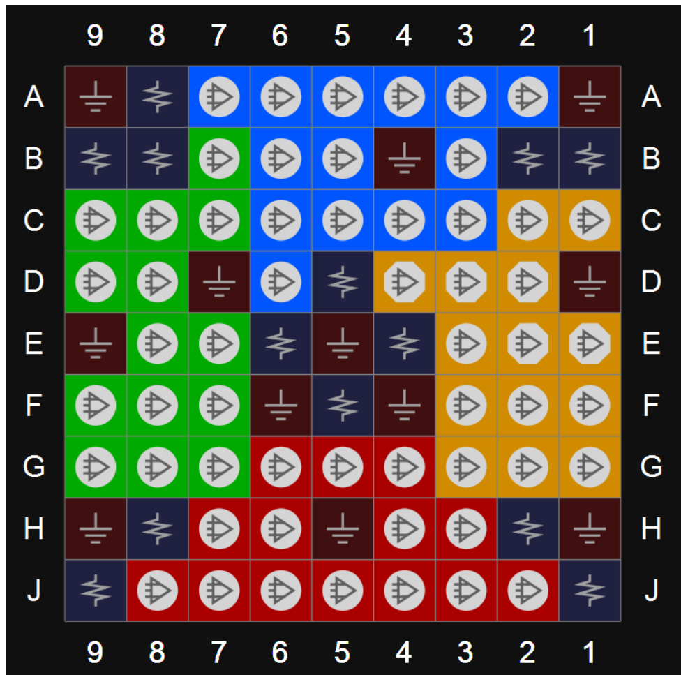
图 3-58 GW1N-9 器件 CS81M 封装管脚分布示意图（顶视图）
