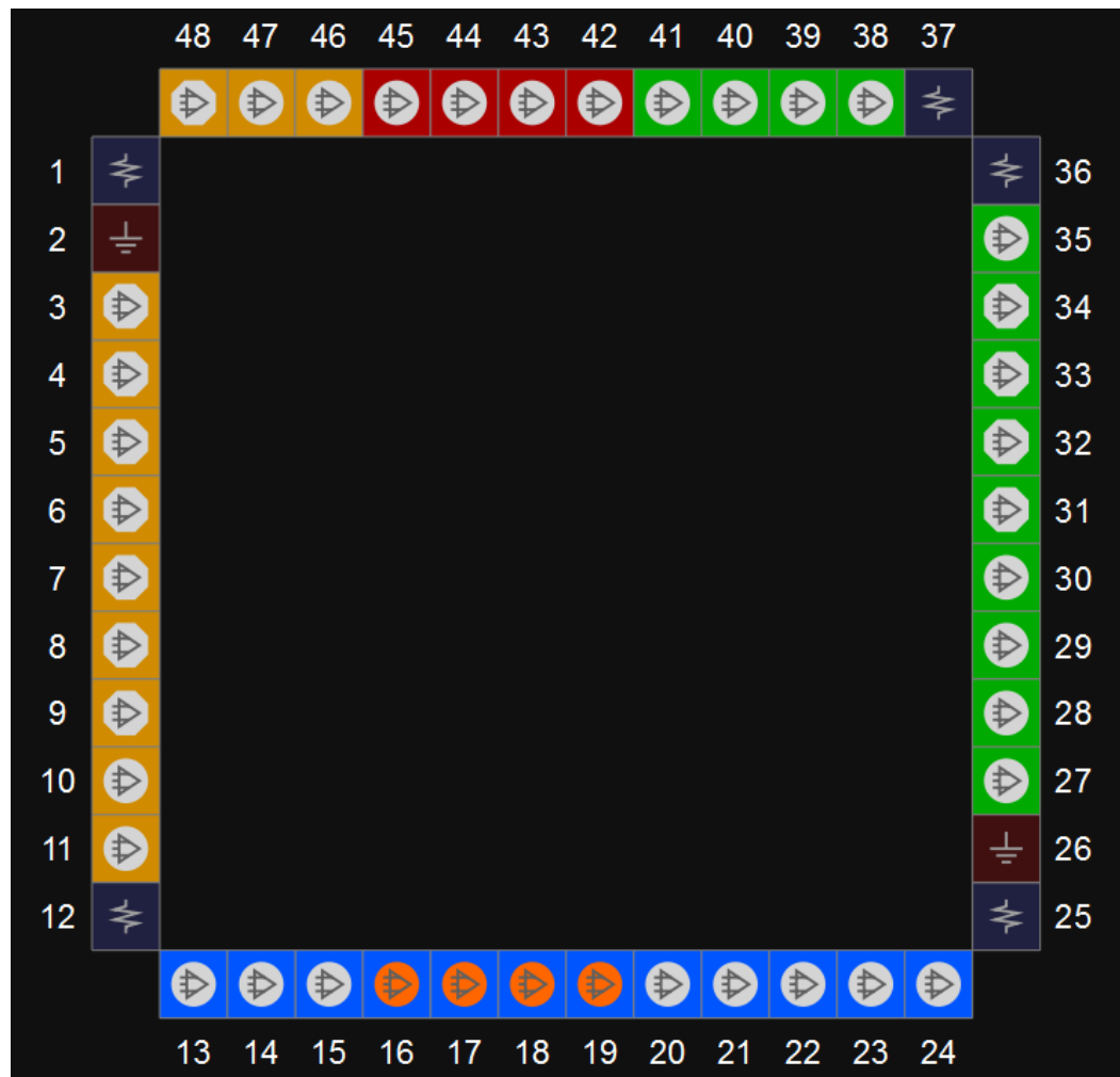
图 3-56 GW1N-9 器件 QN48 封装管脚分布示意图（顶视图）
