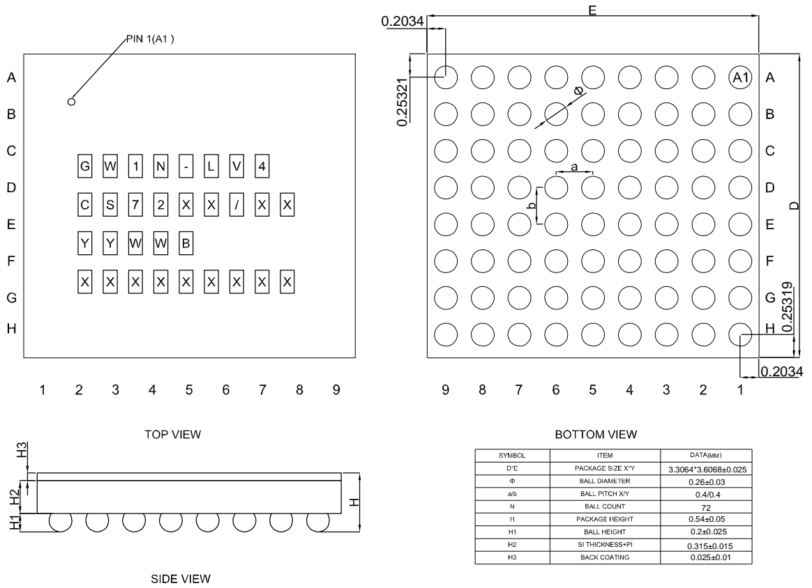
图 4-5 封装尺寸 CS72
