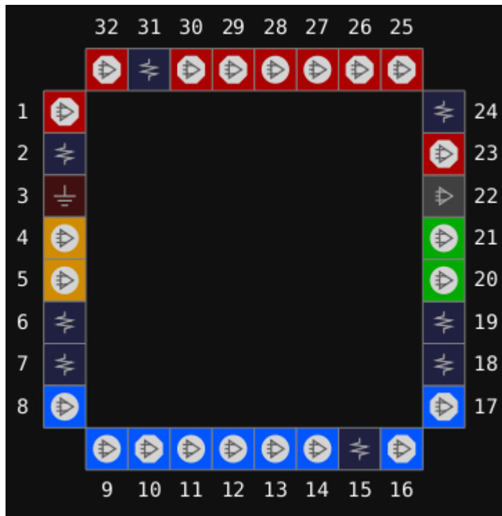
图 3-33 GW1N-2 器件 QN32 LV 版本封装管脚分布示意图（顶视图）
