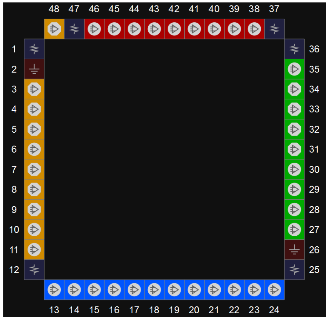
图 3-72 GW1N-9 器件 QN48F 管脚分布示意图（顶视图）
