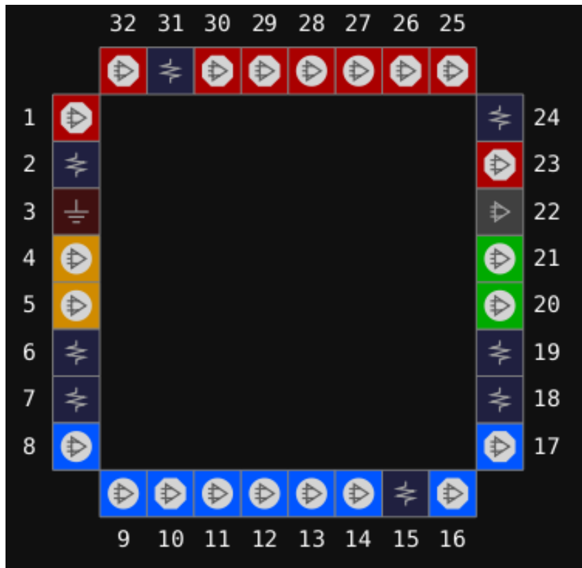
图 3-35 GW1N-2 器件 QN32X LV 版本封装管脚分布示意图（顶视图）
