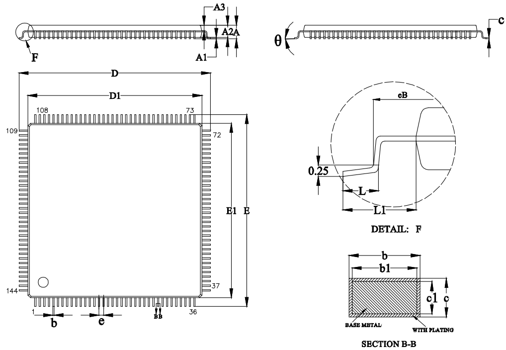
图 4-18 封装尺寸 LQ144 / LQ144X / LQ144F
