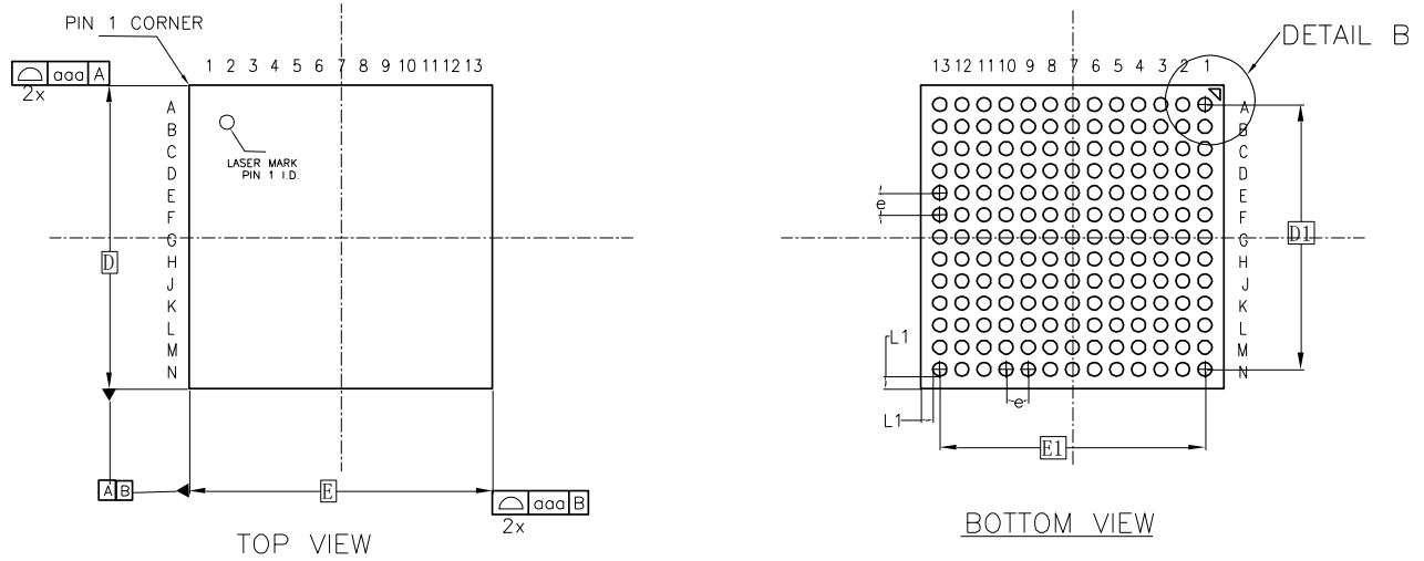
图 4-30 封装尺寸 UG169
