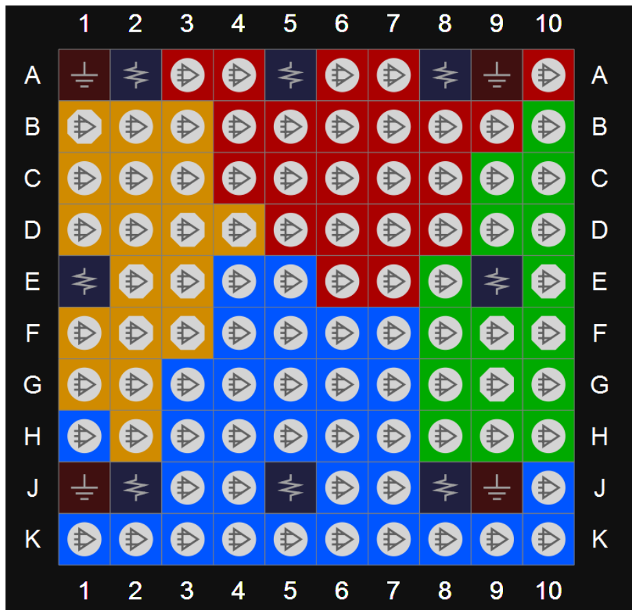
图 3-61 GW1N-9 器件 MG100 封装管脚分布示意图（顶视图）
