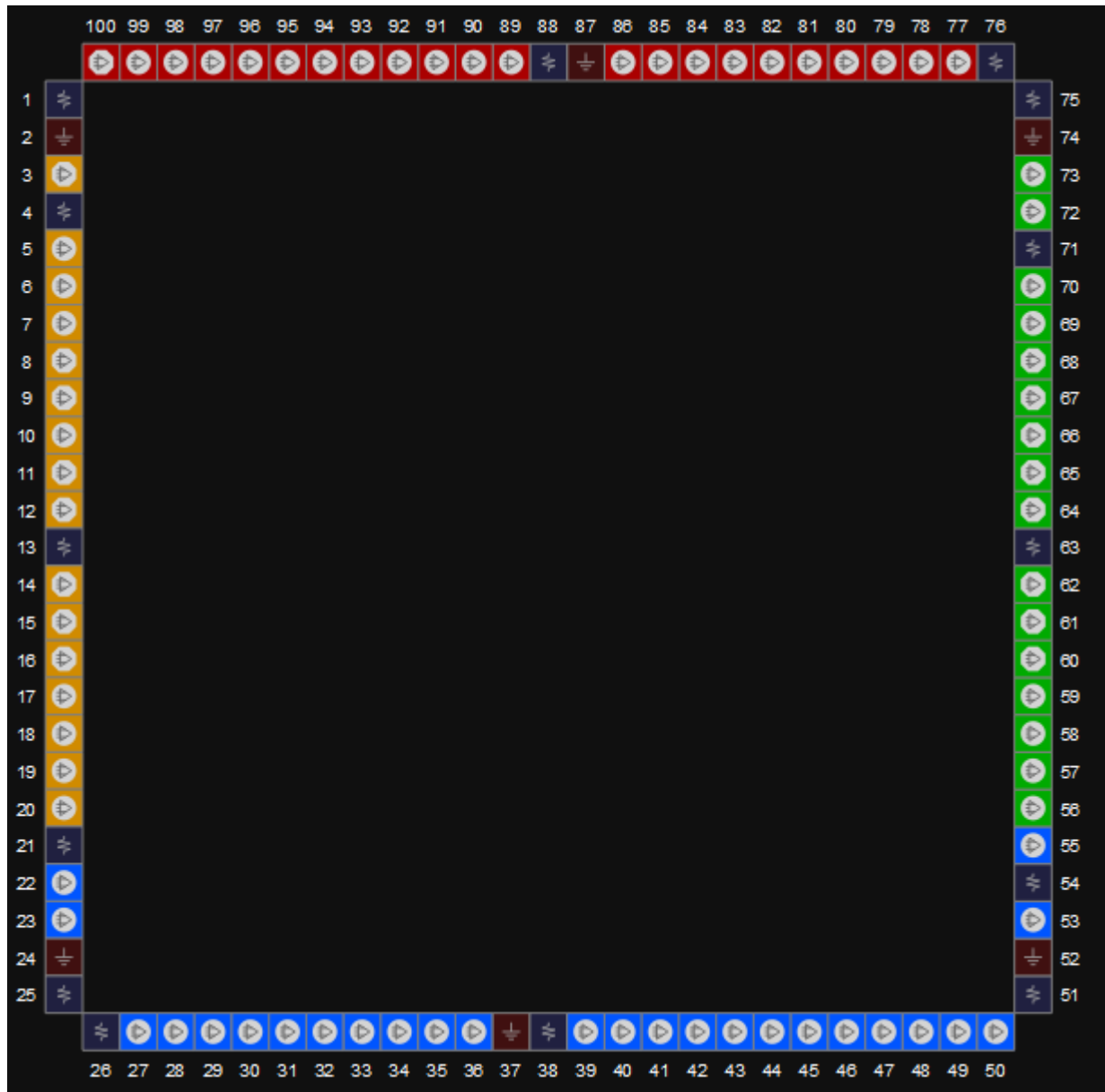
图 3-49 GW1N-4 器件 LQ100 封装管脚分布示意图（顶视图）
