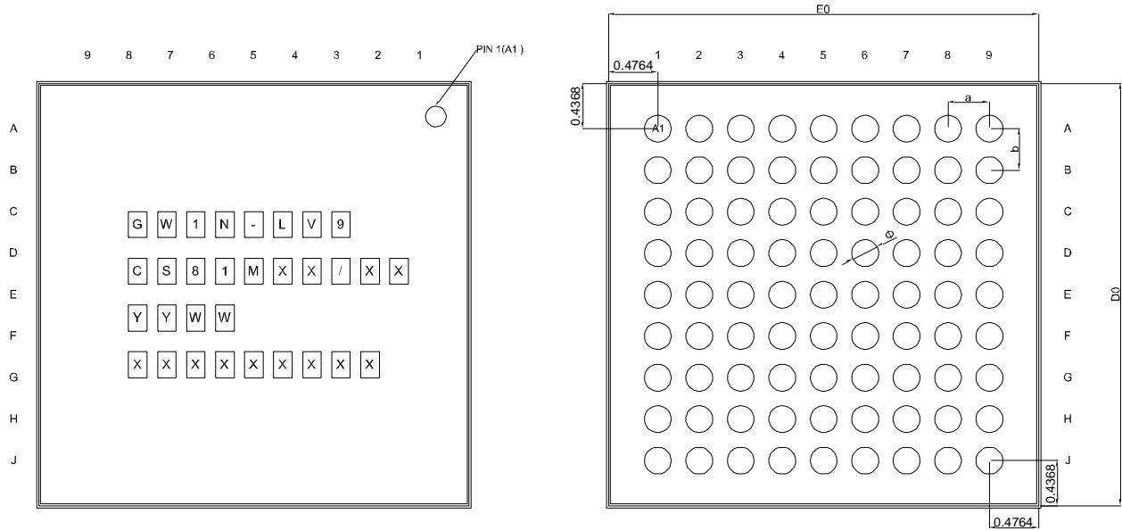
图 4-15 封装尺寸 CS81M
