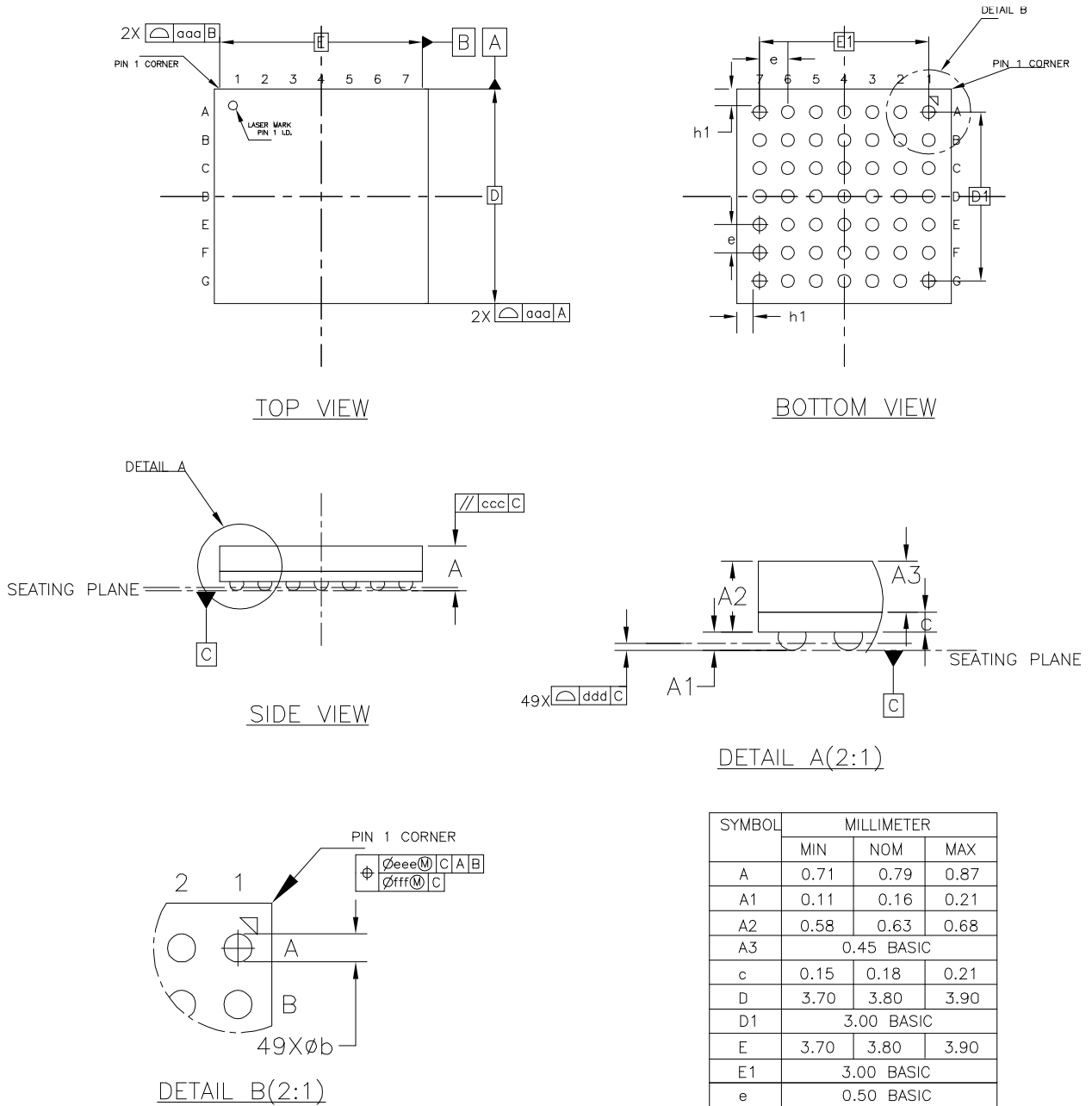
图 4-22 封装尺寸 MG49
