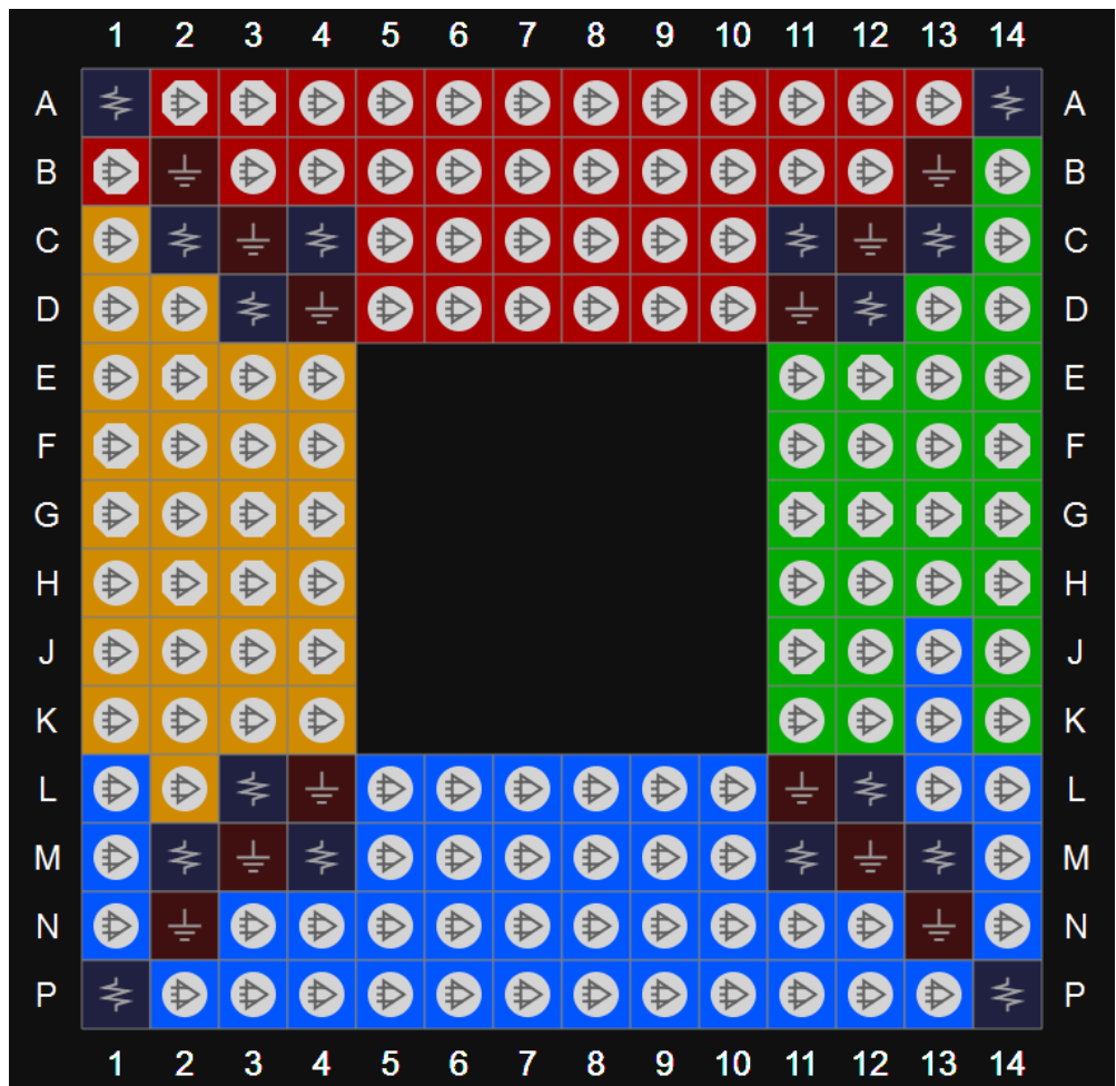
图 3-52 GW1N-4 器件 MG160 封装管脚分布示意图（顶视图）
