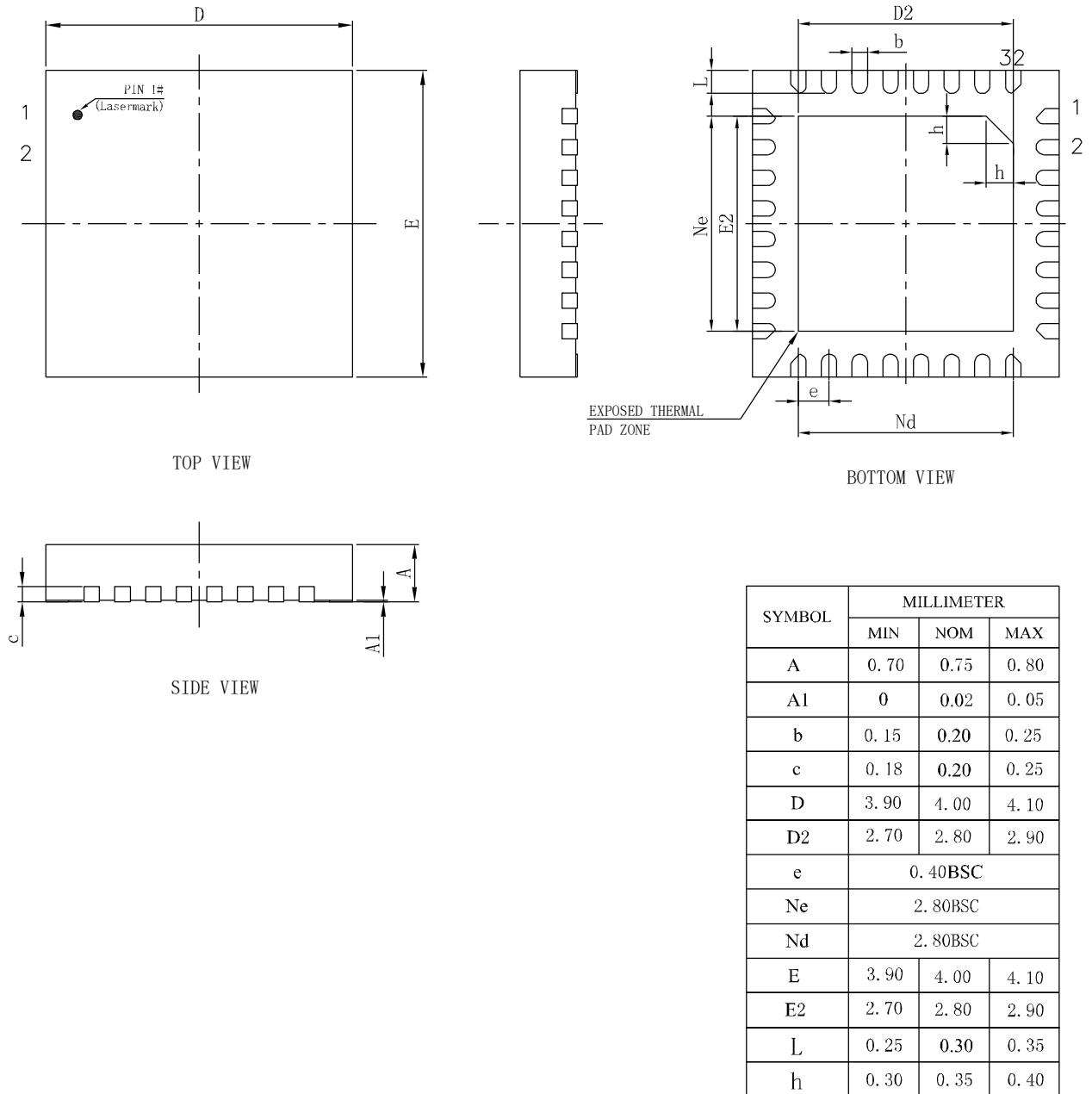
图 4-7 封装尺寸 FN32(GW1N-1S)
