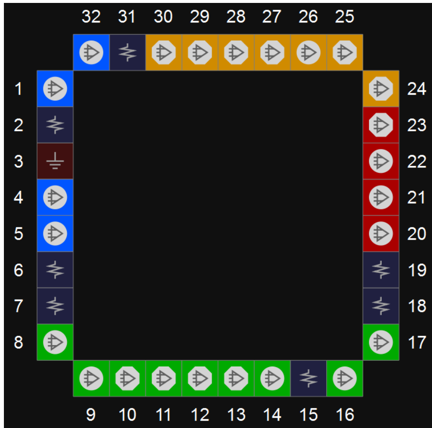
图 3-45 GW1N-4 器件 QN32 封装管脚分布示意图（顶视图）
