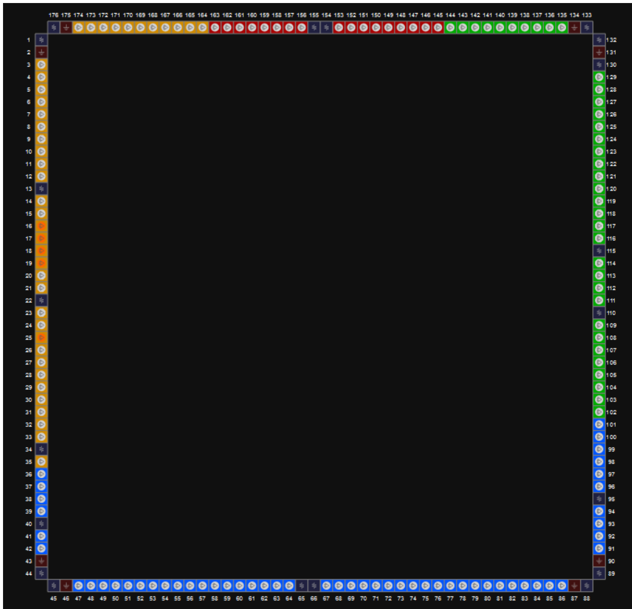
图 3-66 GW1N-9 器件 LQ176 封装管脚分布示意图（顶视图）
