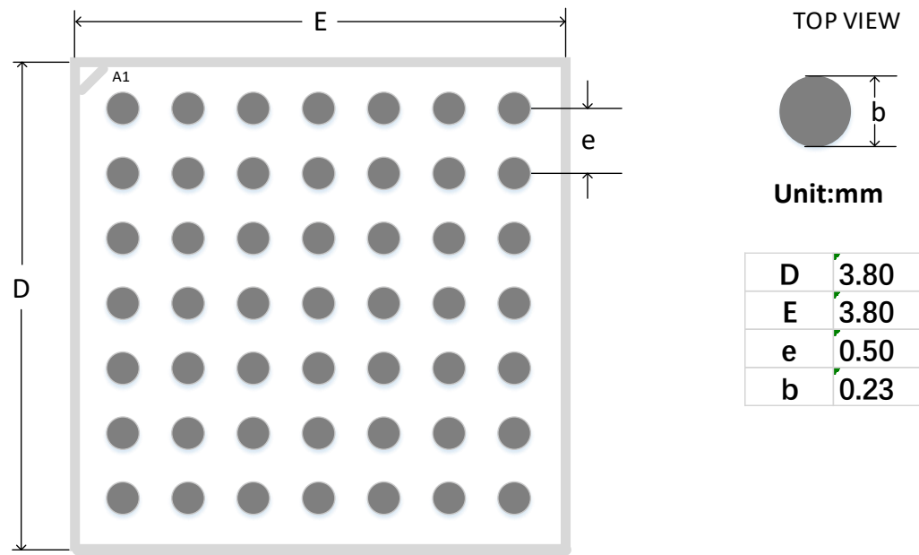
图 4-44 推荐 PCB Layout MG49
