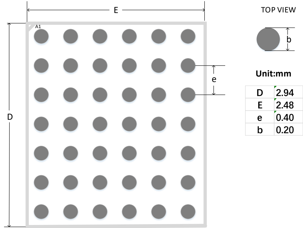
图 4-8 推荐 PCB Layout CS42H
