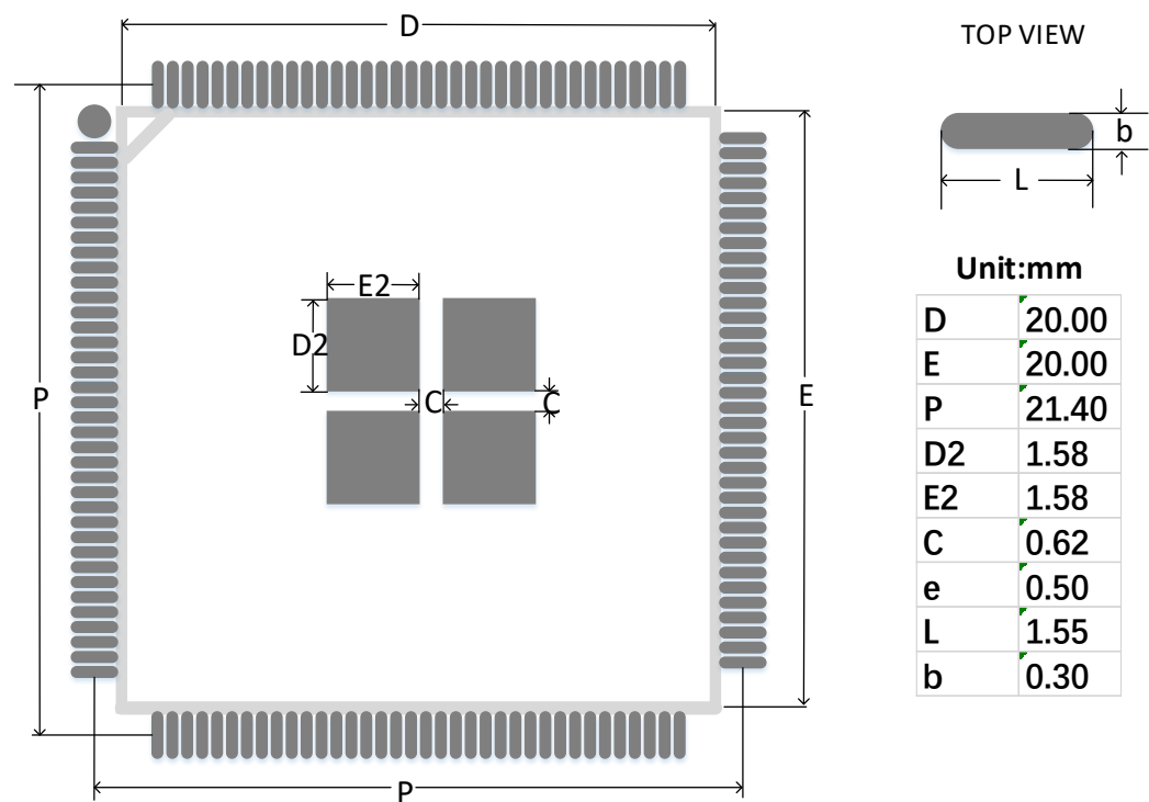
图 4-38 推荐 PCB Layout EQ144
