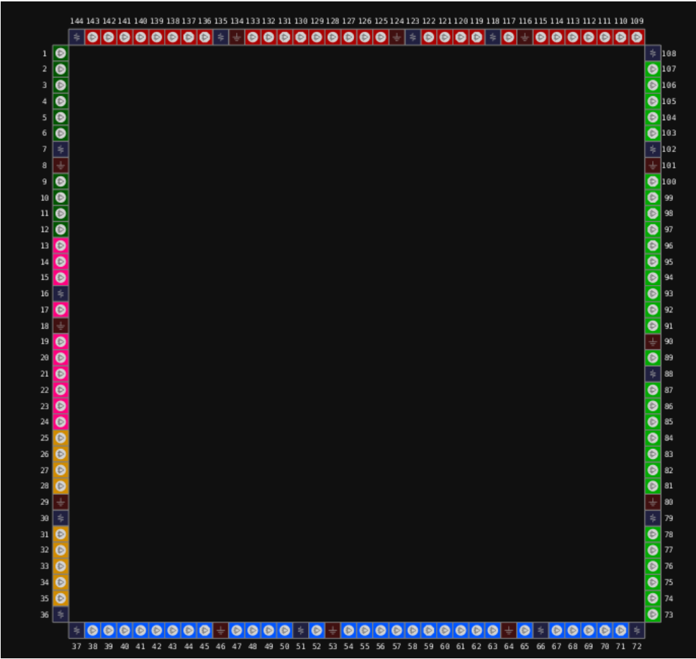
图 3-21 GW1N-2 器件 LQ144F 封装管脚分布示意图（UV 版本,顶视图）
