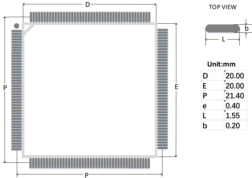
图 4-40 推荐 PCB Layout LQ176
