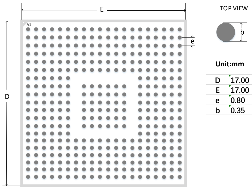
图 4-64 推荐 PCB Layout UG332
