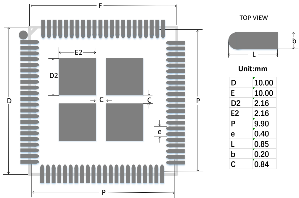
图 4-32 推荐 PCB Layout QN88
