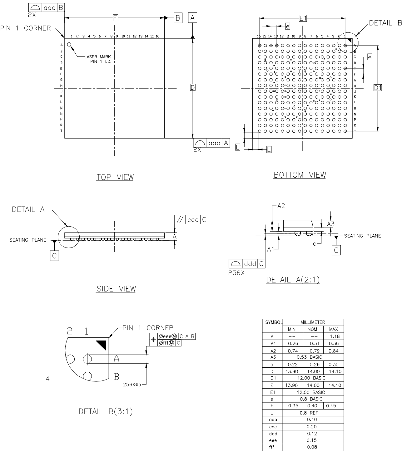
图 4-61 封装尺寸 UG256
