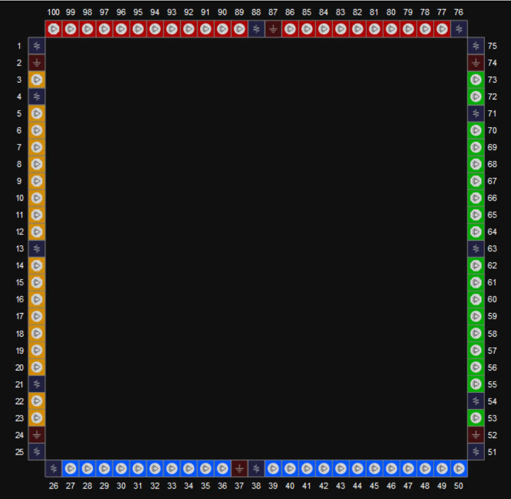
图 3-6 GW1N-1 器件 LQ100 封装管脚分布示意图（顶视图）
