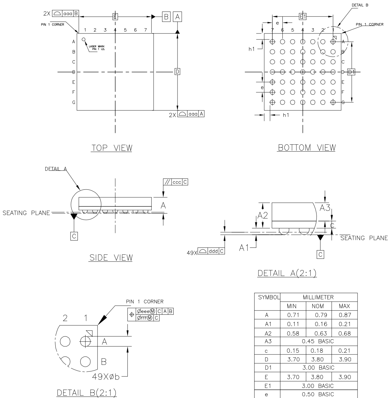
图 4-43 封装尺寸 MG49
