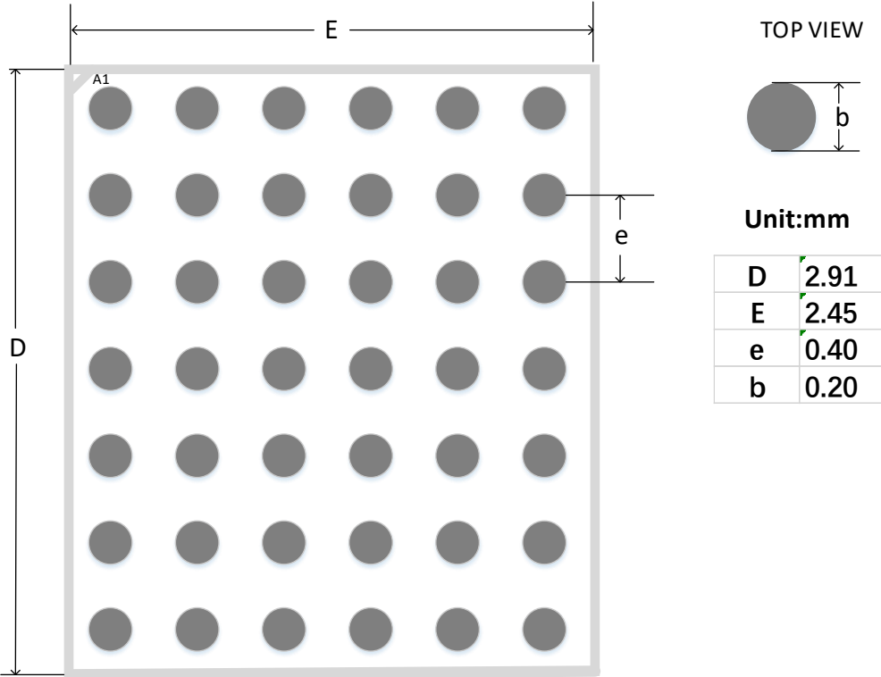
图 4-6 推荐 PCB Layout CS42
