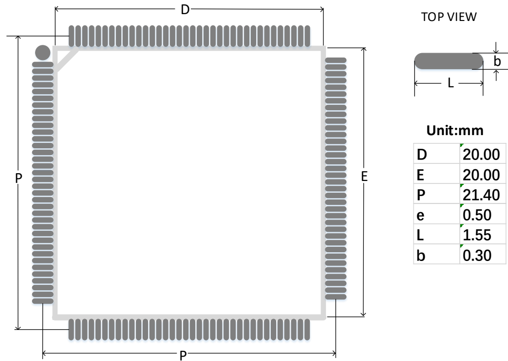
图 4-36 推荐 PCB Layout LQ144/LQ144X/LQ144F
