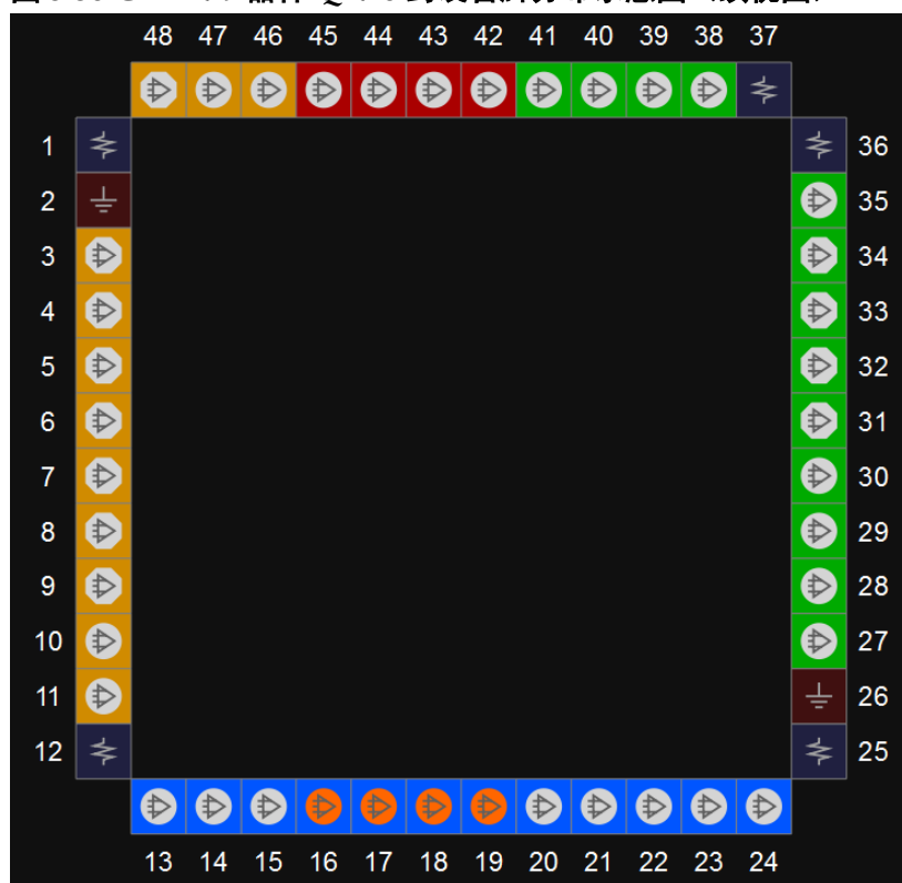
图 3-58 GW1N-9 器件 QN48 封装管脚分布示意图 (顶视图)
