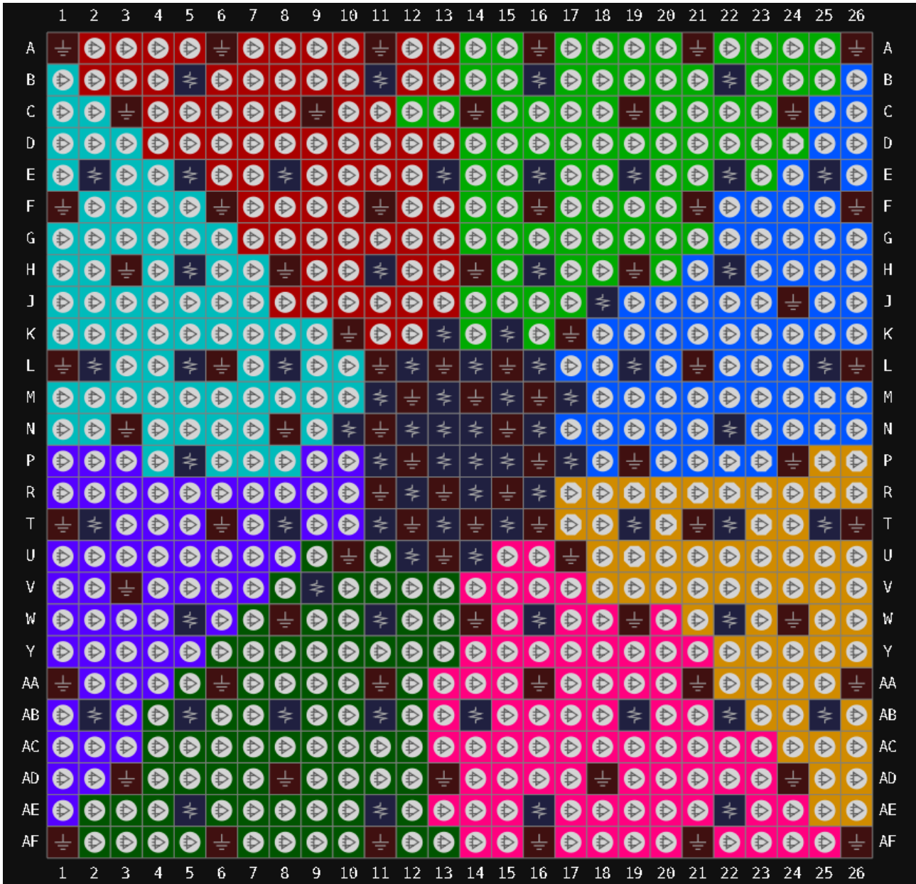
图 3-15 GW 2A-55 器件 UG676 封装管脚分布示意图
