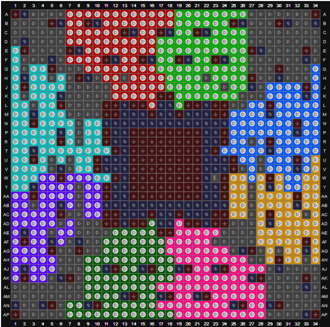
图 3-16 GW 2A-55 器件 PG1156 封装管脚分布示意图
