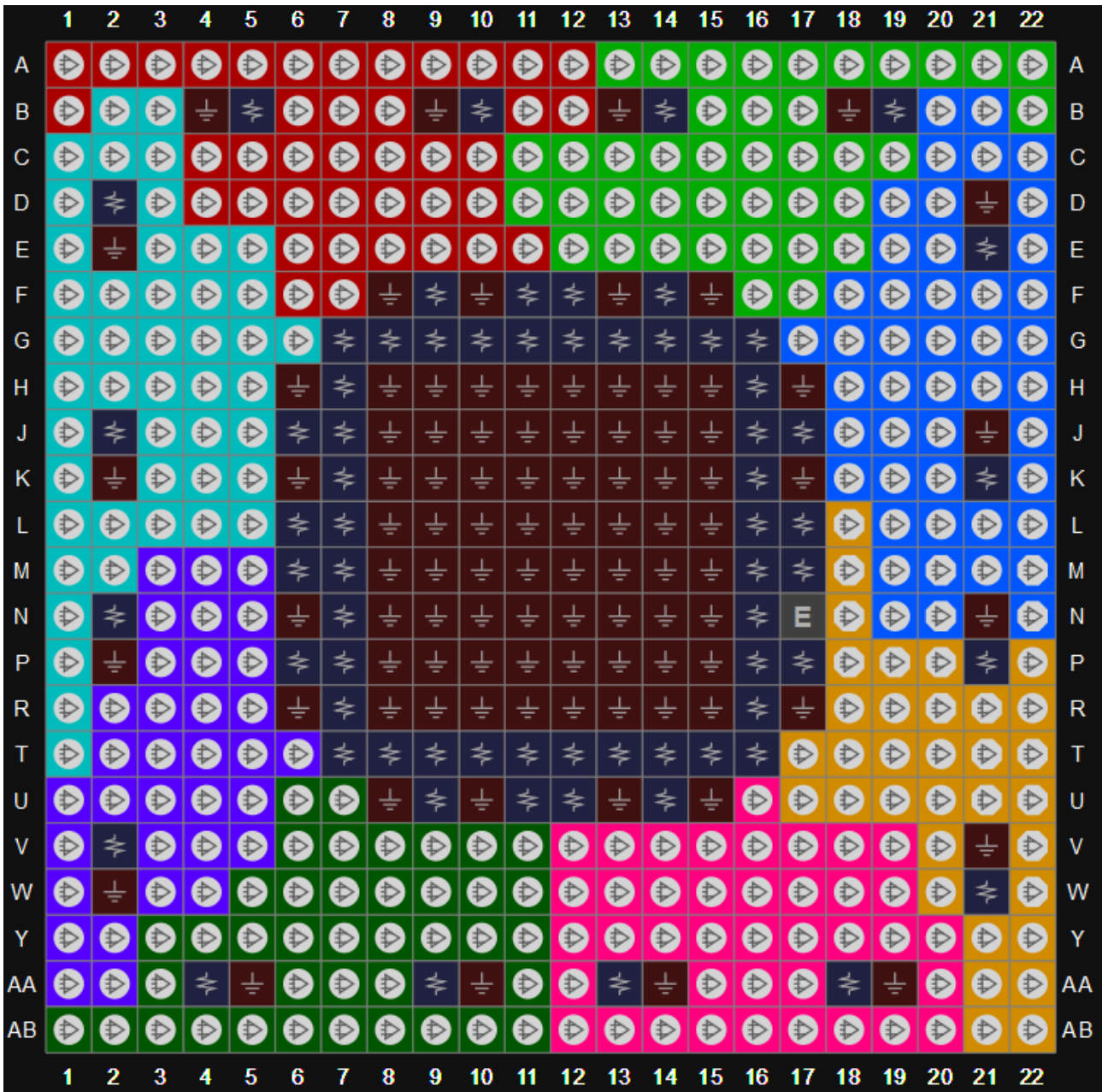
图 3-15 GW2A-55 器件 PG484 封装管脚分布示意图
