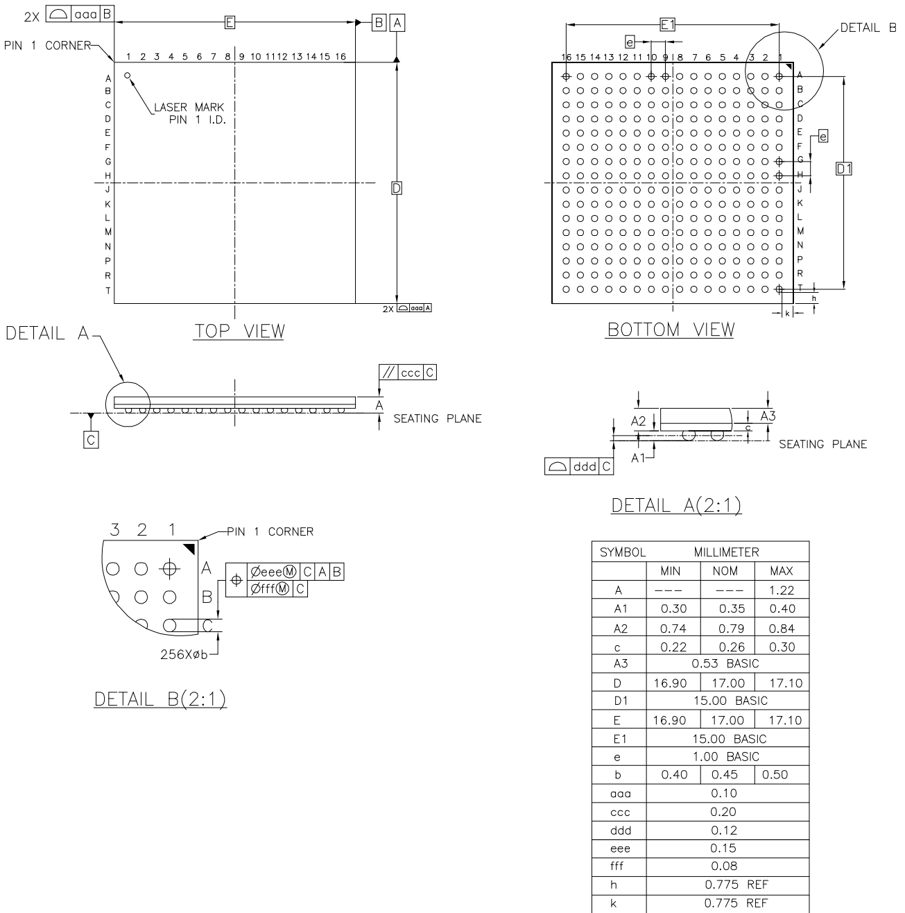
图 4-6 封装尺寸 PG256C/PG256CF
