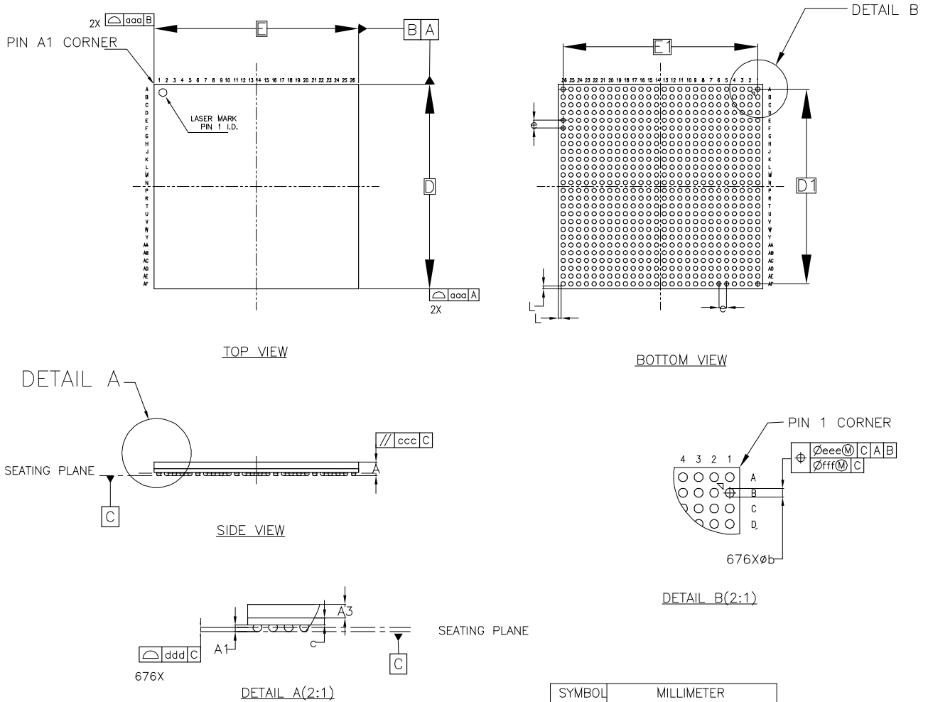
图 4-15 封装尺寸 UG676
