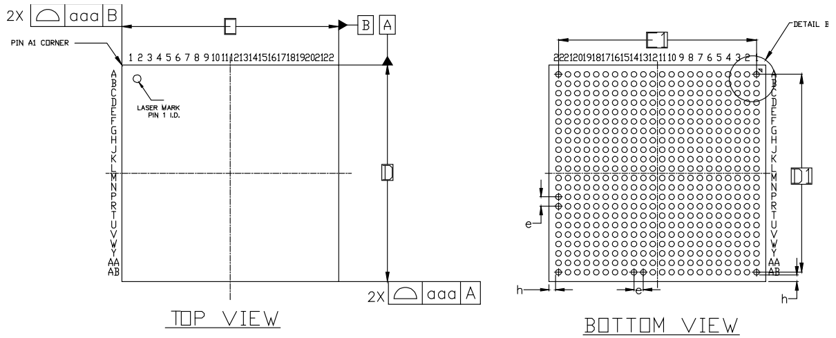
图 4-10 封装尺寸 PG484C
