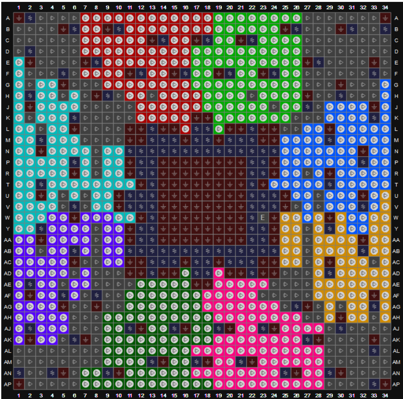
图 3-18 GW2A-55 器件 PG1156 封装管脚分布示意图
