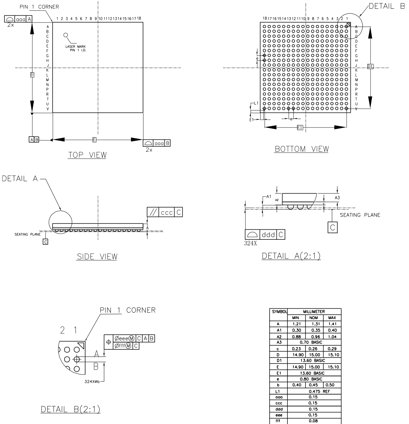
图 4-13 封装尺寸 UG324/UG324D/UG324F
