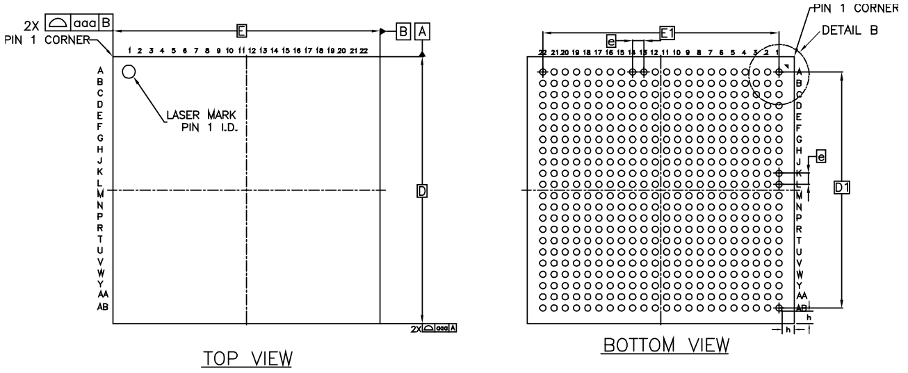
图 4-14 封装尺寸 UG484/UG484S
