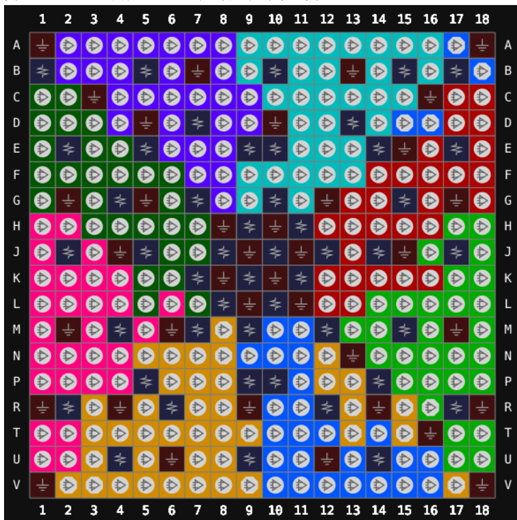
图 3-8 GW2A-18 器件 UG324 封装管脚分布示意图
