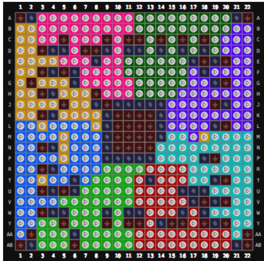
图 3-10 GW2A-18 器件 PG484C 封装管脚分布示意图
