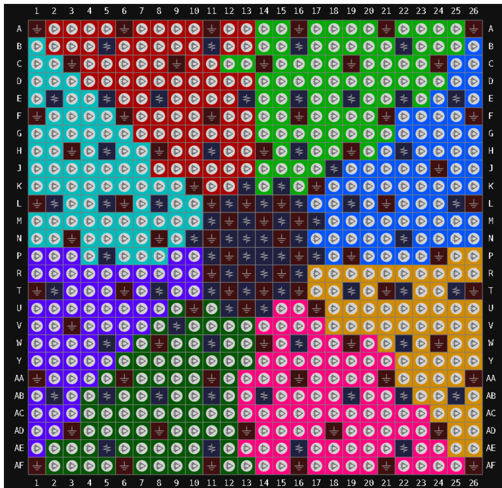
图 3-19 GW2A-55 器件 UG676 封装管脚分布示意图
