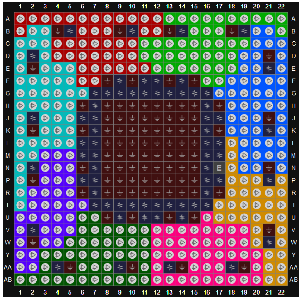
图 3-9 GW2A-18 器件 PG484 封装管脚分布示意图
