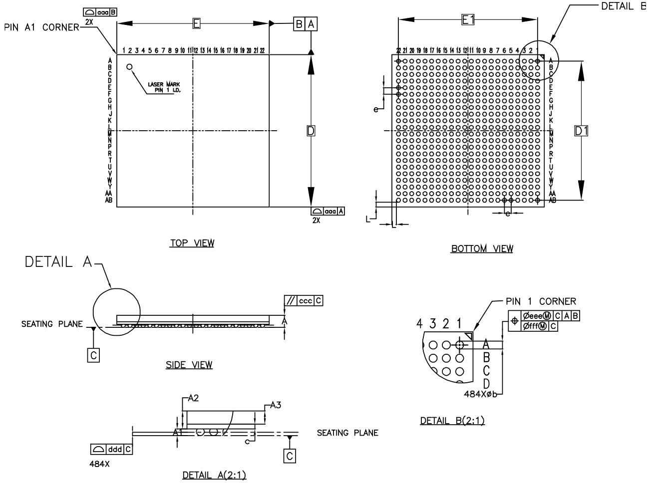
图 4-11 封装尺寸 PG484 (GW2A-55)
