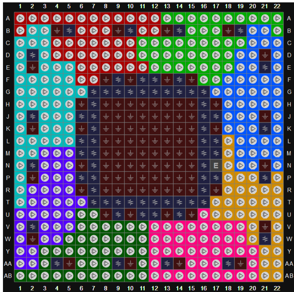
图 3-17 GW2A-55 器件 PG484 封装管脚分布示意图
