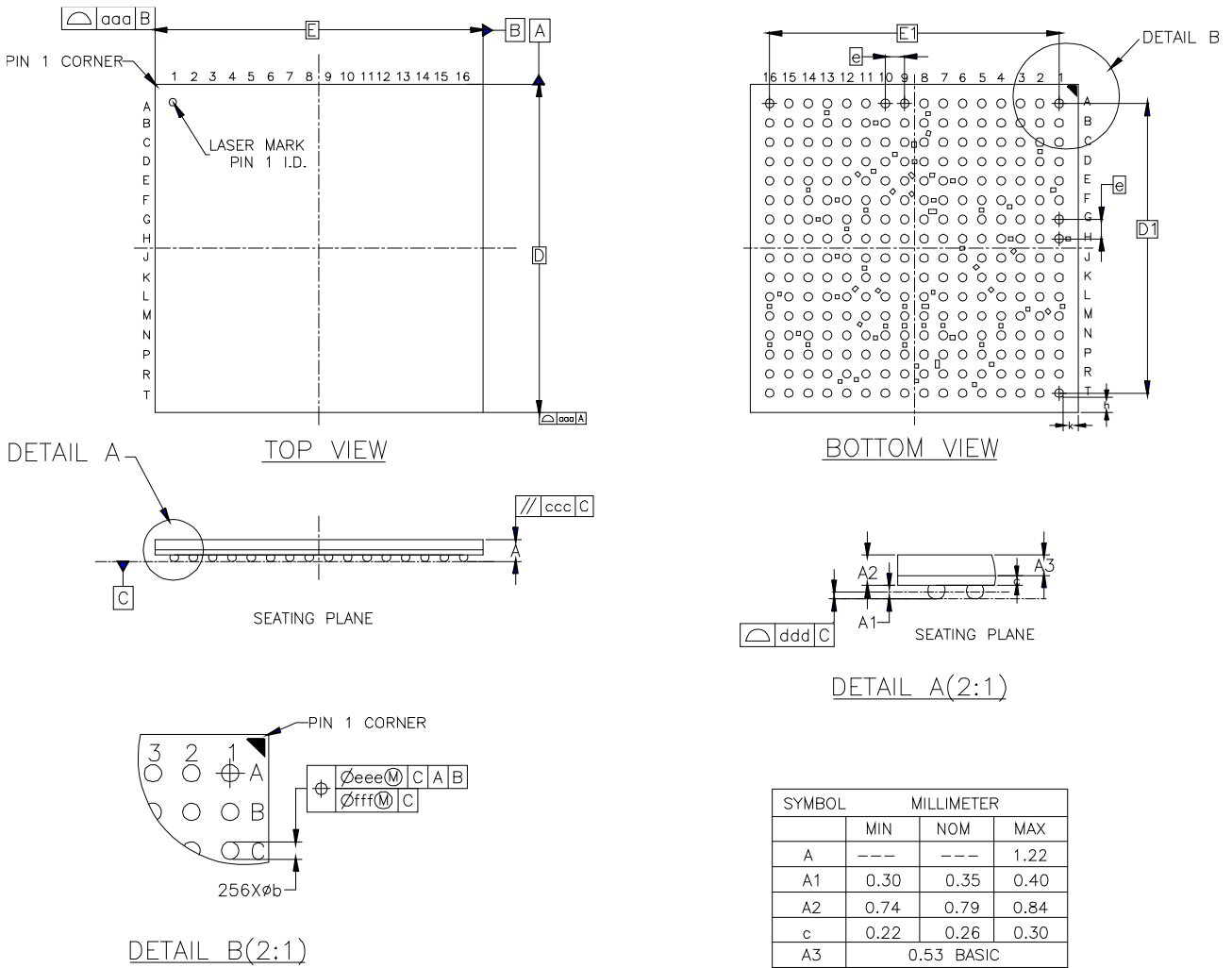
图 4-5 封装尺寸 PG256
