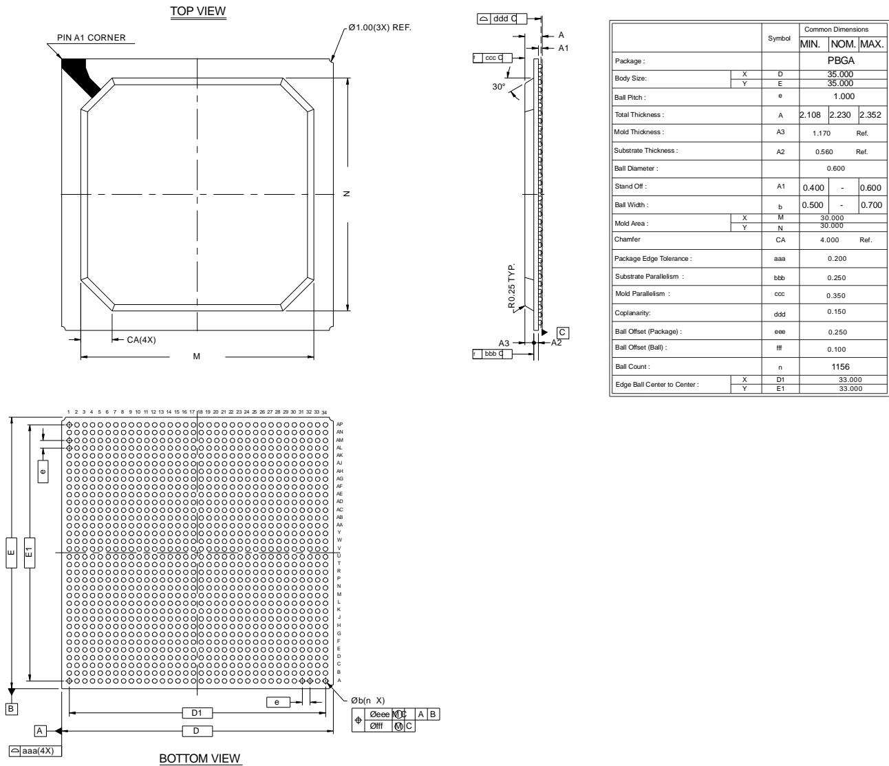
图 4-12 封装尺寸 PG1156
