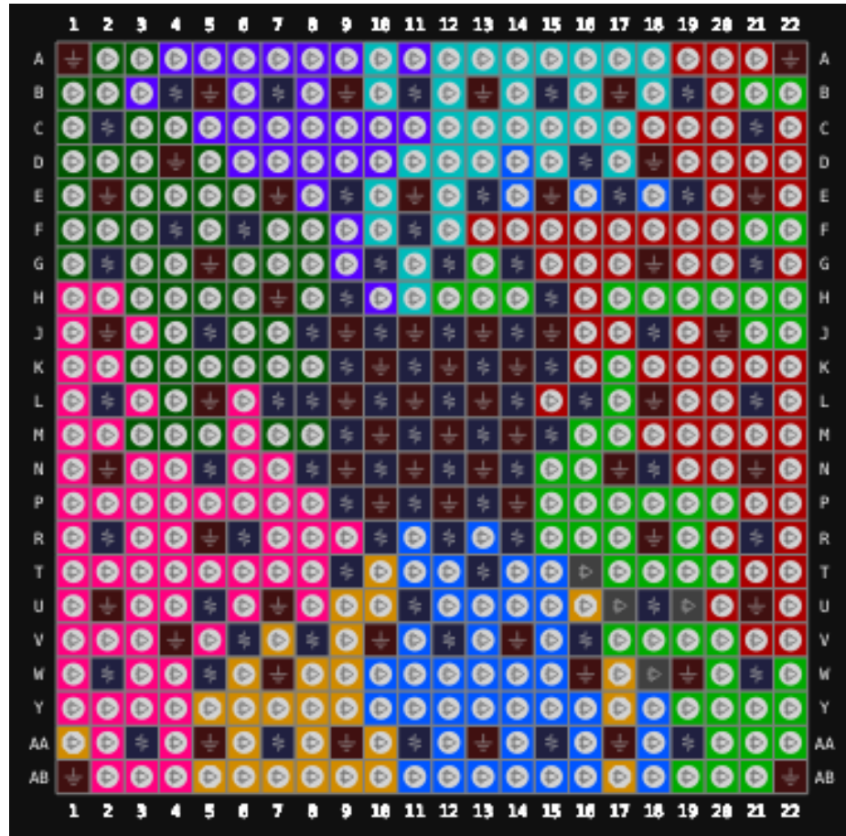
图 3-20 GW2A-55 器件 UG484S 封装管脚分布示意图
