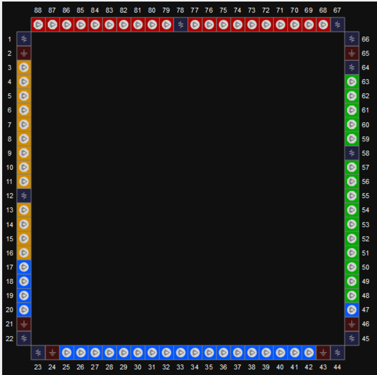
图 3-4 GW1NR-9 器件 QN88 封装管脚分布示意图（顶视图，内嵌 SDRAM）
