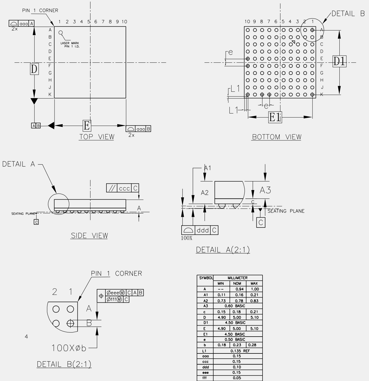
图 4-4 封装尺寸 MG100
