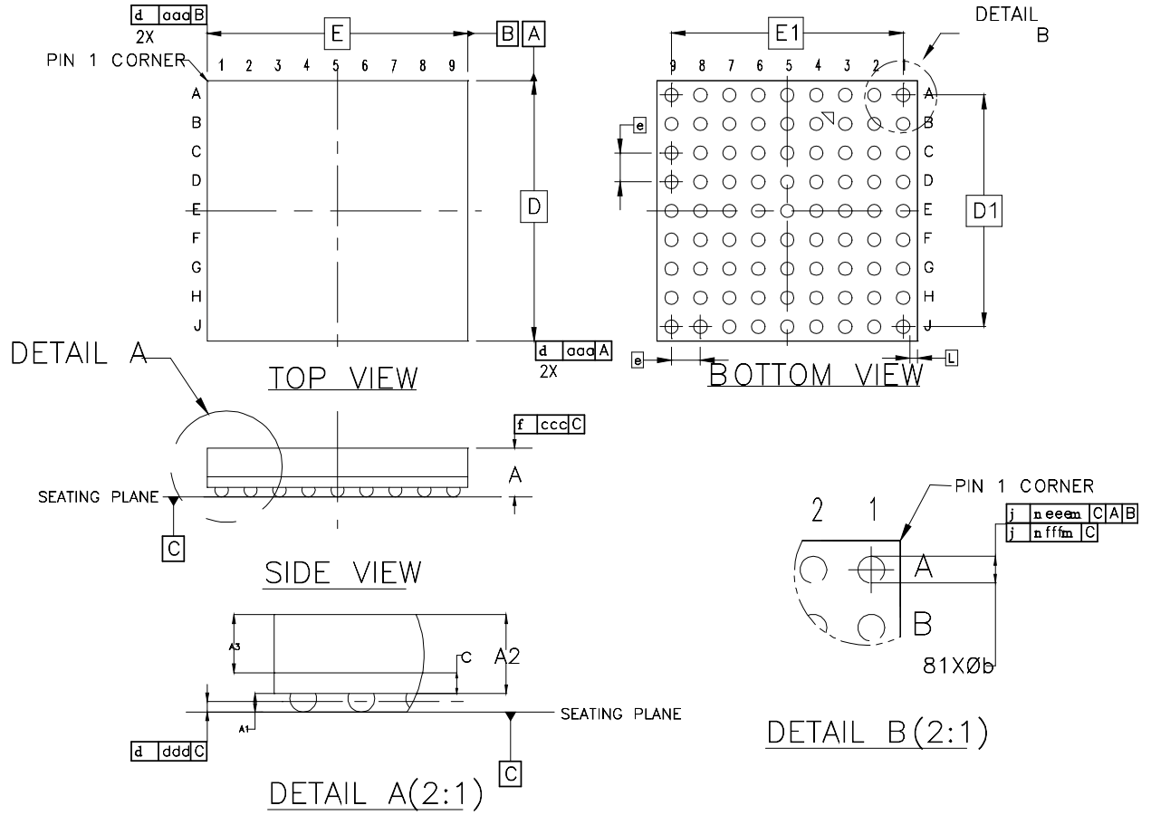
图 4-3 封装尺寸 MG81
