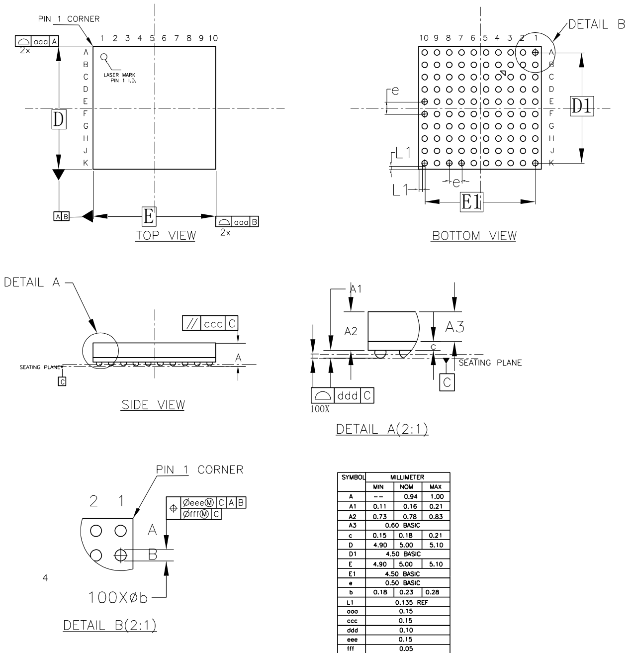
图 4-4 封装尺寸 MG100P/MG100PF/MG100PD
