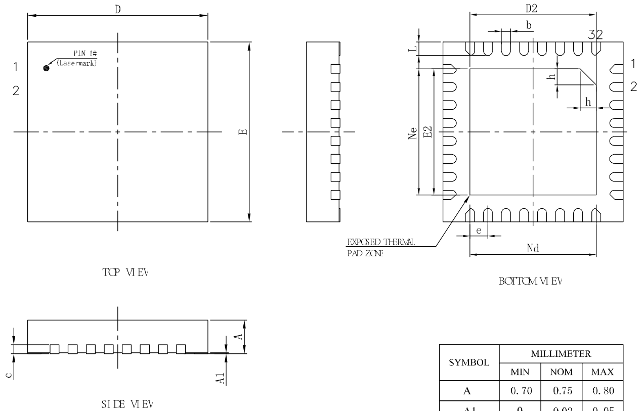
图 4-6 封装尺寸 FN32G
