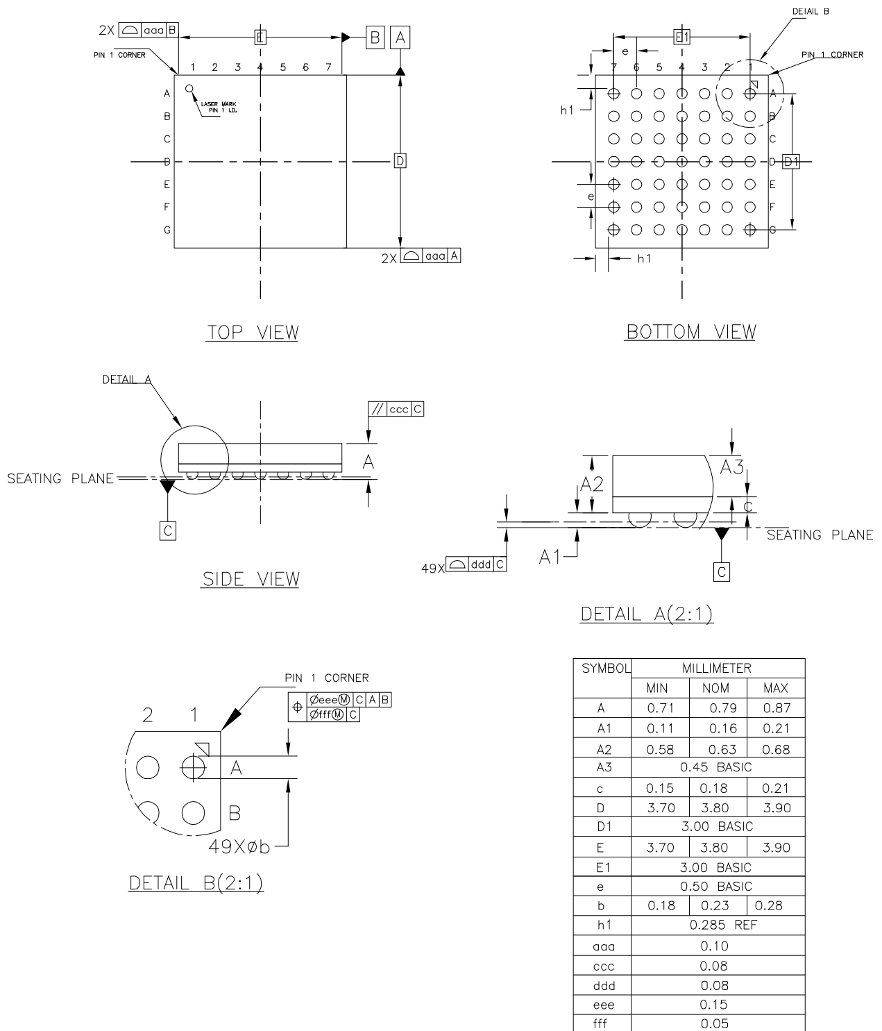
图 4-3 封装尺寸 MG49P/ MG49PG/MG49G
