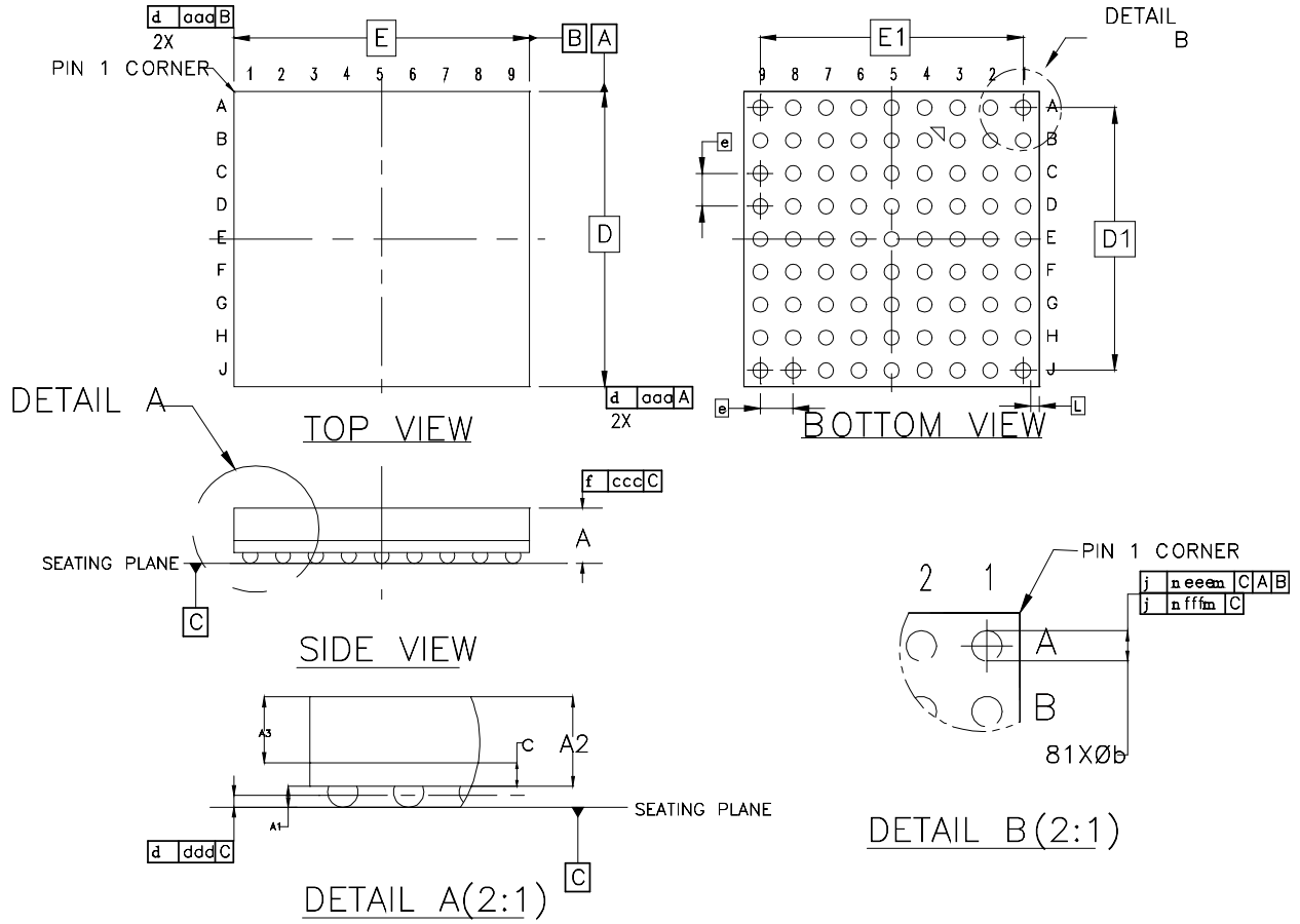
图 4-4 封装尺寸 MG81P
