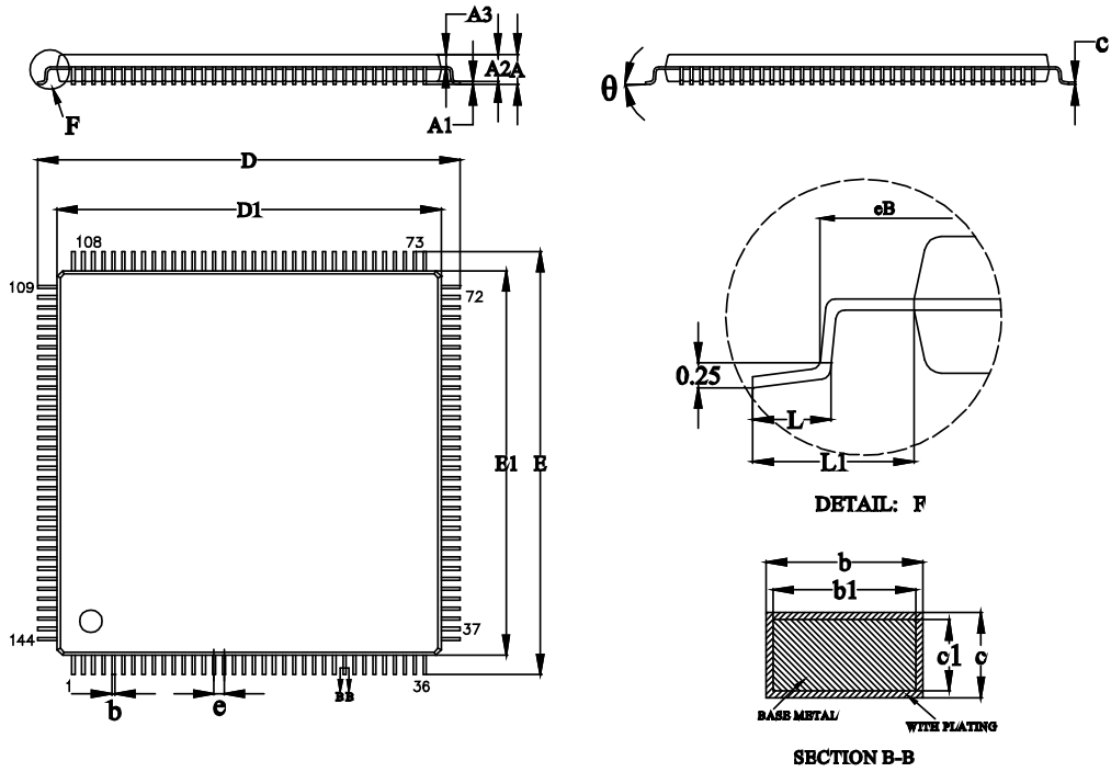
图 4-3 封装尺寸 LQ144/LQ144P
