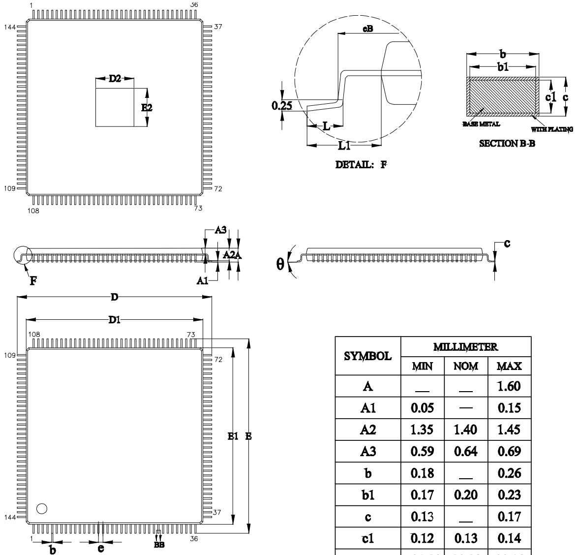
图 4-4 封装尺寸 EQ144G
