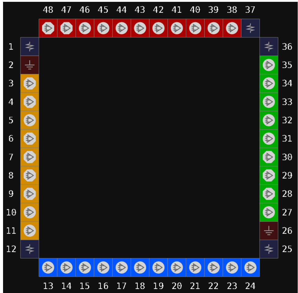
图 3-3 GW1NR-1 器件 QN48G 封装管脚分布示意图（顶视图）
