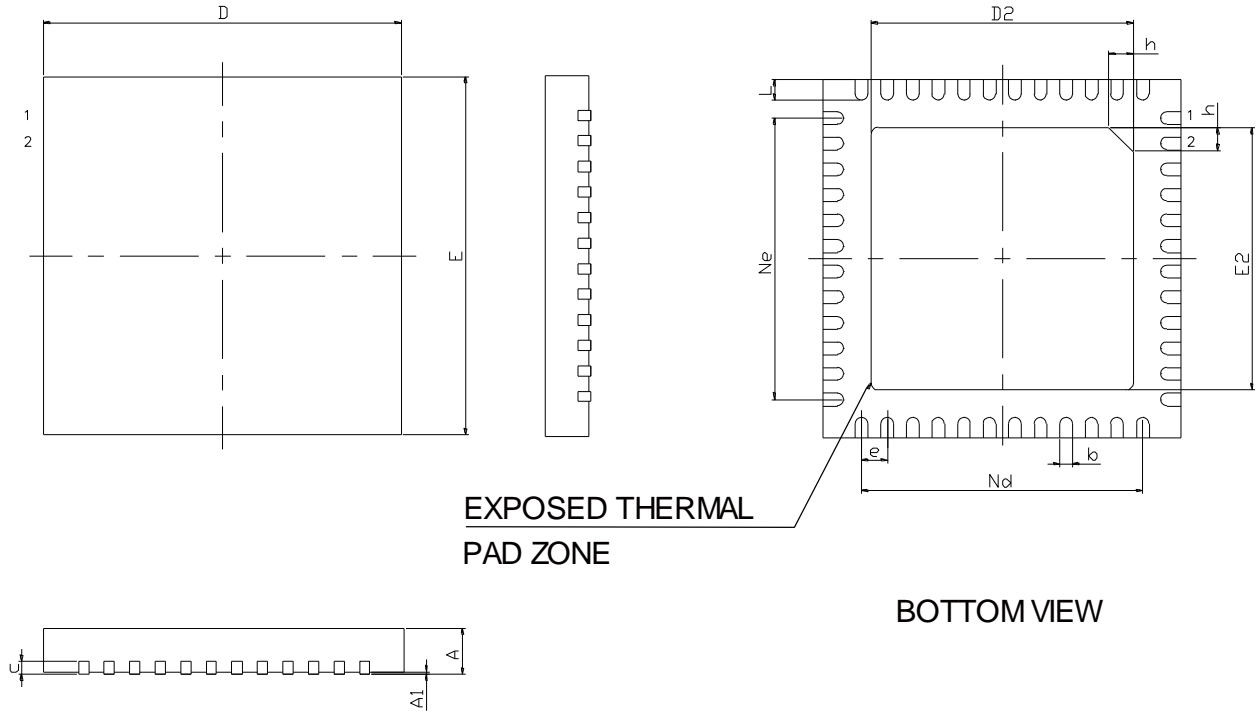
图 4-2 封装尺寸 Q48G
