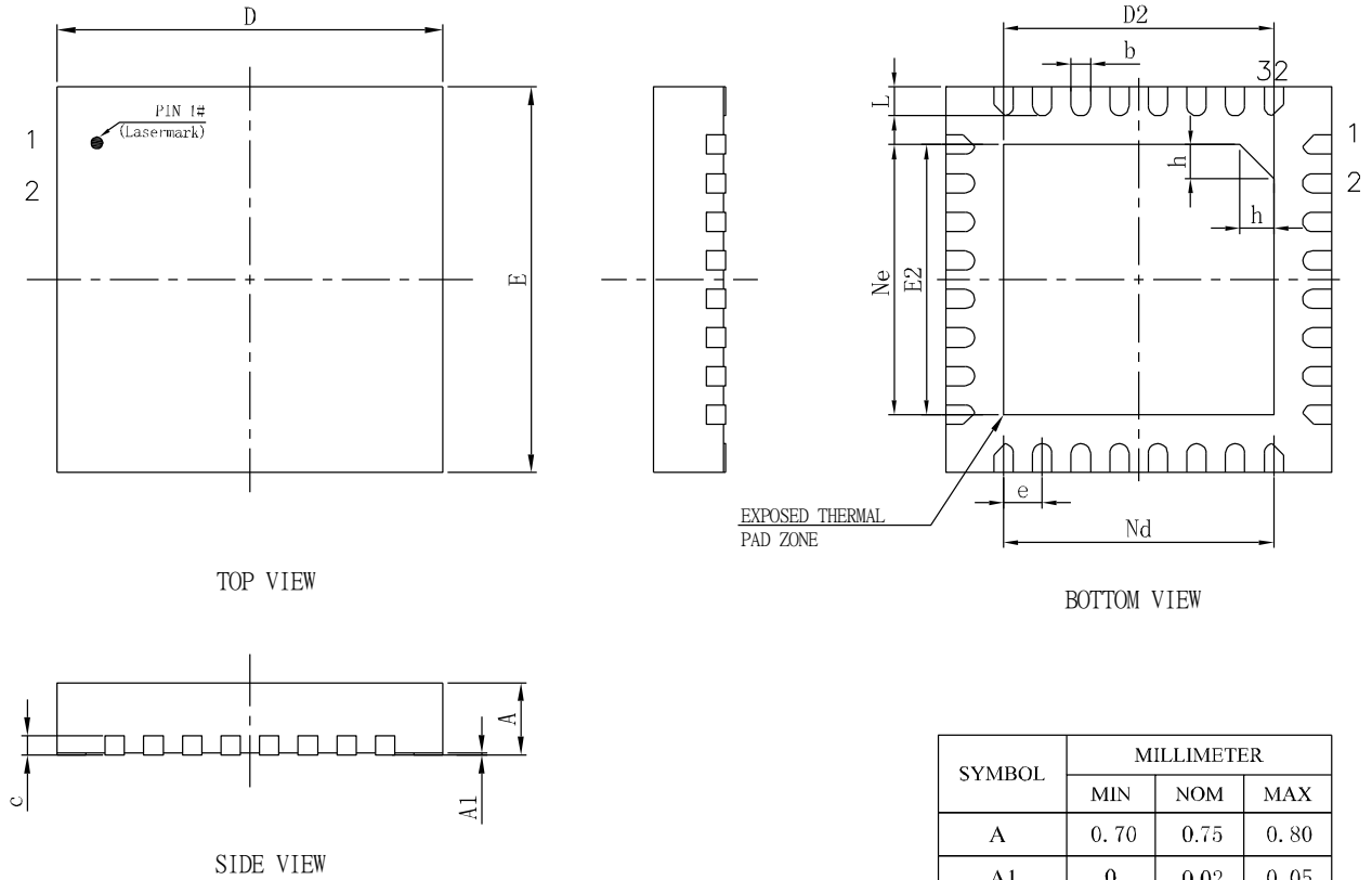
图 4-8 封装尺寸 FN32G
