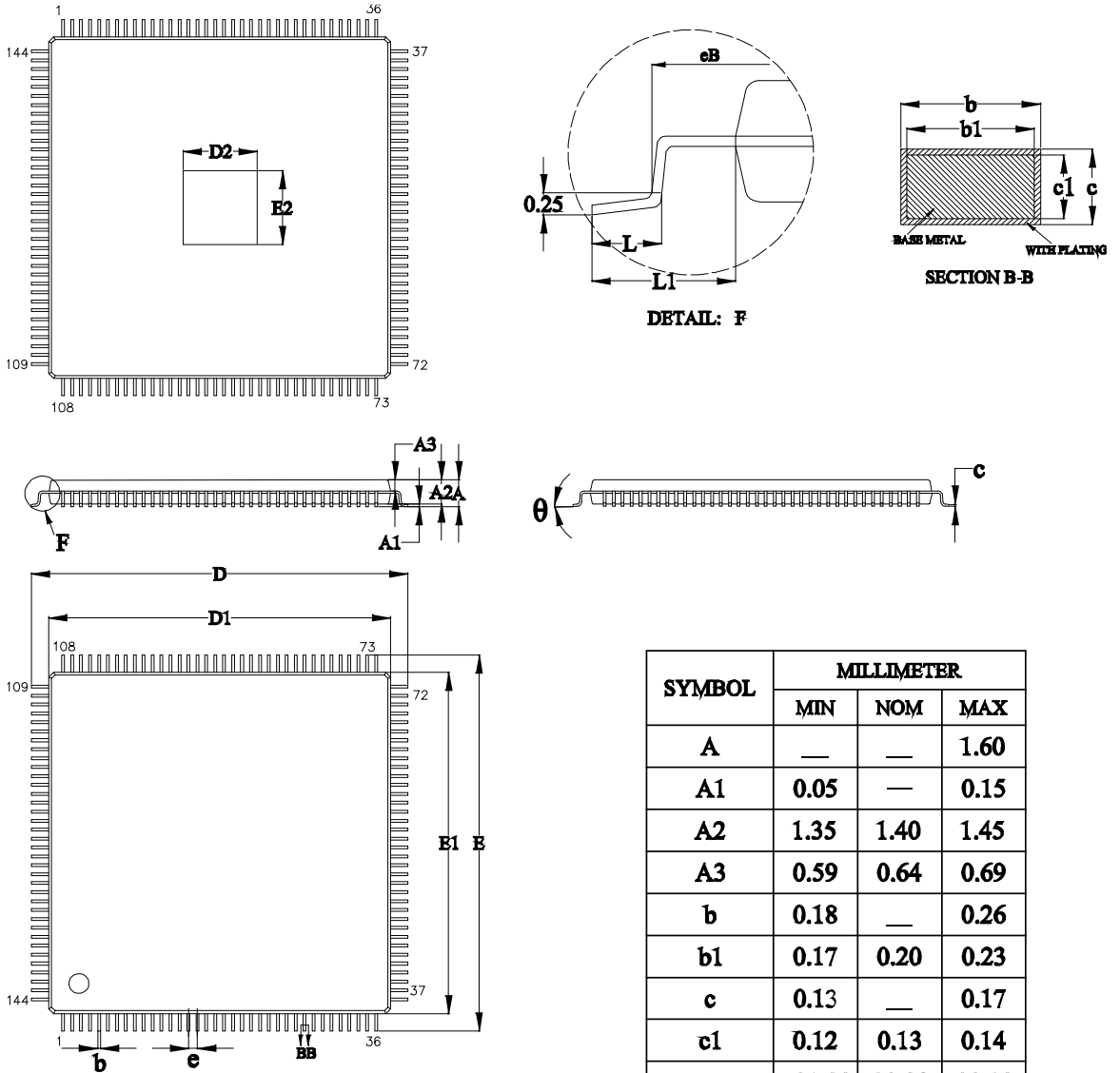
图 4-6 封装尺寸 EQ144G
