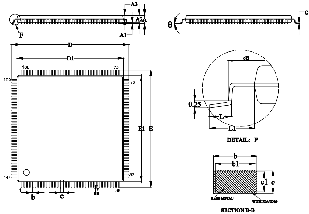
图 4-5 封装尺寸 LQ144/LQ144P
