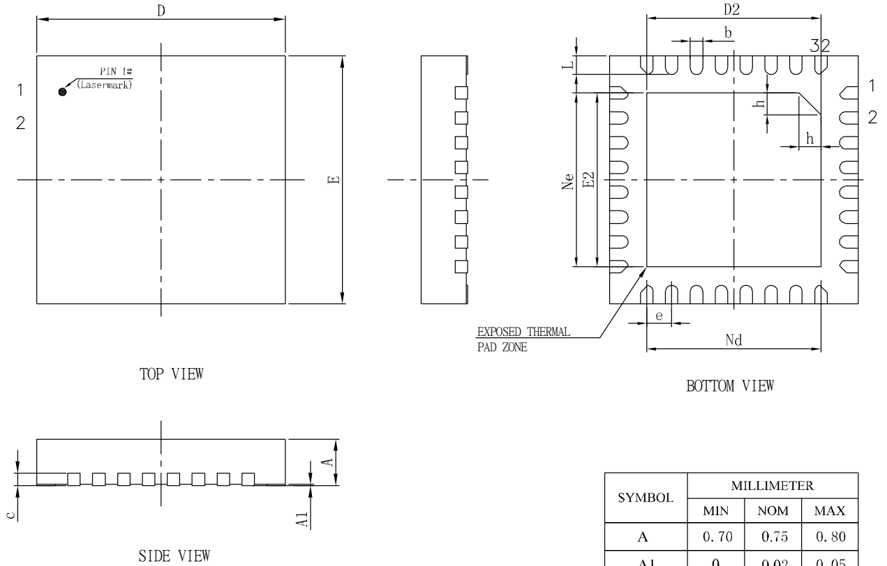
图 4-10 封装尺寸 FN32G
