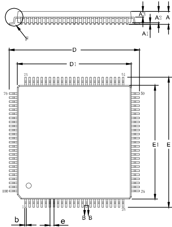
图 4-4 封装尺寸 LQ100G
