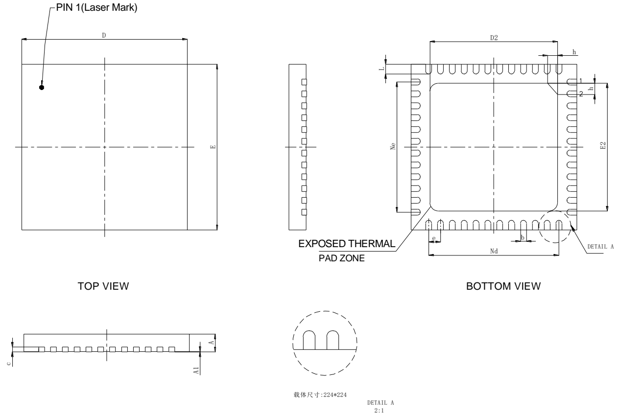
图 4-3 封装尺寸 Q48X
