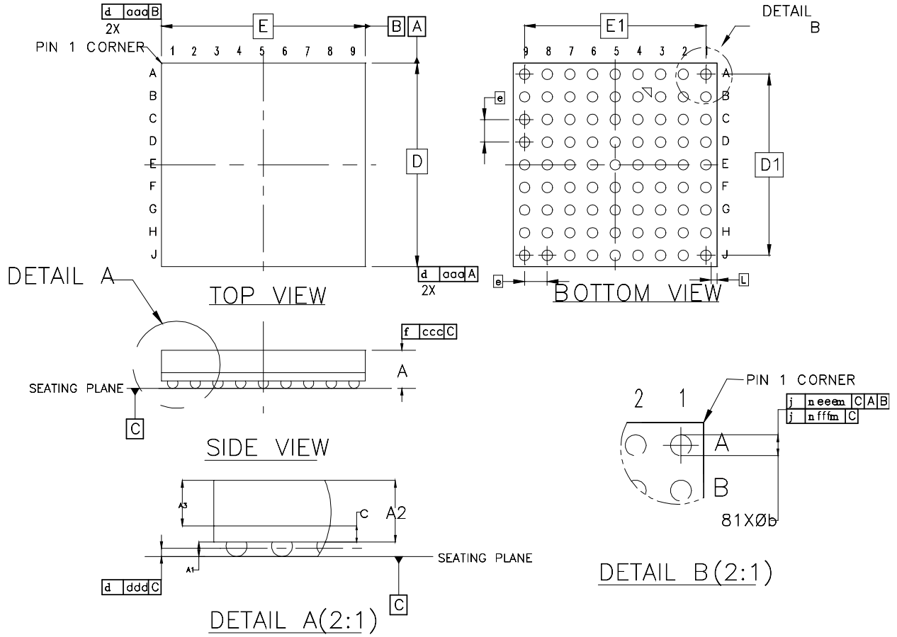
图 4-8 封装尺寸 MG81P
