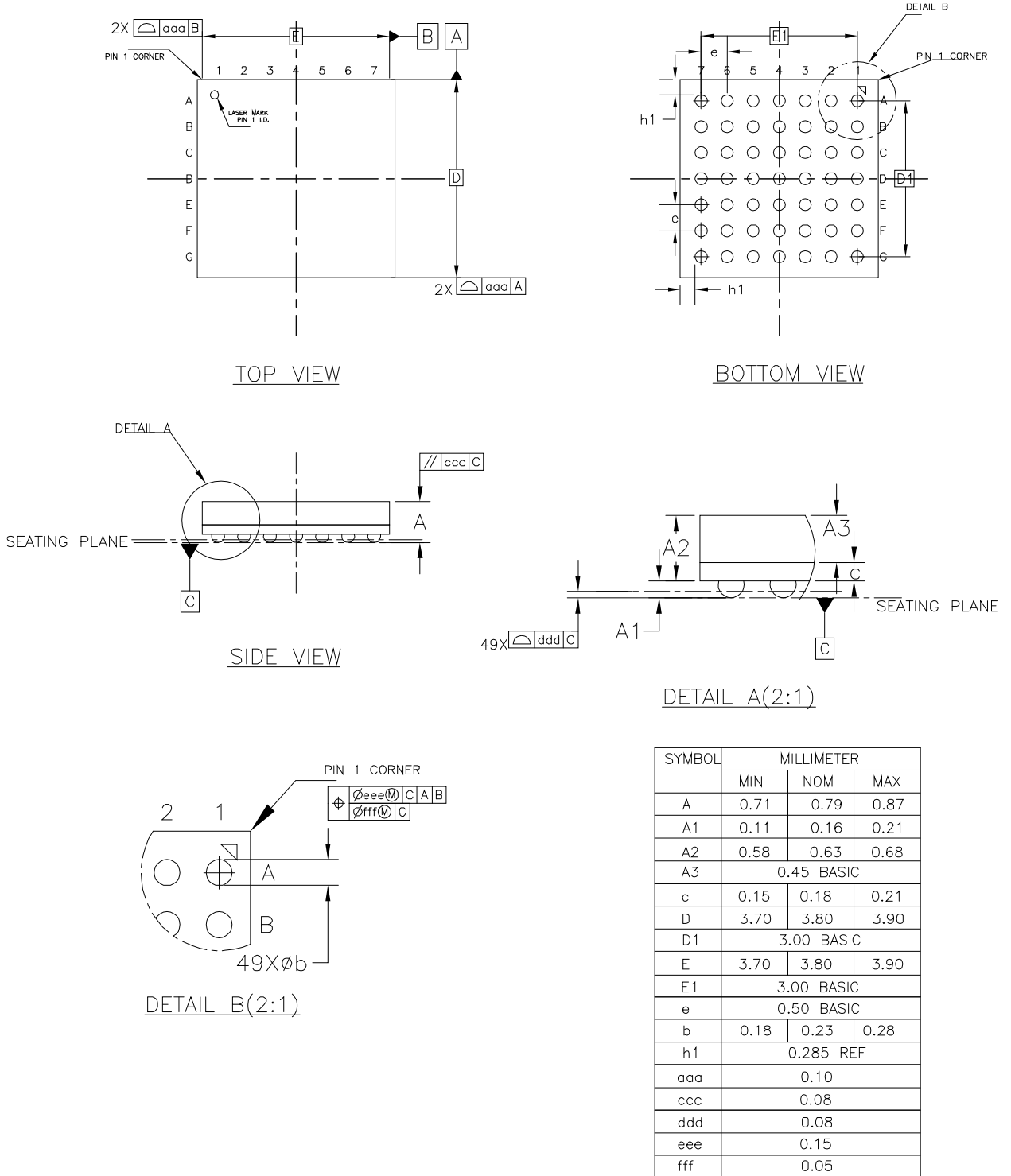
图 4-7 封装尺寸 MG49P/ MG49PG/MG49G
