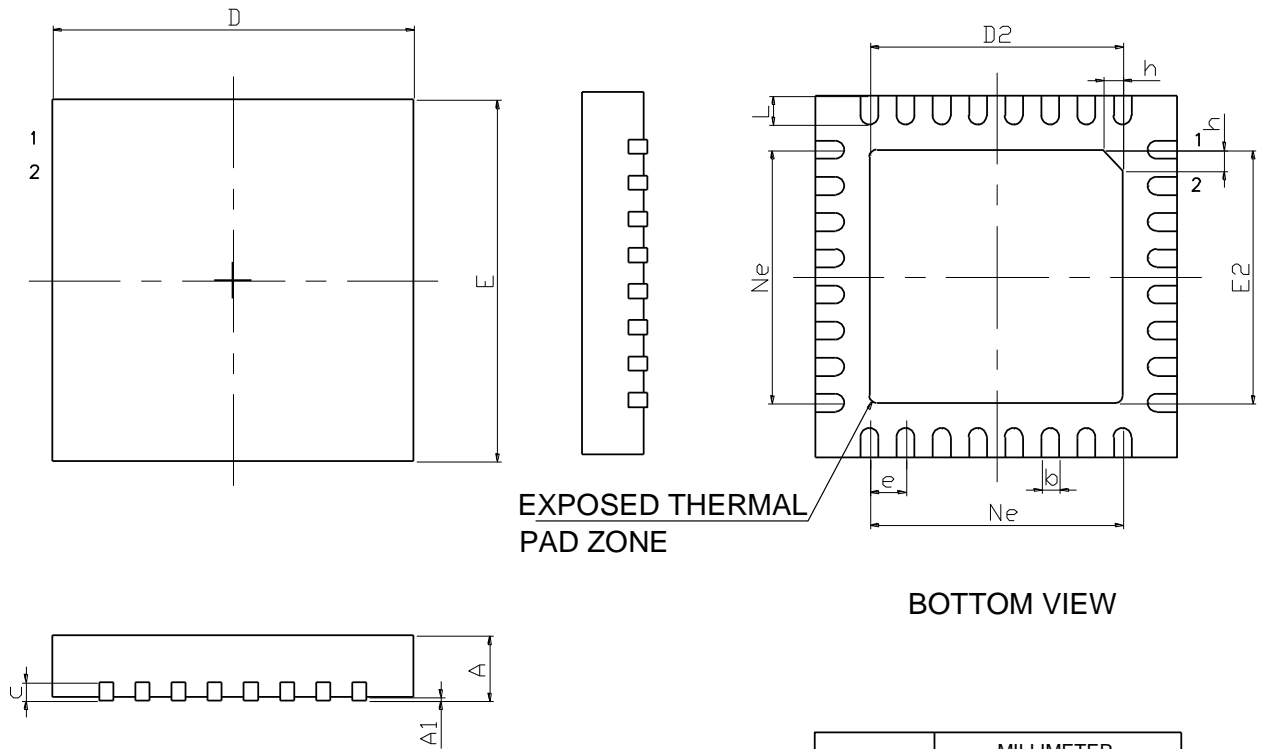
图 4-2 封装尺寸 Q32X
