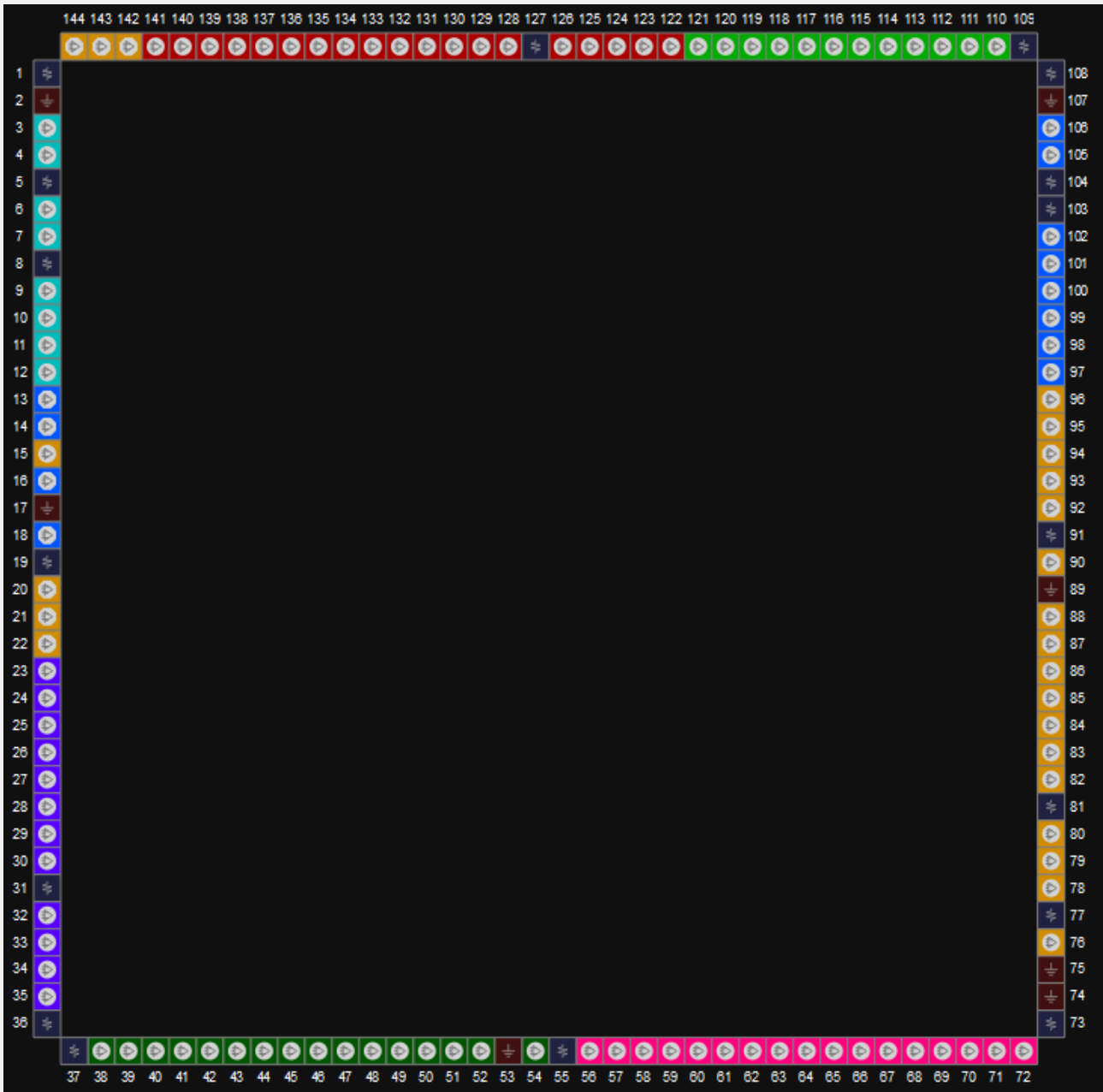
图 3-3 GW2AR-18 器件 LQ144/EQ144 封装管脚分布示意图(内嵌 SDRAM)
