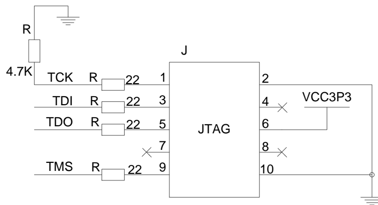
图 2 JTAG 电路参考
