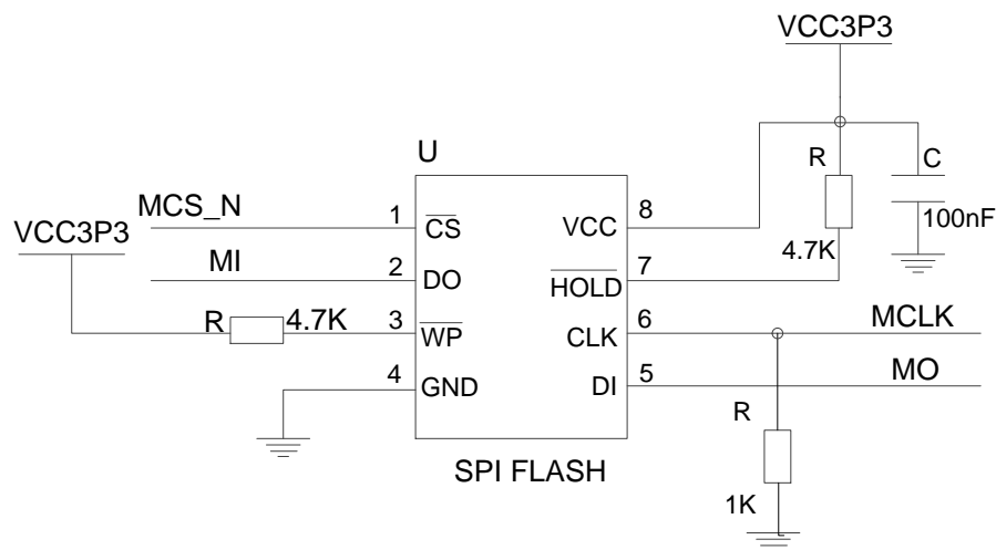
图 3 MSPI 电路参考
