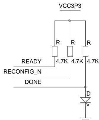
图 4 READY、RECONFIG_N、DONE 参考电路
