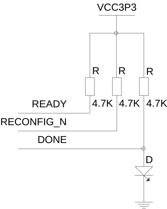
图 5 READY 、 RECONFIG_N 、 DONE 参考电路
