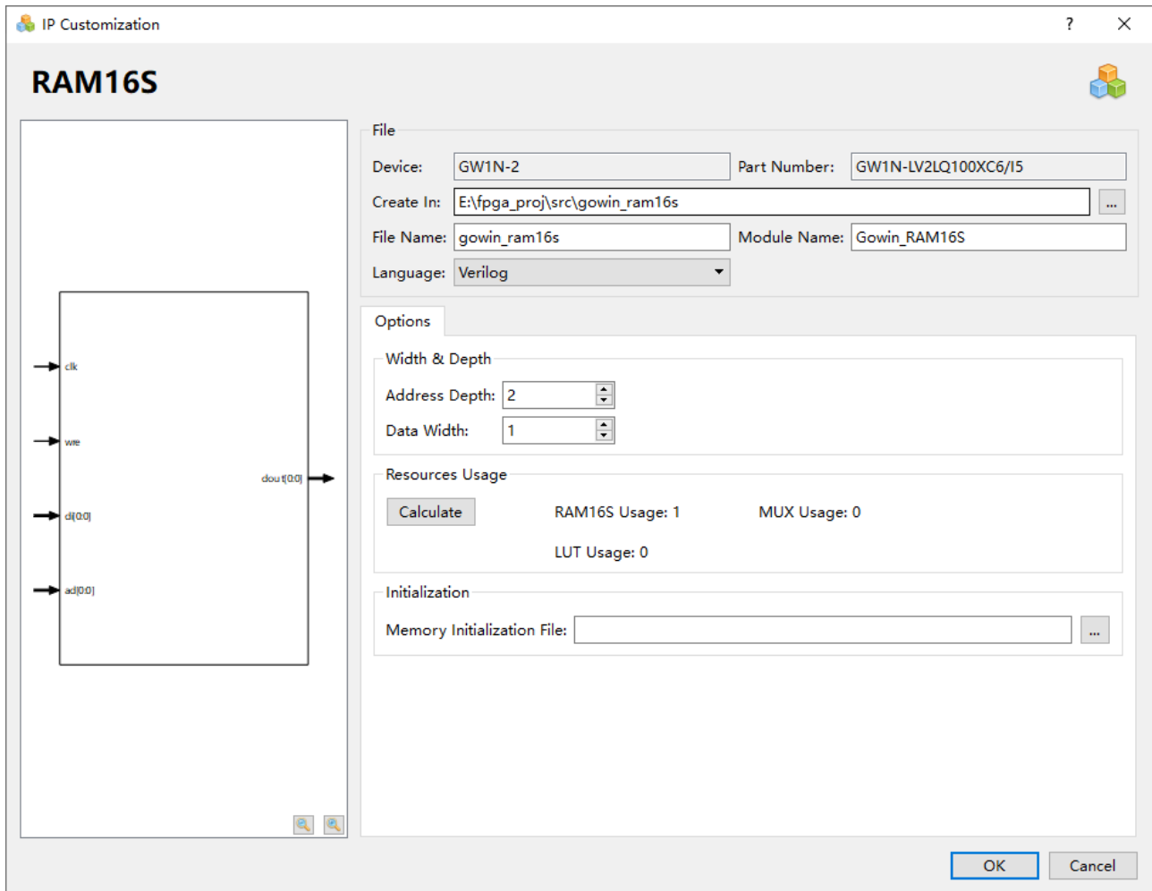
图 6-2 RAM16S 的 IP Customization 窗口结构
