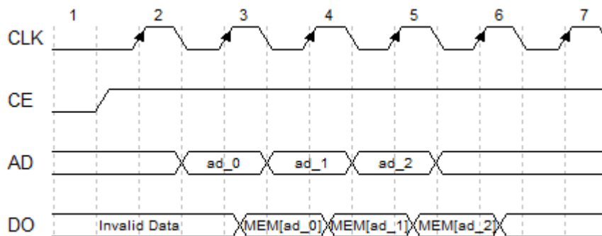
图 3-12ROM 时序波形图（Bypass 模式）
