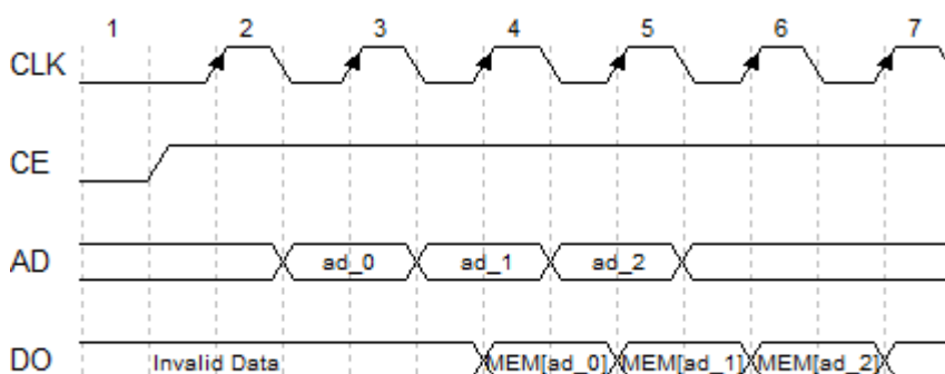
图 3-13ROM 时序波形图（Pipeline 模式）
