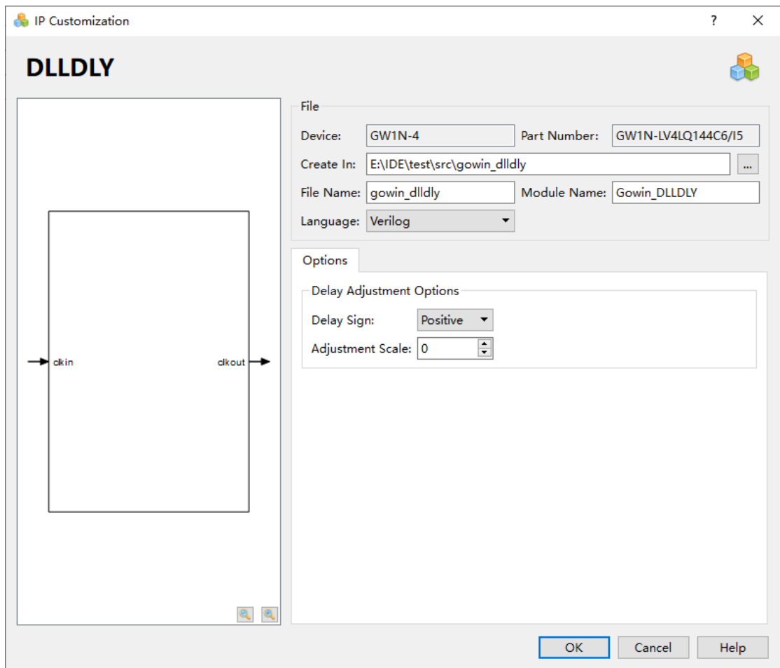
图 5-10 DLLDLY 的 IP Customization 窗口结构
