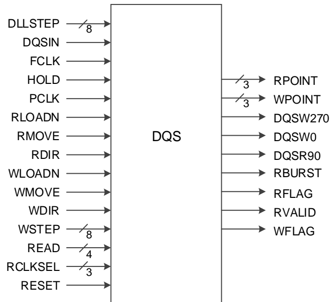
图 5-15 DQS 端口示意图
