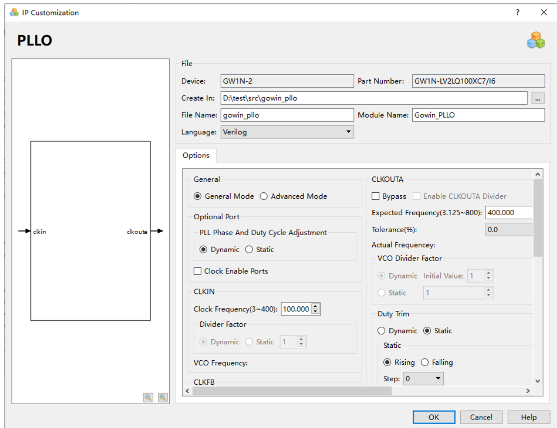
图 5-8 PLL0 的 IP Customization 窗口结构
