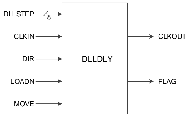
图 5-9 DLLDLY 端口示意图
