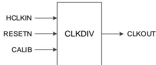
图 5-11 CLKDIV 端口示意图
