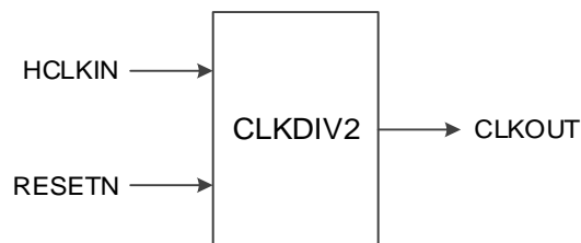
图 4-7 CLKDIV2 端口示意图
