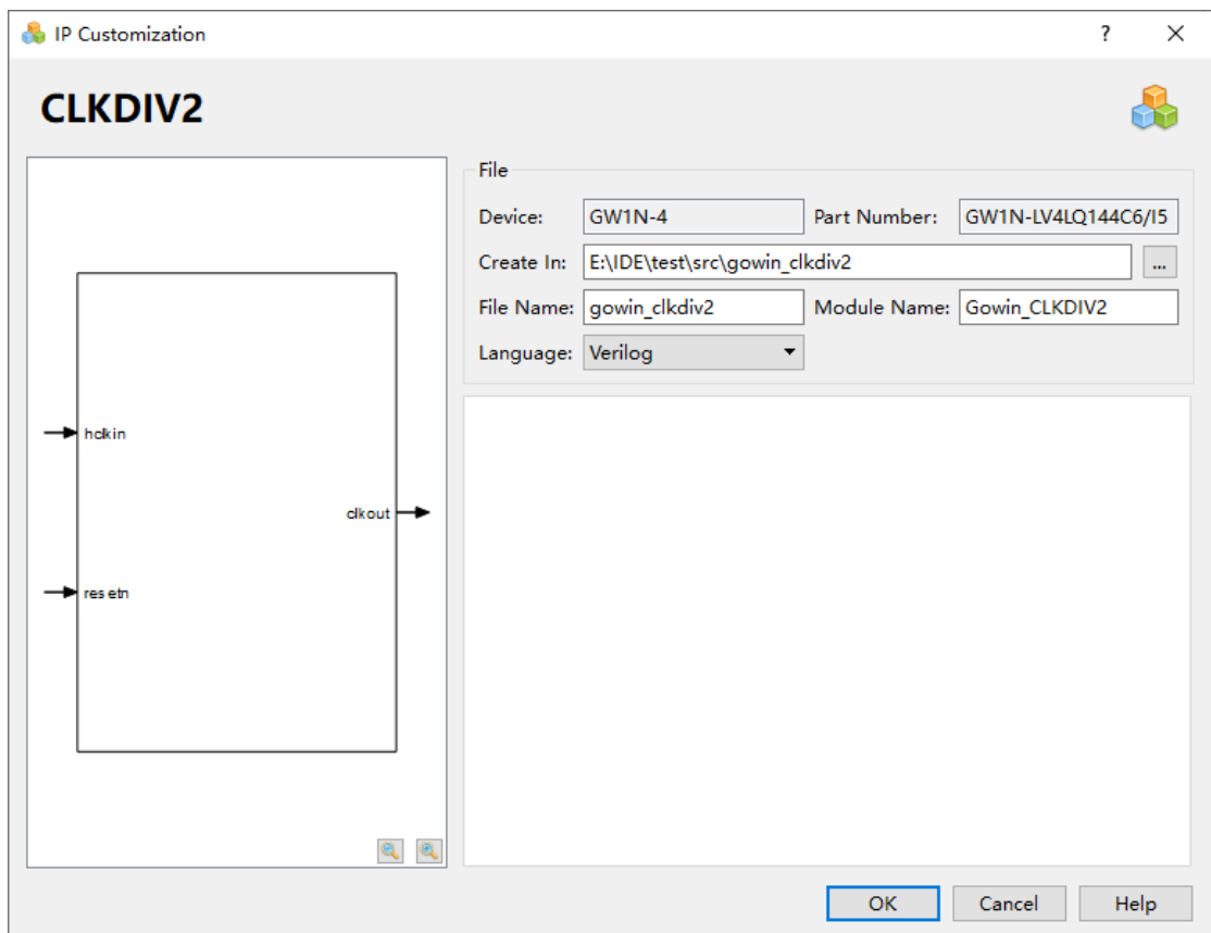
图 4-8 CLKDIV2 的 IP Customization 窗口结构
