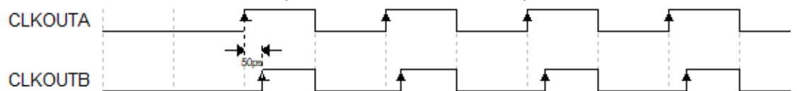
图 5-7 B 通道占空比微调时序图(微调方向为 1'b0, 步长为 1)
