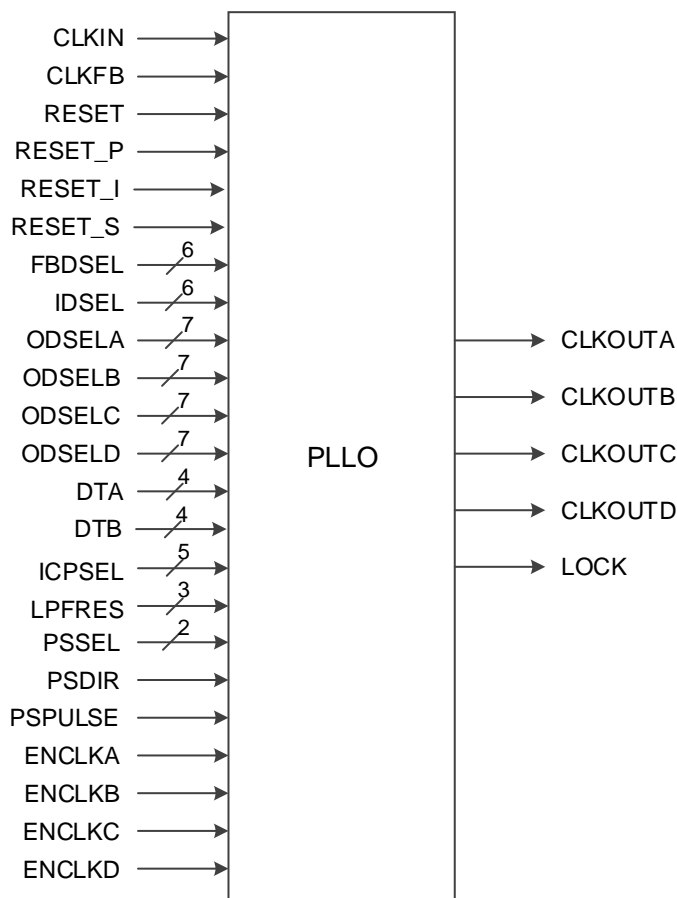
图 5-5 PLLO 端口示意图
