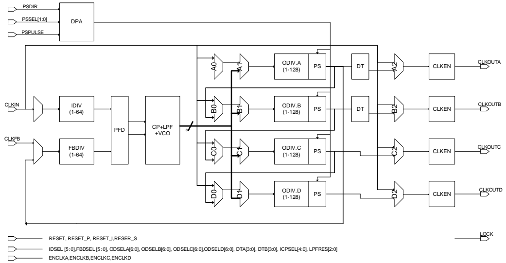
图 2-3 PLL 示意图
