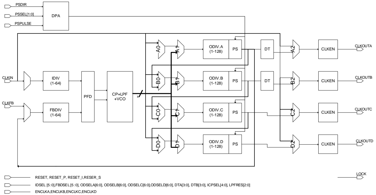
图 2-3 PLL 示意图
