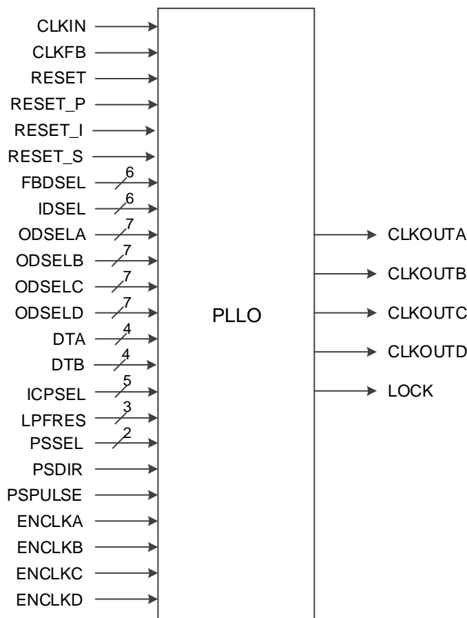
图 5-7 PLL0 端口示意图
