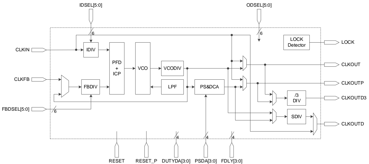
图 2-4 PLL 示意图
