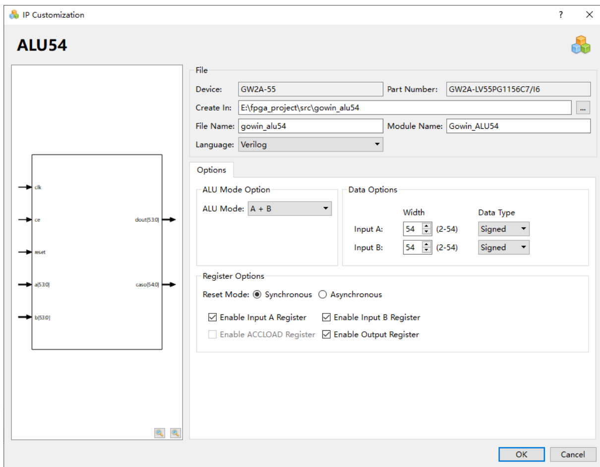
图 5-1 ALU54 的 IP Customization 窗口结构
