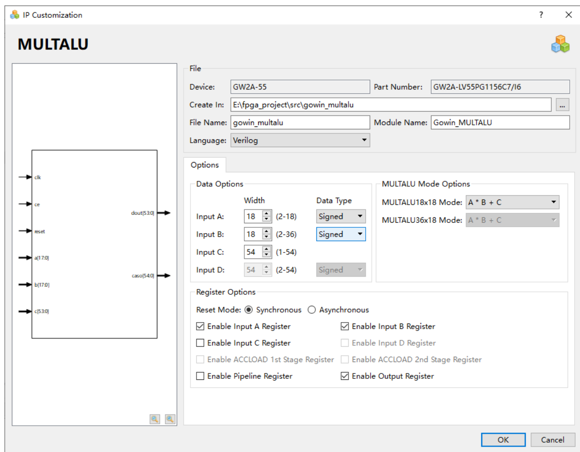
图 5-4 MULTALU 的 IP Customization 窗口结构
