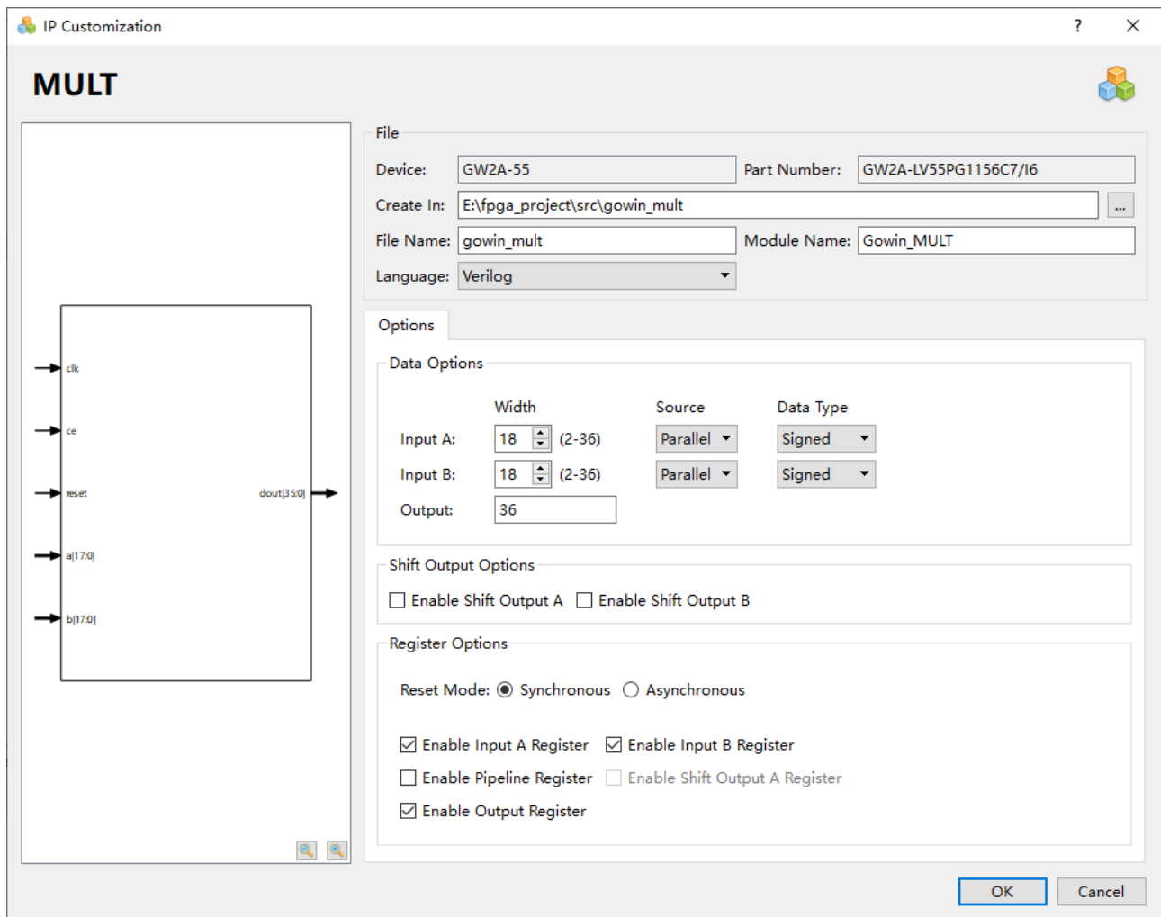
图 5-2 MULT 的 IP Customization 窗口结构
