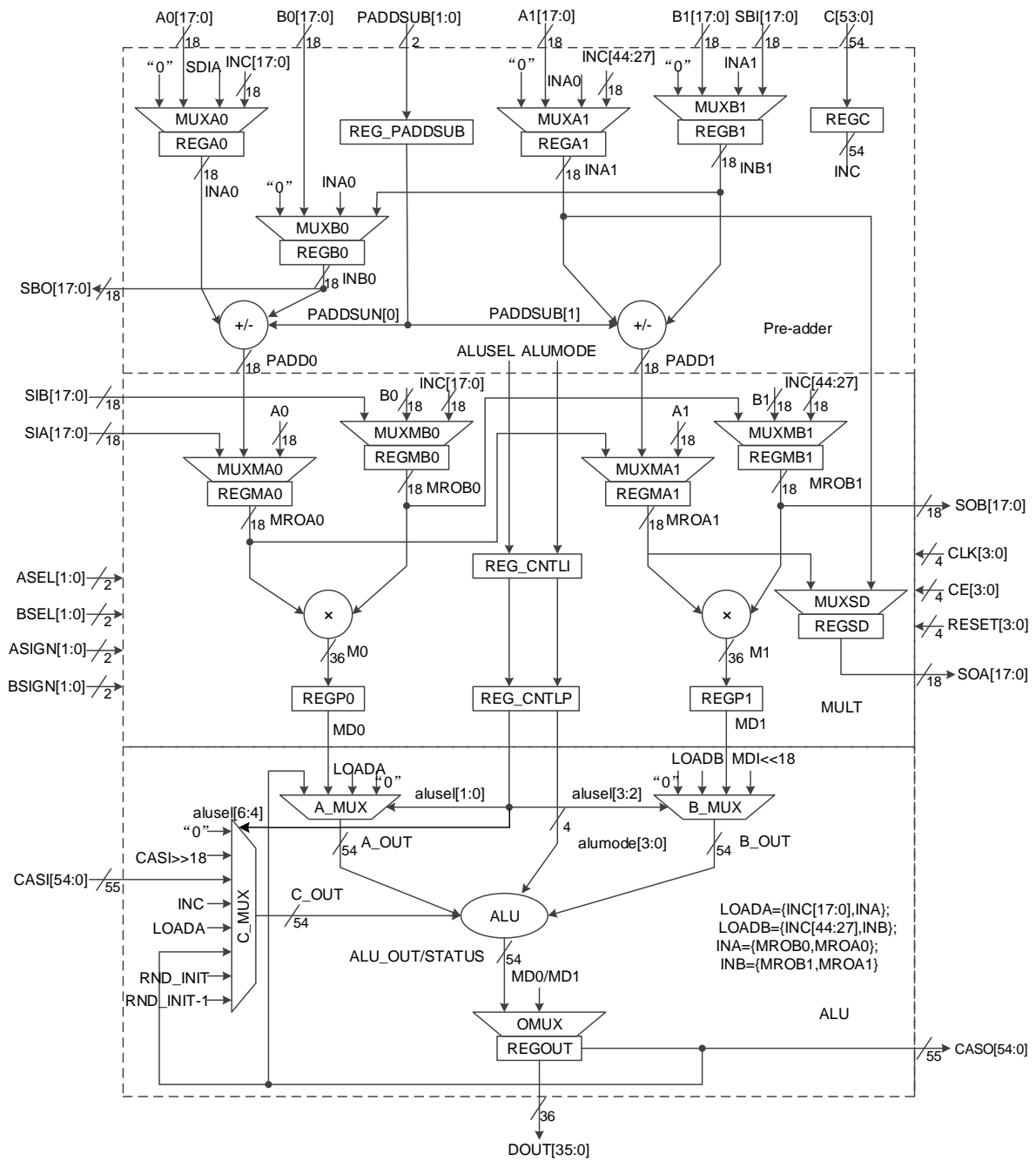
图 3-1 宏单元的组成结构
