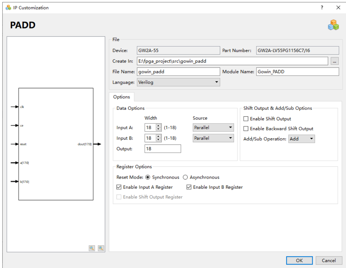
图 5-5 PADD 的 IP Customization 窗口结构
