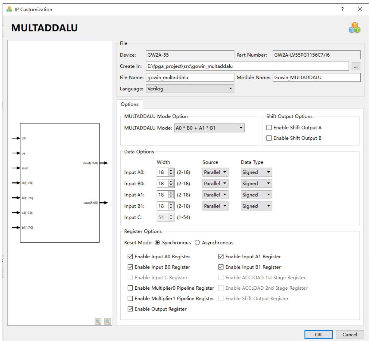
图 5-3 MULTADDALU 的 IP Customization 窗口结构
