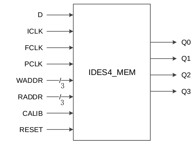
图 4-14 IDES4_MEM 端口示意图
