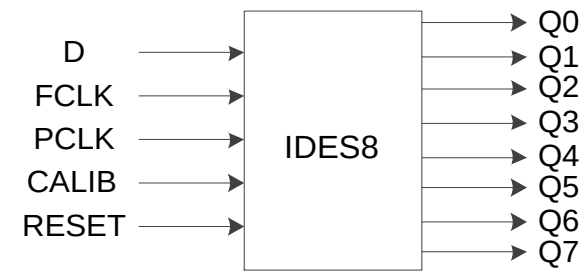
图 4-9 IDES8 端口示意图
