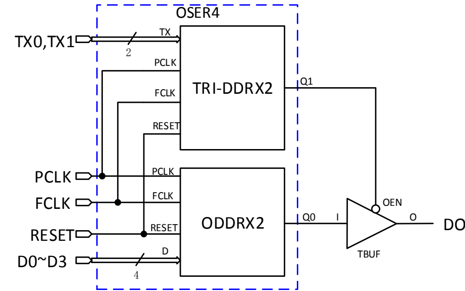
图 4-21 OSER4 逻辑框图
