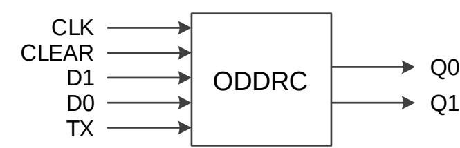
图 4-20 ODDRC 端口示意图
