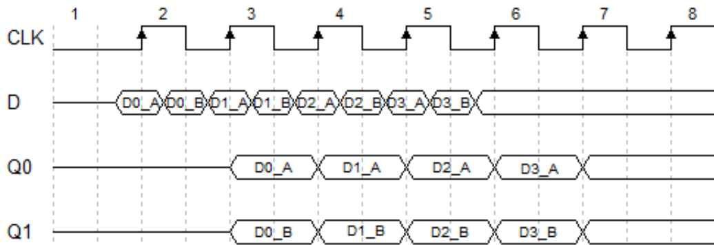
图 4-4 IDDR 时序图
