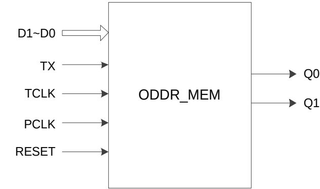
图 4-29 ODDR_MEM 端口示意图
