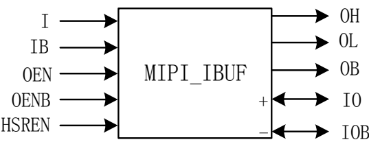
图 3-15 MIPI_IBUF 端口示意图
