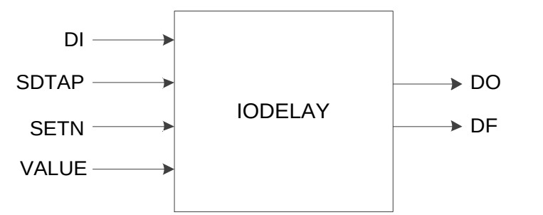
图 4-34 IODELAY 端口示意图
