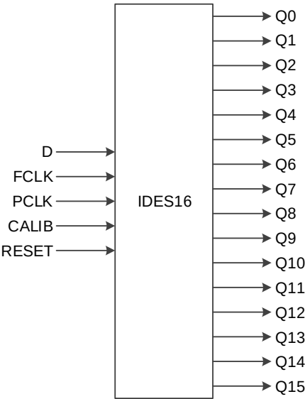
图 4-12 IDES16 端口示意图
