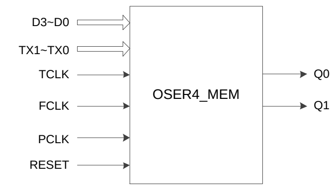
图 4-31 OSER4_MEM 端口示意图
