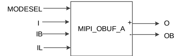
图 3-17 MIPI_OBUF_A 端口示意图
