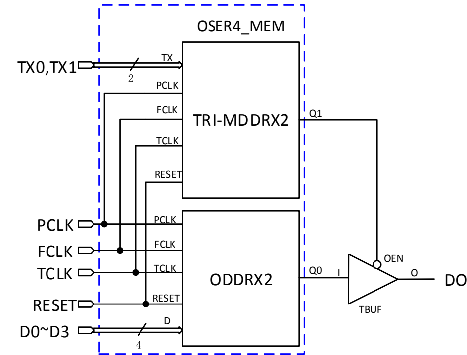
图 4-30 OSER4_MEM 逻辑框图
