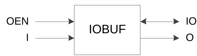
图 3-10 IOBUF 端口示意图
