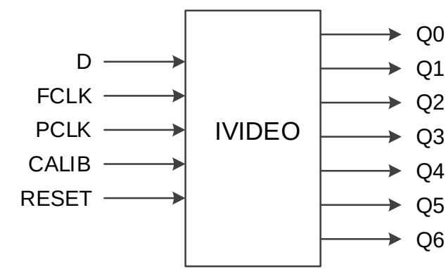
图 4-11 IVIDEO 端口示意图
