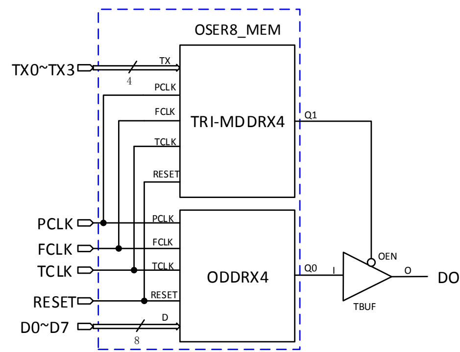
图 4-32 OSER8_MEM 逻辑框图
