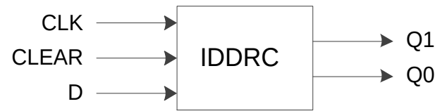
图 4-6 IDDRC 端口示意图
