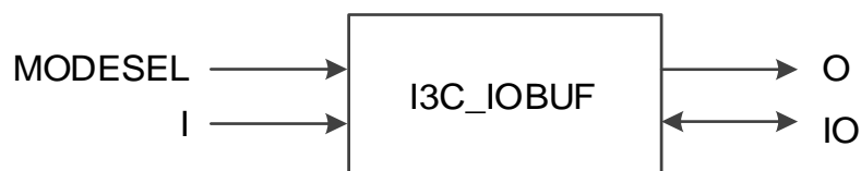
图 3-16 I3C_IOBUF 端口示意图
