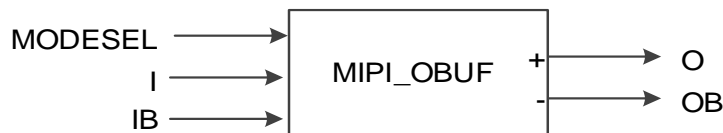
图 3-14 MIPI_OBUF 端口示意图
