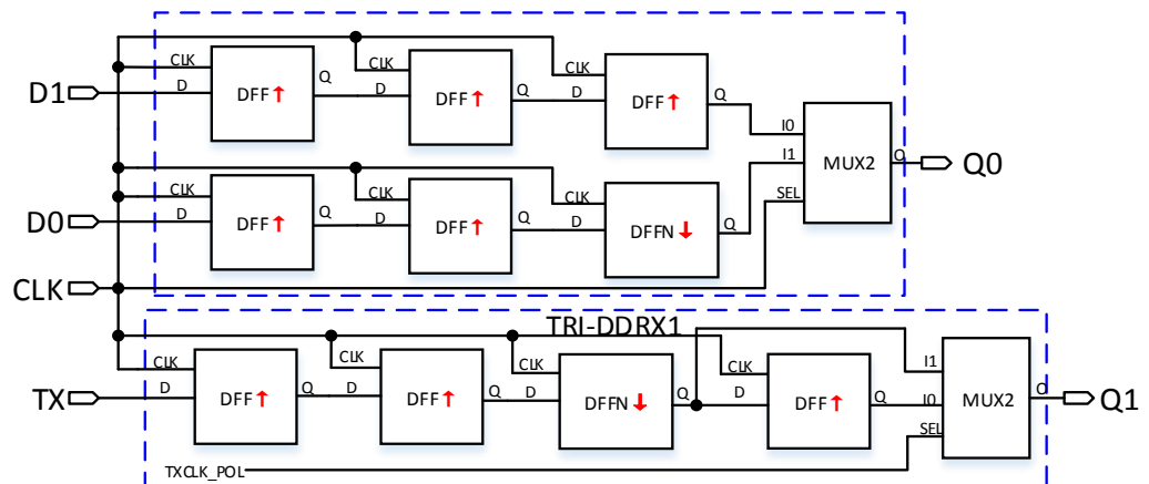
图 4-16 ODDR 逻辑框图
