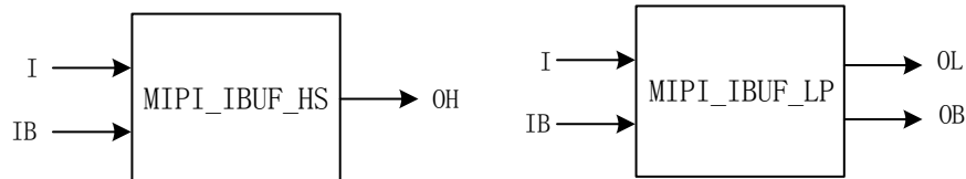
图 3-17 MIPI_IBUF_HS/MIPI_IBUF_LP 端口示意图
