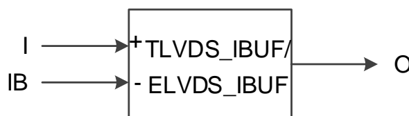
图 3-9 TLVDS_IBUF/ELVDS_IBUF 端口示意图
