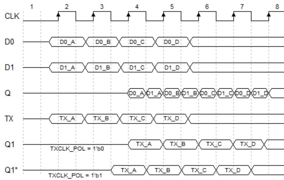
图 4-17 ODDR 时序图
