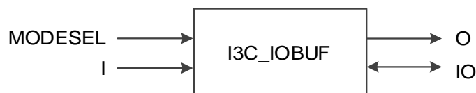
图 3-16 I3C_IOBUF 端口示意图
