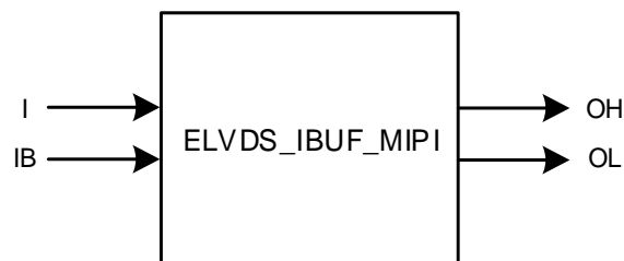
图 3-18 ELVDS_IBUF_MIPI 端口示意图
