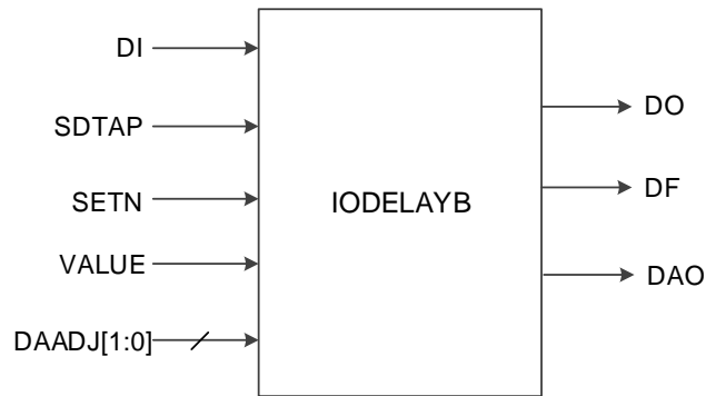
图 4-37 IODELAYB 端口示意图
