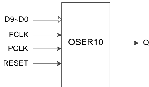
图 4-25 OSER10 端口示意图
