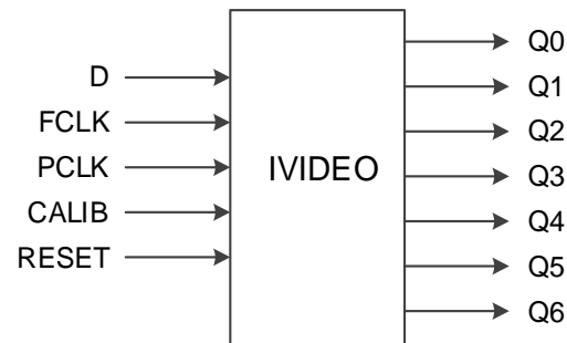
图 4-11 IVIDEO 端口示意图
