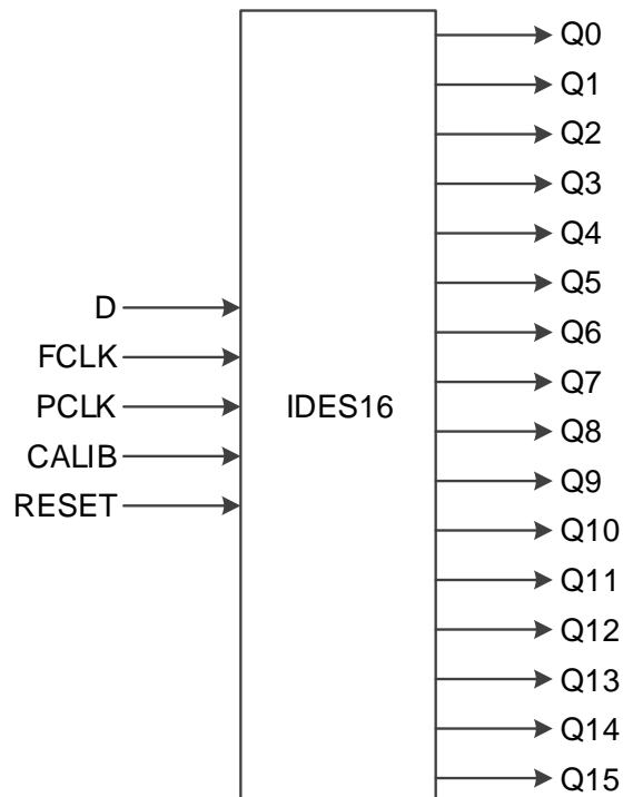
图 4-12 IDES16 端口示意图
