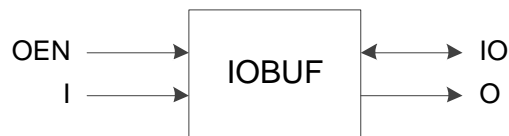
图 3-8 IOBUF 端口示意图
