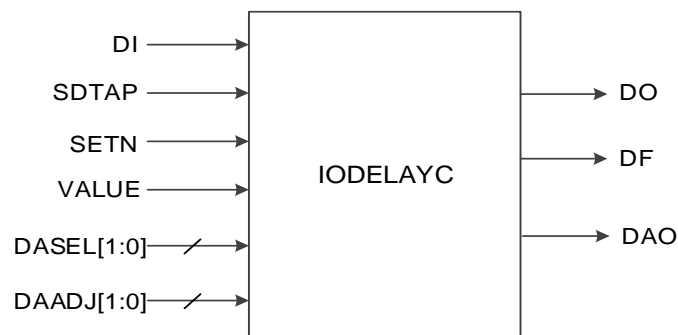
图 4-35 IODELAYC 端口示意图
