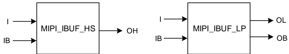
图 3-17 MIPI_IBUF_HS/MIPI_IBUF_LP 端口示意图
