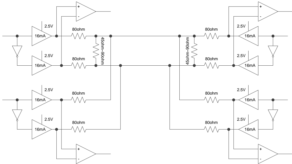
图 3-4 BLVDS 匹配网络
