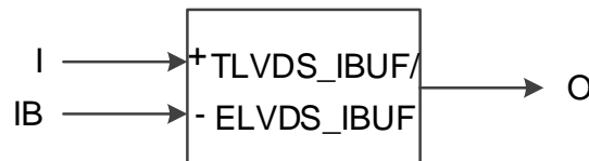
图 3-9 TLVDS_IBUF/ELVDS_IBUF 端口示意图
