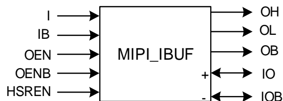
图 3-13 MIPI_IBUF 端口示意图
