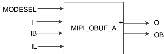
图 3-15 MIPI_OBUF_A 端口示意图
