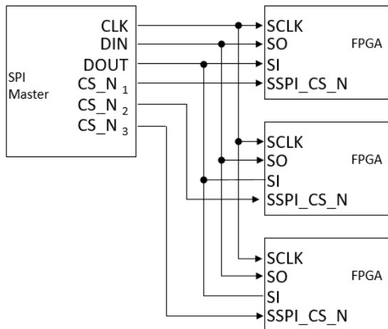
图 5-38 多 FPGA 连线示意图 1
