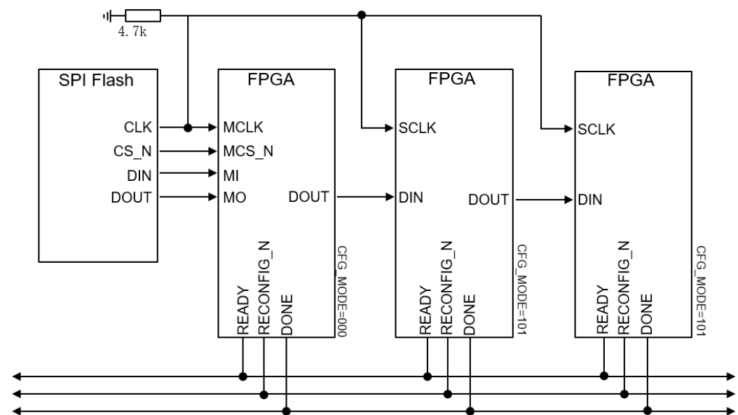
图 5-46 MSPI 模式下的多 FPGA 模式连接示意图
