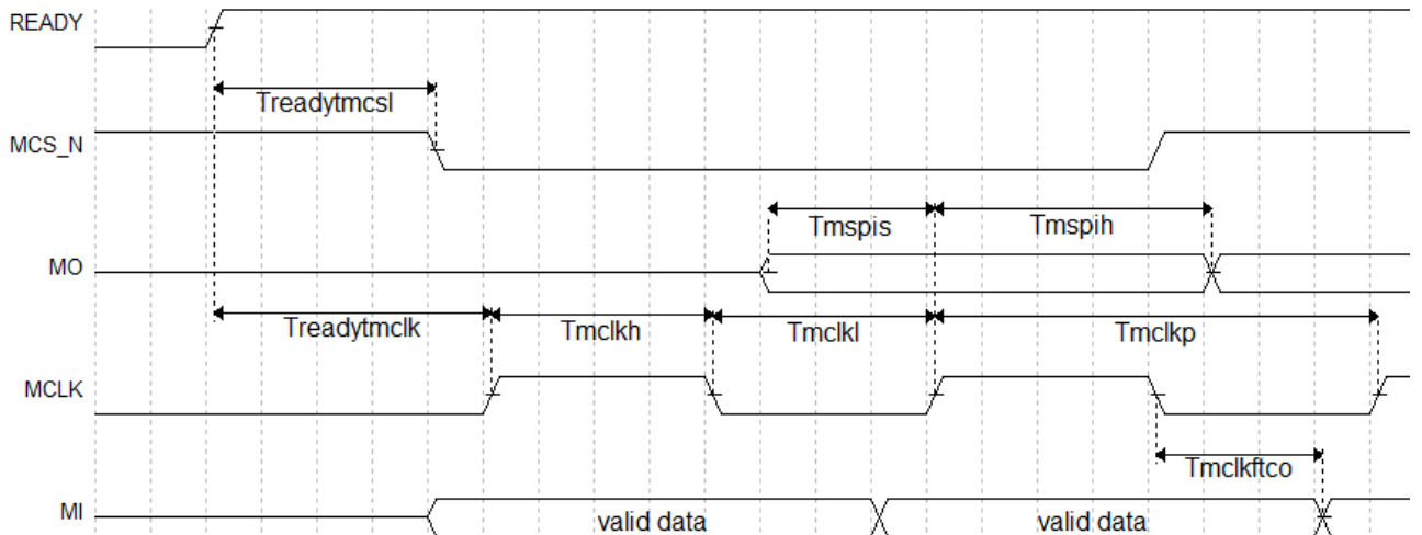
图 5-45 MSPI 下载模式时序图
