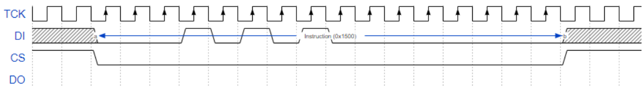
图 5-32 Write Enable (0x15) 时序示意图
