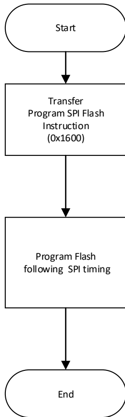
图 5-37 SSPI 配置 Flash 流程图
