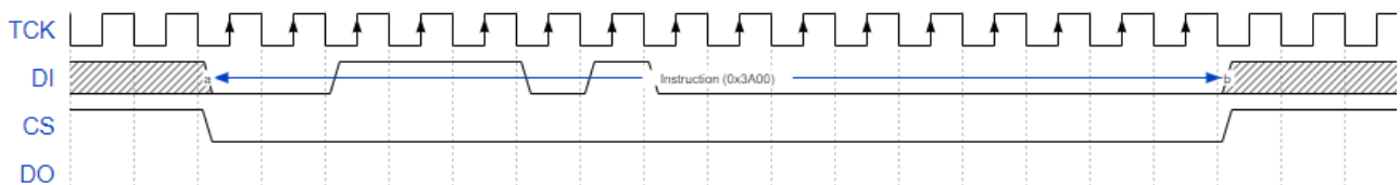
图 5-33 Write Disable (0x3A00) 时序示意图
