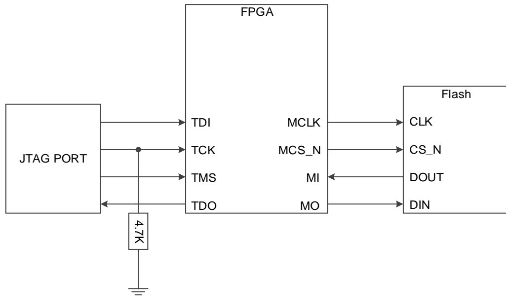
图 5-41 JTAG 接口编程外部 Flash 的连接示意图
