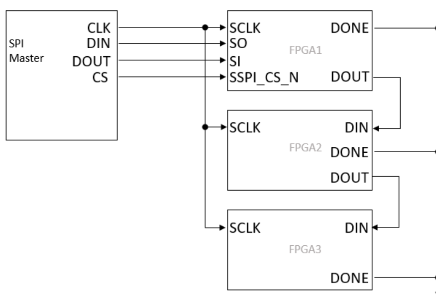
图 5-39 多 FPGA 连线示意图 2
