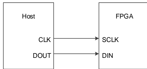
图 5-50 SERIAL 配置模式连接示意图
