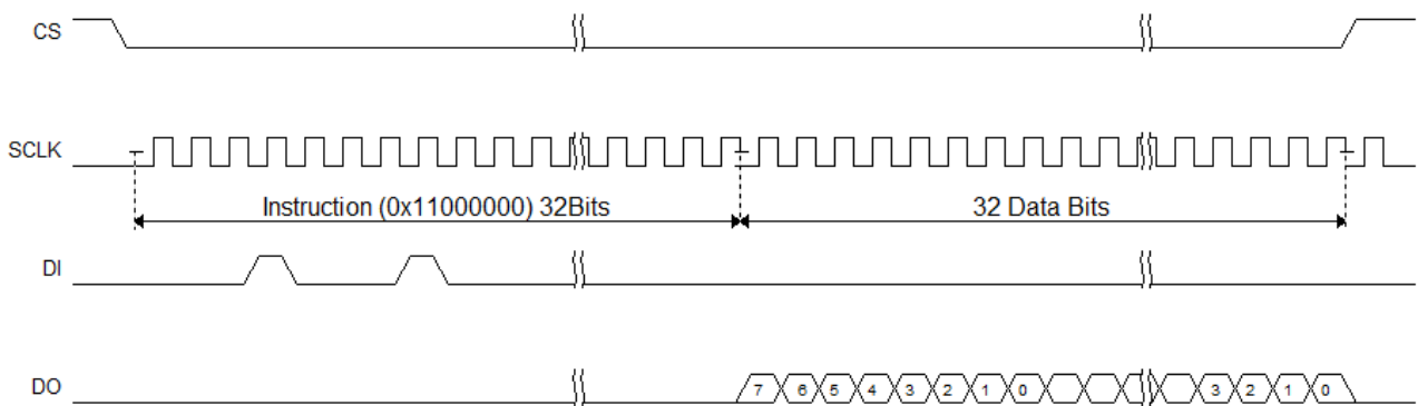
图 5-31 读取 ID Code 时序示意图
