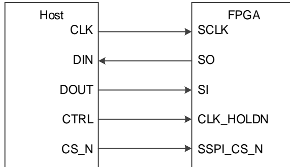
图 5-35 SSPI 配置模式连接示意图
