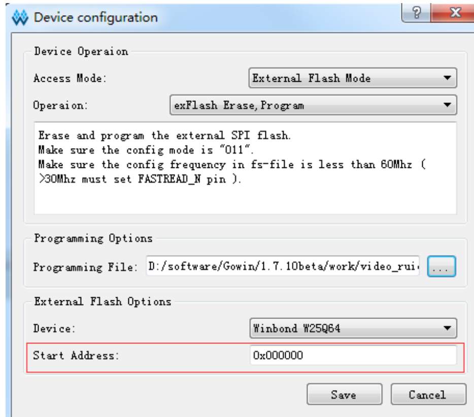
图 5-43 设置外部 Flash 的编程地址
