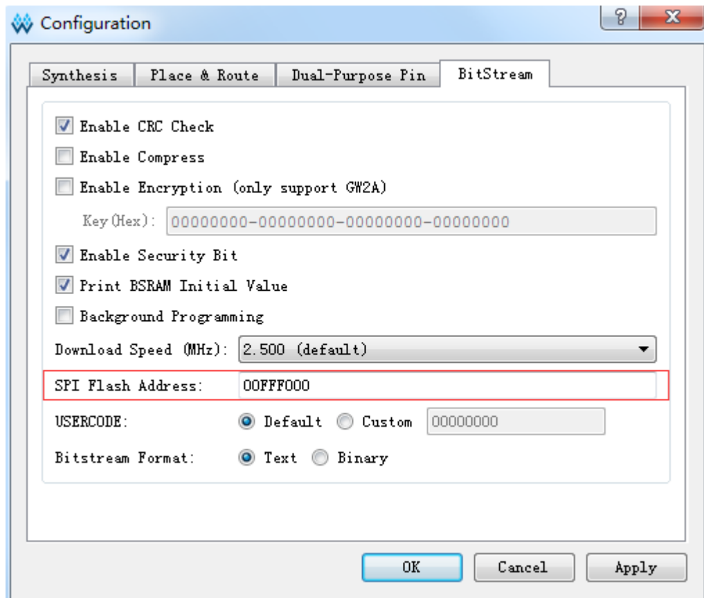
图 5-42 设置下一个 BitStream 的启动地址
