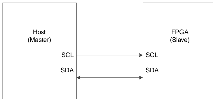
图 5-52 I 2 C 配置模式连接示意图
