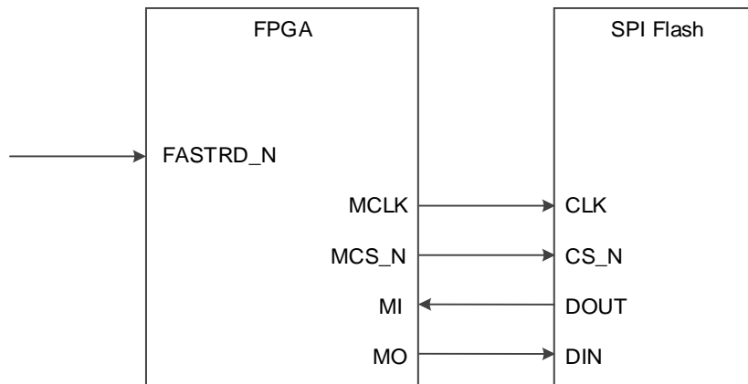
图 5-40 MSPI 配置模式连接示意图
