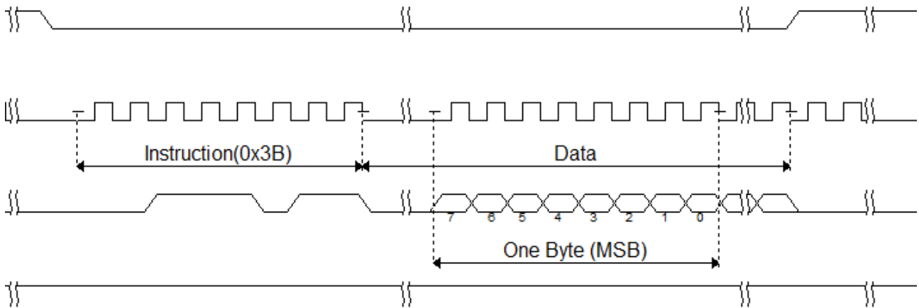
图 5-34 Write Data (0x3B) 时序示意图
