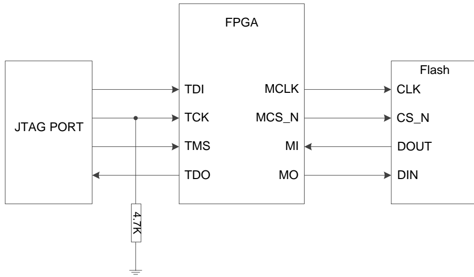
图 5-24 JTAG 接口编程外部 Flash 连接示意图
