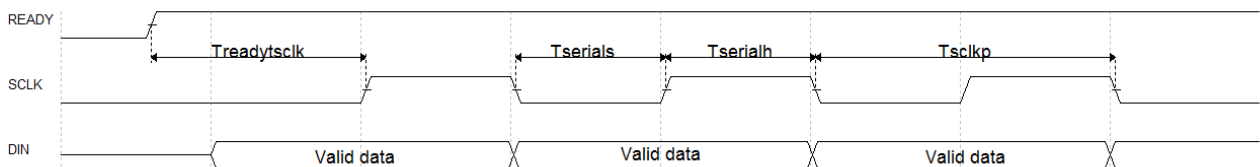
图 5-51 SERIAL 配置模式时序图
