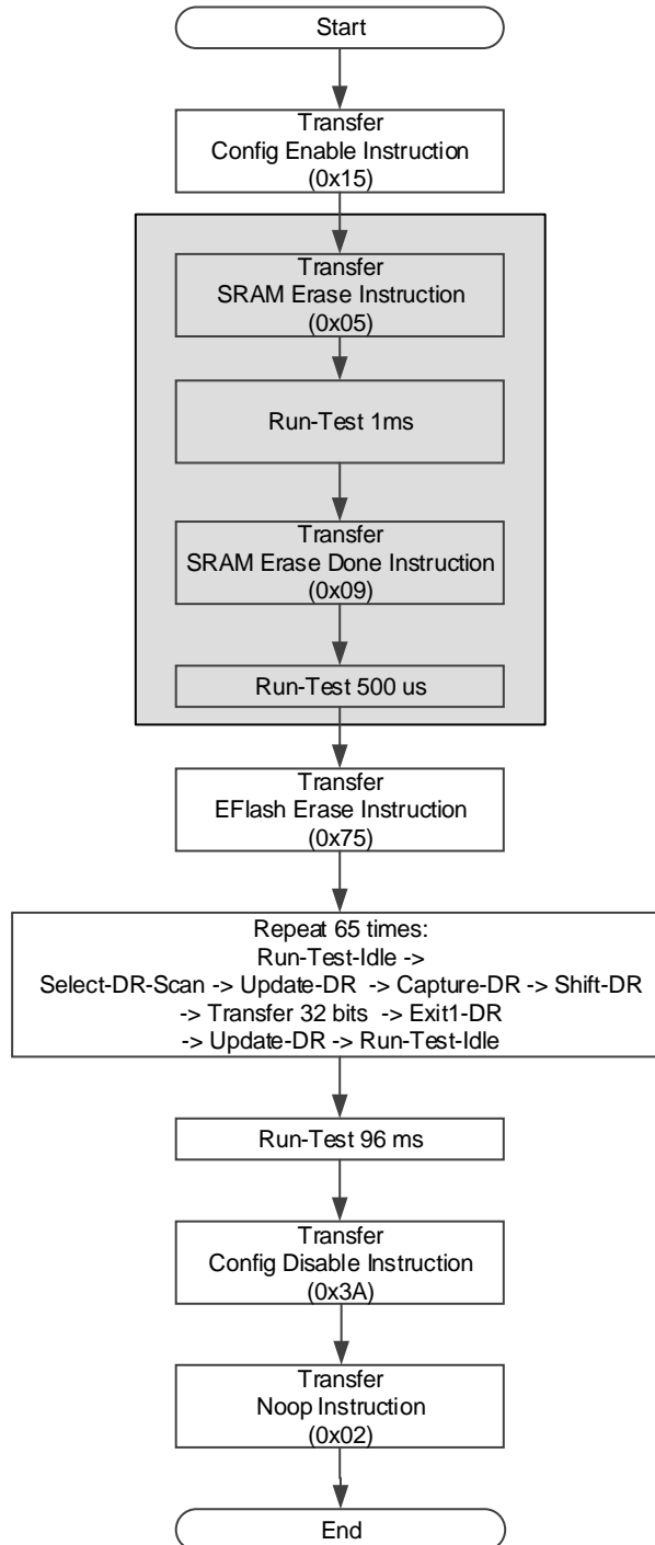
图 5-16 擦除 S 工艺 FPGA 内部 Flash 流程
