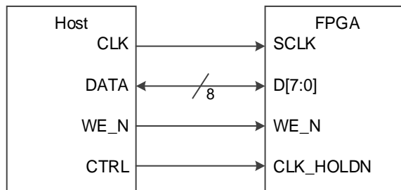
图 5-48 CPU 配置模式连接示意图
