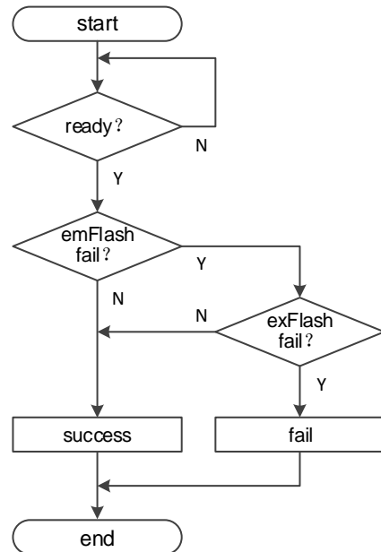
图 5-47 双启动配置模式流程图
