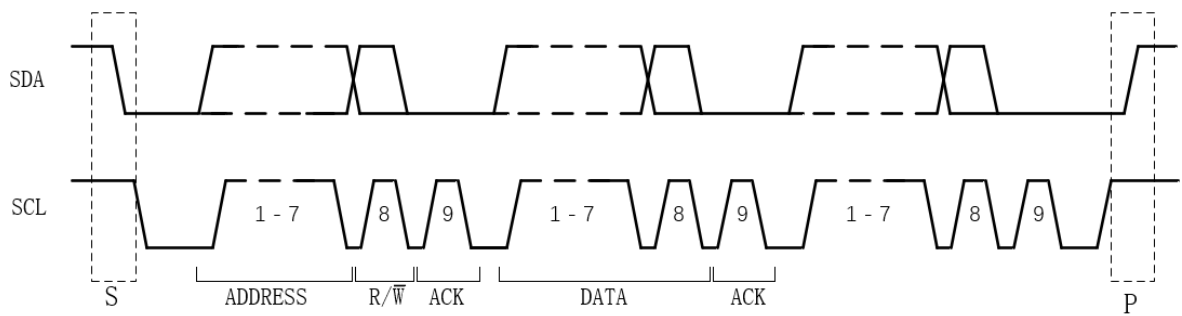
图 5-53 I 2 C 配置模式时序图
