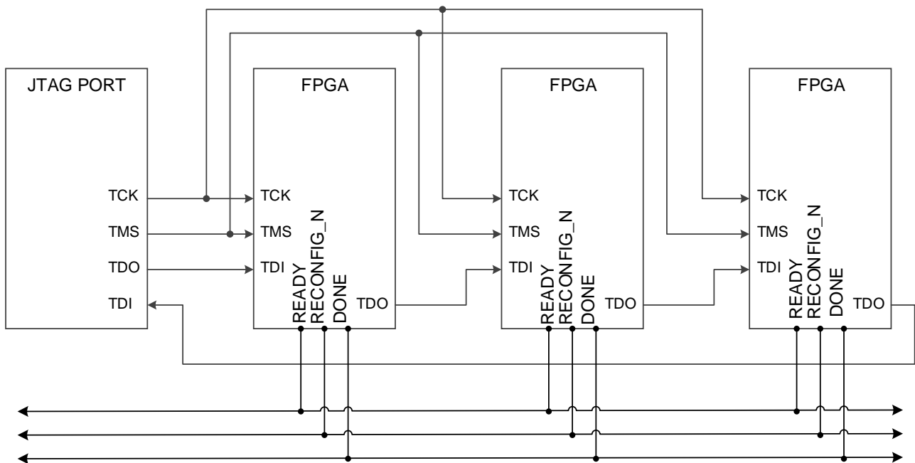
图 5-29 菊花链连接示意图
