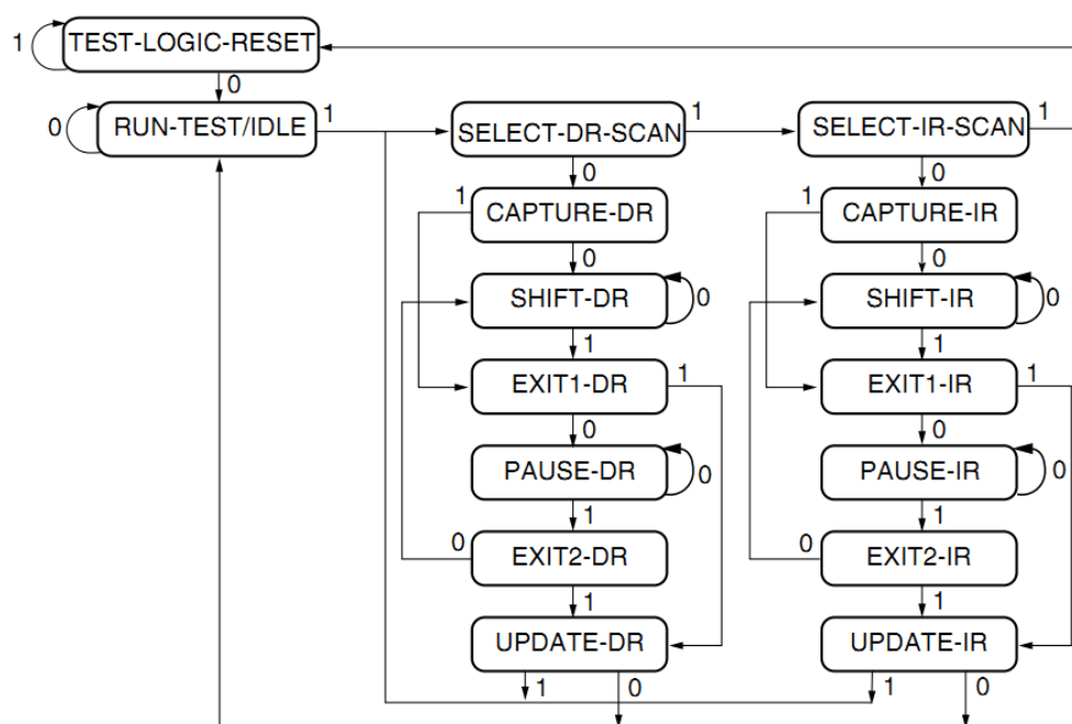
图 5-7 TAP 状态机
