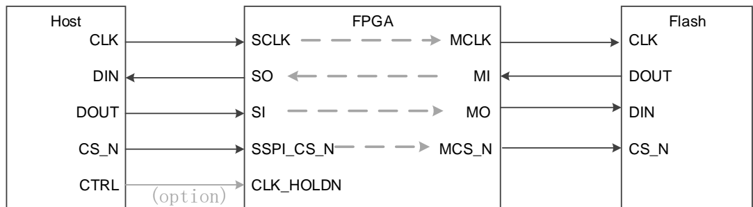
图 5-36 SSPI 编程外部 Flash 连接示意图
