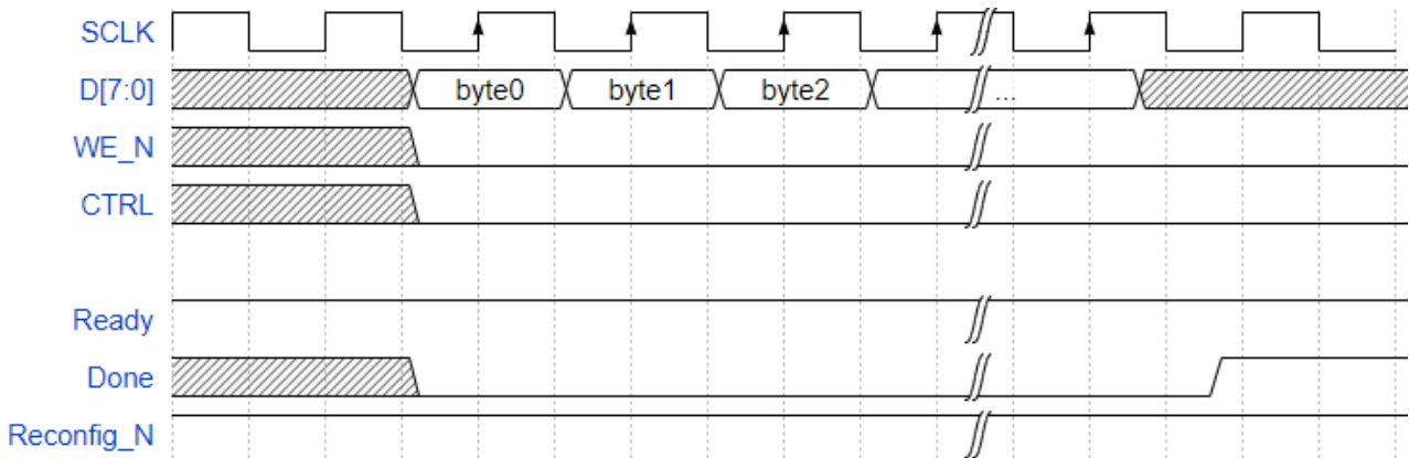
图 5-49 CPU Mode 配置时序示意图
