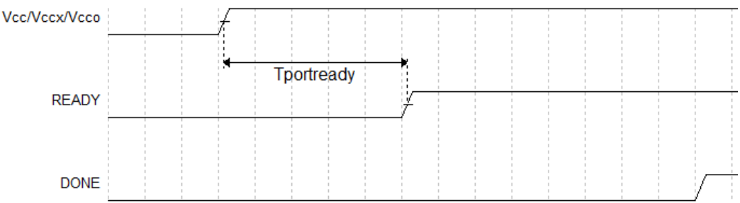
图 6-2 重新上电时序图
