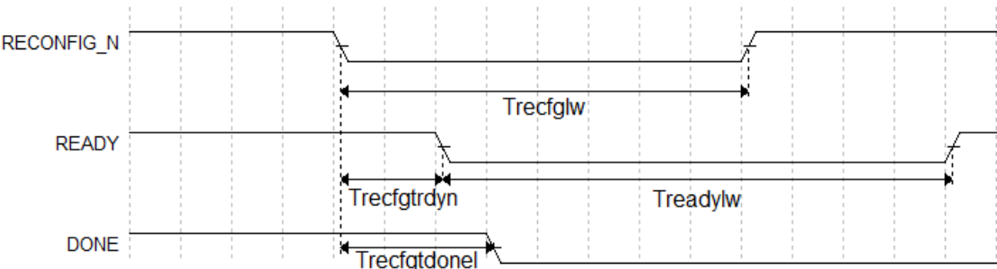
图 6-3 触发时序图
