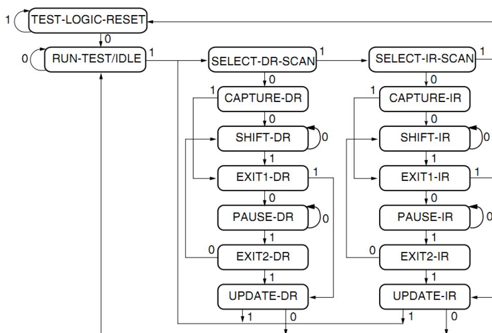
图 6-7 TAP 状态机
