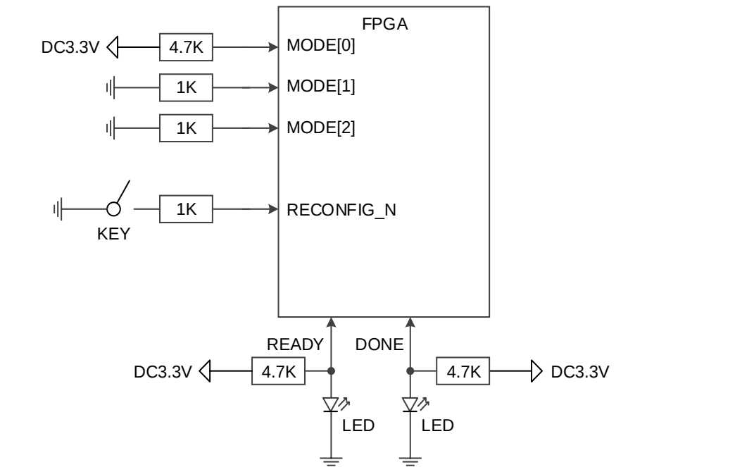
图 6-1 固定管脚推荐接法
