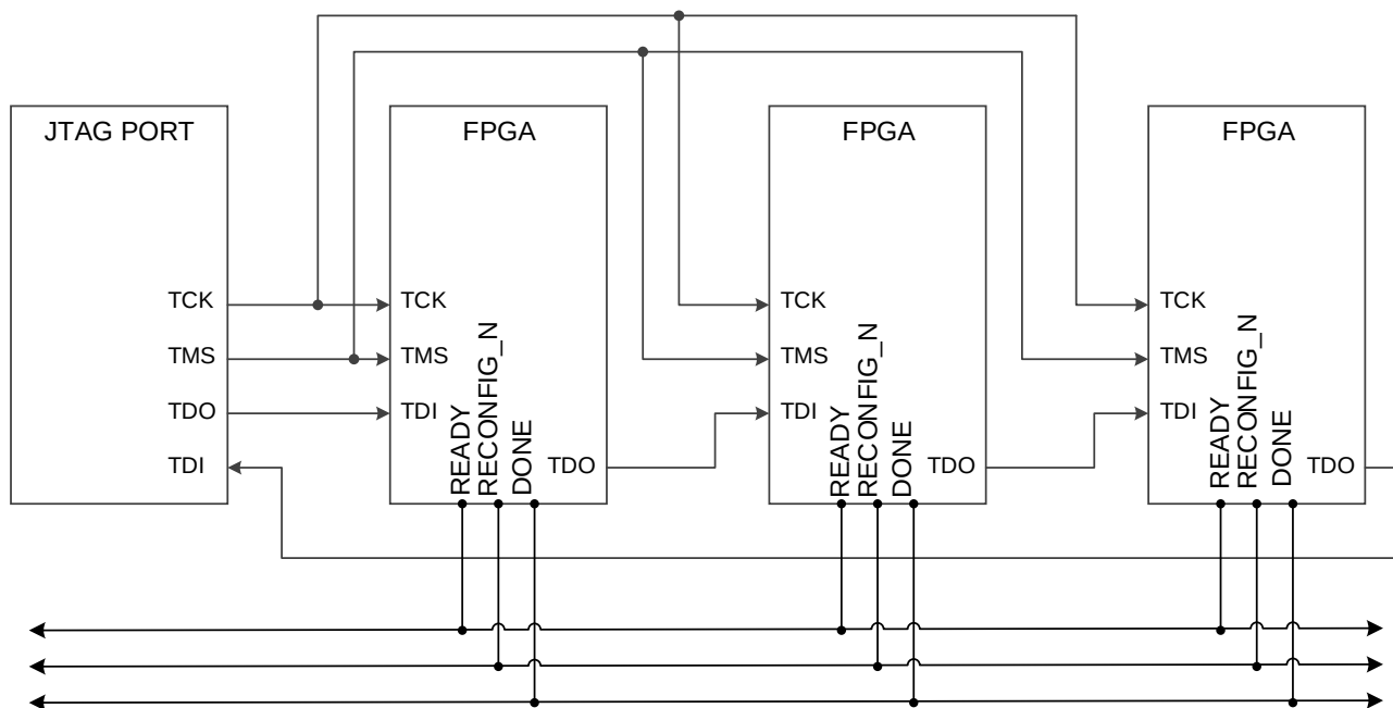
图 6-35 菊花链连接示意图
