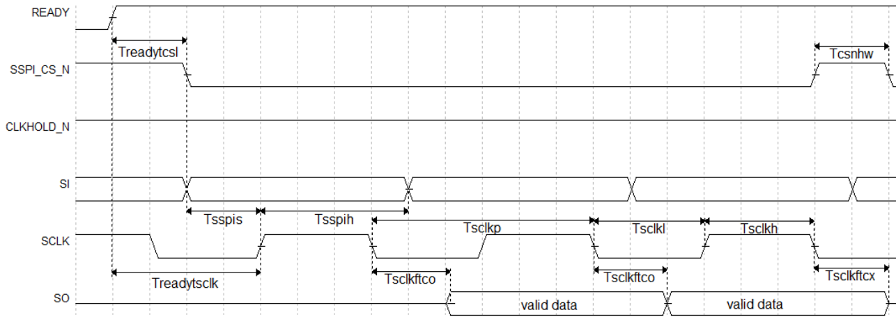
图 6-36 SSPI 配置模式时序图
