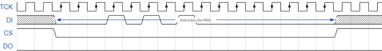
图 6-38 Write Enable（0x15）时序示意图
