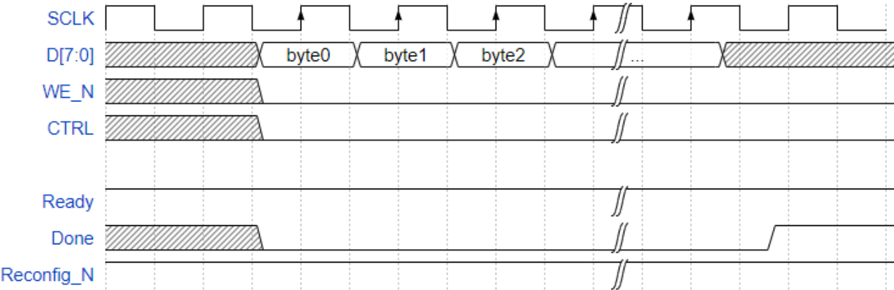
图 6-60 CPU 模式配置流程示意图
