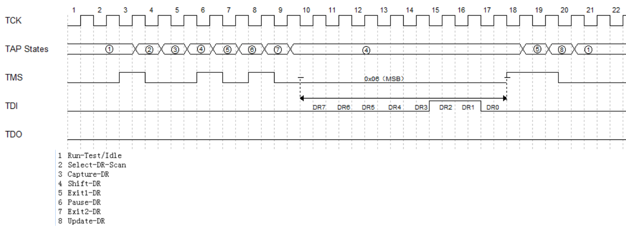
图 6-33 GW1N 系列 JTAG 模拟 SPI 发送 0x06 指令时序图
