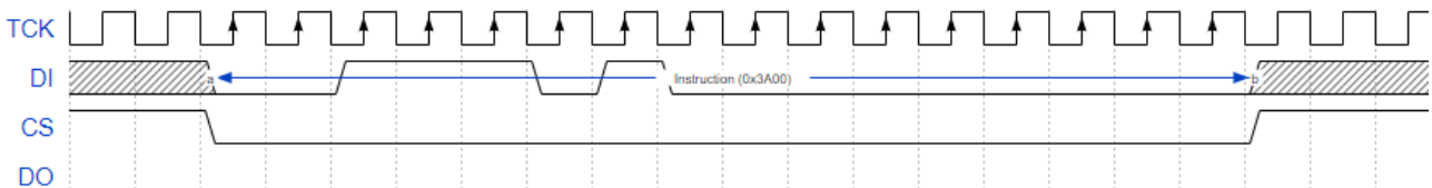
图 6-39 Write Disable (0x3A00) 时序示意图
