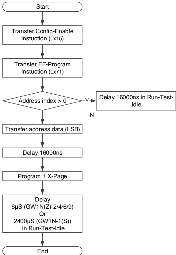
图 6-20 X-page 编程流程图
