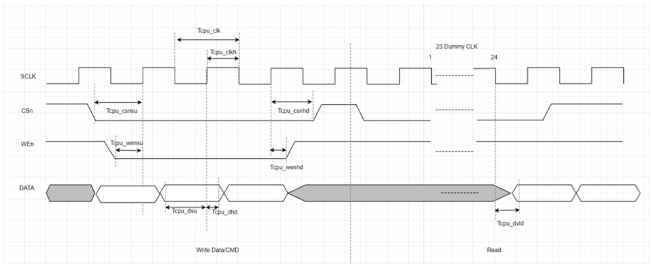
图 6-61 CPU 配置模式时序图
